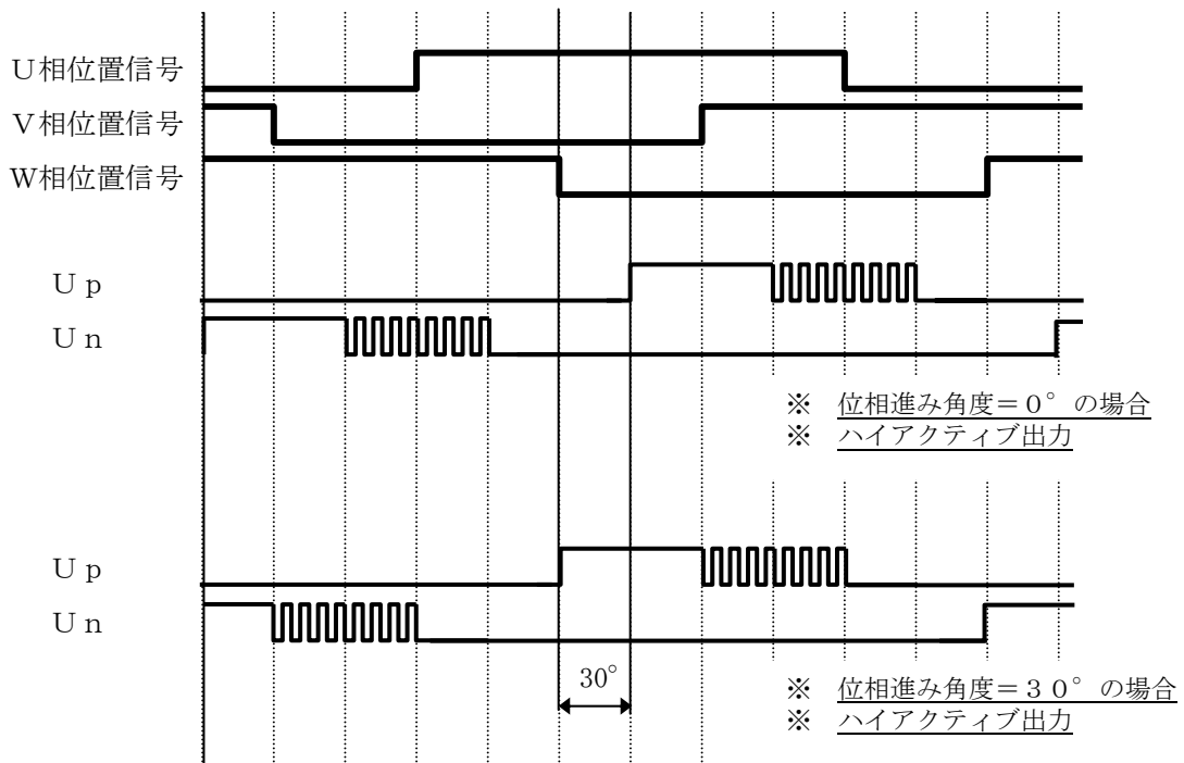
図 3.3.7 位相進み角度
