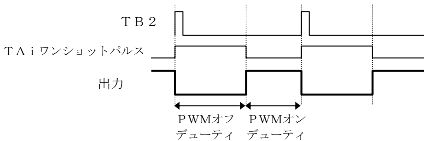
図 3.3.9 PWM デューティ
