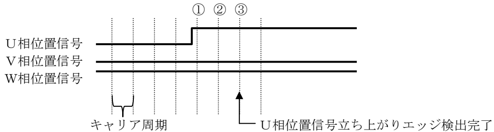
図 3.3.5 位置信号のエッジ検出方法
