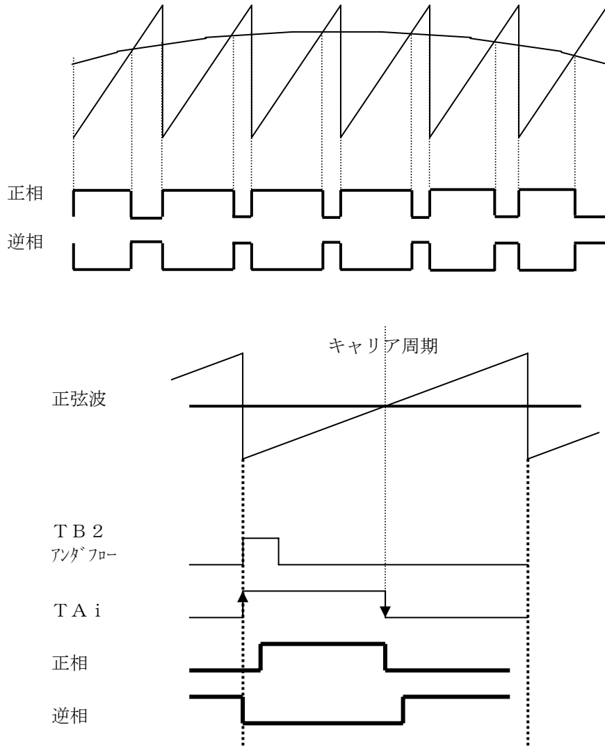
図 3.2.4 短絡防止時間を設定した場合の鋸波変調時のタイマとPWMの関係
