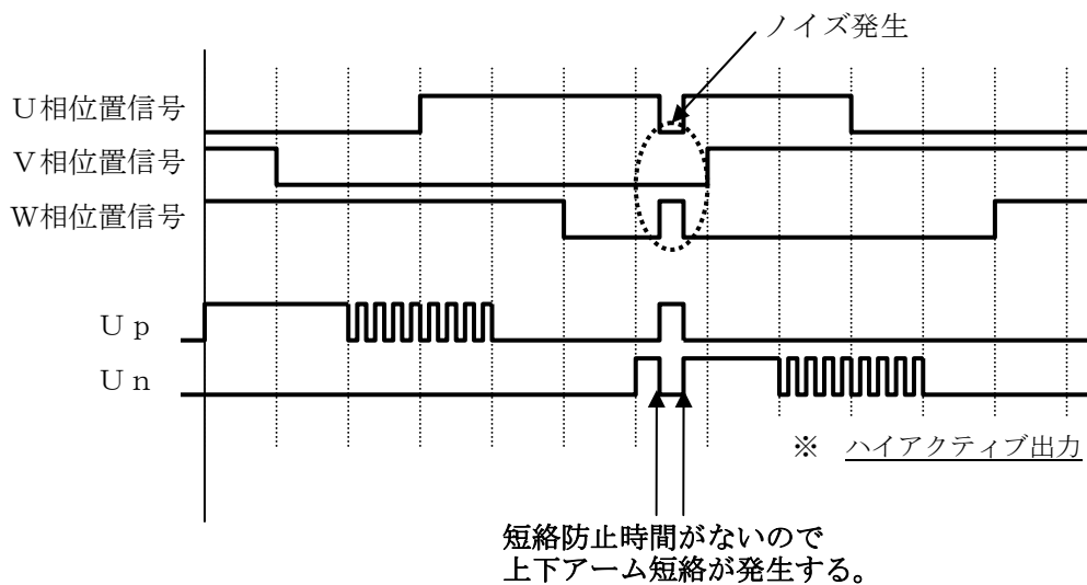
図 3.3.10 位置信号誤検出による上下アーム短絡について
