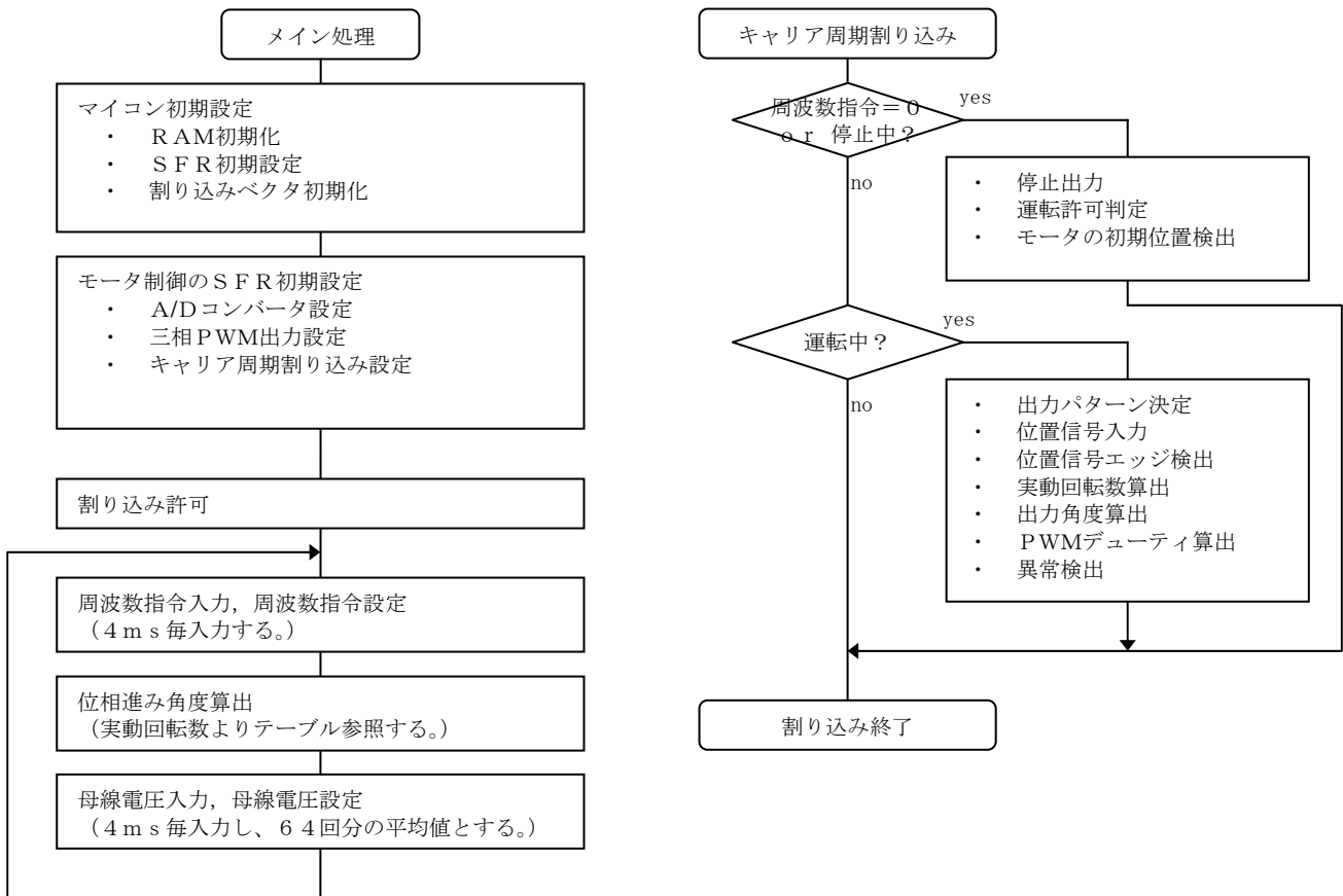
図 3.1.4 概略フロー図
