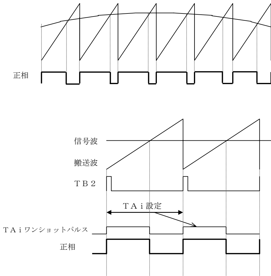
図 3.2.3 キャリアの変調方式
