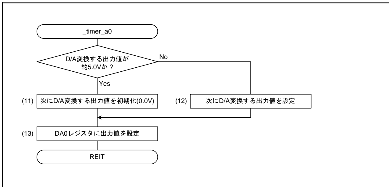
図 3.3 タイマA0割り込み関数のフローチャート
