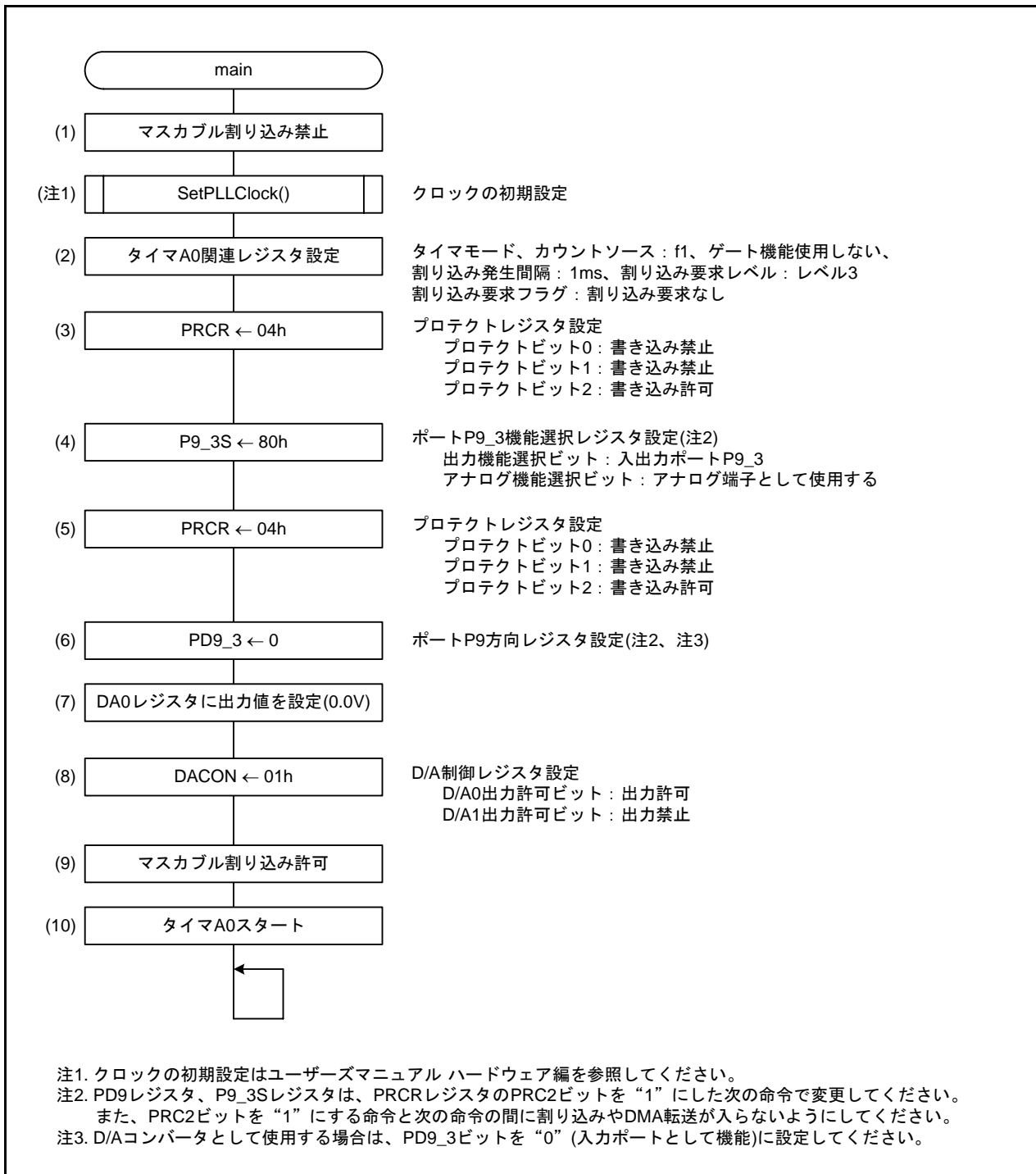
図 3.2 メイン関数のフローチャート
