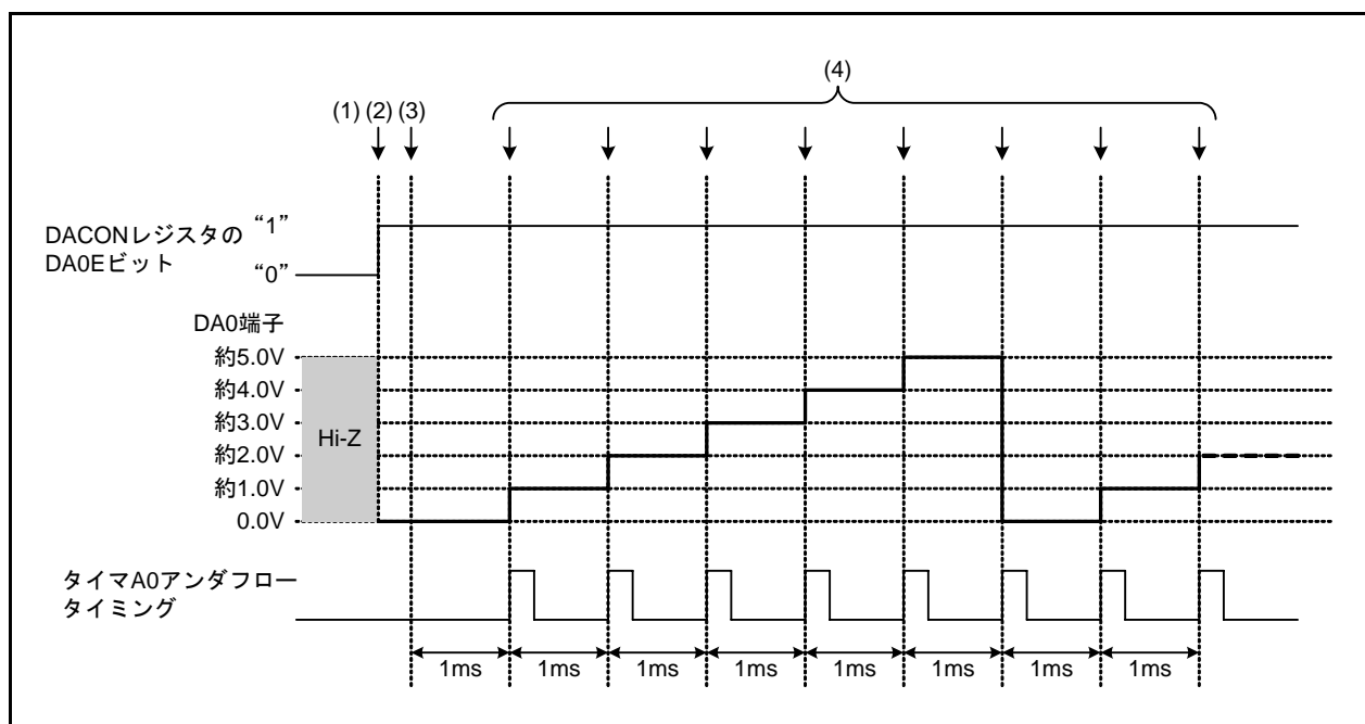
図 3.1 D/Aコンバータの動作例
