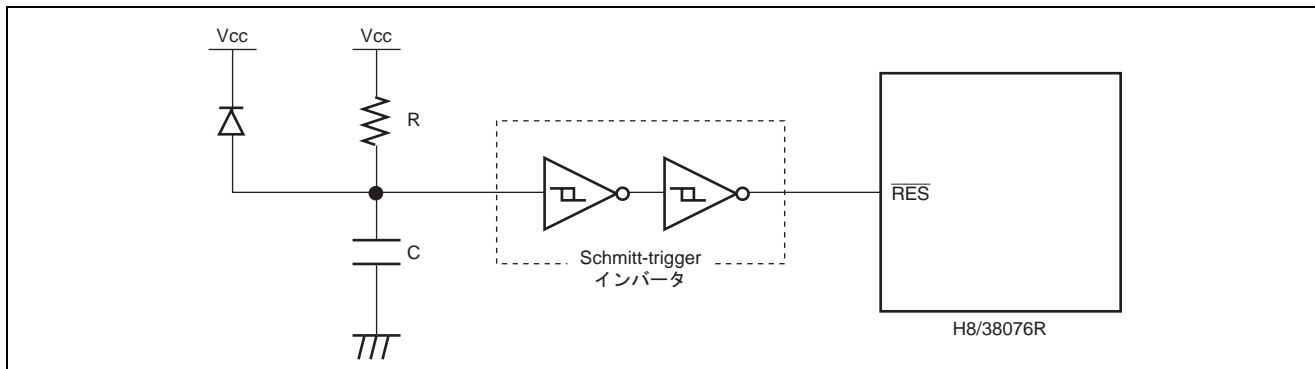
図1 外部リセット回路によるパワーオンリセット動作
