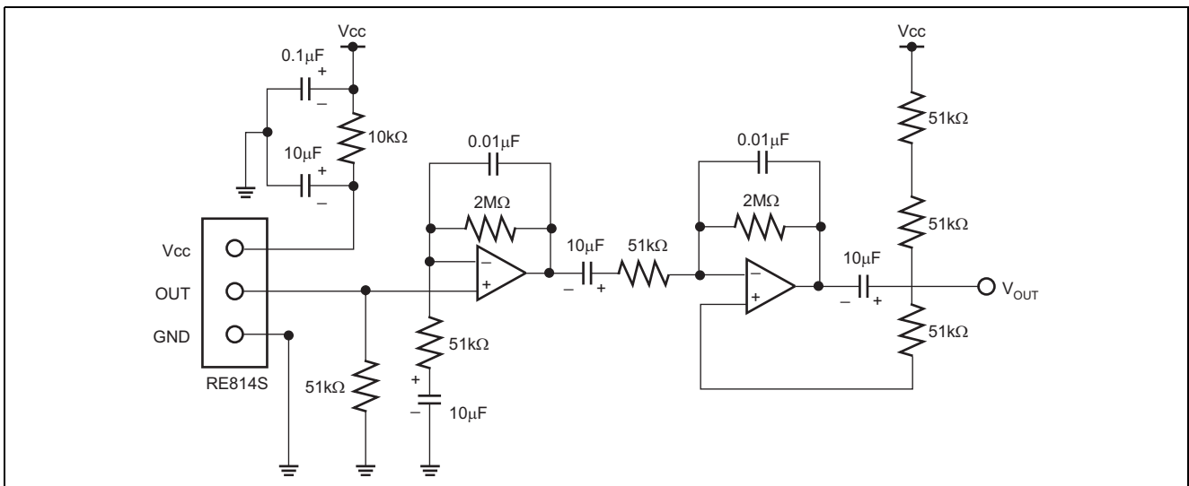
図 1.2 センサ出力アンプ回路例（参考）
