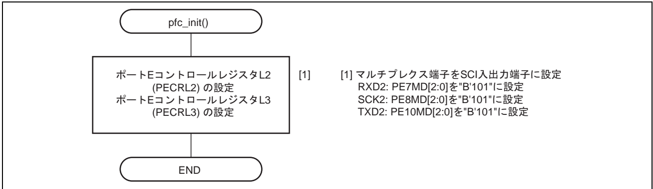
図7 ピンファンクションコントローラの設定フロー
