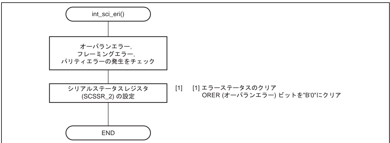
図10 クロック同期式モード受信エラー割り込み処理フロー
