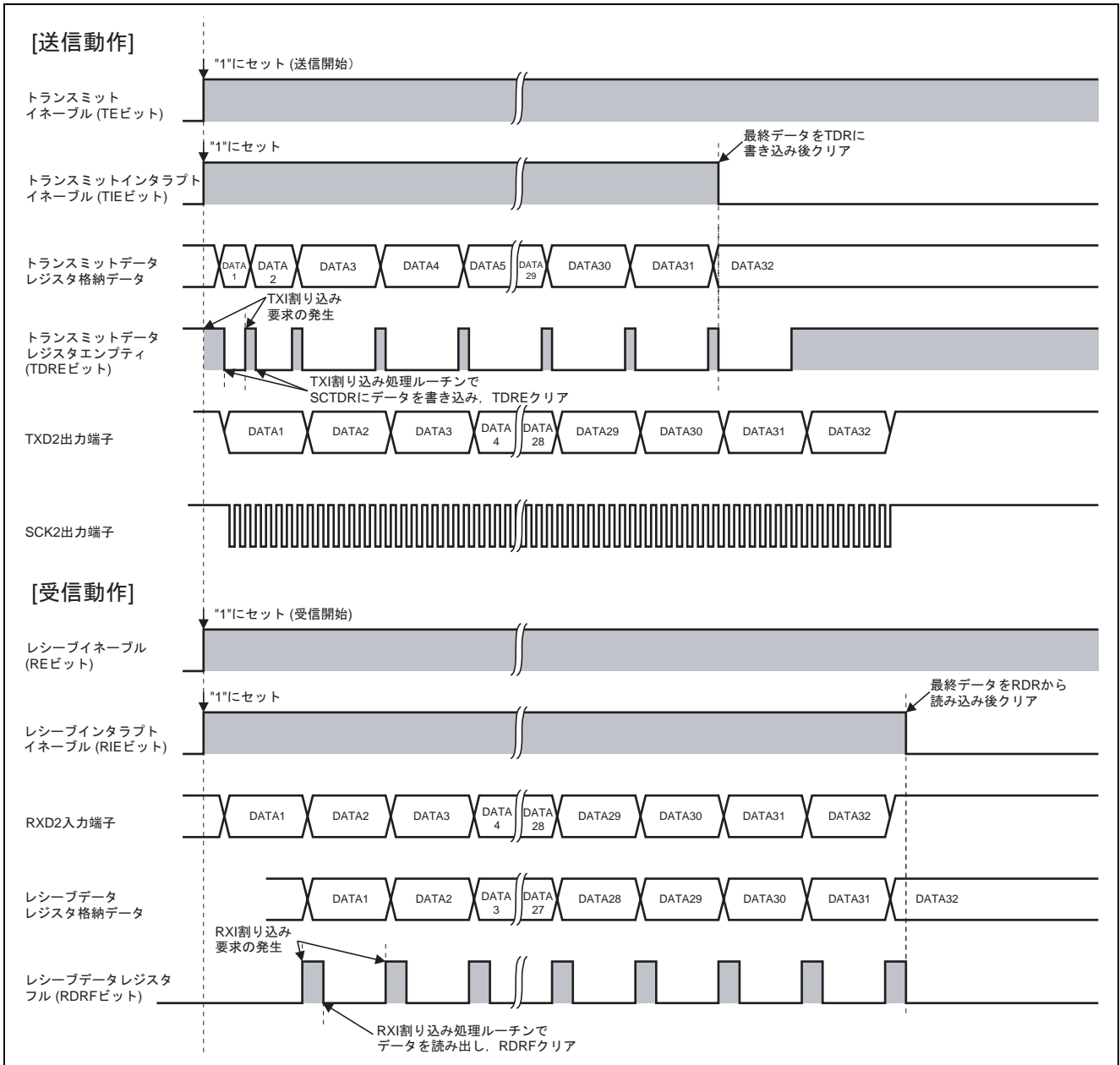
図3 動作説明図
