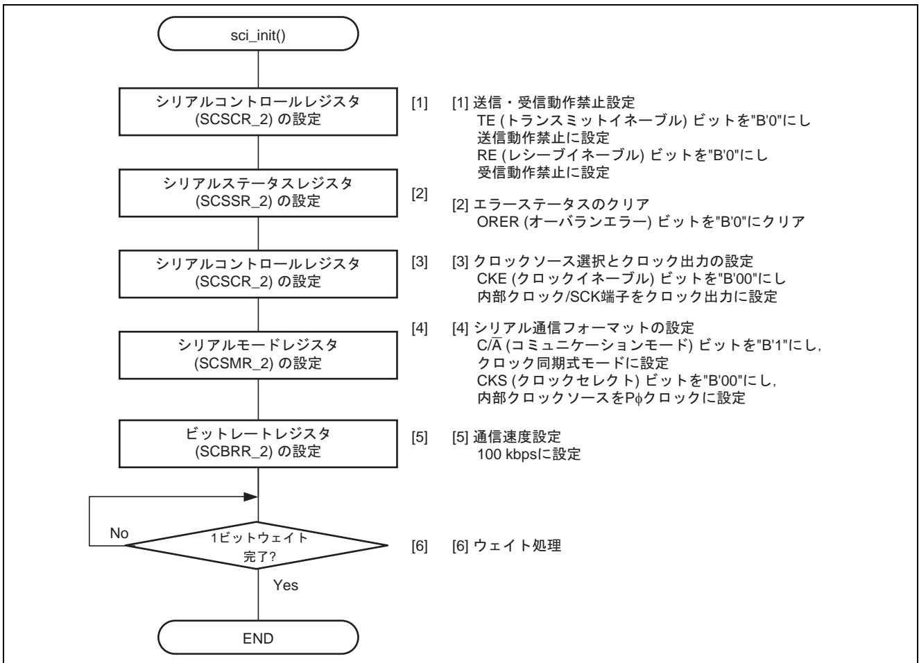
図6 クロック同期式モード送受信初期設定フロー
