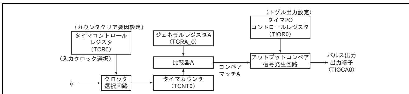
図 2 パルス出力ブロック図
