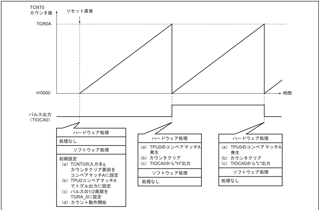
図3 パルス出力動作原理
