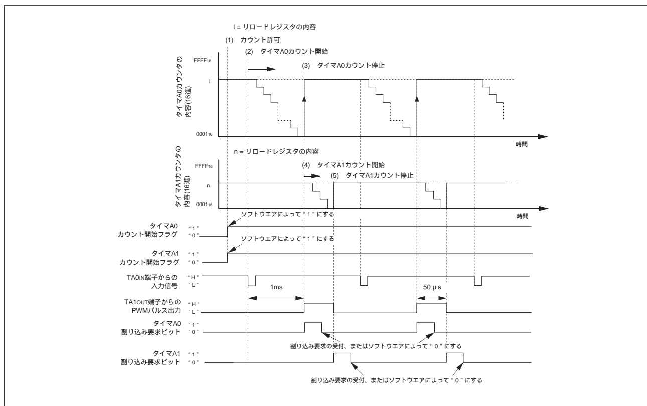
図2 ディレードワンショット出力の動作タイミング
