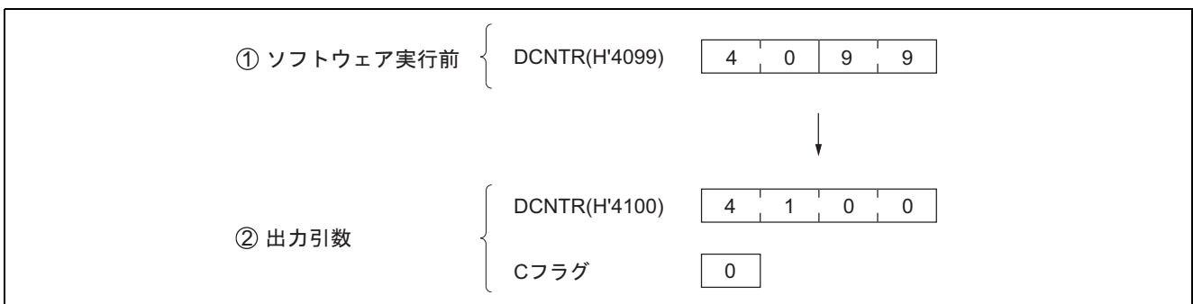
図 11-1 ソフトウェア DECNT の実行例
