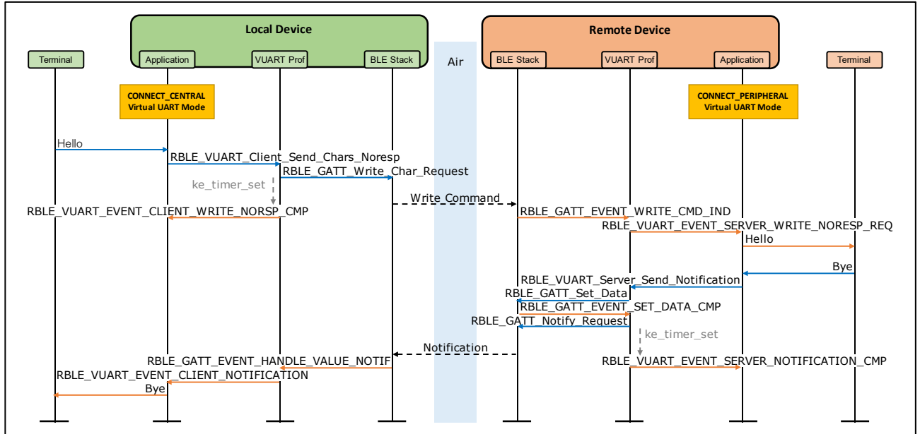
図 8-5 データ送受信シーケンス(Write Command/Notification)
