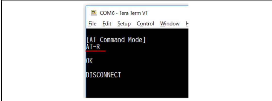
図 9-21 仮想 UART サーバからの切断
