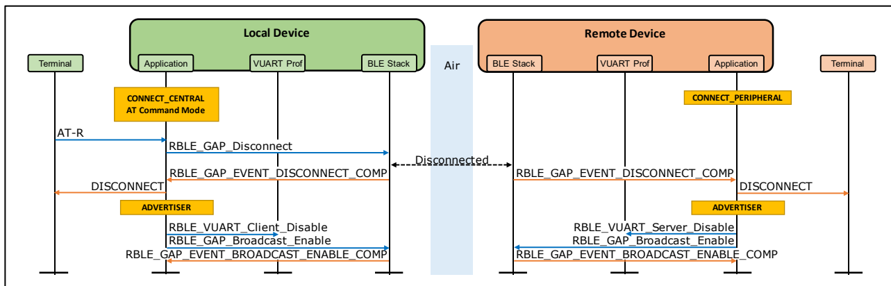
図 8-6 切断シーケンス
