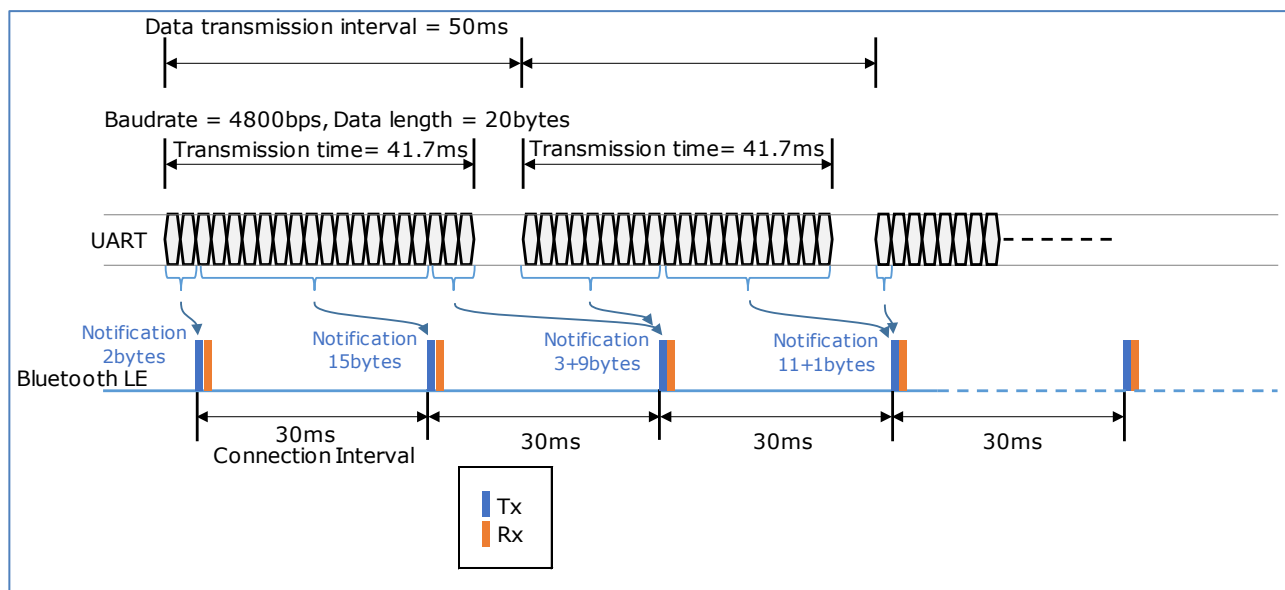
図 8-8 ターミナルからのデータ受信と Notification 送信例
