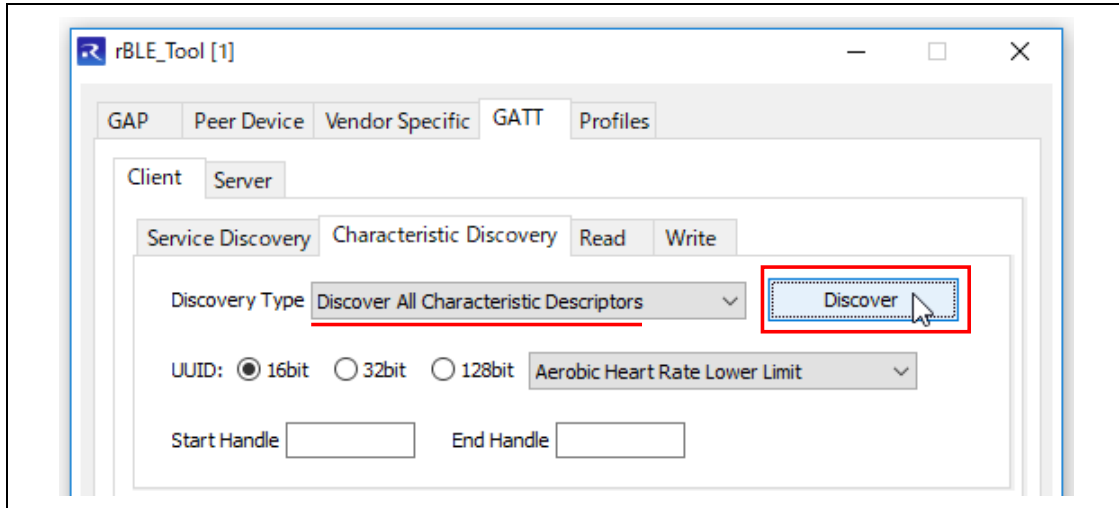
図 9-13 ディスクリプタ検索
