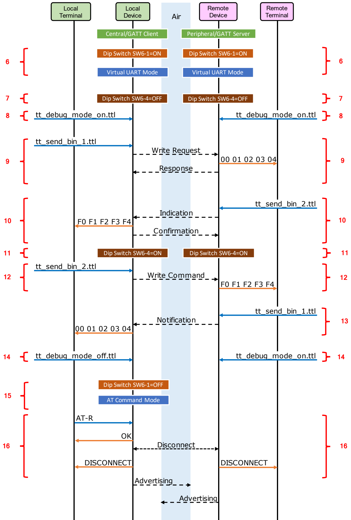
図 7-6 バイナリデータ送受信 実行例のシーケンス (2/2)
