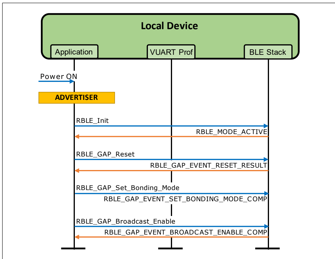
図 8-2 起動シーケンス
