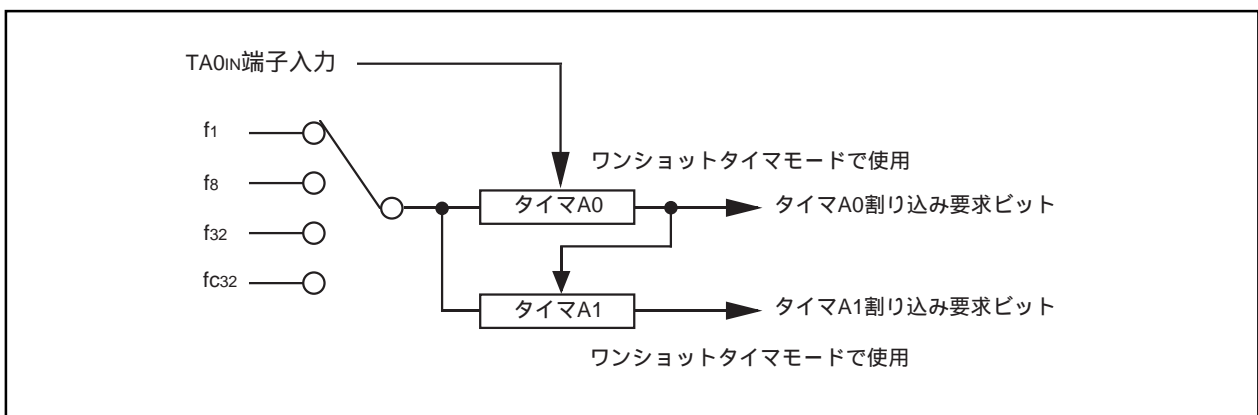
図2 ディレードワンショット出力のタイマ接続図
