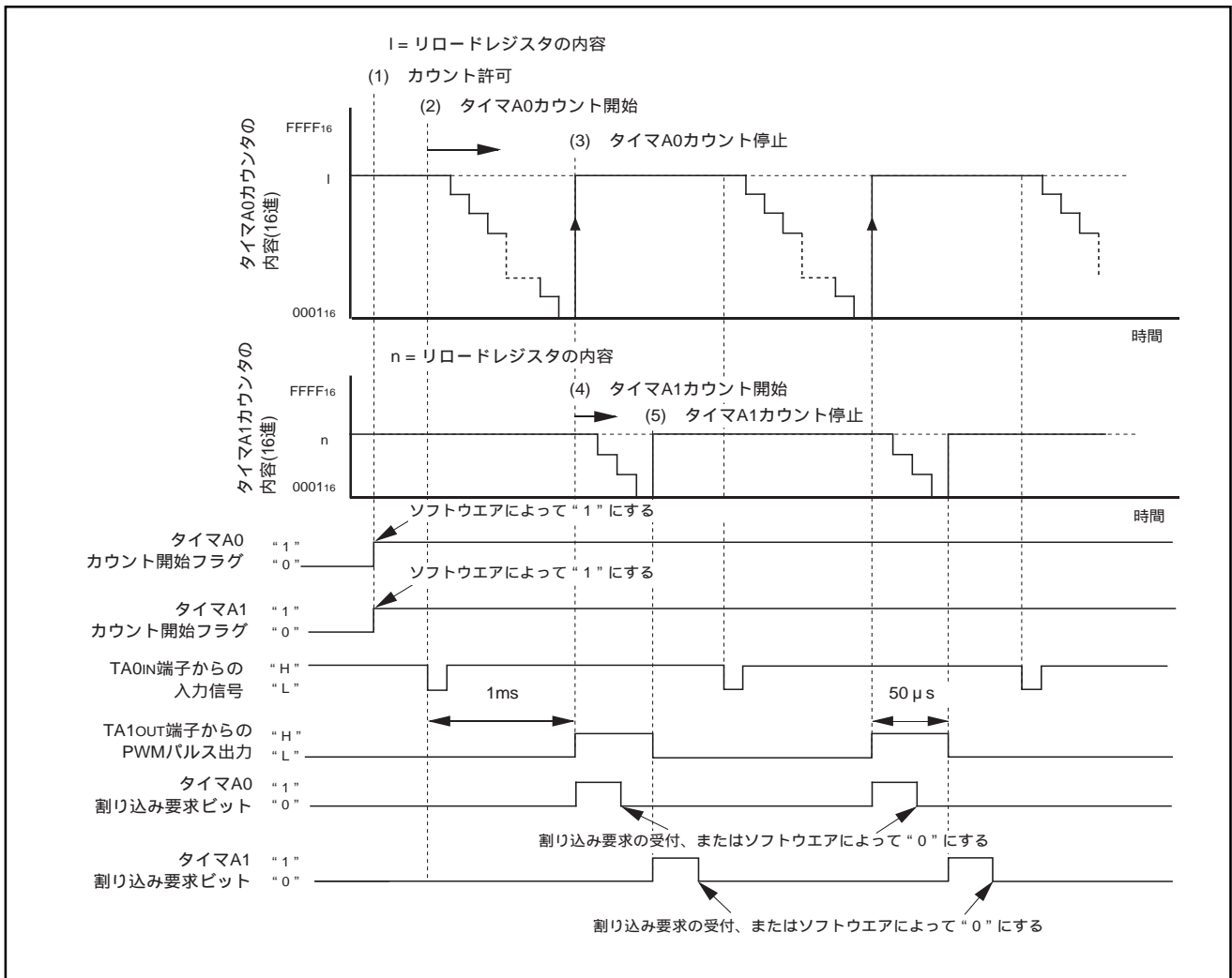
図1 ディレードワンショット出力の動作タイミング
