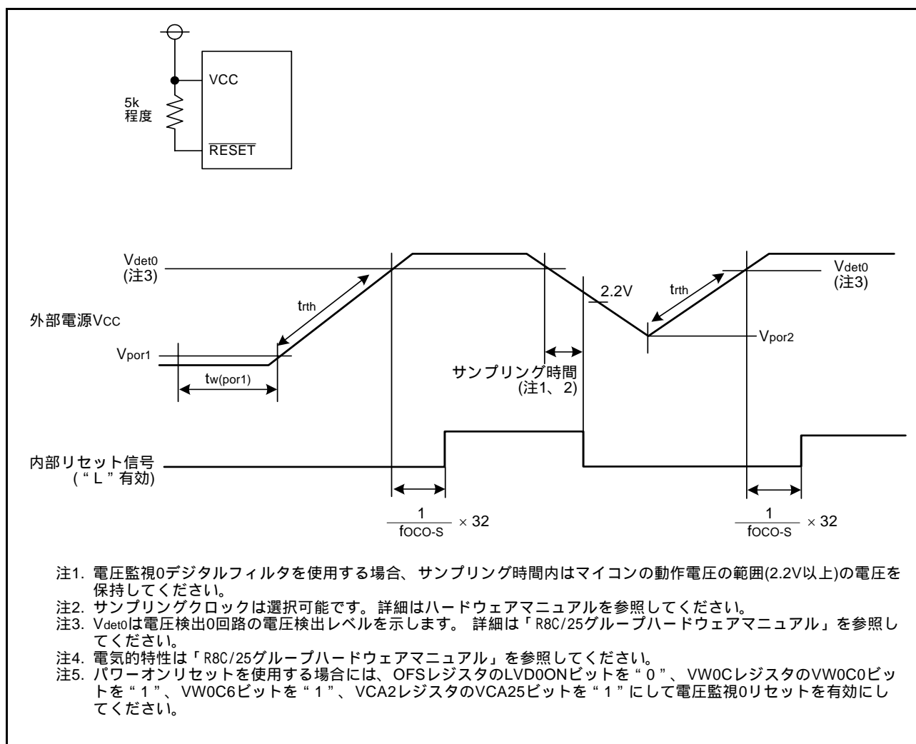
図 3.3 パワーオンリセット回路例と動作
