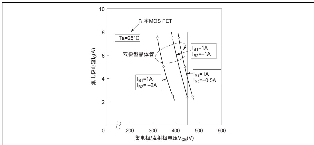
图 33 反向偏压 ASO
