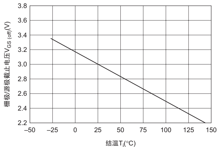
图 4 相对于结温的 V_{GS(off)} 变化
