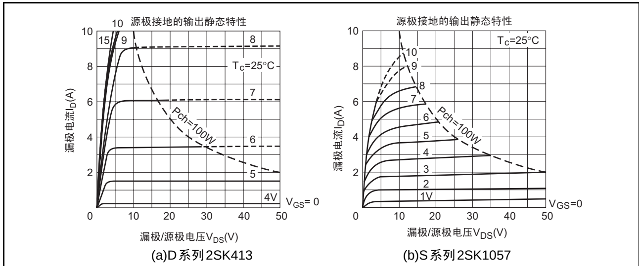
图6 功率 MOS FET 的输出静态特性
