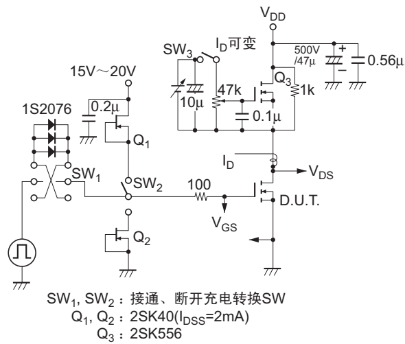
N-ch测量电路
