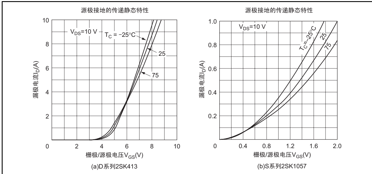
图34 传递静态特性
