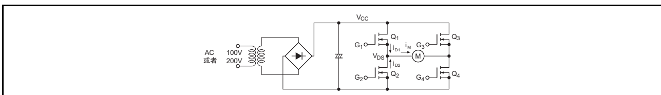
图 40 马达控制的基本电路
