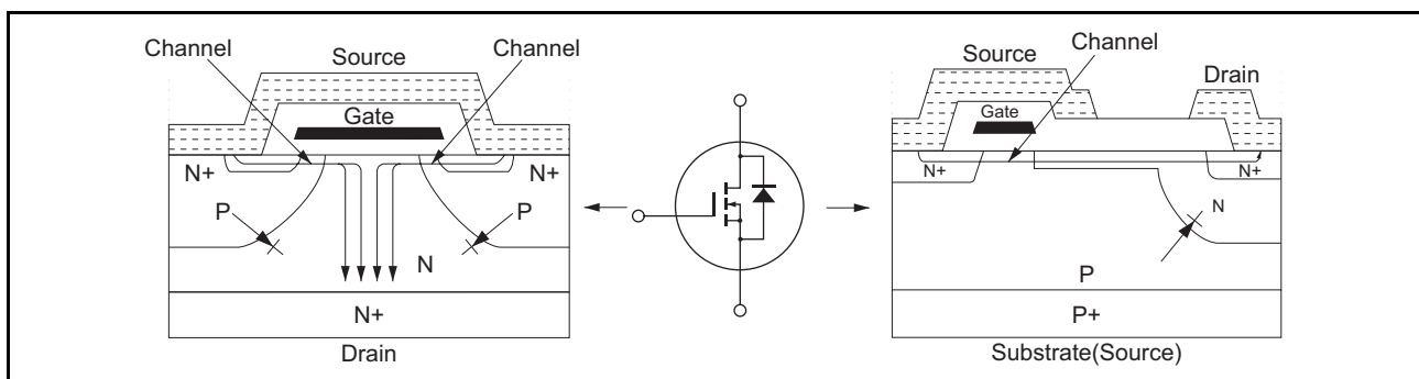
图35 D系列 (纵向) 的结构 (N沟道)
