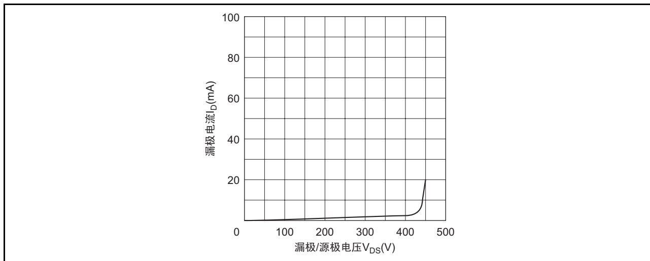
图 45 击穿特性
