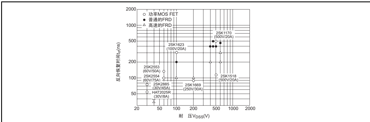
图 39 内部二极管与FRD的 t_{rr} 比较
