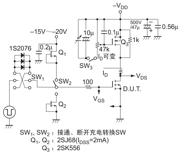
P-ch测量电路
