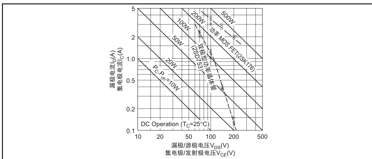
图29 功率MOS FET的破坏强度
