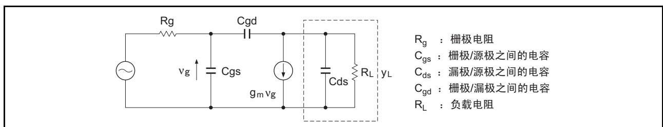
图7 饱和区域的等效电路
