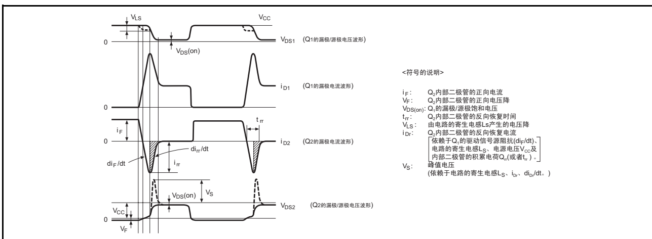
图 41 马达控制工作时的波形
