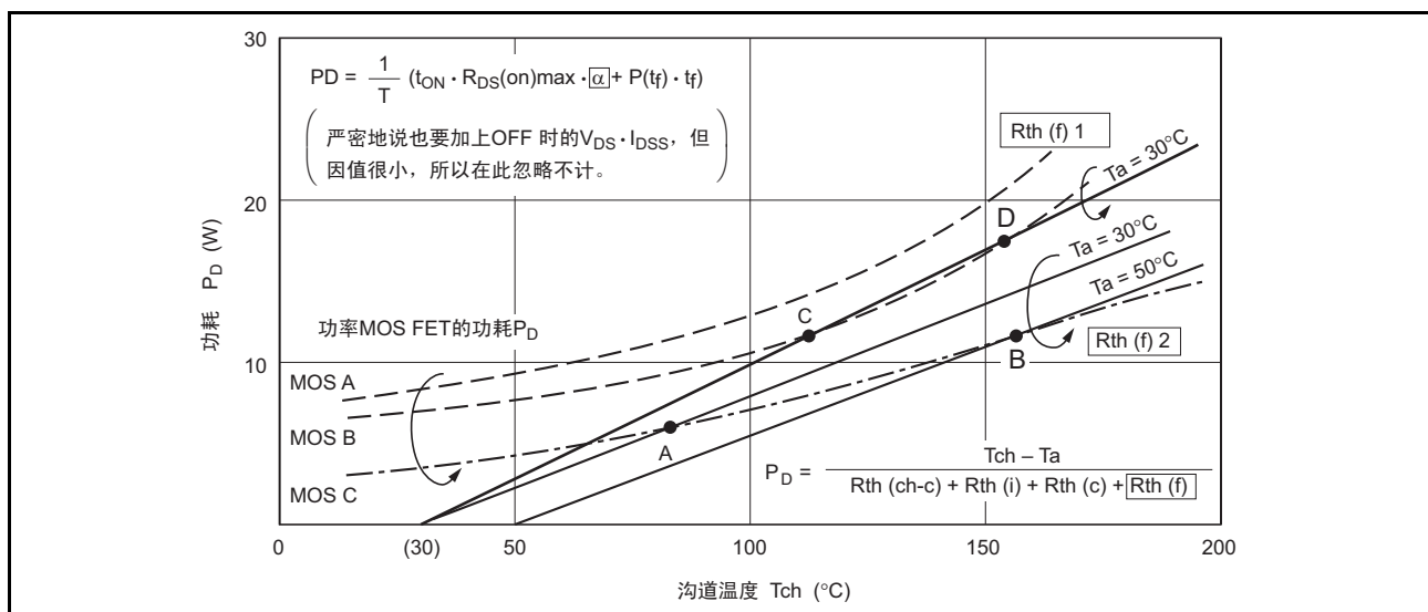
图56 沟道温度Tch与功耗 P_D 的关系
