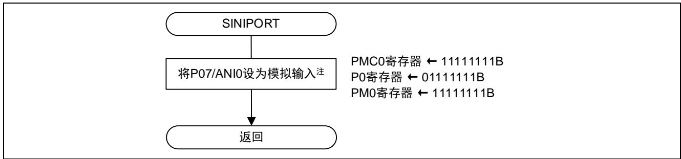
图 4.3 设置 I/O 端口的函数
