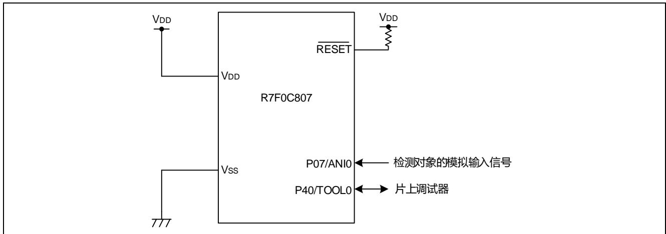
图 3.1 硬件配置
