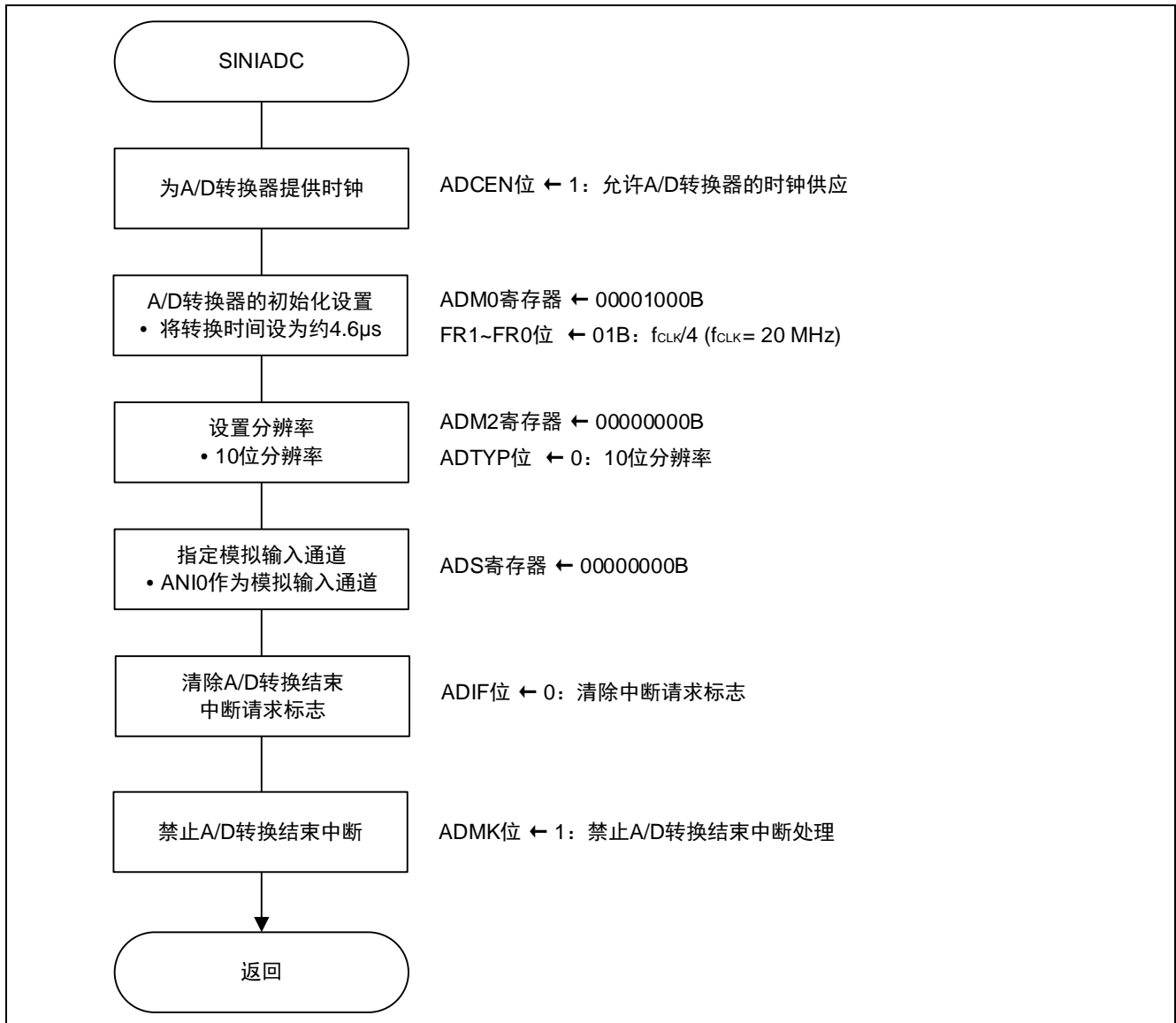
图 4.5 设置 A/D 转换器
