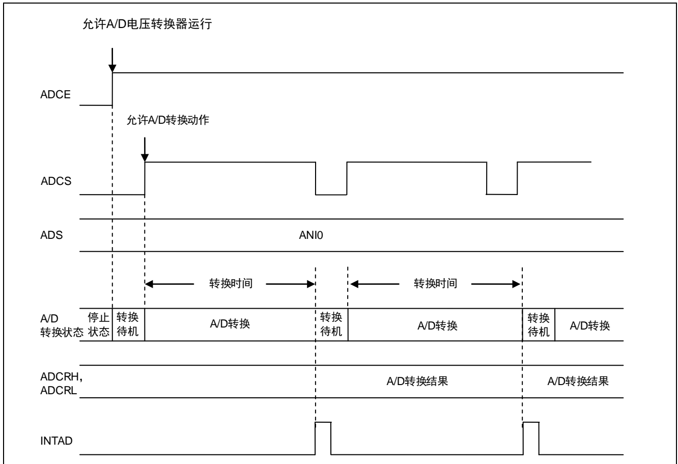
图 1.1 A/D 转换器的转换处理
