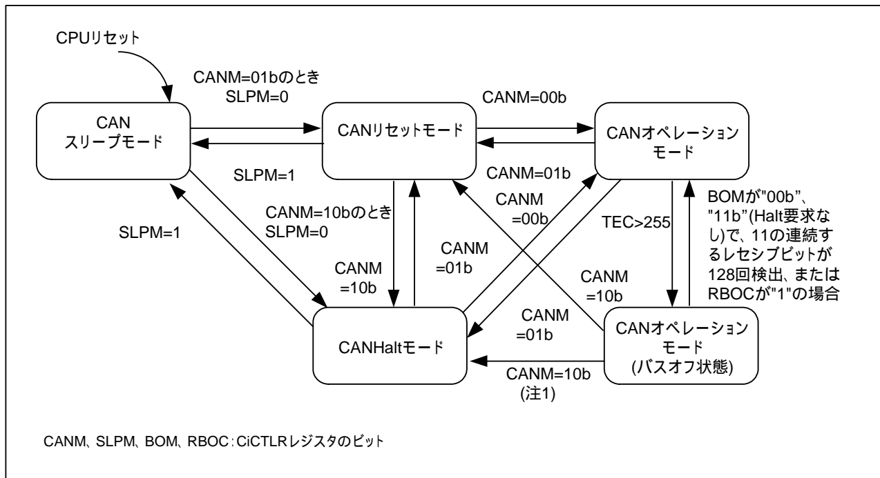
図 1. CAN 動作モード間の状態遷移
