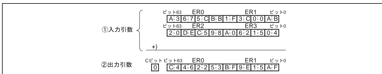
図 1 ソフトウェア ADD の実行例
