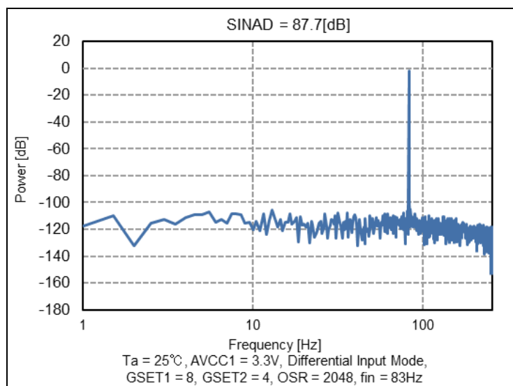
図 18 周波数と出力の対比 ( G_{SET1} = 8 、 G_{SET2} = 4 、 OSR = 2048 )
