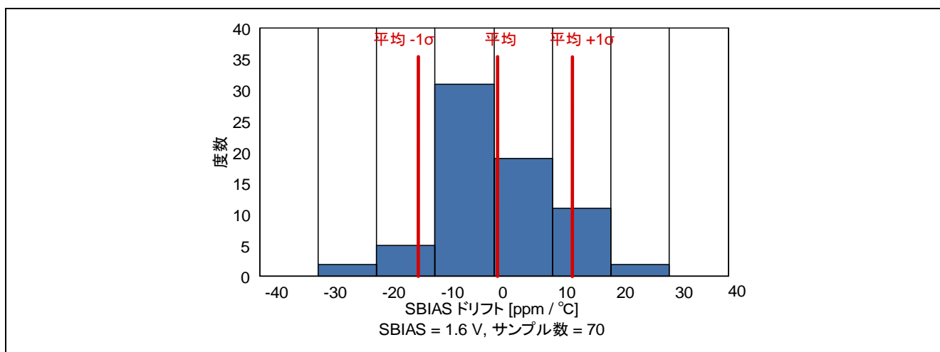
図 22 SBIAS ドリフトのヒストグラム
