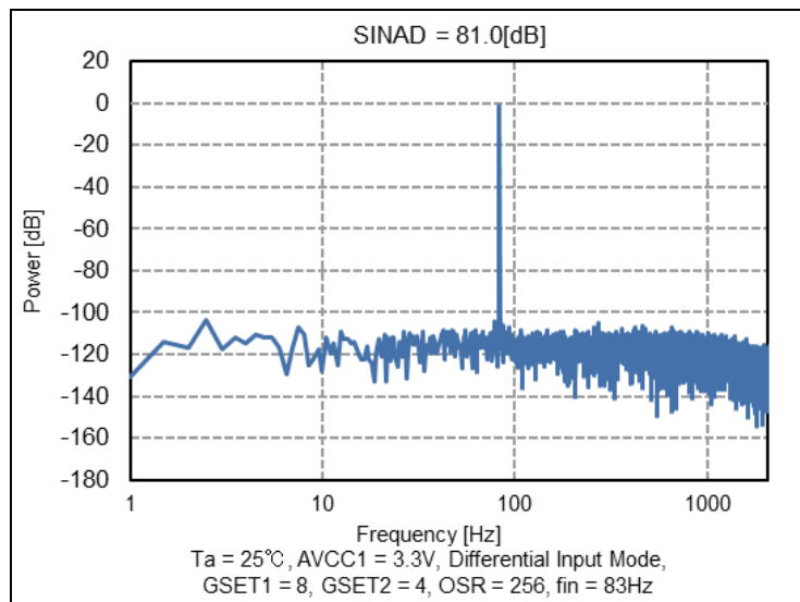
図 17 周波数と出力の対比 ( G_{SET1} = 8 、 G_{SET2} = 4 、 OSR = 256 )
