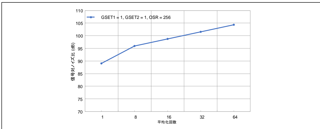
図 19 SNR と平均化回数の対比
