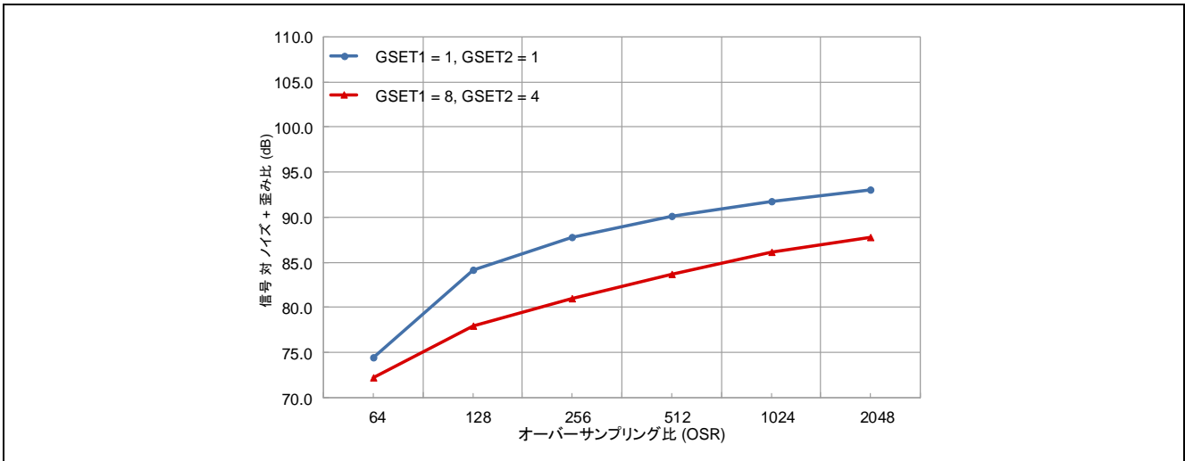
図 8 SINAD と OSR の対比
