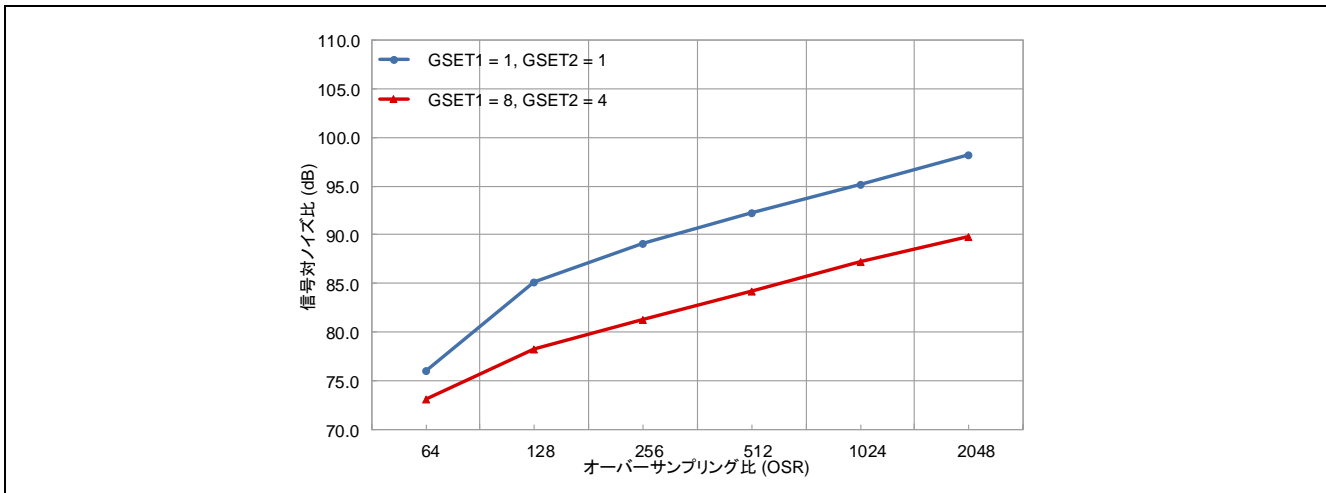
図 7 SNR と OSR の対比
