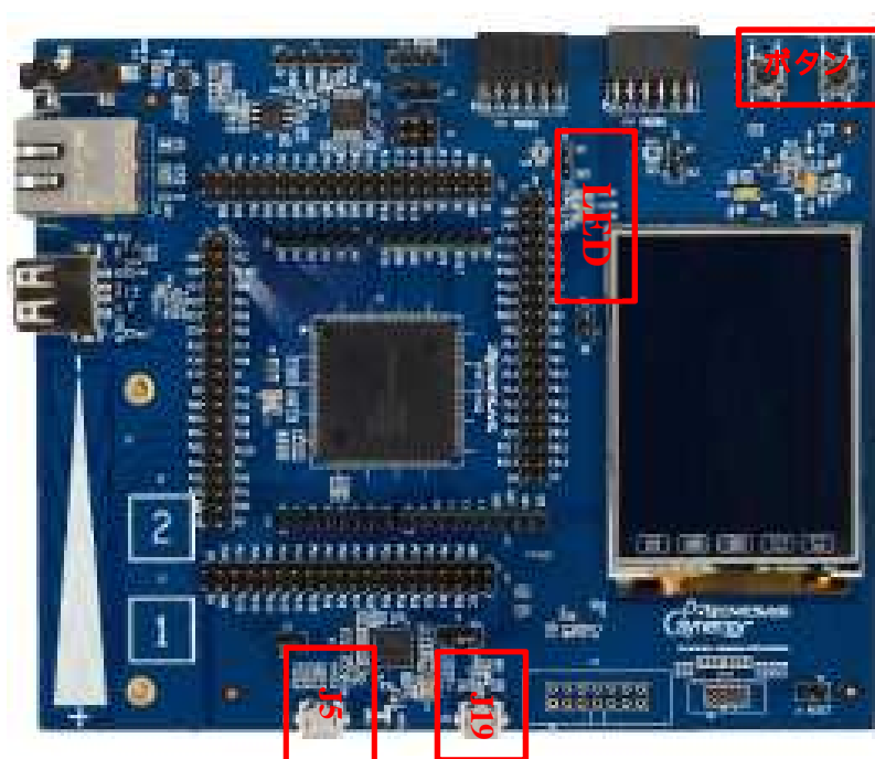
図 1 : 機能の配置
