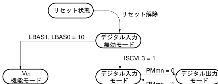
図16-8 V L3 /P125端子機能の状態遷移図
