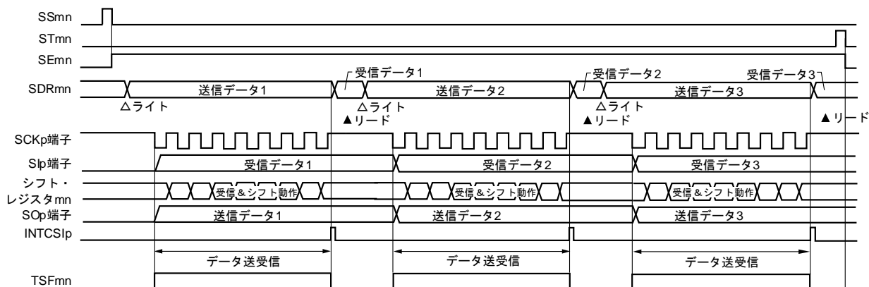
図14-67 スレーブ送受信（シングル送受信モード時）のタイミング・チャート（タイプ1：DAPmn = 0, CKPmn = 0）
