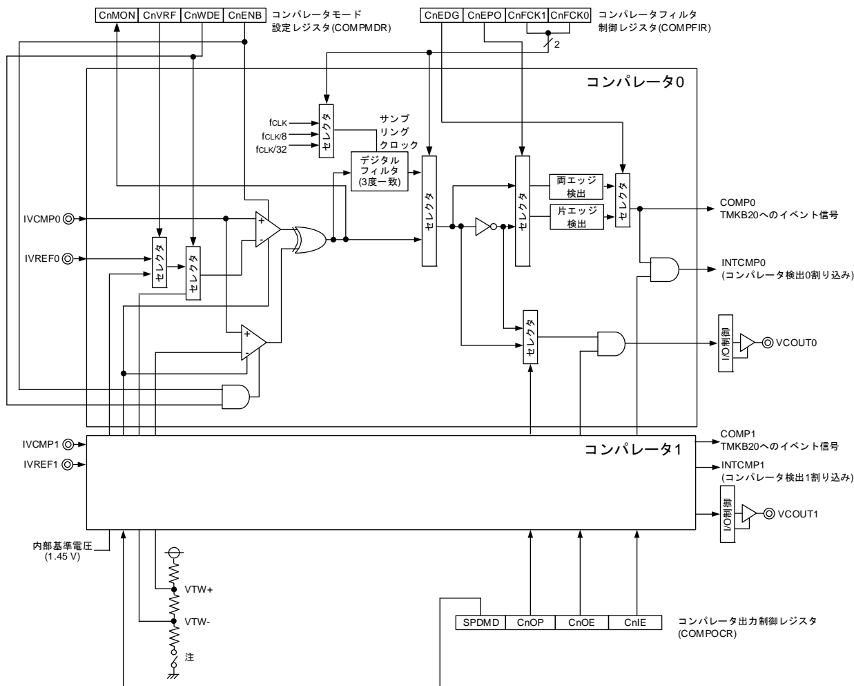
図13-1 コンパレータのブロック図
