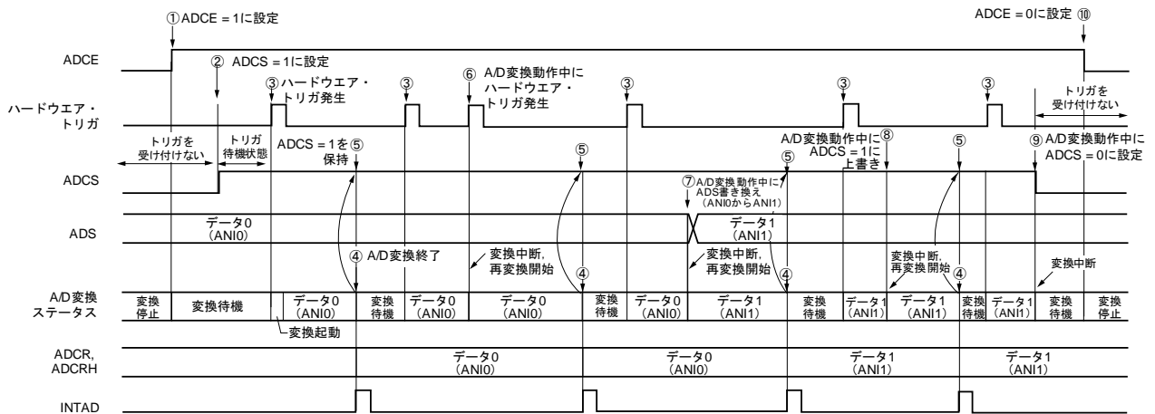
図12-20 ハードウェア・トリガ・ノーウエイト・モード（ワンショット変換モード）動作タイミング例
