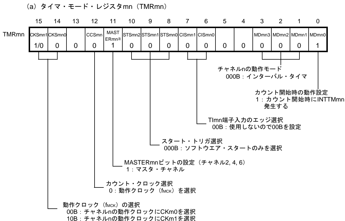
図6-70 PWM機能時（マスタ・チャンネル）のレジスタ設定内容例
