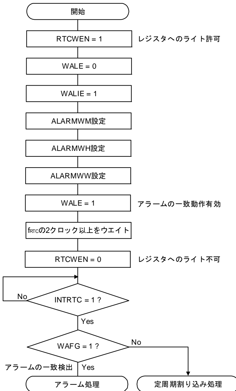
図8-24 アラーム設定手順
