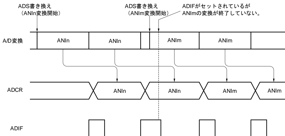
図12-39 A/D変換終了割り込み要求発生タイミング
