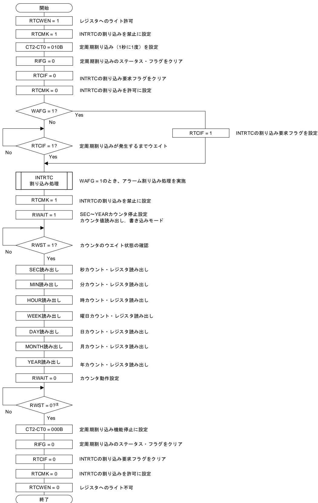
図8-21 リアルタイム・クロック2の読み出し手順（アラーム割り込み機能使用時）
