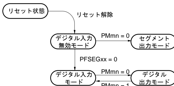
図4-12 SEGxx/ポート端子機能の状態遷移図
