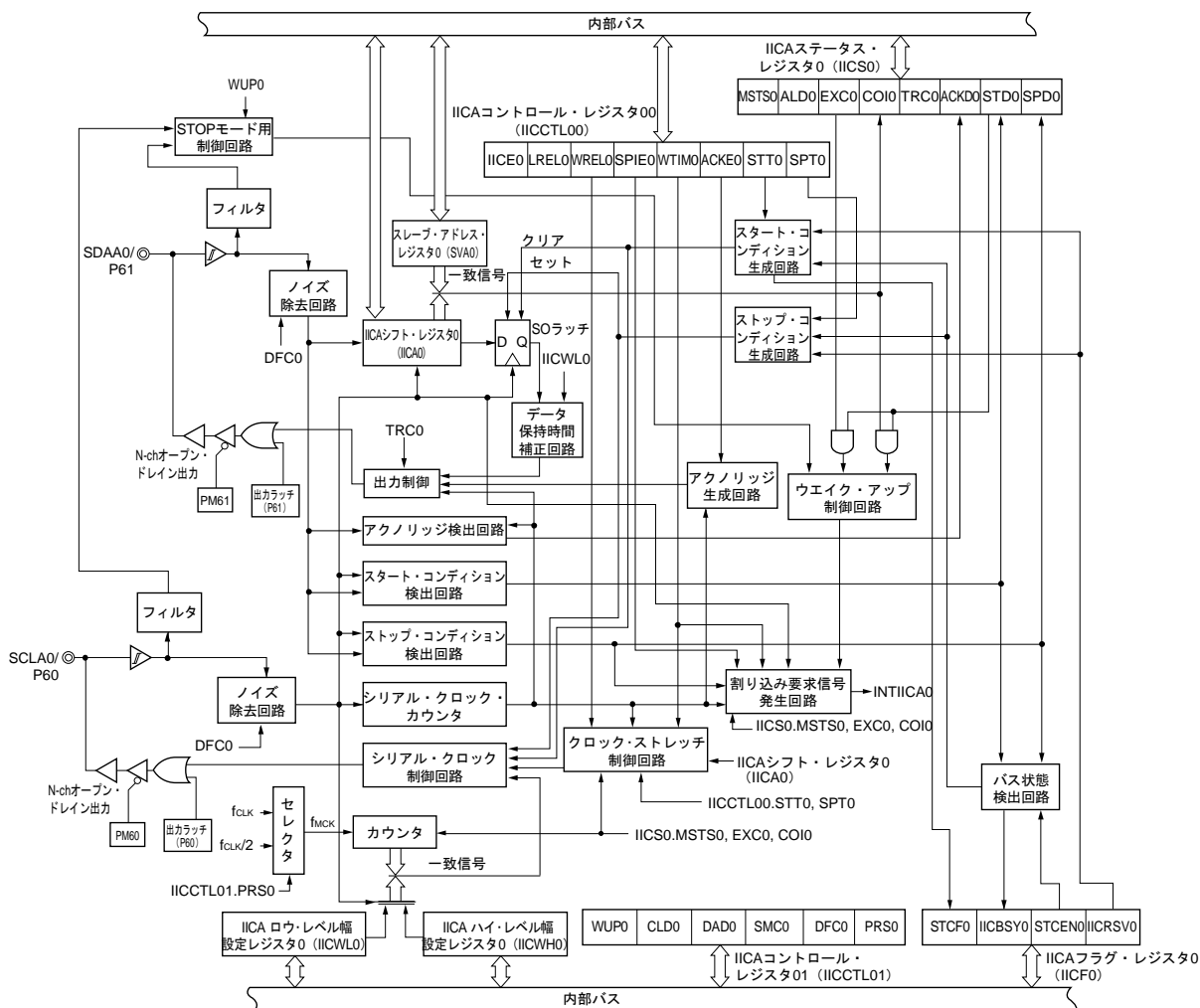
図15-1 シリアル・インタフェースIICA0のブロック図
