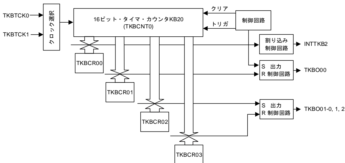
図7-40 単体動作時の構成図（TKBCR00による周期制御）
