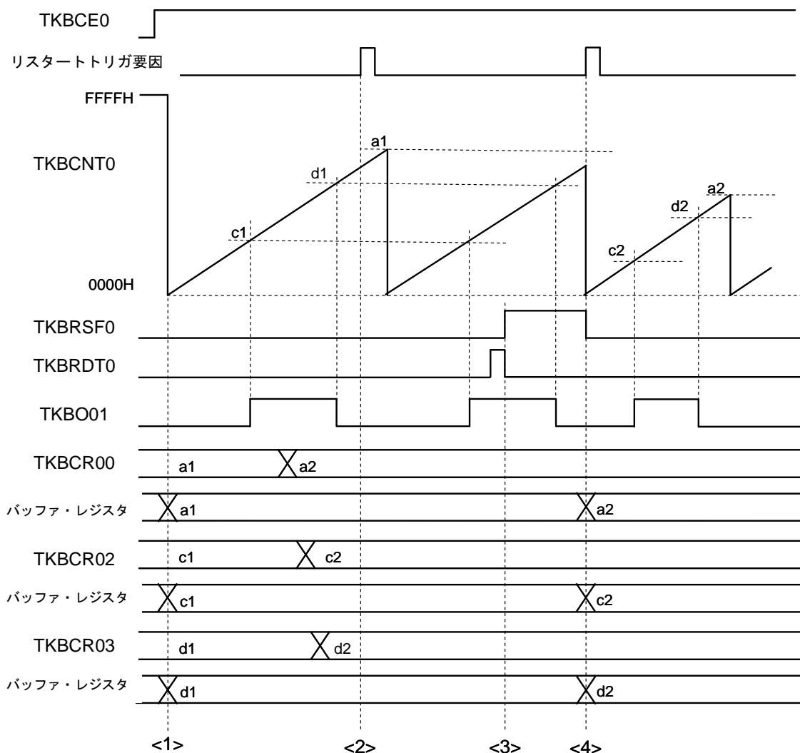
図7-66 IH制御用のPWM出力機能としての動作のコンペア・レジスタ00, 02, 03更新タイミング図
