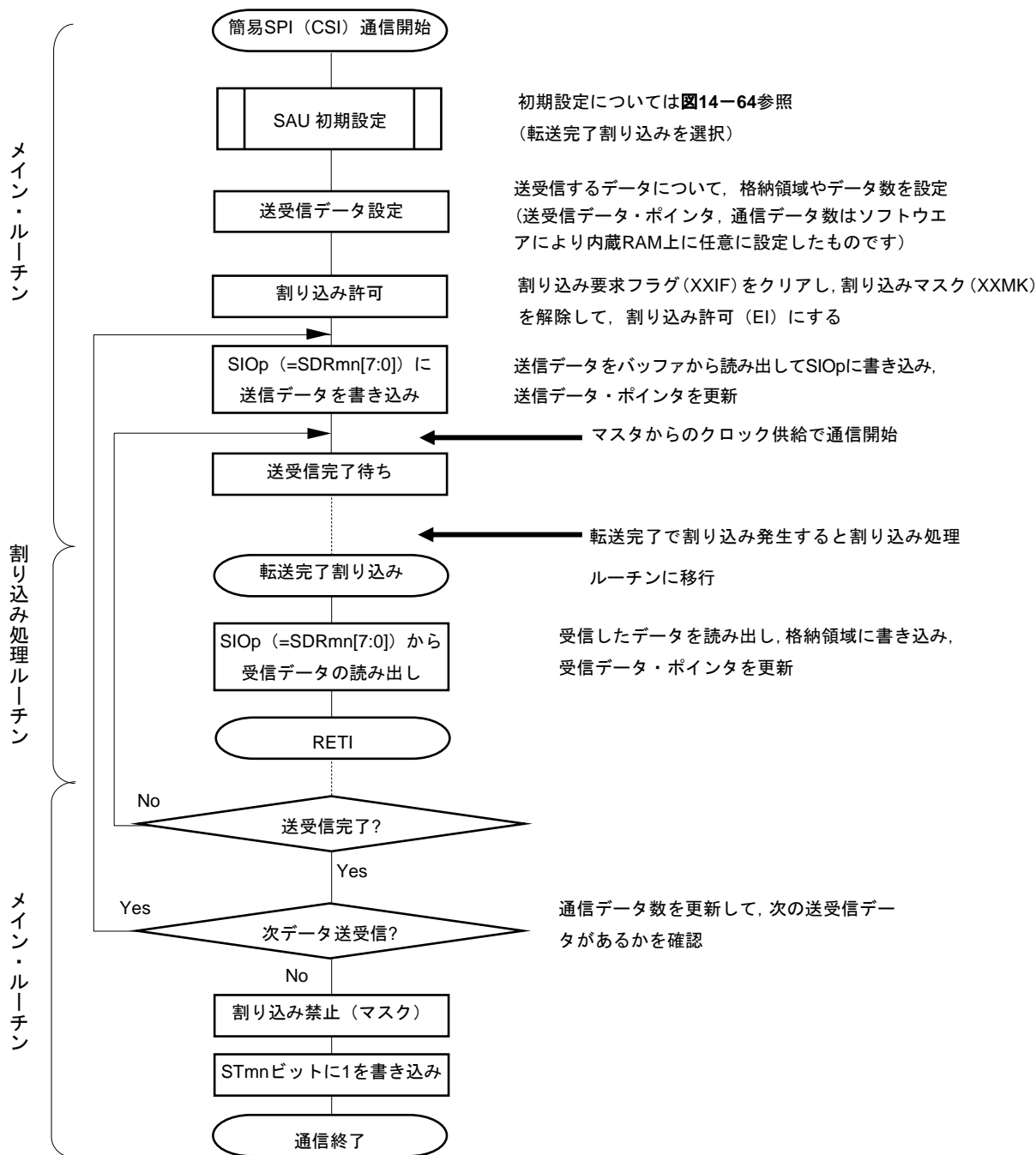
図14-68 スレーブ送受信（シングル送受信モード時）のフロー・チャート
