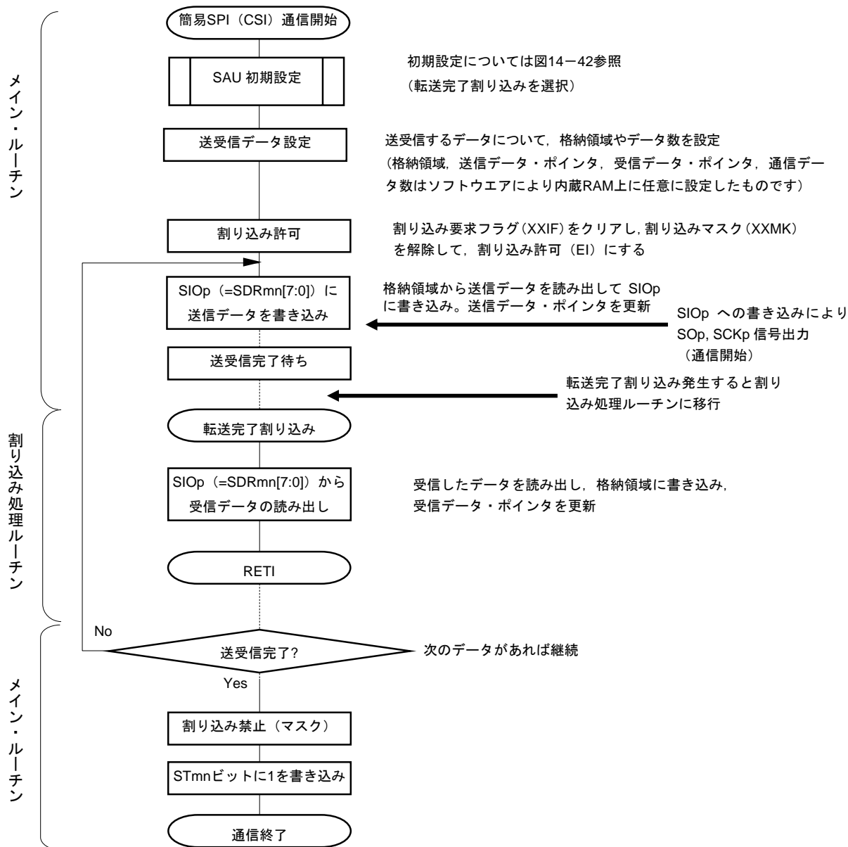
図14-46 マスタ送受信（シングル送受信モード時）のフロー・チャート
