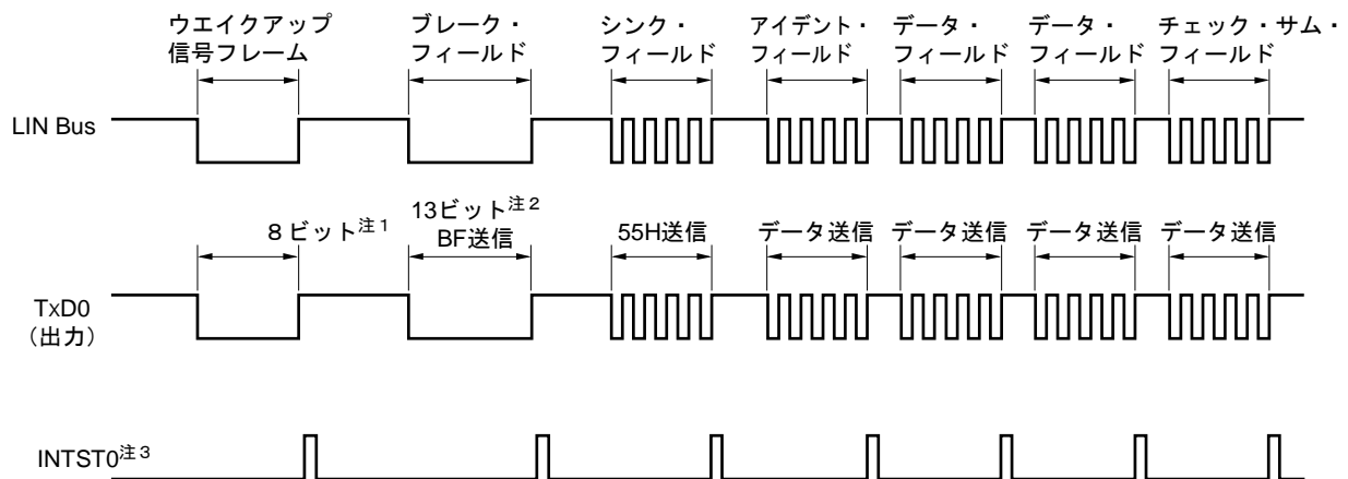
図14-98 LINの送信操作
