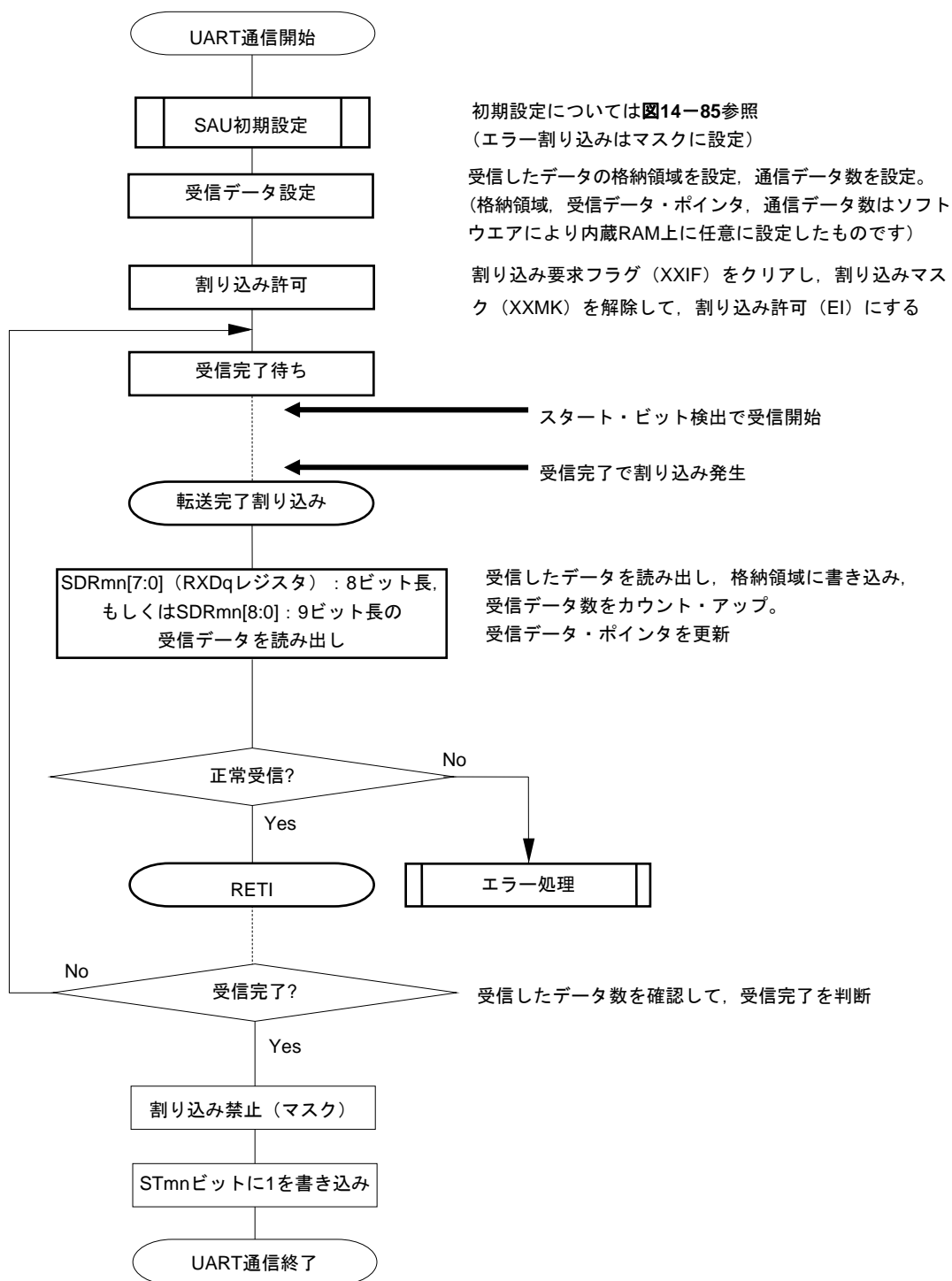
図14-89 UART受信のフロー・チャート
