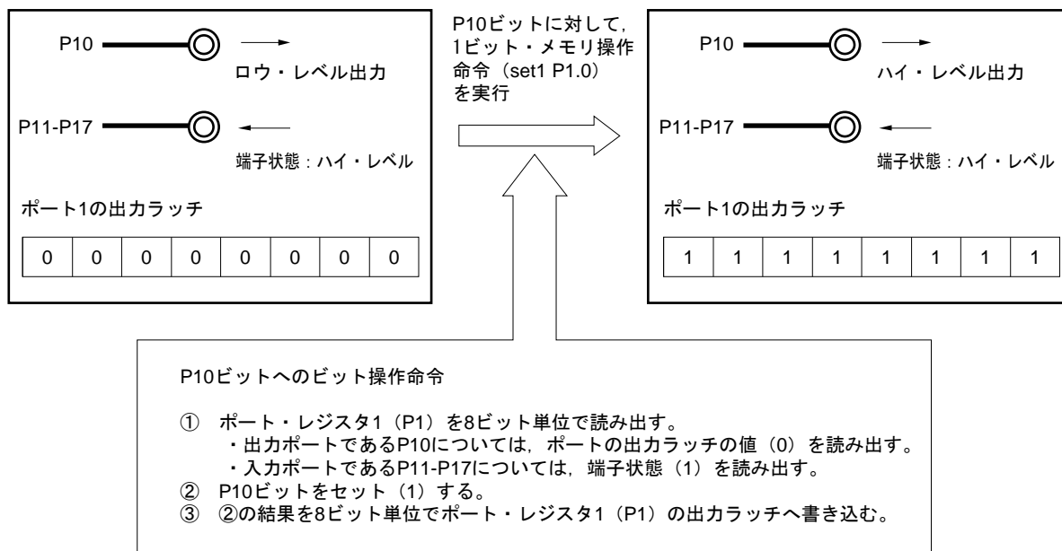
図4-17 1ビット・メモリ操作命令（P10の場合）
