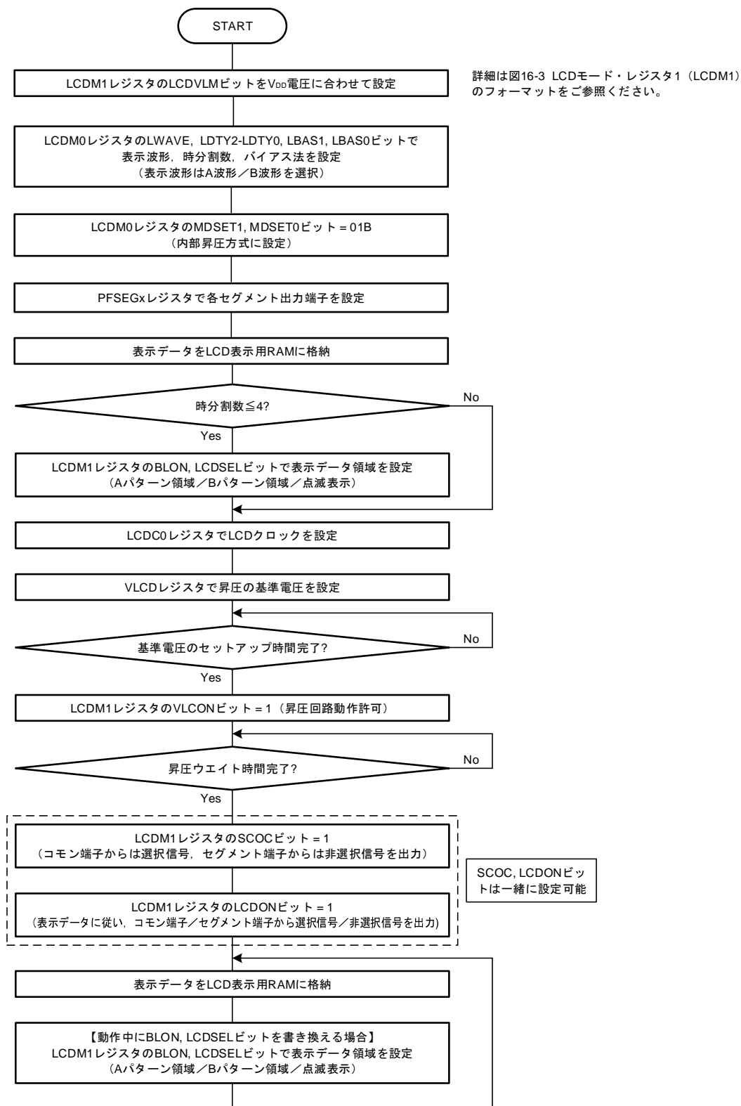
図16-18 内部昇圧方式の設定手順
