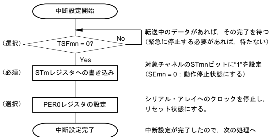
図14-86 UART受信の中断手順
