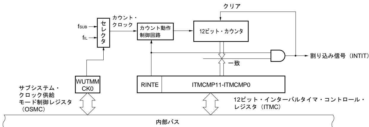
図9-1 12ビット・インターバル・タイマのブロック図
