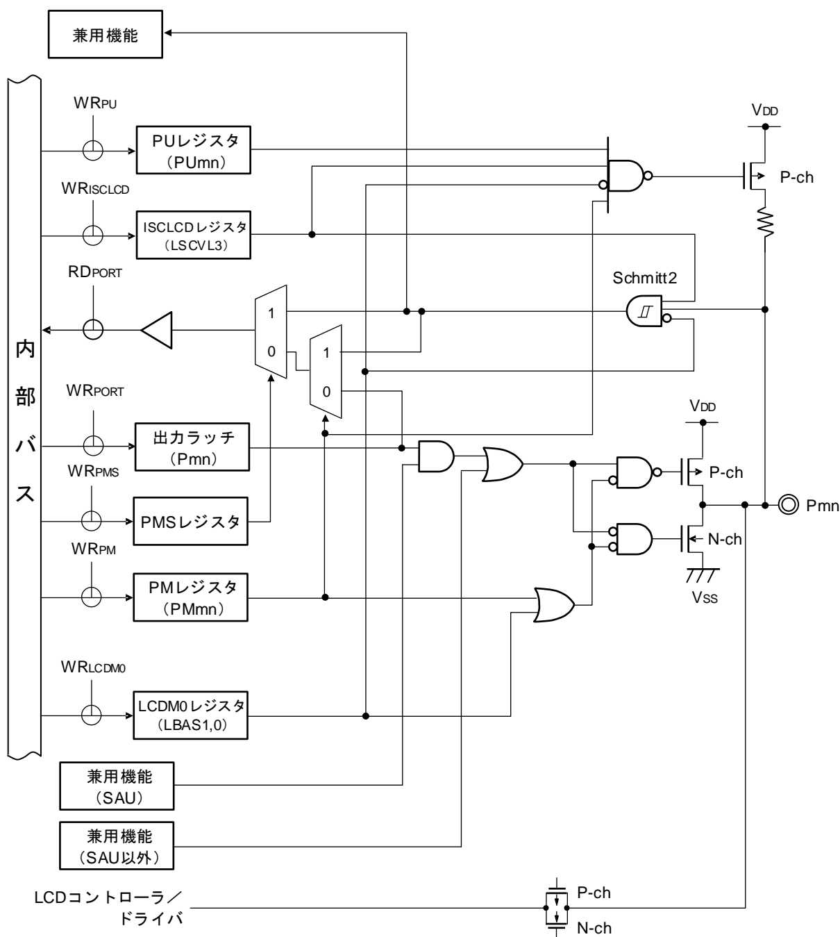
図2-8 端子タイプ 7-5-6 の端子ブロック図
