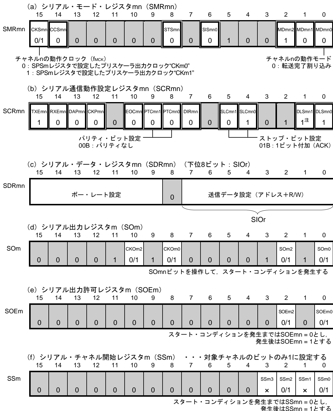
図14-103 簡易I 2 C (IIC00, IIC10) のアドレス・フィールド送信時のレジスタ設定内容例
