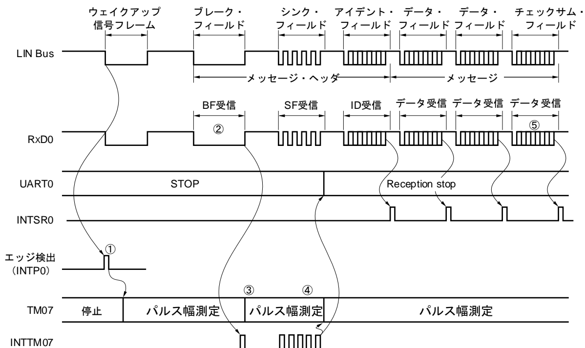
図14-100 LINの受信操作
