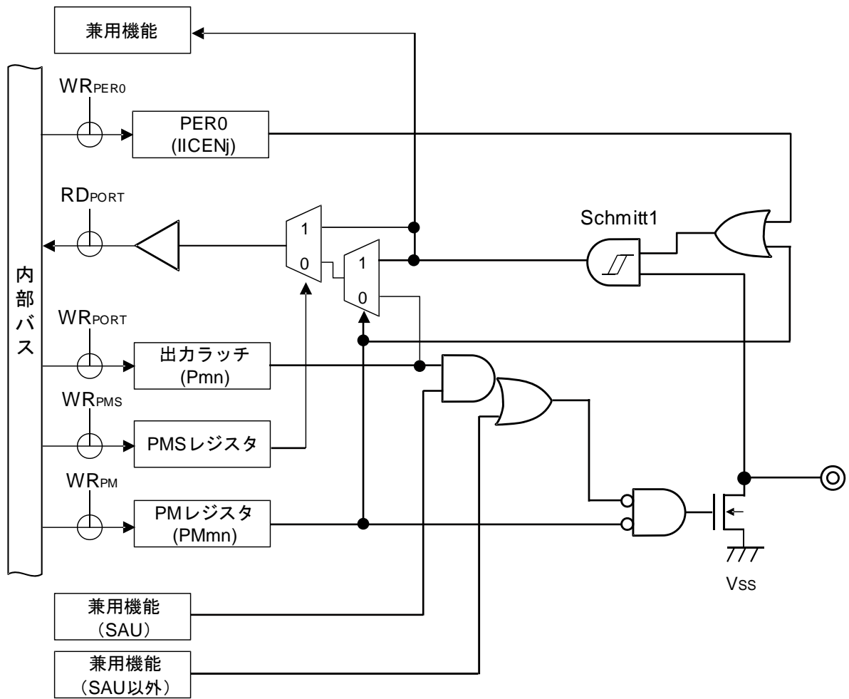
図2-17 端子タイプ 12-1-3 の端子ブロック図
