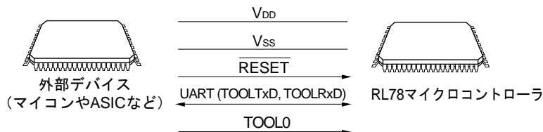
図28-3 フラッシュ・メモリにプログラムを書き込むための環境
