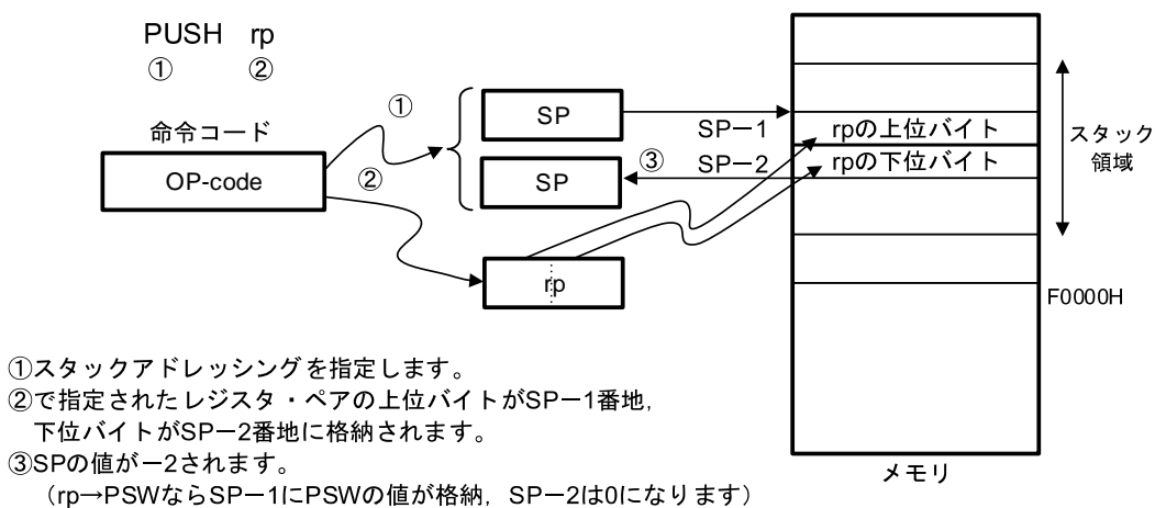
図3-37 PUSH rpの例
