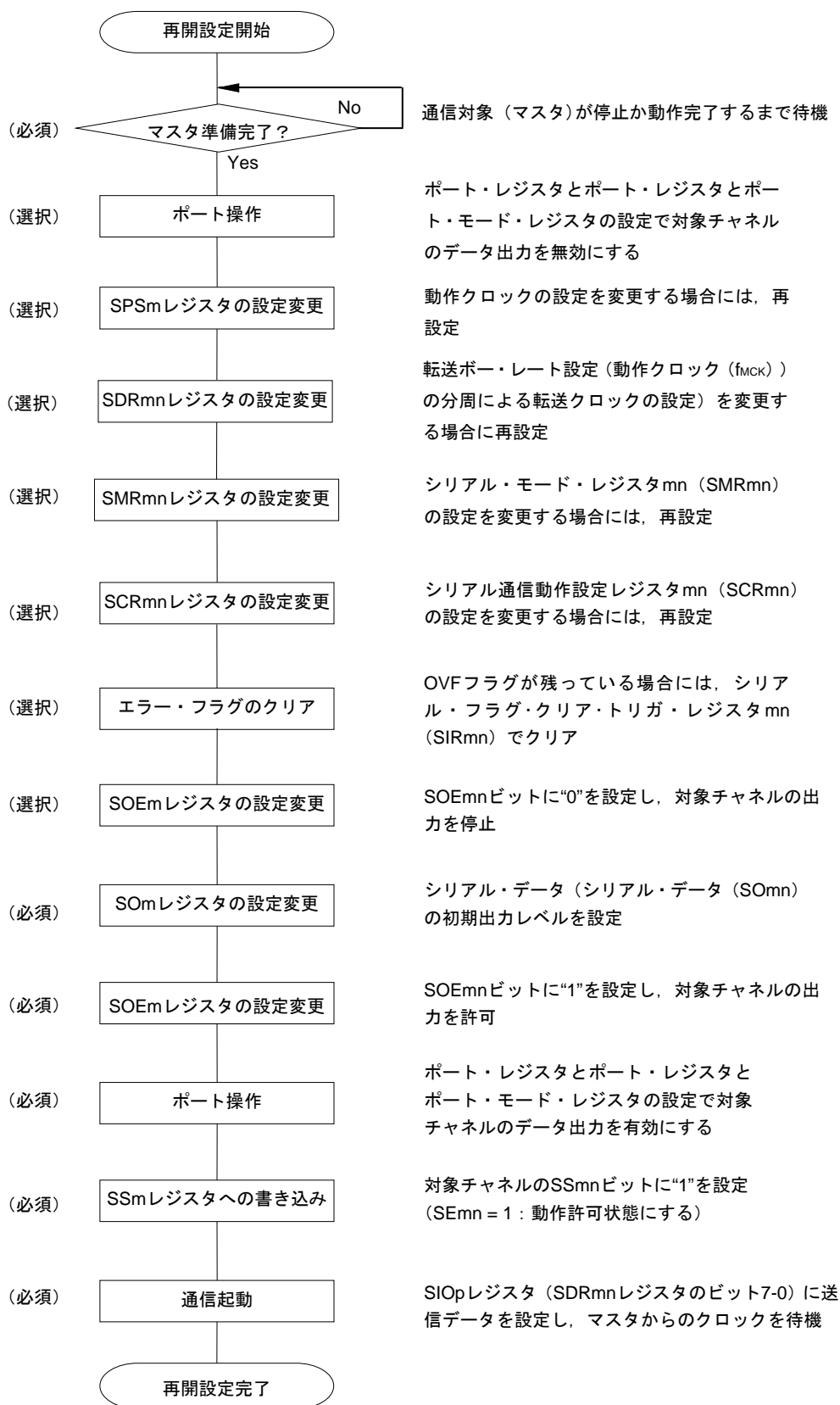
図14-52 スレーブ送信の再開設定手順
