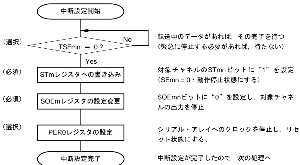
図14-59 スレーブ受信の中断手順
