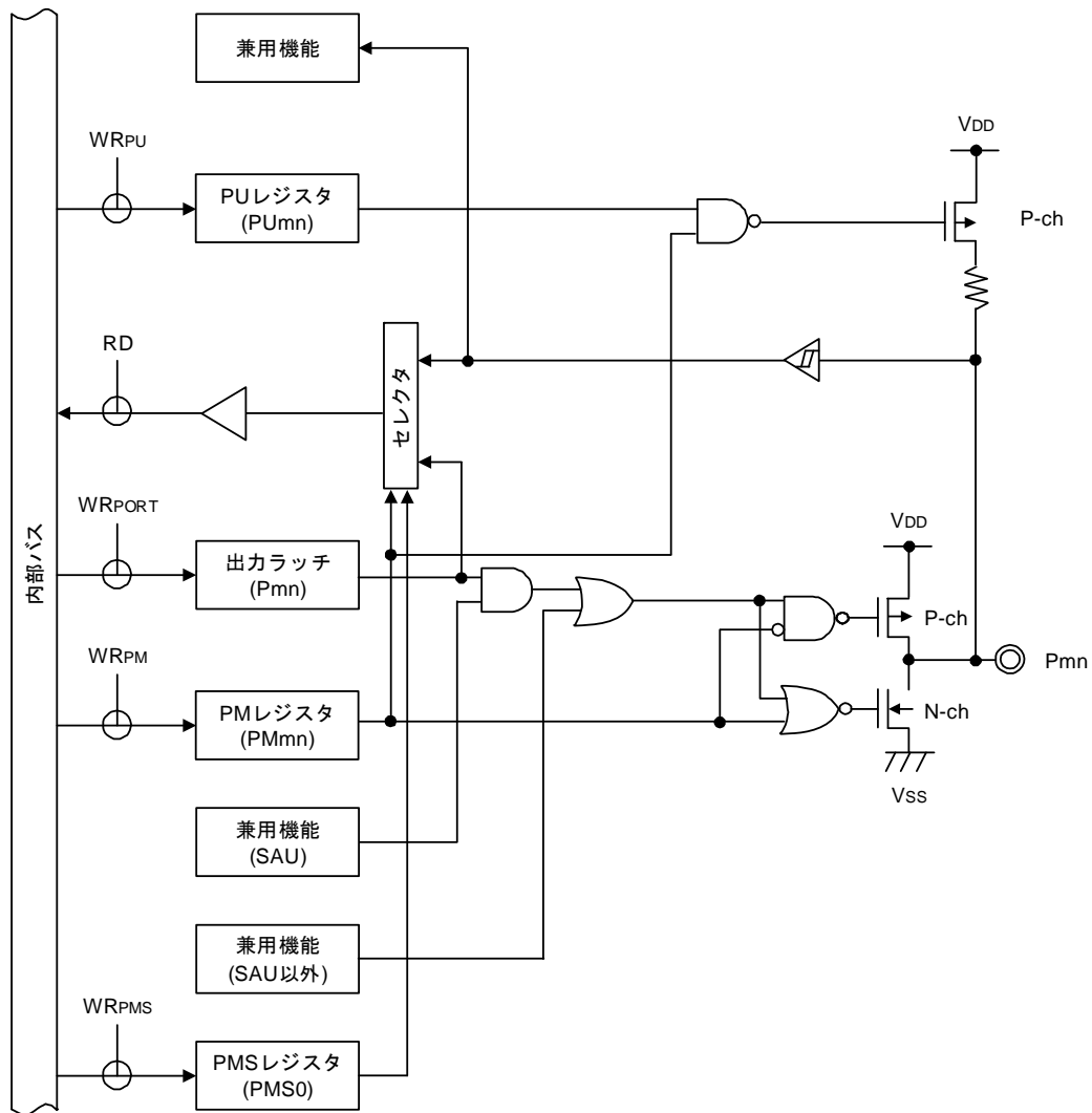
図2-5 端子タイプ 7-1-3 の端子ブロック図
