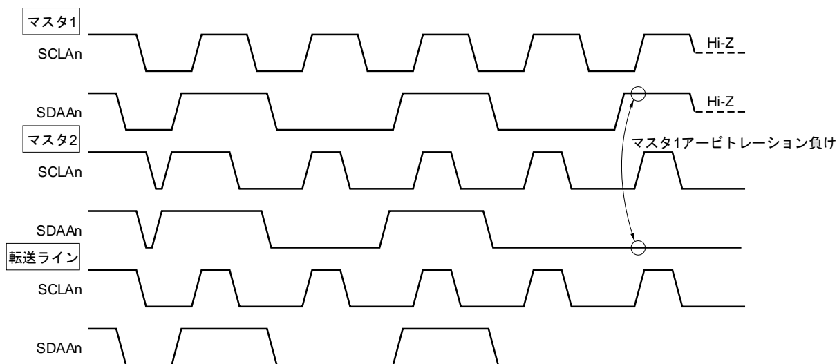
図15-21 アービトレーション・タイミング例
