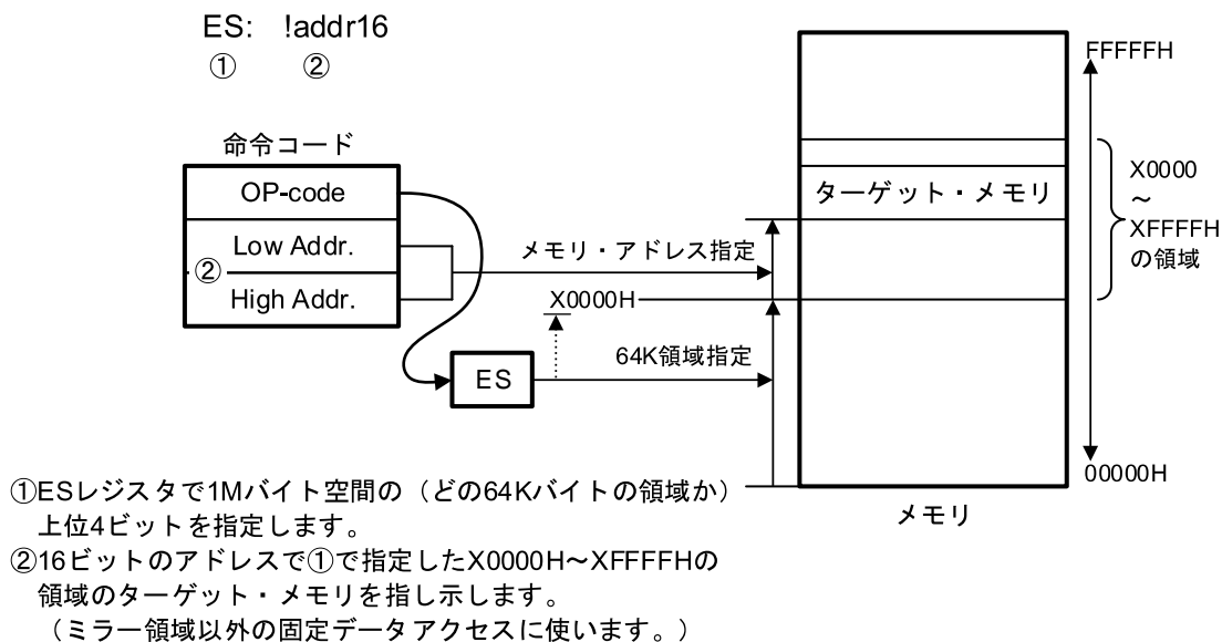
図3-23 ES:!addr16の例
