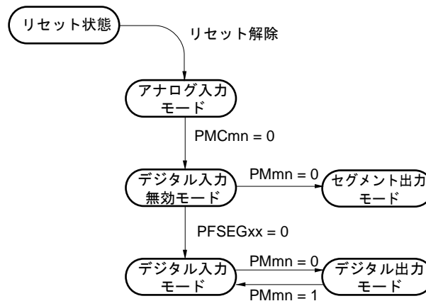
図16-12 ANlxx/SEGxx/ポート端子機能の状態遷移図
