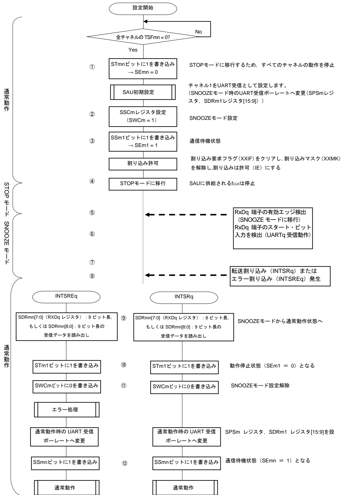
図14-92 SNOOZEモード動作 (EOCm1 = 0, SSECm = 0/1もしくはEOCm1 = 1, SSECm = 0) 時の フロー・チャート
