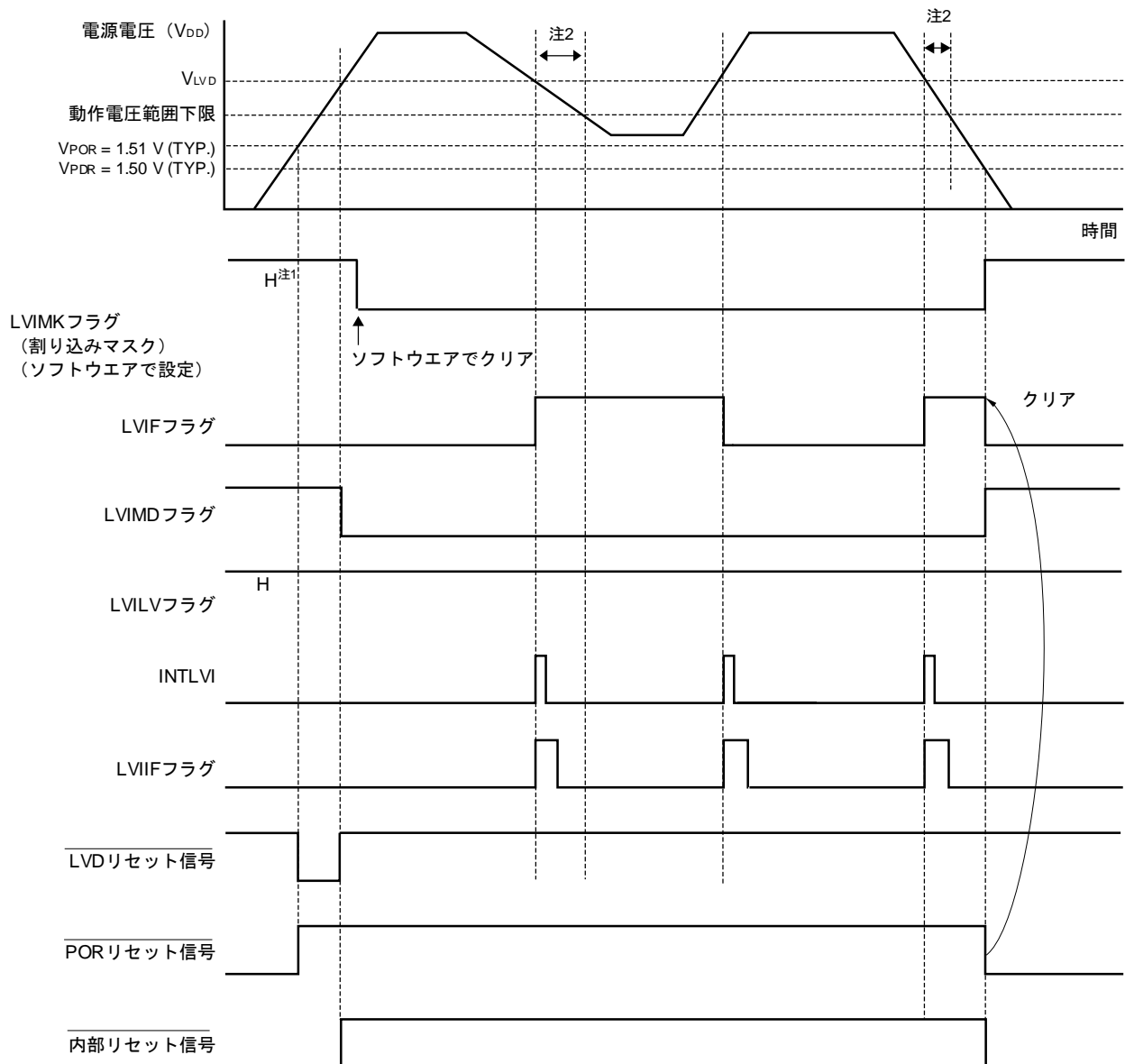
図24-6 割り込み信号発生タイミング (オプション・バイトのLVIMDS1, LVIMDS0 = 0, 1)
