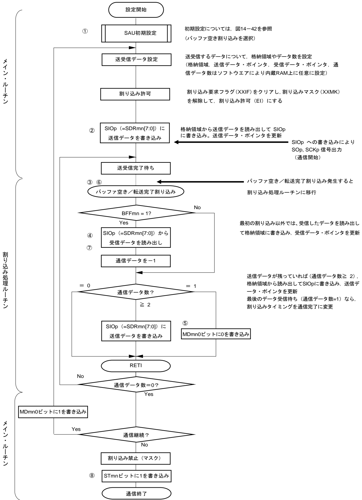
図14-48 マスタ送受信（連続送受信モード時）のフロー・チャート
