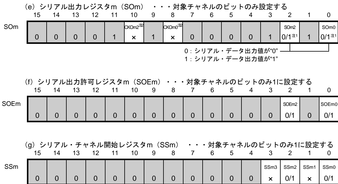
図14-76 UART (UART0-UART3) のUART送信時のレジスタ設定内容例 (80ピン製品) (2/2)
