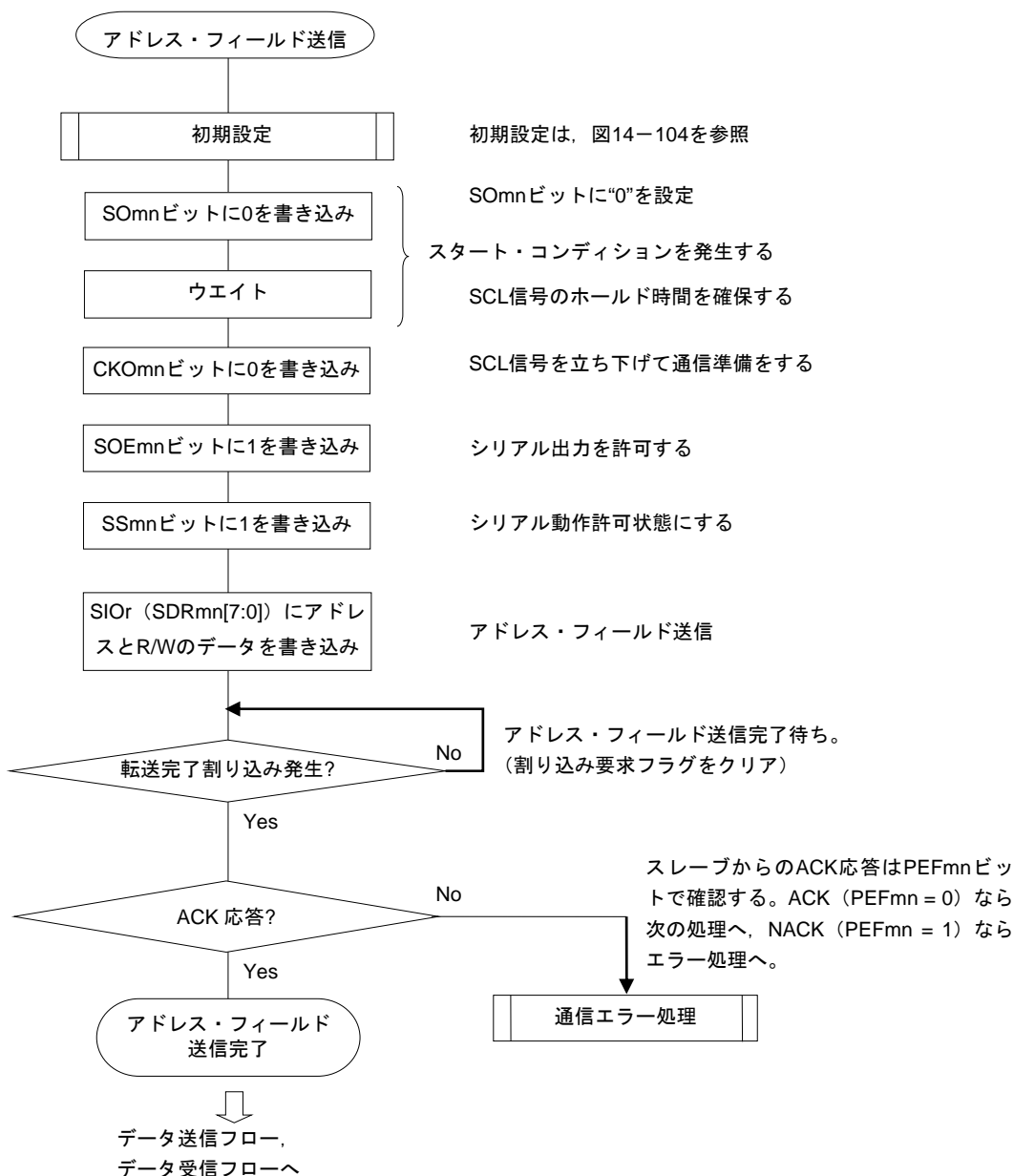
図14-106 簡易I 2 Cアドレス・フィールド送信のフロー・チャート
