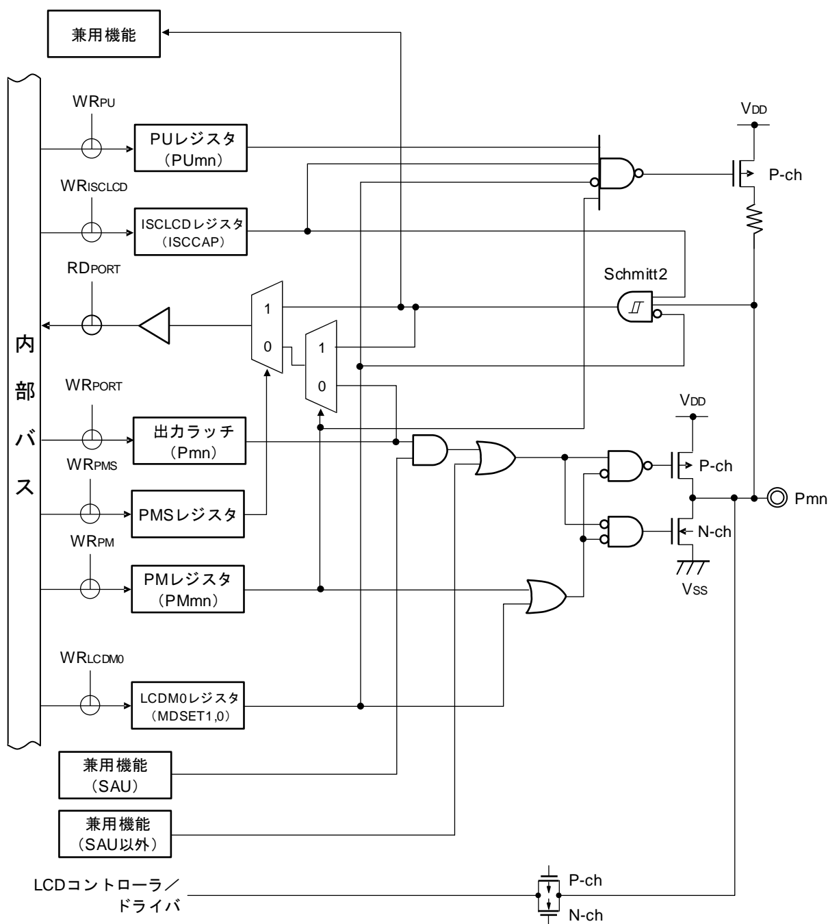
図2-7 端子タイプ 7-5-5 の端子ブロック図
