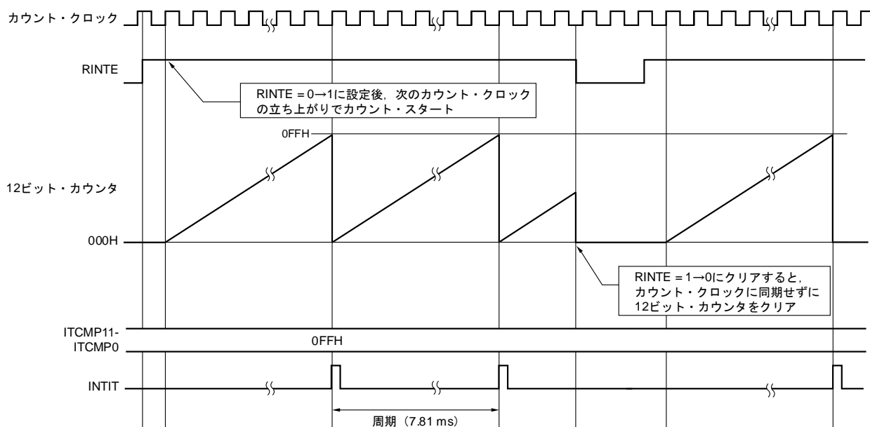
図9-5 12ビット・インターバル・タイマ動作のタイミング (ITMCMP11-ITMCMP0 = 0FFH, カウント・クロック : f_{SUB} = 32.768 kHz)
