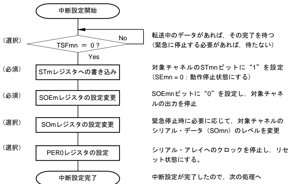
図14-65 スレーブ送受信の中断手順
