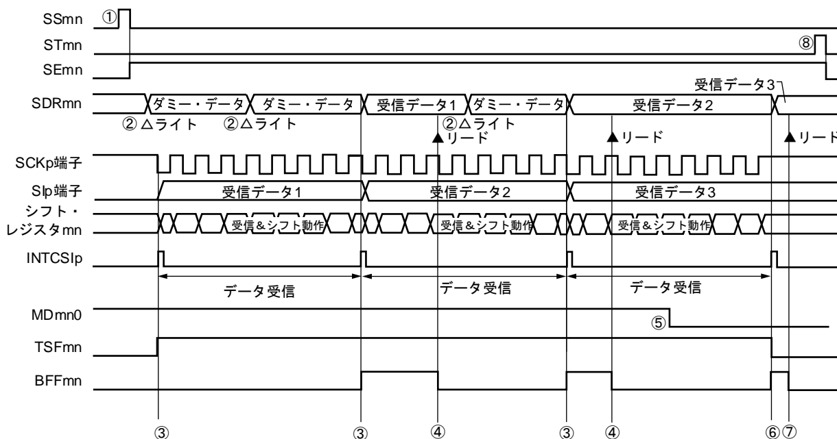
図14-39 マスタ受信（連続受信モード時）のタイミング・チャート（タイプ1：DAPmn = 0, CKPmn = 0）
