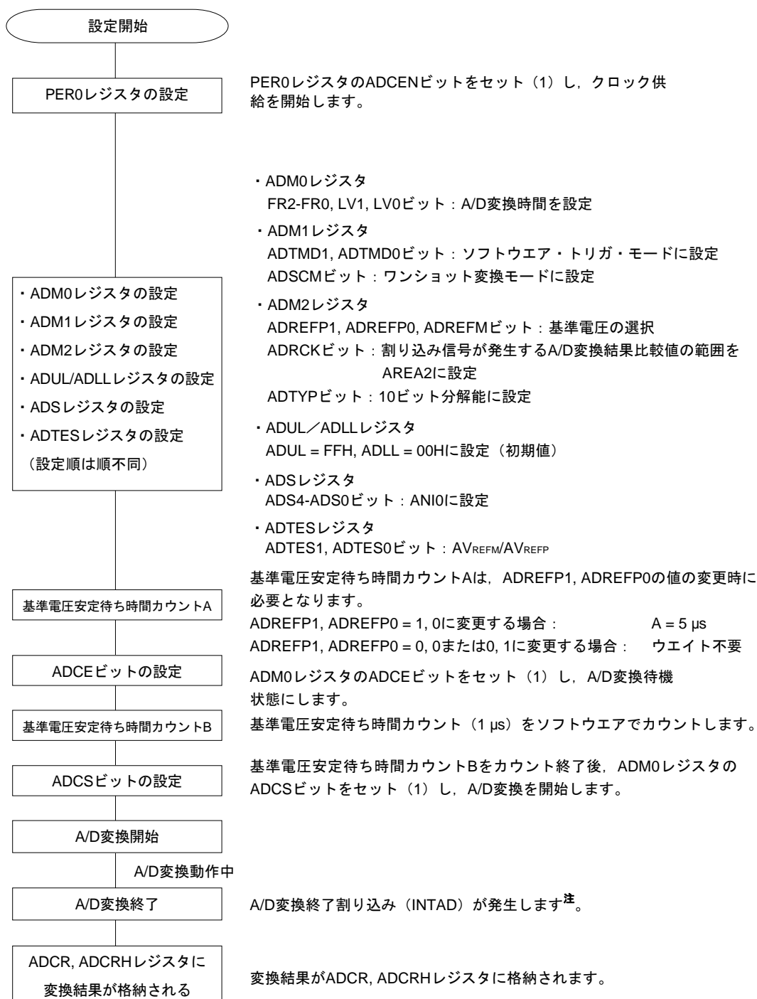
図12-27 テスト・モード設定
