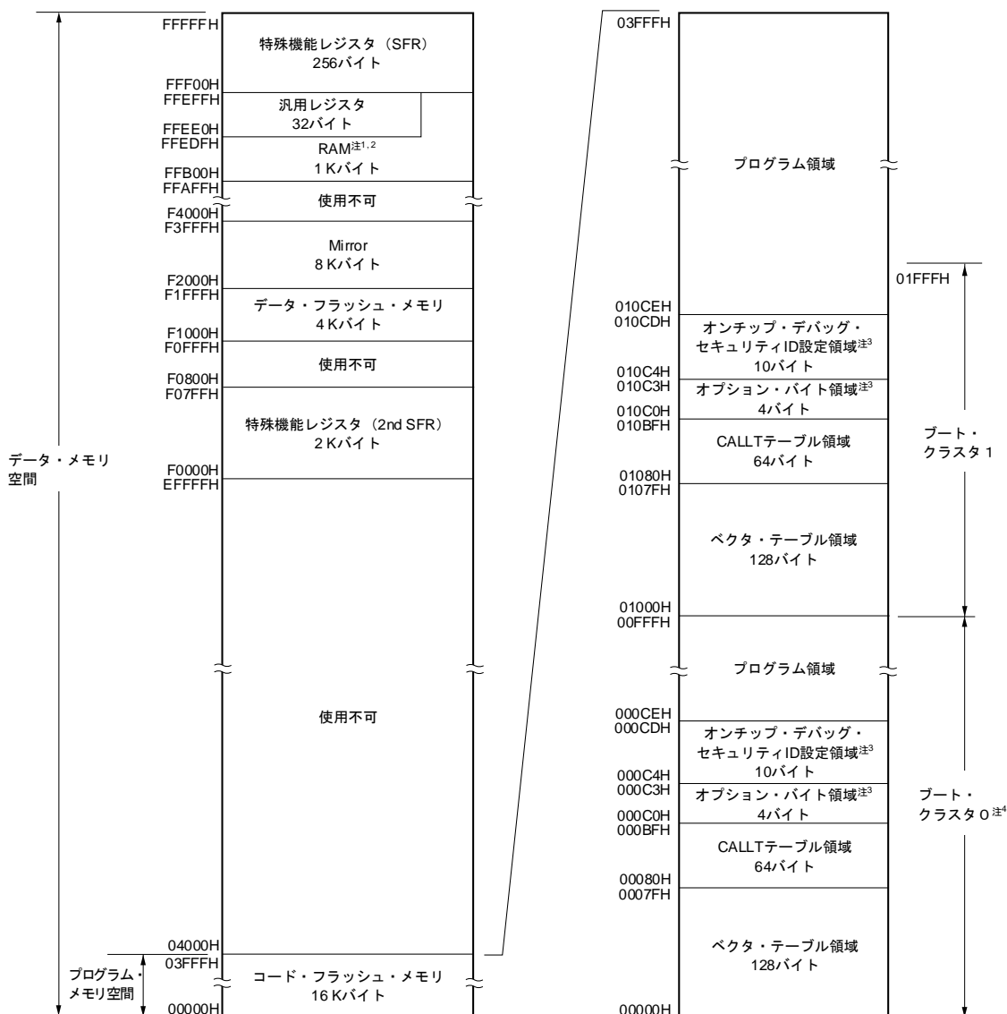
図3-1 メモリ・マップ (R5F10WLA, R5F10WMA)
