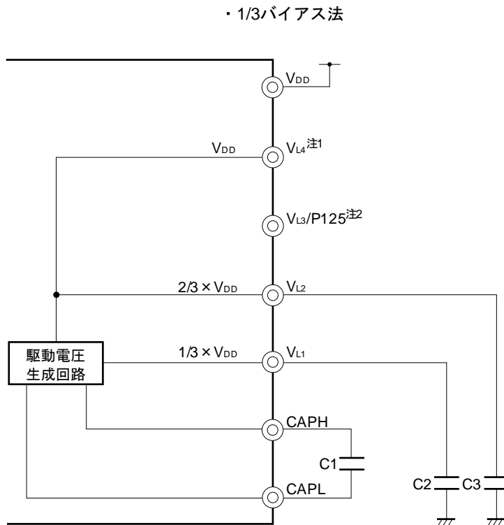
図16-23 LCD駆動電源の接続例（容量分割方式）
