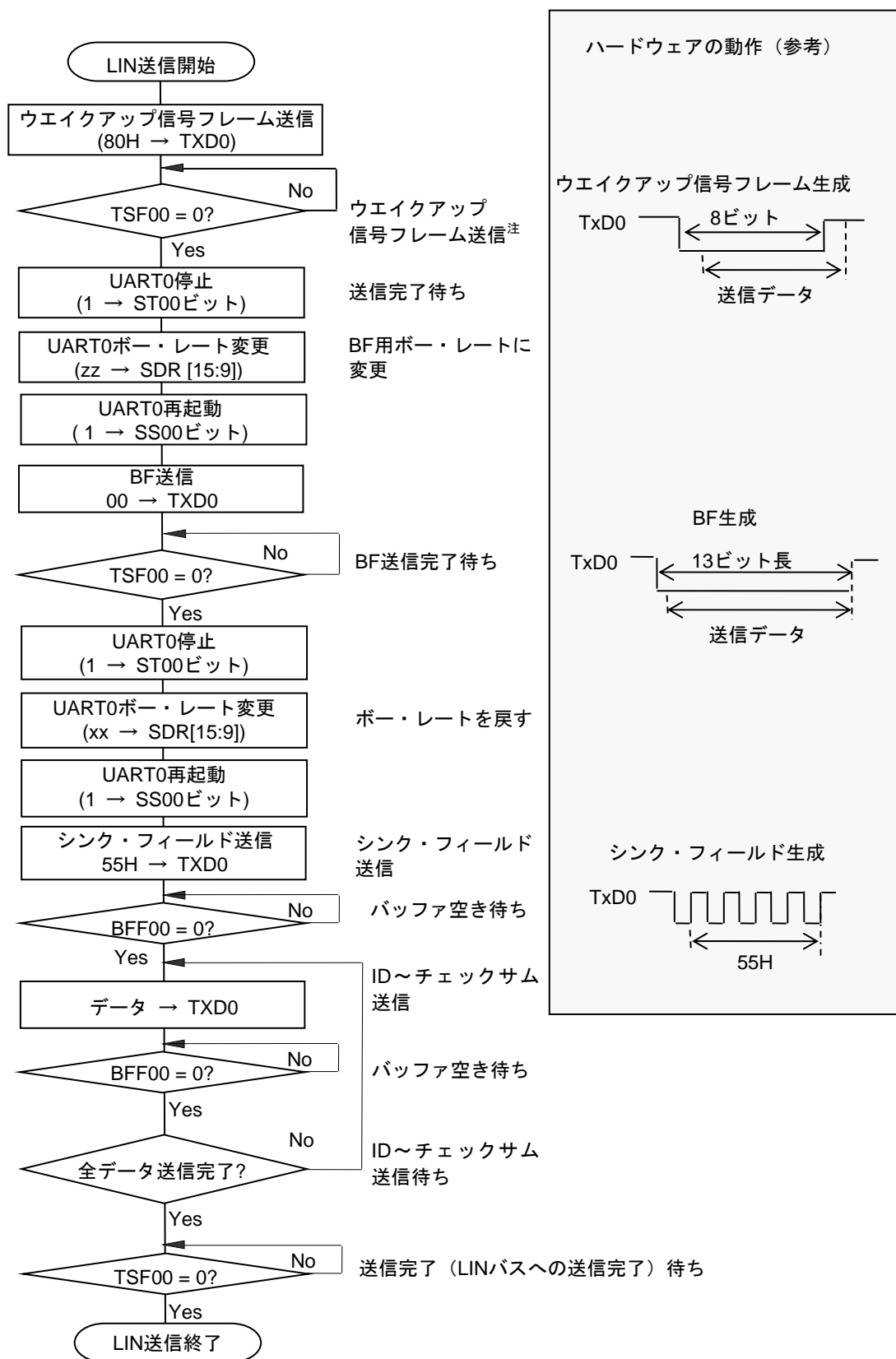
図14-99 LIN送信のフロー・チャート
