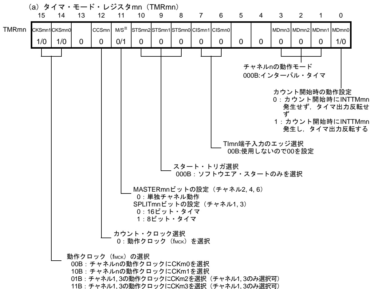
図6-45 インターバル・タイマ／方形波出力時のレジスタ設定内容例
