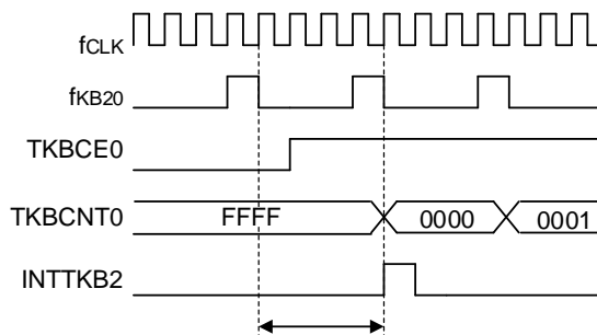
図7-35 動作開始のタイミング図 (TKBCE0を“0”から“1”に変更した場合)
