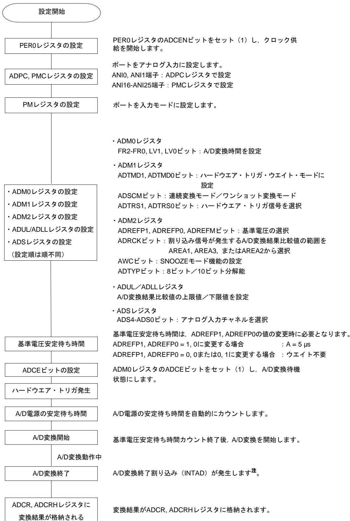
図12-25 ハードウェア・トリガ・ウエイト・モード設定
