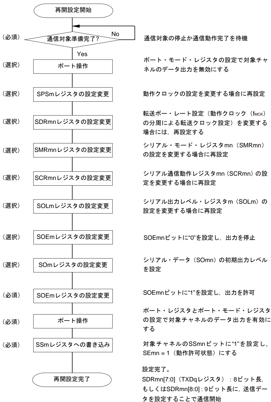
図14-79 UART送信の再開設定手順
