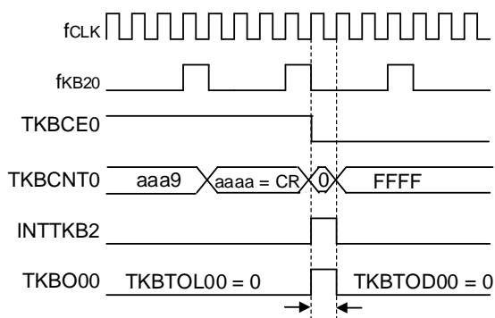
図7-38 動作停止のタイミング図 (TKBCE0の操作がタイマ・カウント・クロックの発生と同時の場合)
