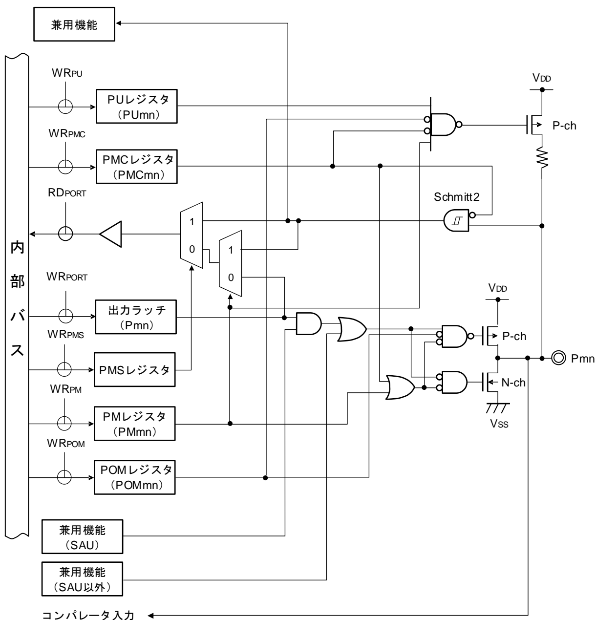
図2-11 端子タイプ 7-6-4 の端子ブロック図
