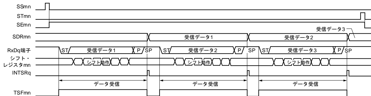
図14-88 UART受信のタイミング・チャート
