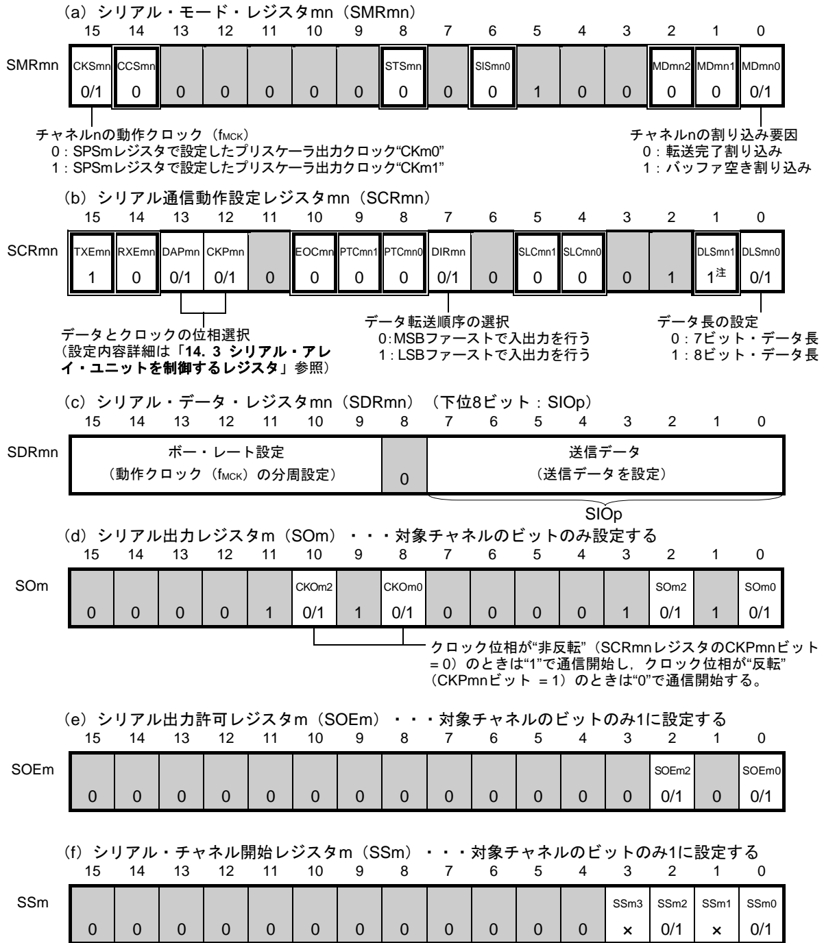
図14-25 簡易SPI (CSI00, CSI10) のマスタ送信時のレジスタ設定内容例
