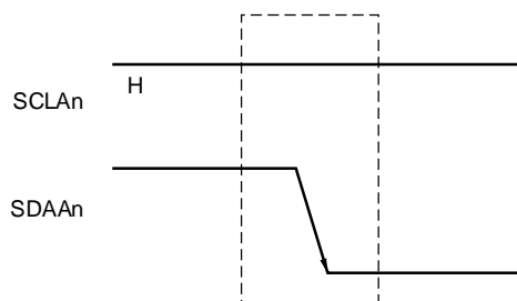
図15-15 スタート・コンディション
