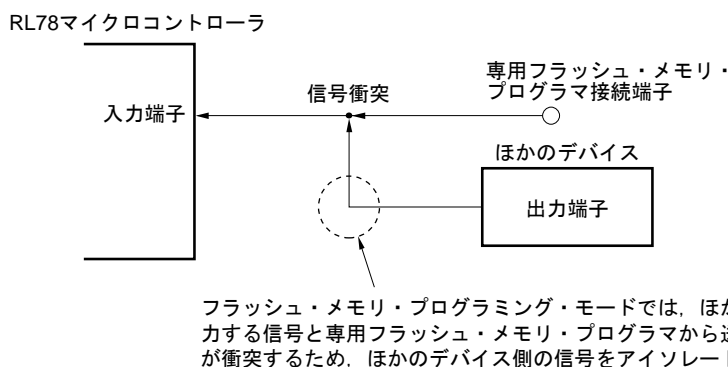
図28-5 信号の衝突 (RESET端子)
