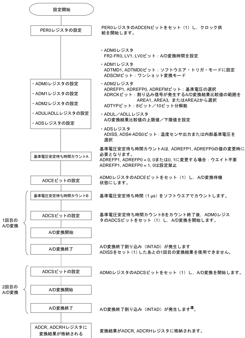
図12-26 温度センサ使用時の設定
