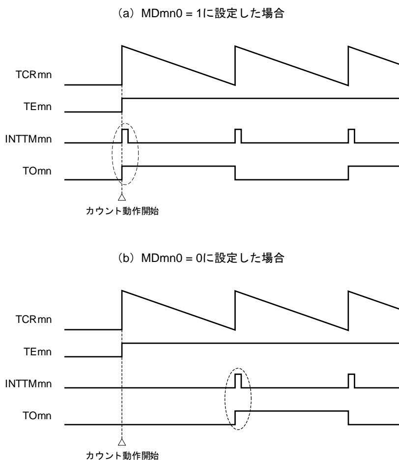
図6-40 カウント動作開始時のタイマ割り込み、TOMn出力の動作例
