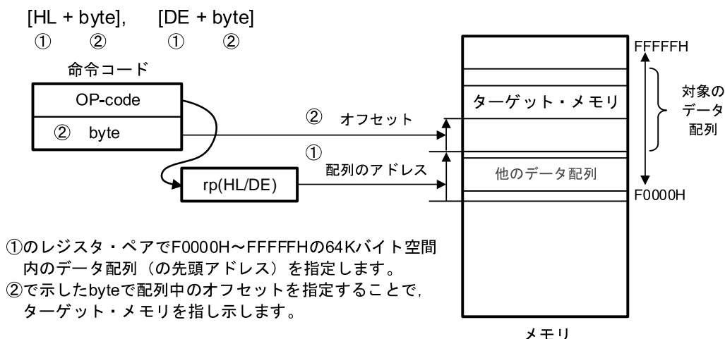
図3-30 word[B], word[C]の例
