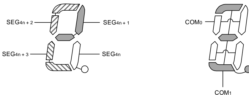
図16-29 2時分割LCD表示パターンと電極結線
