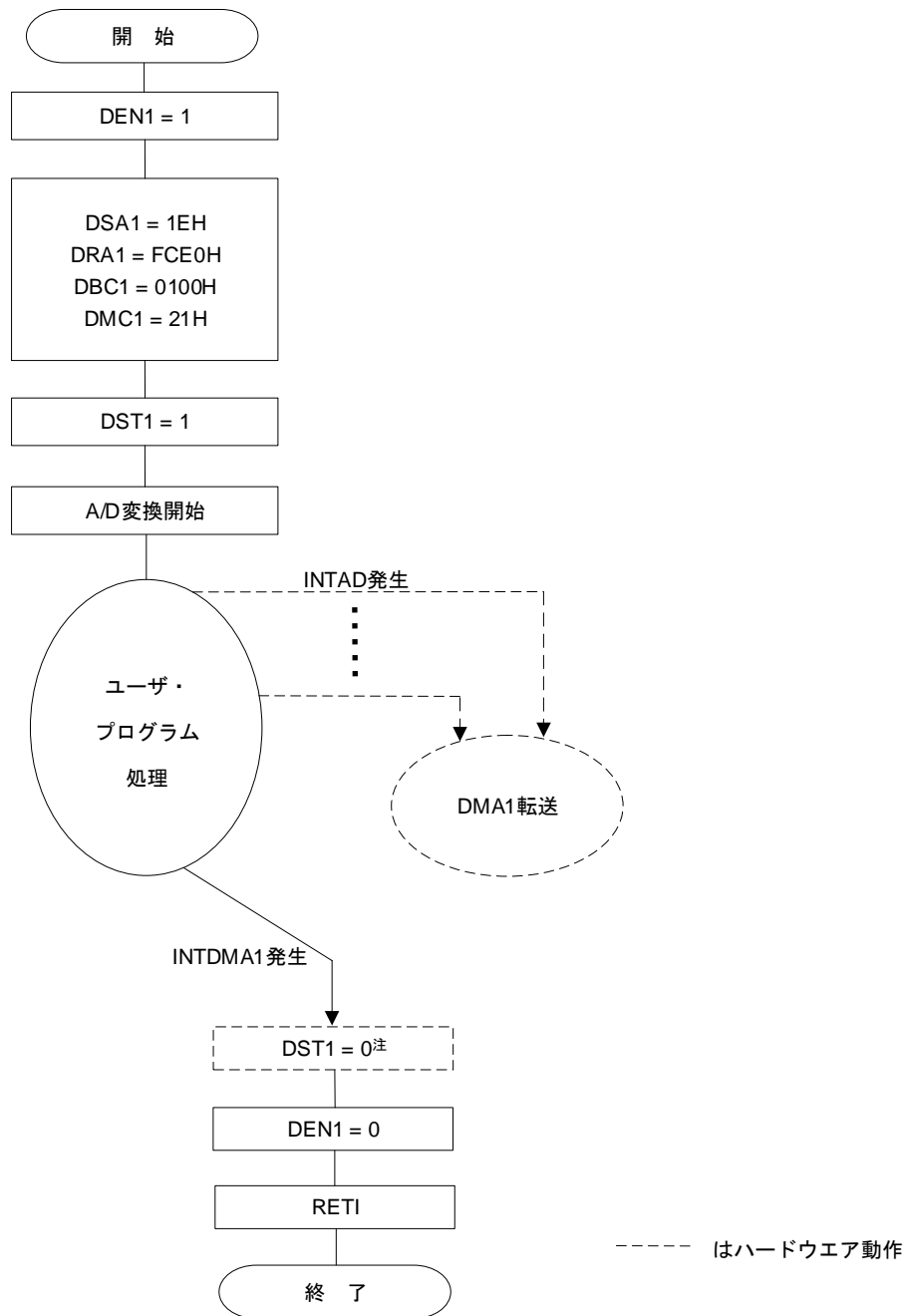
図18-8 A/D変換結果の連続取り込みの設定例
