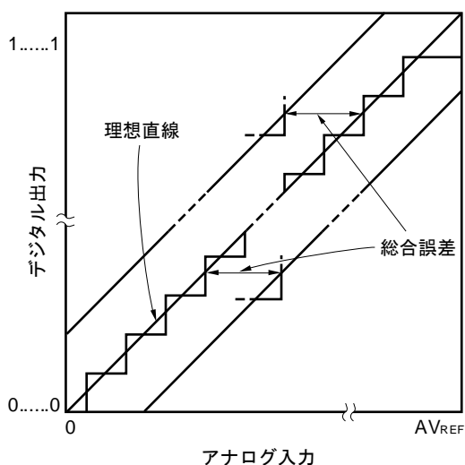
図12-32 総合誤差
