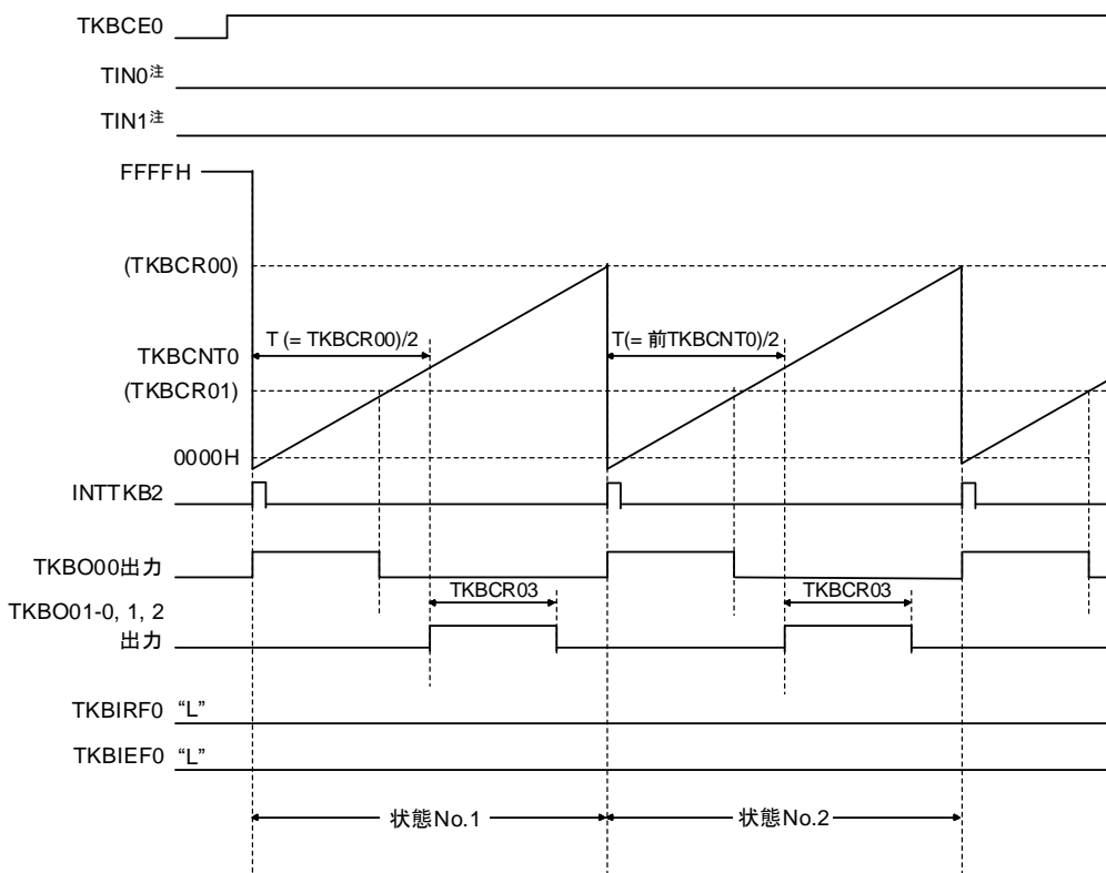
図7-48 インターリーブPFCモードのタイミング図 (状態No.1~No.2の動作)
