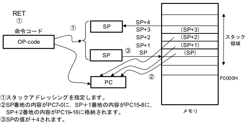
図3-40 RETの例
