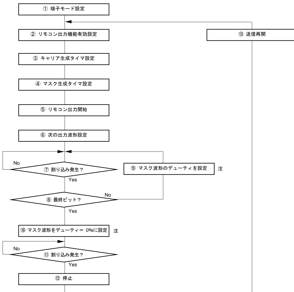
図6-79 リモコン出力機能設定手順 (1/2)
