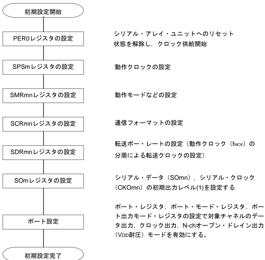
図14-104 簡易I 2 Cアドレス・フィールド送信の初期設定手順
