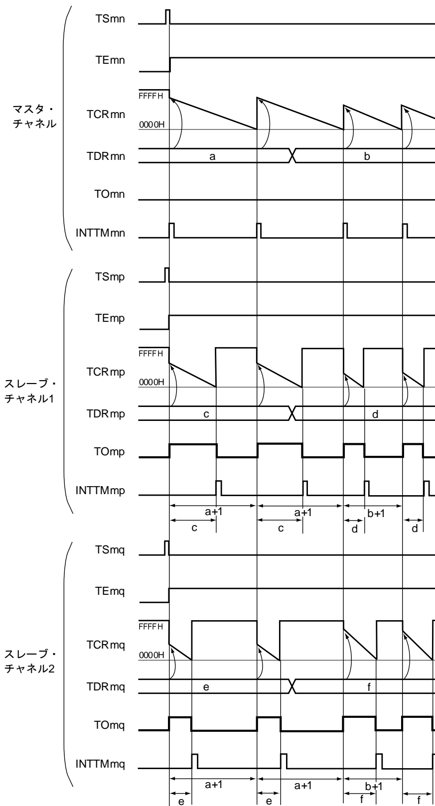
図6-74 多重PWM出力機能としての動作の基本タイミング例（2種類のPWMを出力する場合）
