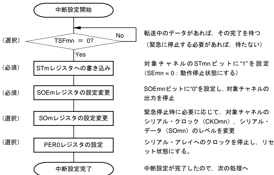
図14-43 マスタ送受信の中断手順
