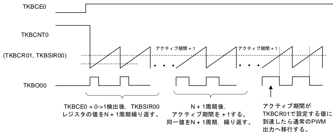
図7-61 PWM出力ソフト・スタート機能TKBO00出力の例
