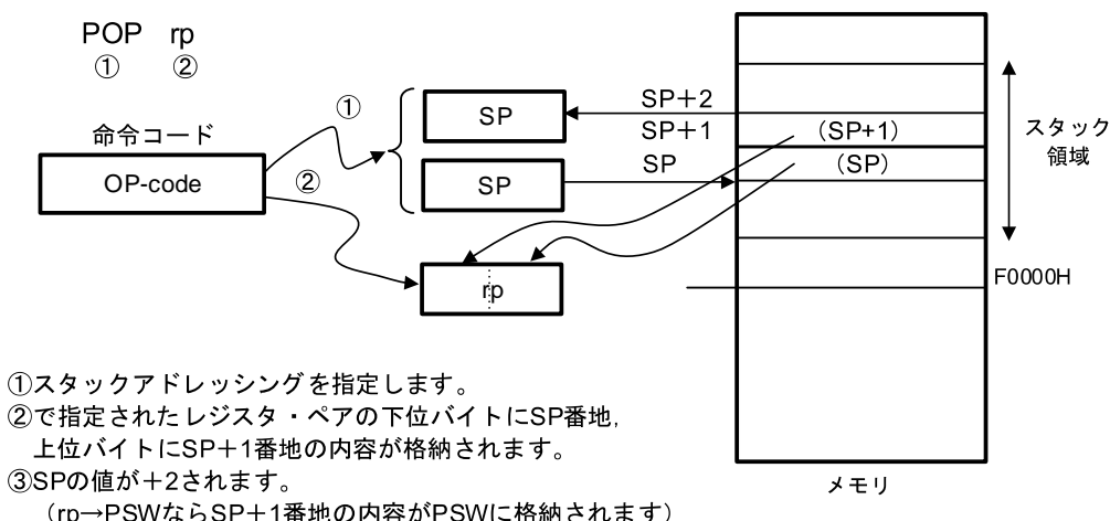
図3-38 POPの例
