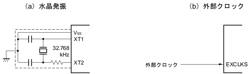
図5-13 XT1発振回路の外付け回路例
