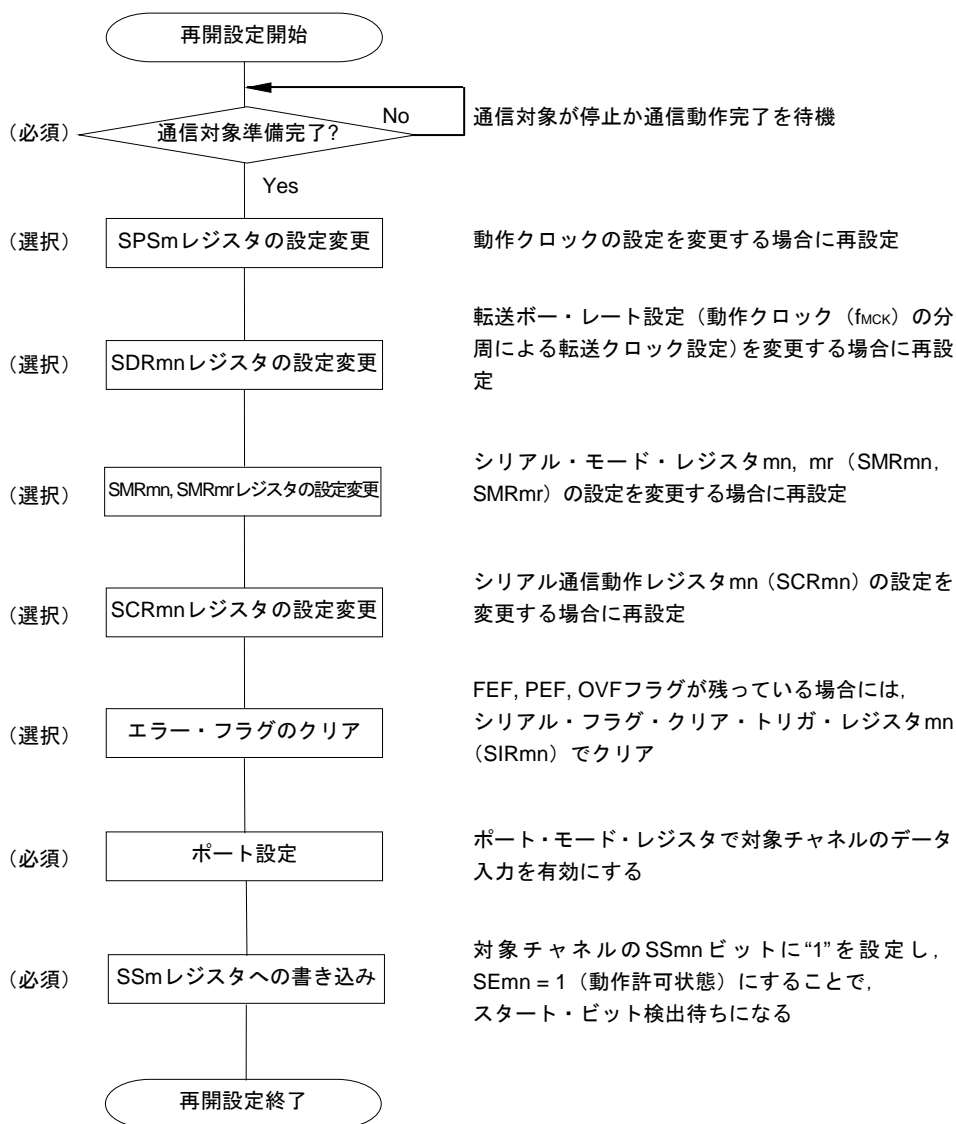
図14-87 UART受信の再開設定手順
