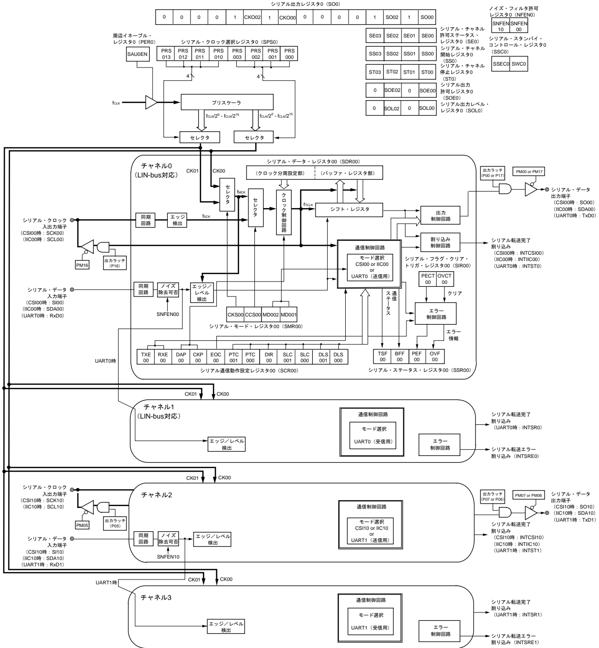
図14-1 シリアル・アレイ・ユニット0のブロック図
