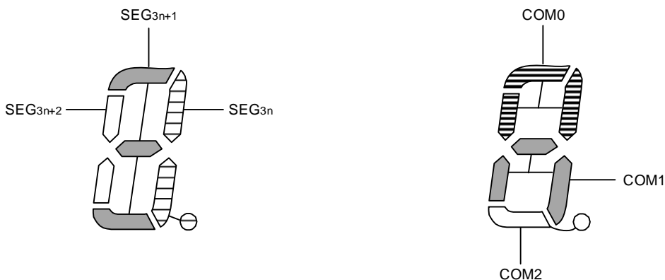
図16-32 3時分割LCD表示パターンと電極結線
