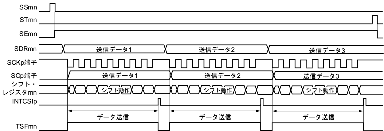
図14-29 マスタ送信（シングル送信モード時）のタイミング・チャート（タイプ1：DAPmn = 0, CKPmn = 0）
