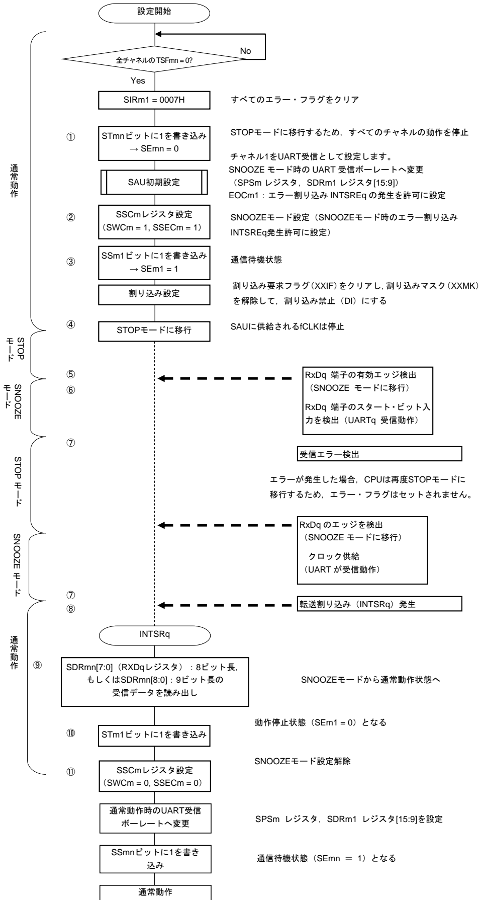
図14-94 SNOOZEモード動作 (EOCm1 = 1, SSECm = 1) 時のフロー・チャート
