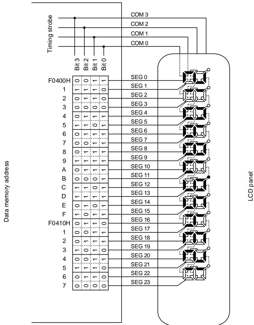
図16-37 4時分割LCDパネルの結線例
