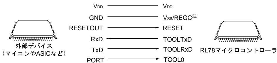
図28-4 外部デバイスとの通信
