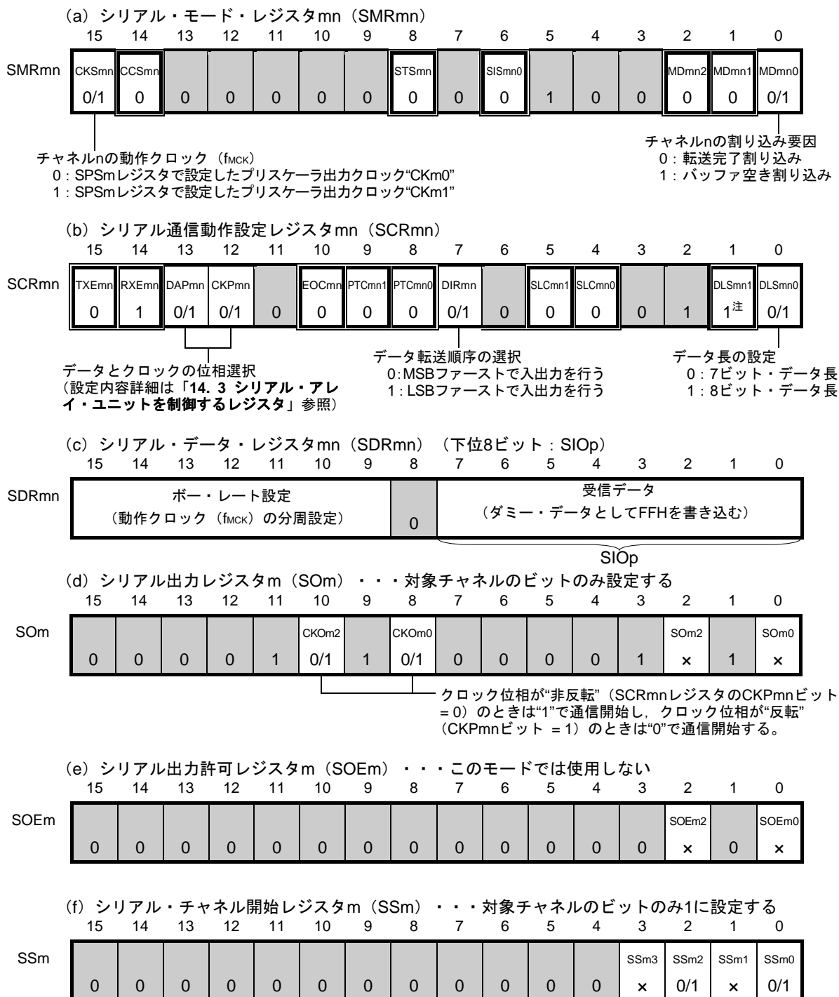
図14-33 簡易SPI (CSI00, CSI10) のマスタ受信時のレジスタ設定内容例
