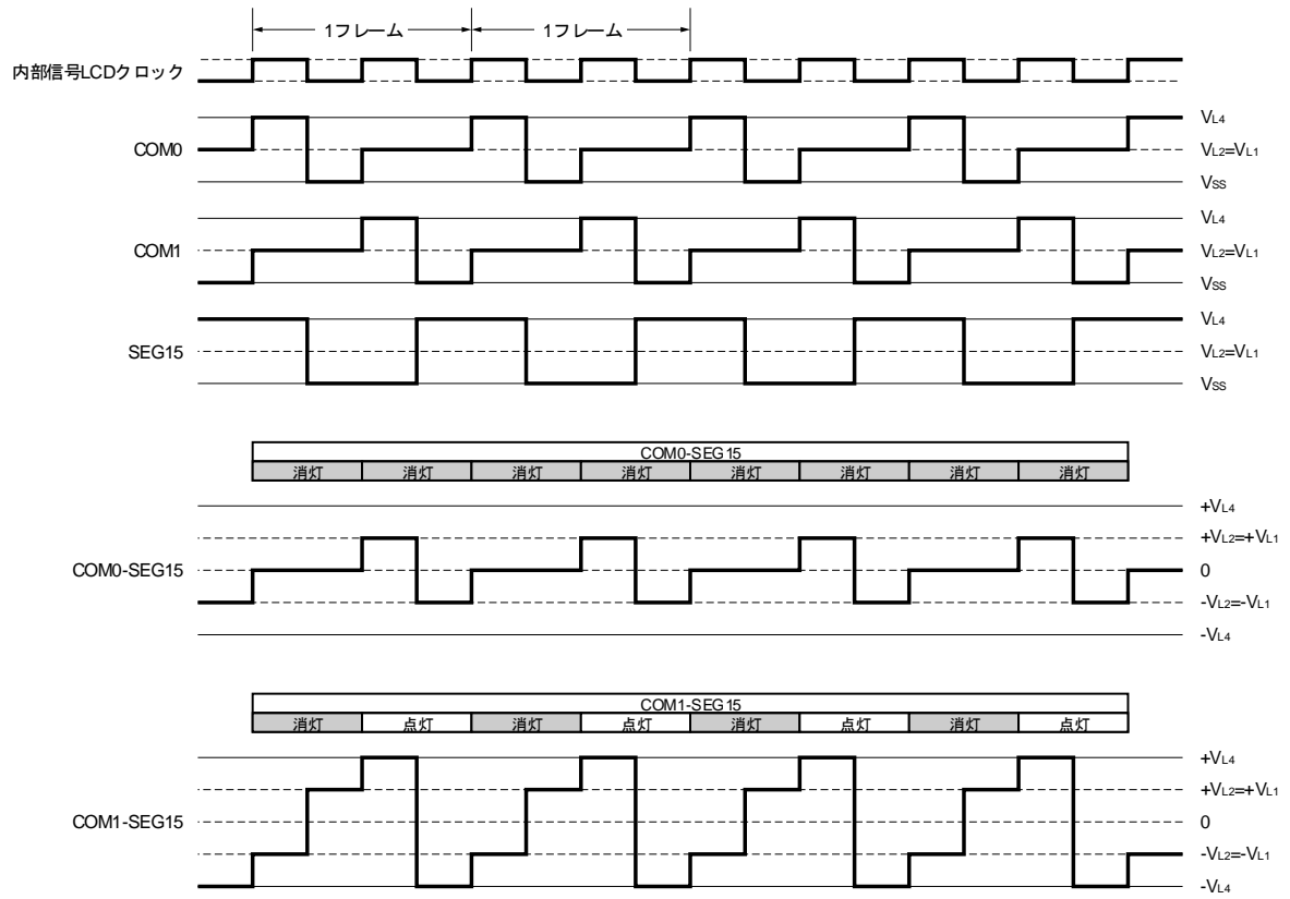
図16-31 SEG15と各コモン信号間の2時分割LCD駆動波形例（1/2バイアス法）
