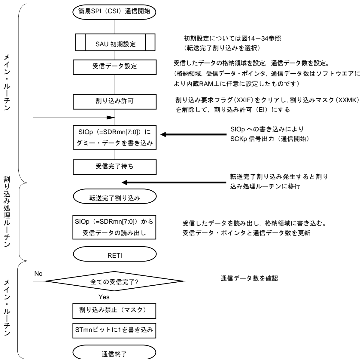
図14-38 マスタ受信（シングル受信モード時）のフロー・チャート
