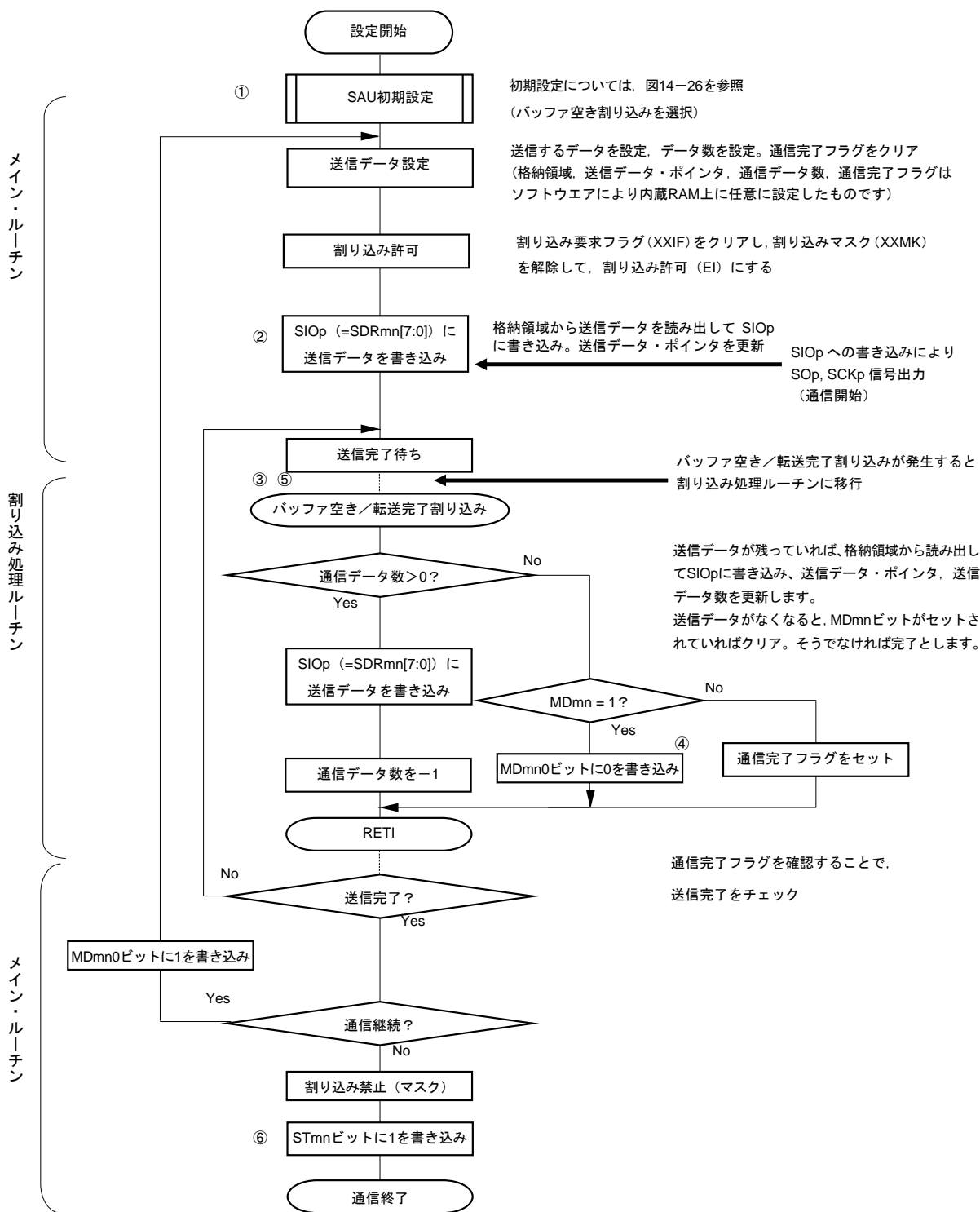
図14-32 マスタ送信（連続送信モード時）のフロー・チャート
