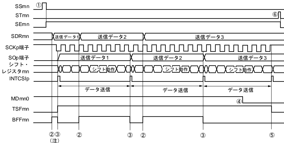
図14-55 スレーブ送信（連続送信モード時）のタイミング・チャート（タイプ1：DAPmn = 0, CKPmn = 0）
