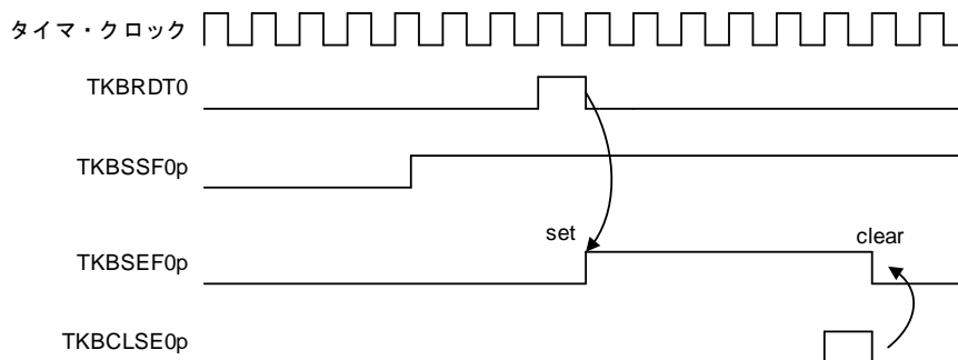
図7-62 ソフト・スタート機能動作中 (TKBSSF0p = 1) のTKBCR00/TKBCR01/TKBCR02/TKBCR03/TKBSIR00/TKBSIR01/TKBSSR00/TKBSSR01レジスタの書き換え
