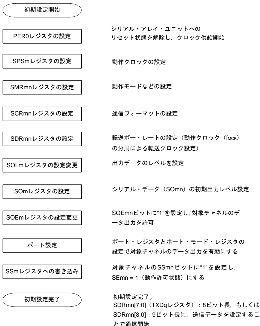
図14-77 UART送信の初期設定手順
