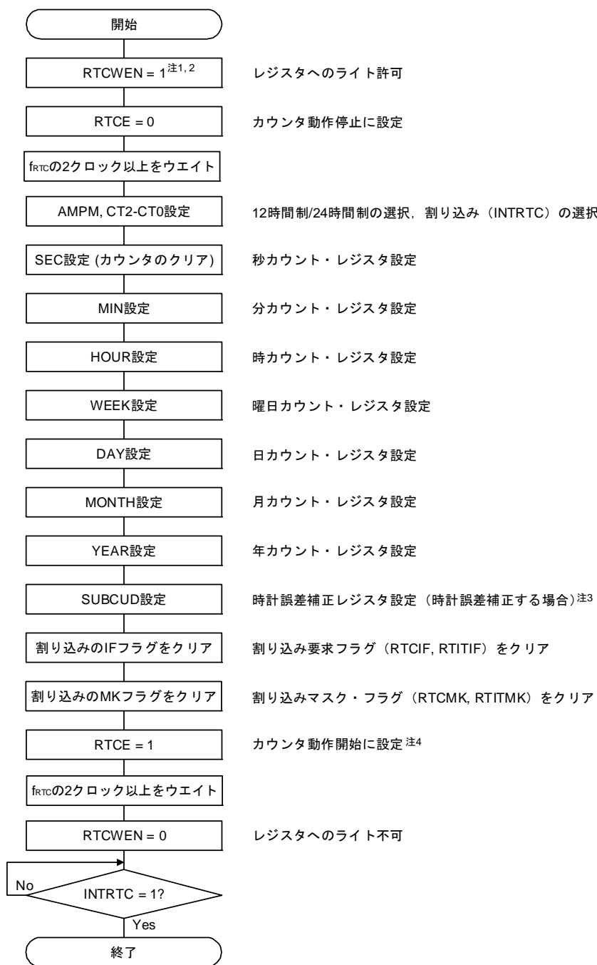
図8-18 リアルタイム・クロック2の動作開始手順
