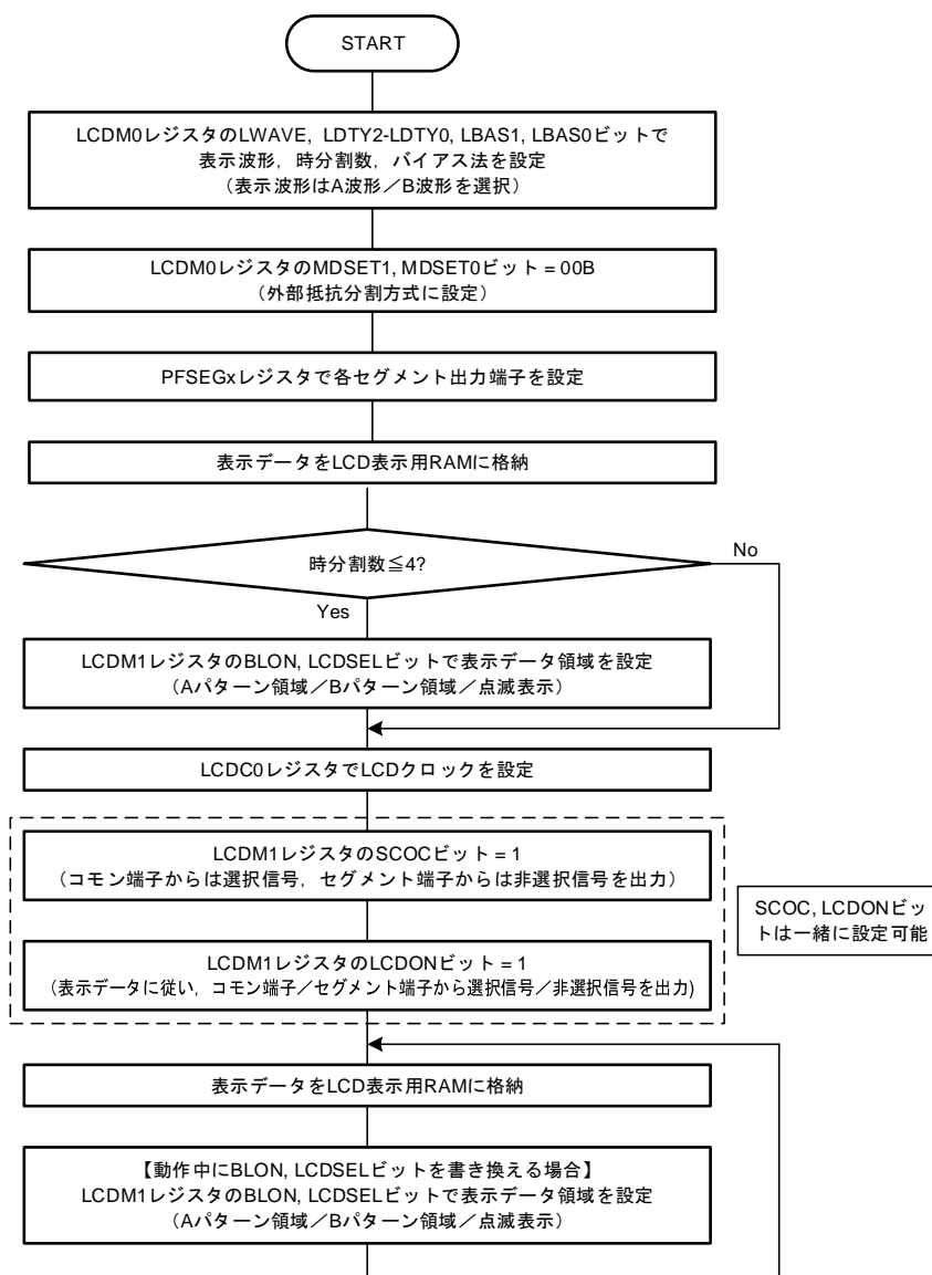
図16-17 外部抵抗分割方式の設定手順
