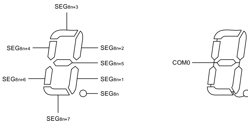
図16-26 スタティックLCDの表示パターンと電極結線
