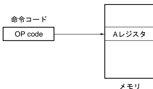
図3-20 インプライド・アドレッシングの概略
