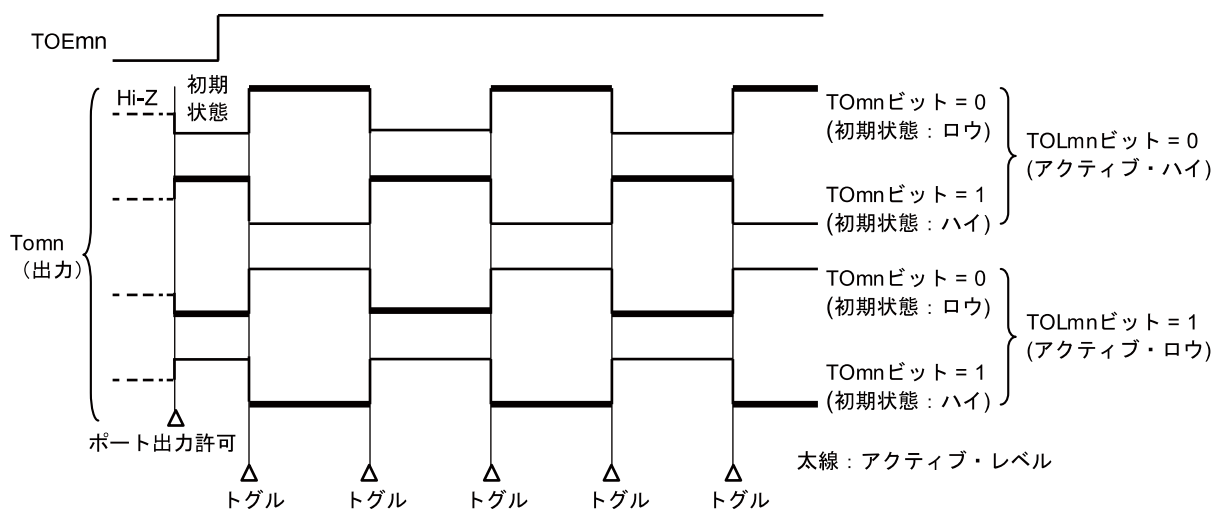
図6-34 トグル出力時 (TOMmn = 0) のTOmn端子出力状態
