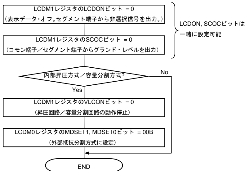
図16-20 動作停止手順
