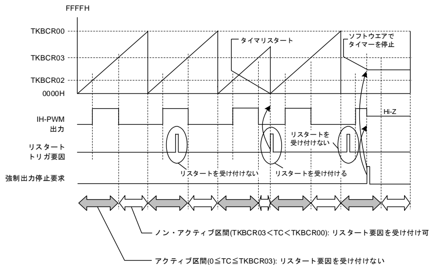
図7-65 IH制御用のPWM出力機能
