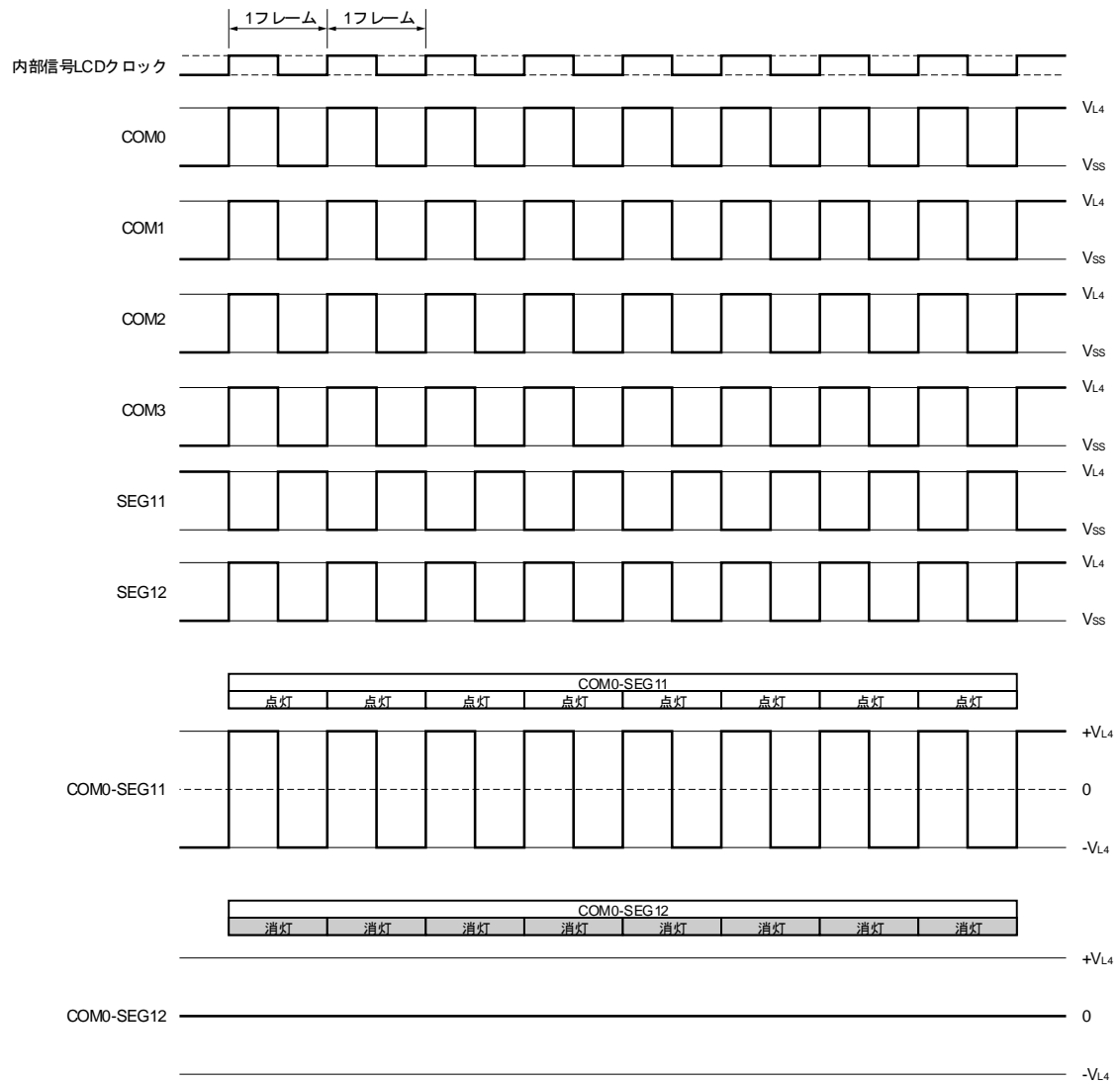
図16-28 SEG11, SEG12とCOM0とのスタティックLCD駆動波形例
