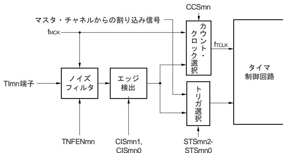
図6-41 入力回路構成図
