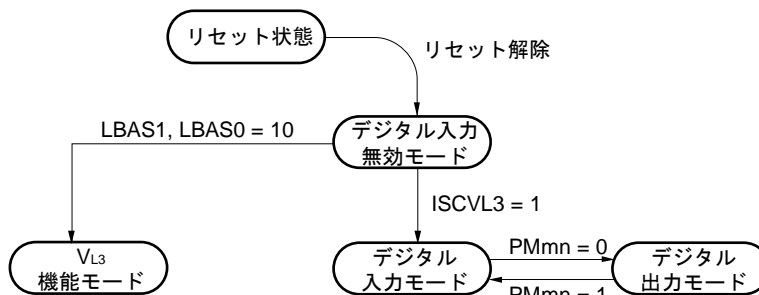
図4-14 VL3/P125端子機能の状態遷移図
