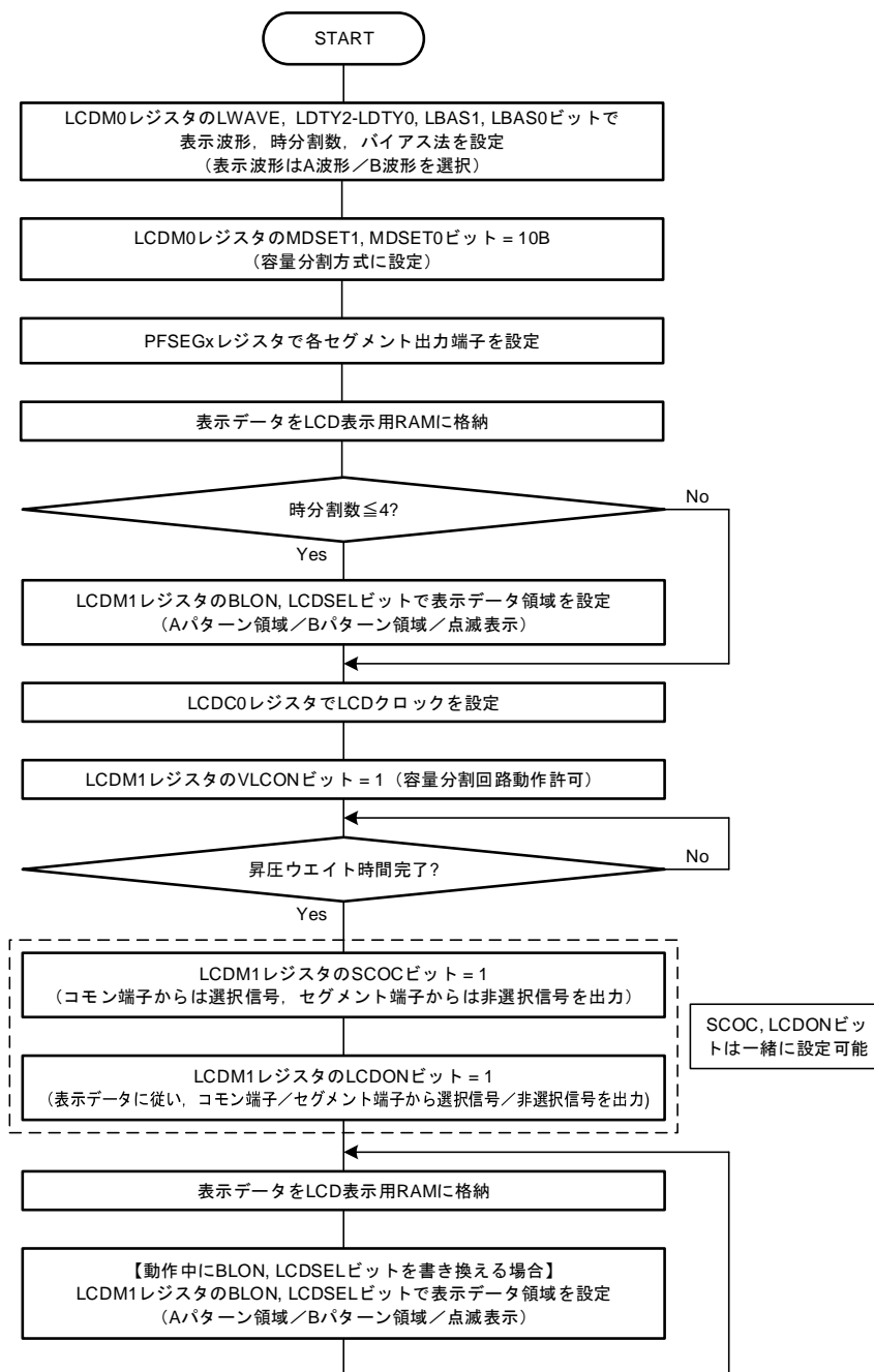
図16-19 容量分割方式の設定手順
