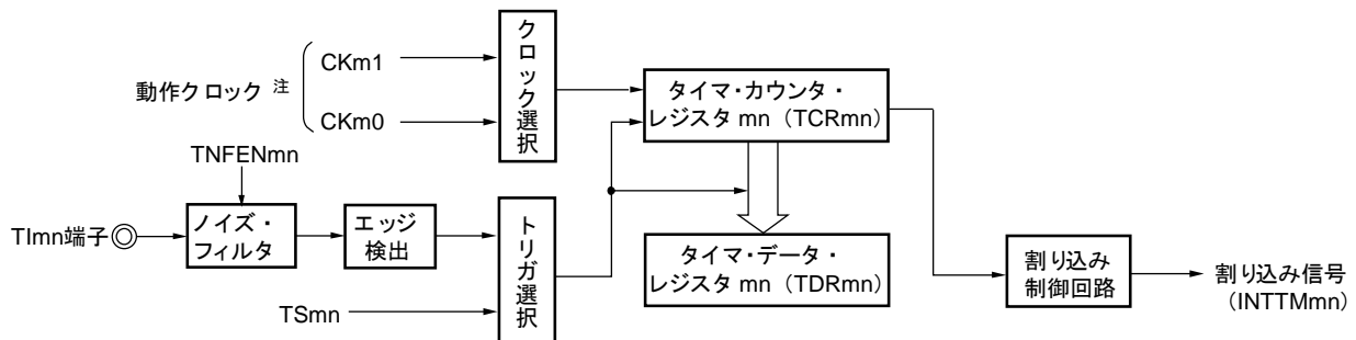
図6-51 入力パルス間隔測定としての動作のブロック図
