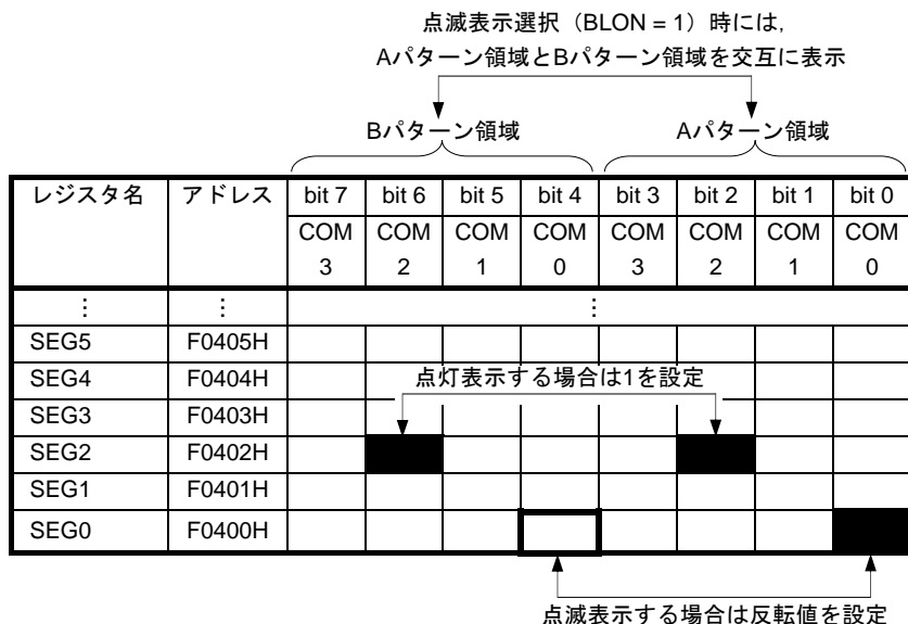
図16-14 パターン切り替え表示時のLCD表示レジスタの設定例
