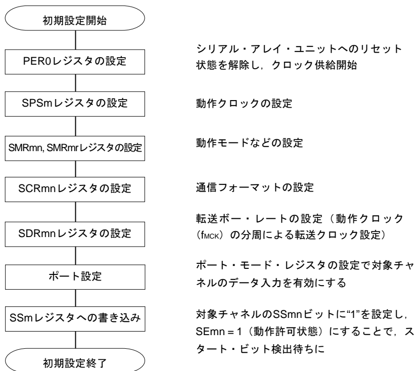
図14-85 UART受信の初期設定手順
