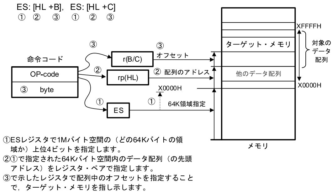
図3-36 ES:[HL+B], ES:[HL+C]の例
