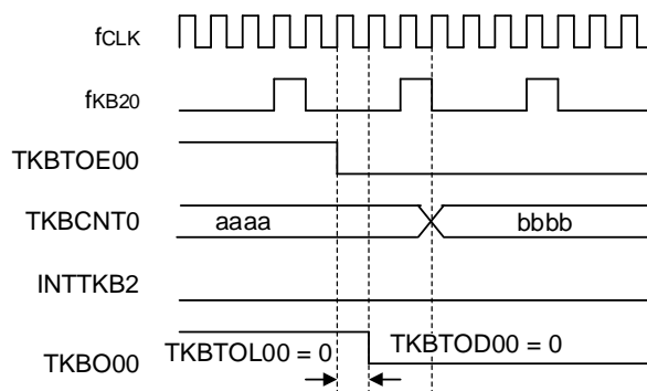
図7-30 デフォルトレベルとアクティブ・レベルのタイミング図 (TKBTOE00を“1”から“0”に変更した場合)
