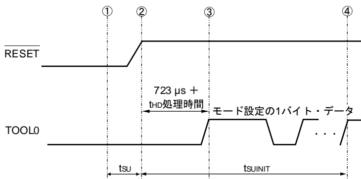
図28-7 フラッシュ・メモリ・プログラミング・モードへの引き込み
