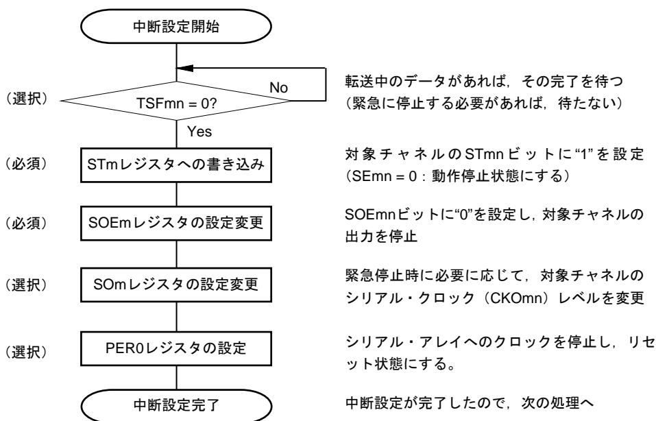
図14-35 マスタ受信の中断手順
