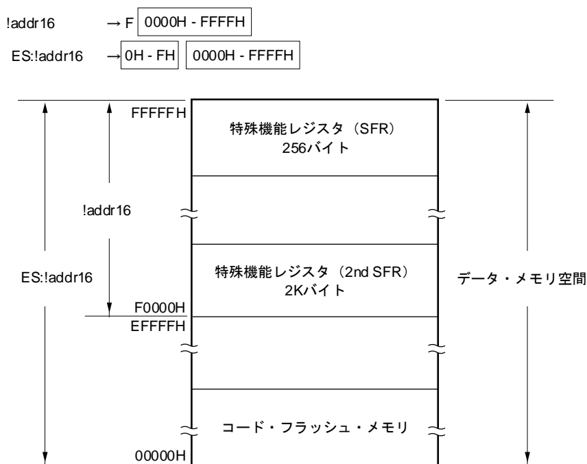
図3-14 データ・アクセス領域の拡張
