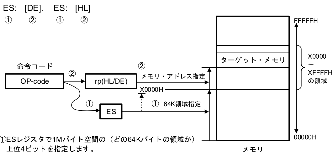
図3-27 ES:[DE], ES:[HL]の例
