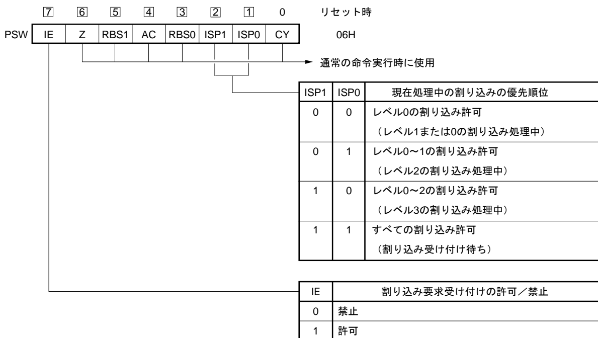
図19-6 プログラム・ステータス・ワードの構成
