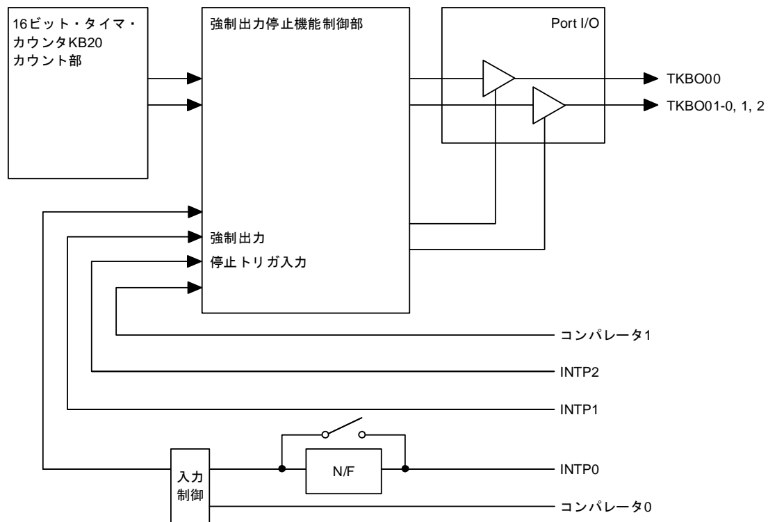
図7-68 強制出力停止機能のシステム構成図
