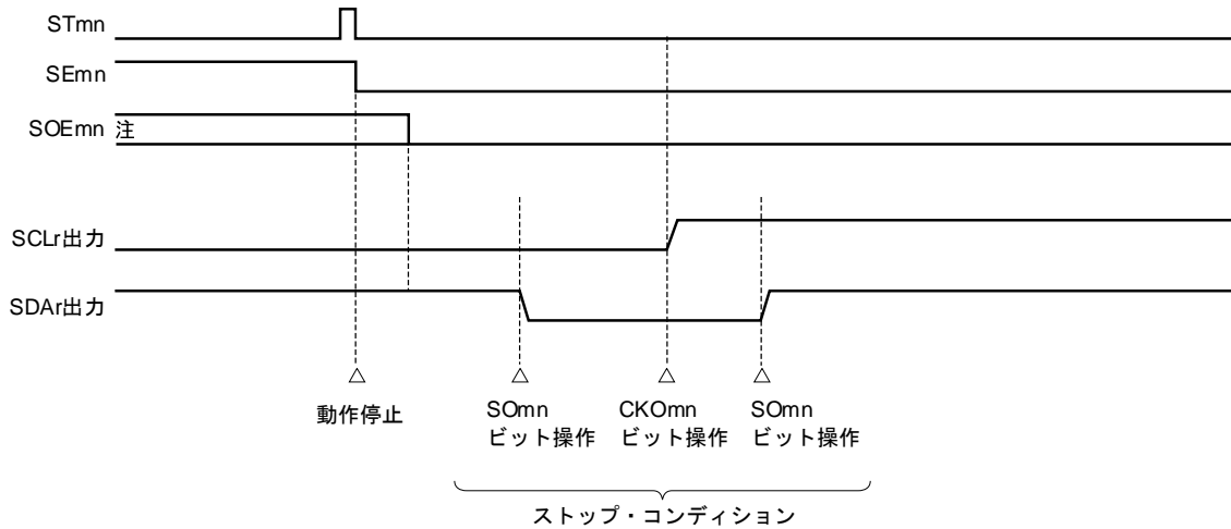
図14-113 ストップ・コンディション発生のタイミング・チャート
