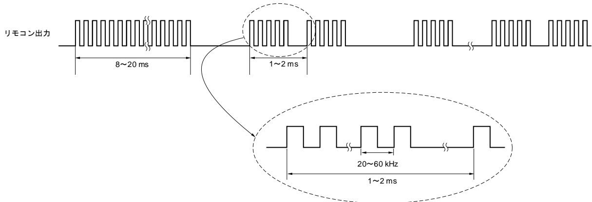
図6-78 リモコン出力
