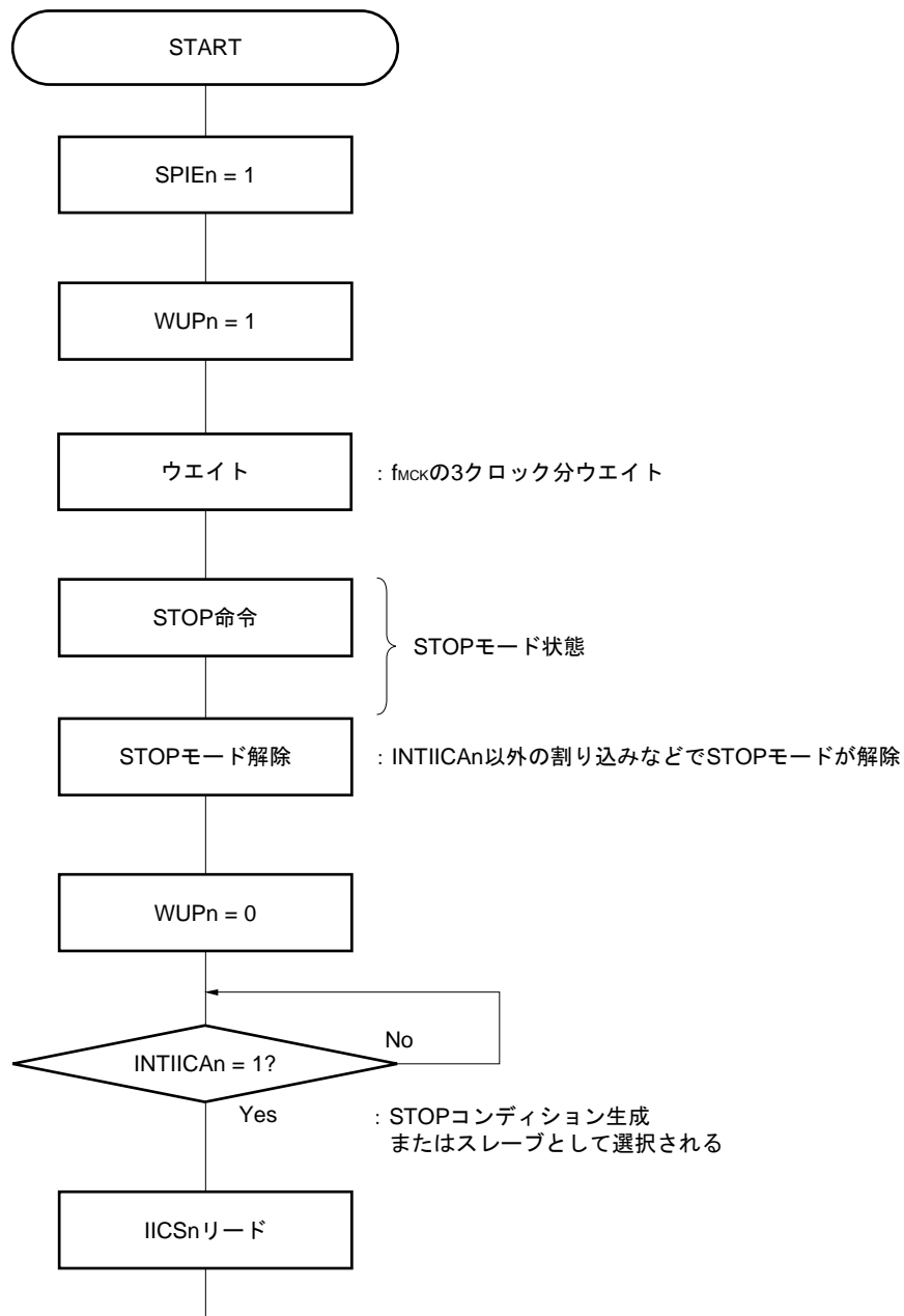
図15-24 INTIICAn以外でSTOPモードが解除後にマスタとして動作させる場合
