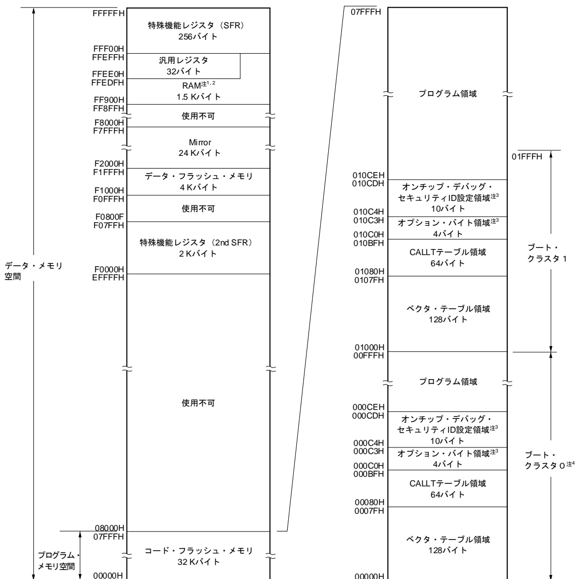
図3-2 メモリ・マップ (R5F10WLC, R5F10WMC)
