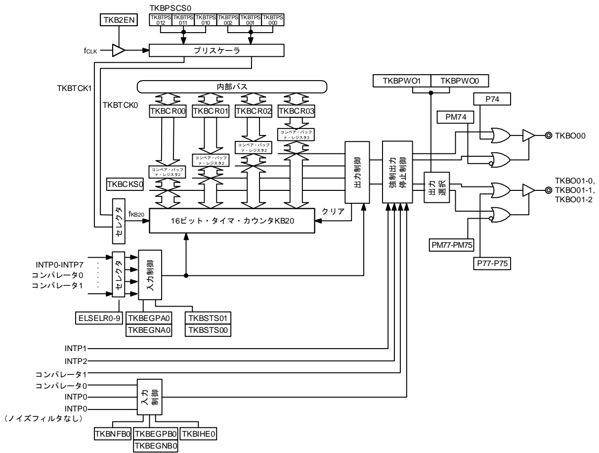
図7-1 16ビット・タイマKB20のブロック図
