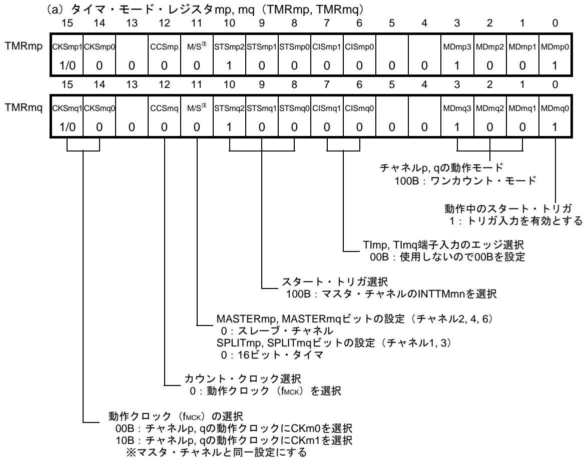
図6-76 多重PWM機能時（スレーブ・チャンネル）のレジスタ設定内容例（2種類のPWMを出力する場合）
