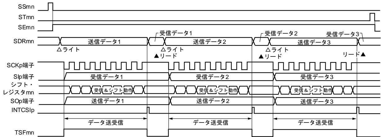
図14-45 マスタ送受信（シングル送受信モード時）のタイミング・チャート（タイプ1：DAPmn = 0, CKPmn = 0）
