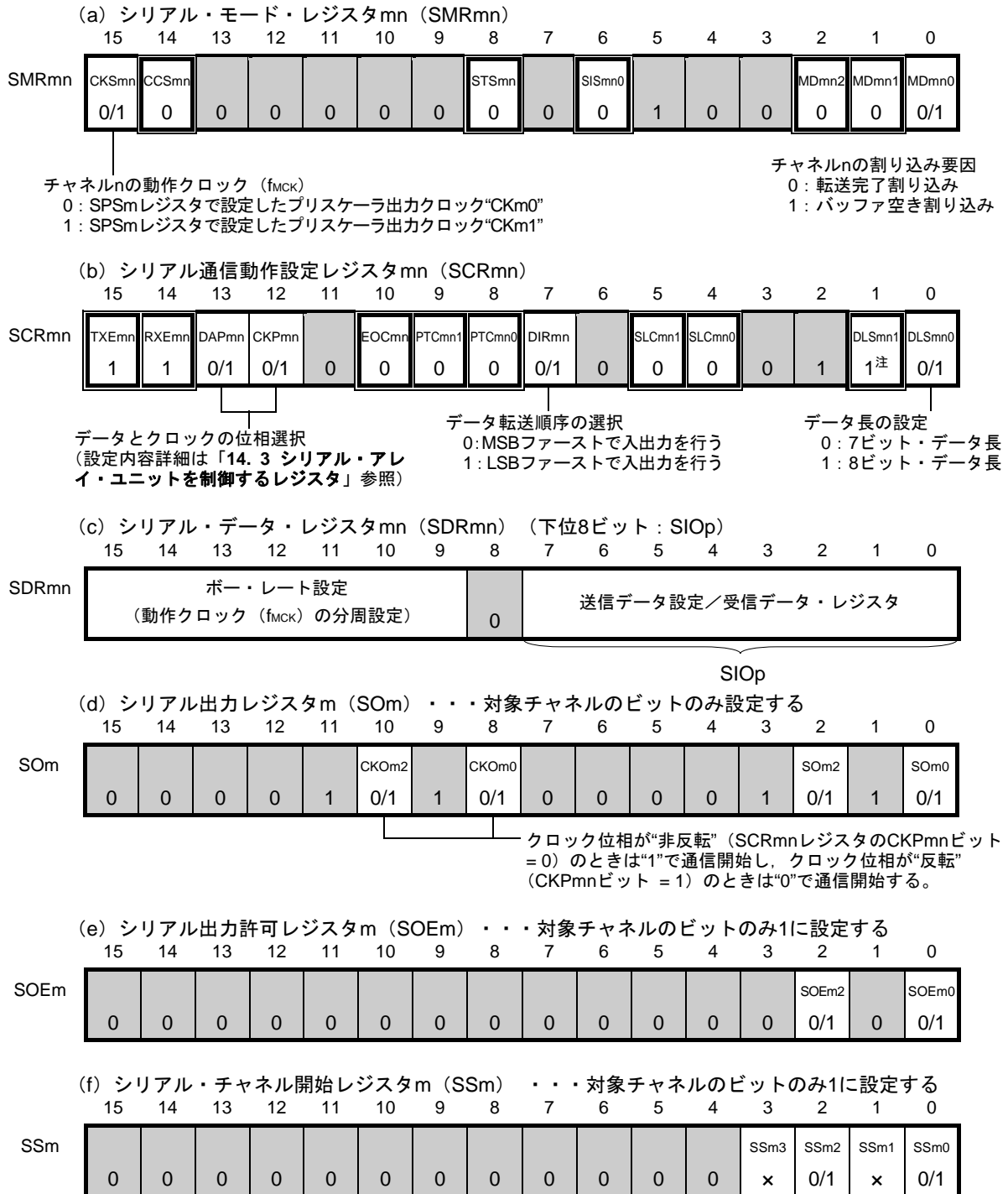
図14-41 簡易SPI (CSI00, CSI10) のマスタ送受信時のレジスタ設定内容例
