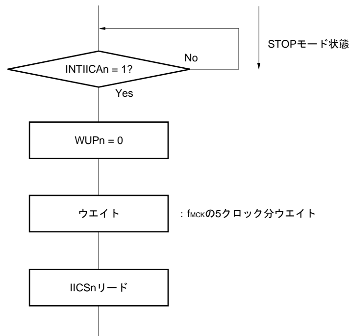
図15-23 アドレス一致によりWUPn = 0に設定する場合のフロー（拡張コード受信含む）
