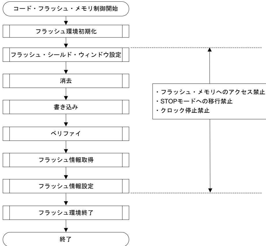
図28-8 セルフ・プログラミング（フラッシュ・メモリの書き換え）の流れ
