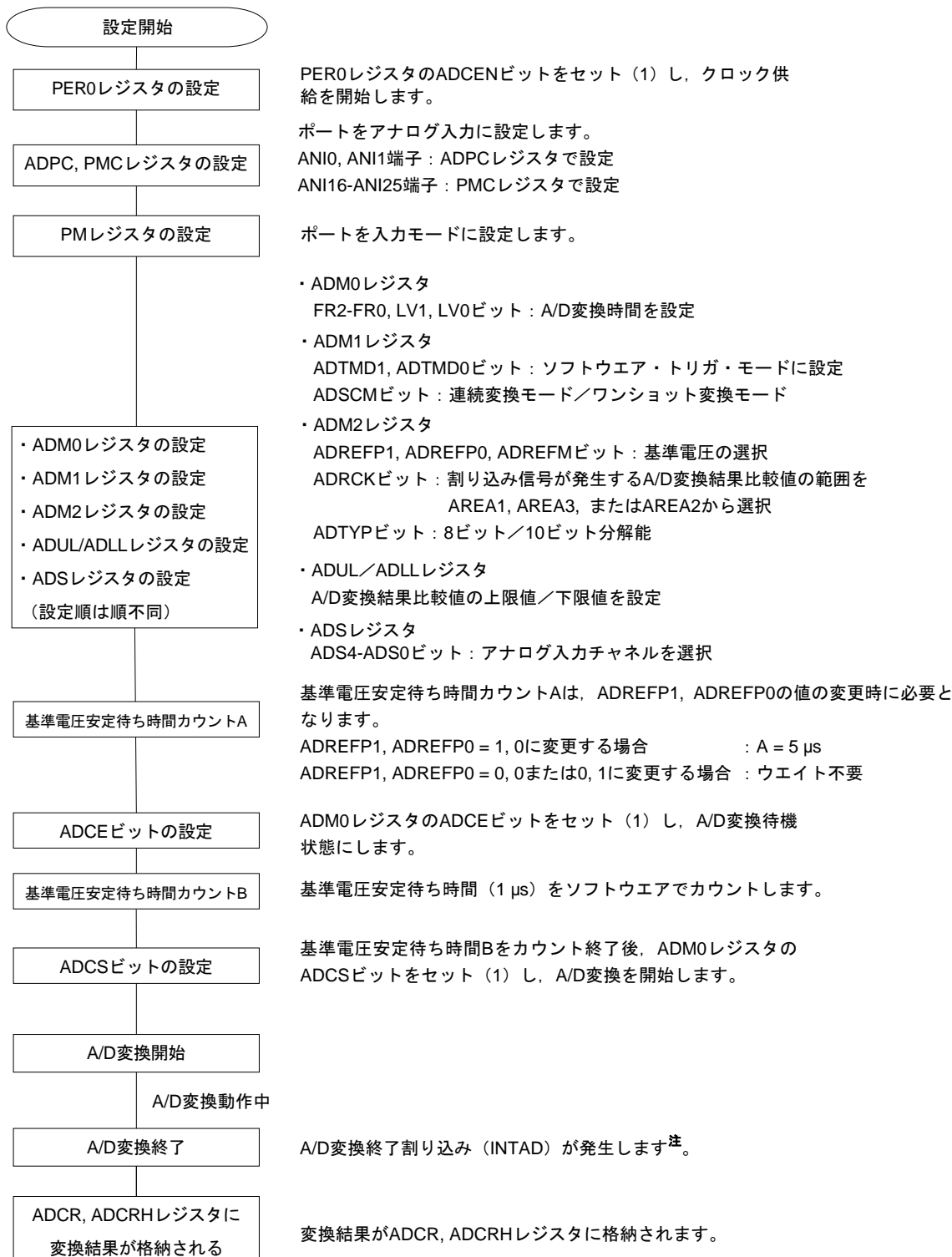
図12-23 ソフトウェア・トリガ・モード設定
