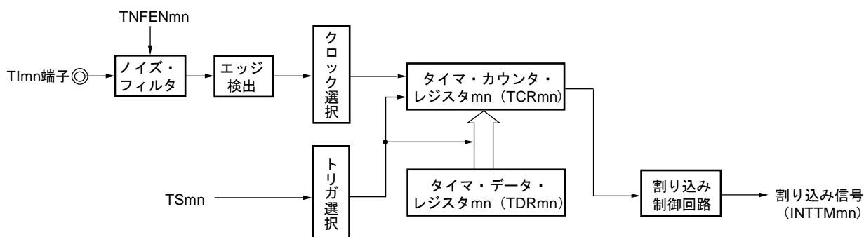
図6-47 外部イベント・カウンタとしての動作のブロック図
