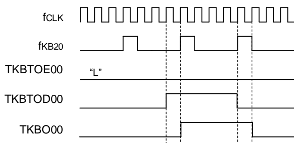
図7-33 デフォルトレベルとアクティブ・レベルのタイミング図 (TKBTOE00 = 0でTKBTOD00を変更した場合)
