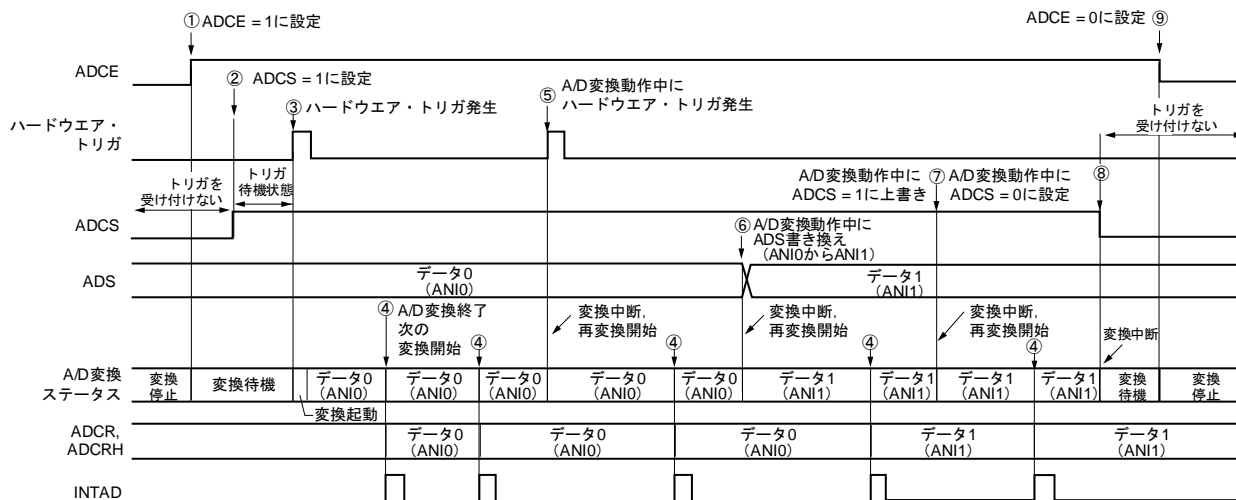
図12-19 ハードウェア・トリガ・ノーウエイト・モード（連続変換モード）動作タイミング例
