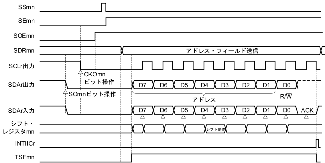
図14-105 アドレス・フィールド送信のタイミング・チャート
