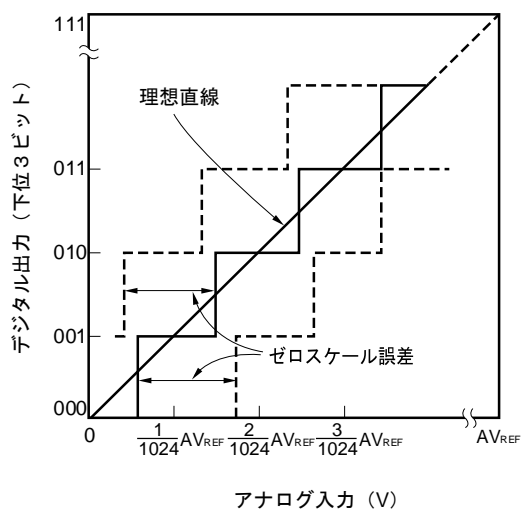
図12-34 ゼロスケール誤差
