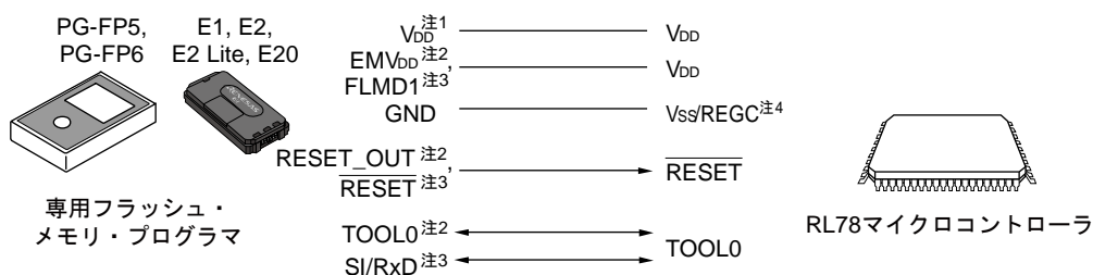
図28-2 専用フラッシュ・メモリ・プログラマとの通信
