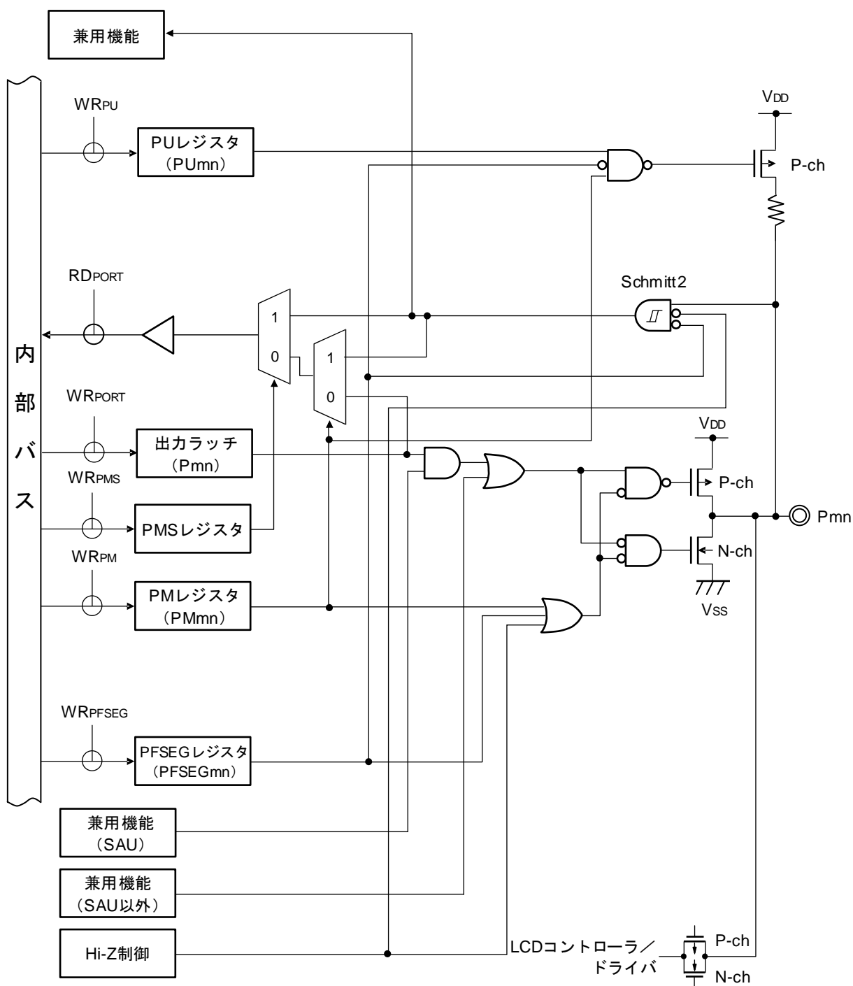
図2-10 端子タイプ 7-5-16 の端子ブロック図
