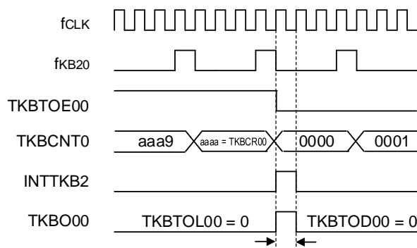
図7-32 デフォルトレベルとアクティブ・レベルのタイミング図 (TKBTOE00の操作がタイマ・カウント・クロックの発生と同時の場合)
