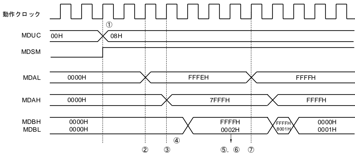
図17-7 乗算（符号付）動作のタイミング図（ -2 \times 32767 = -65534 ）
