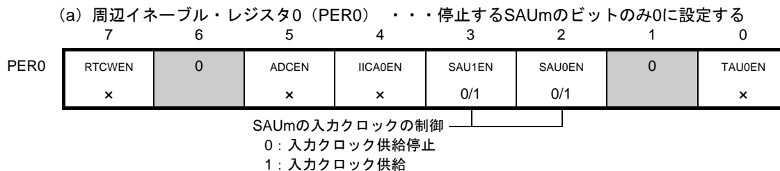
図14-23 ユニット単位で動作停止とする場合の周辺イネーブル・レジスタ0 (PER0) の設定
