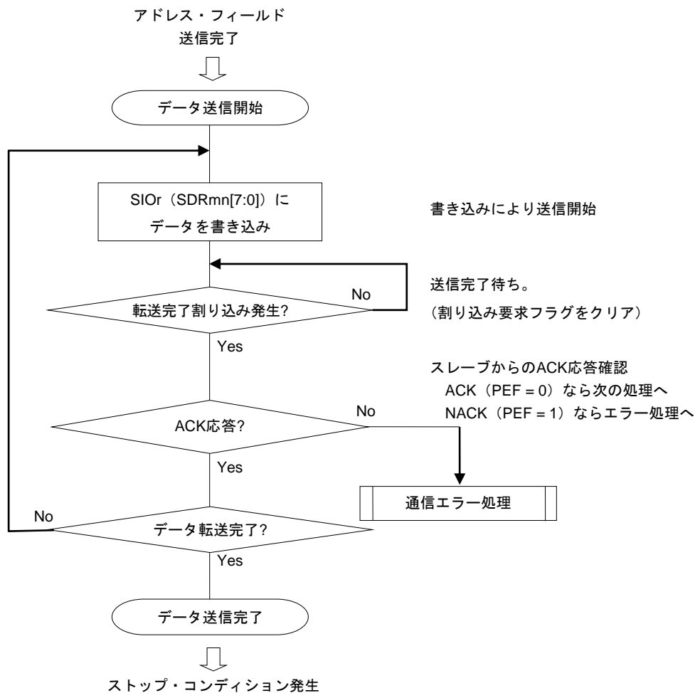
図14-109 簡易I 2 Cデータ送金のフロー・チャート
