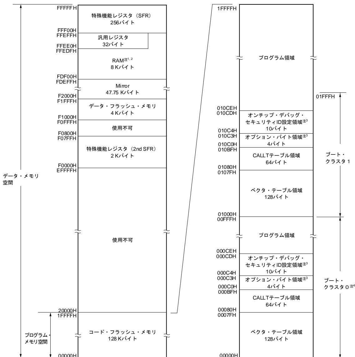
図3-6 メモリ・マップ (R5F10WLG, R5F10WMG)
