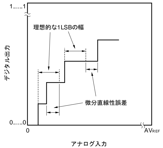
図12-37 微分直線性誤差
