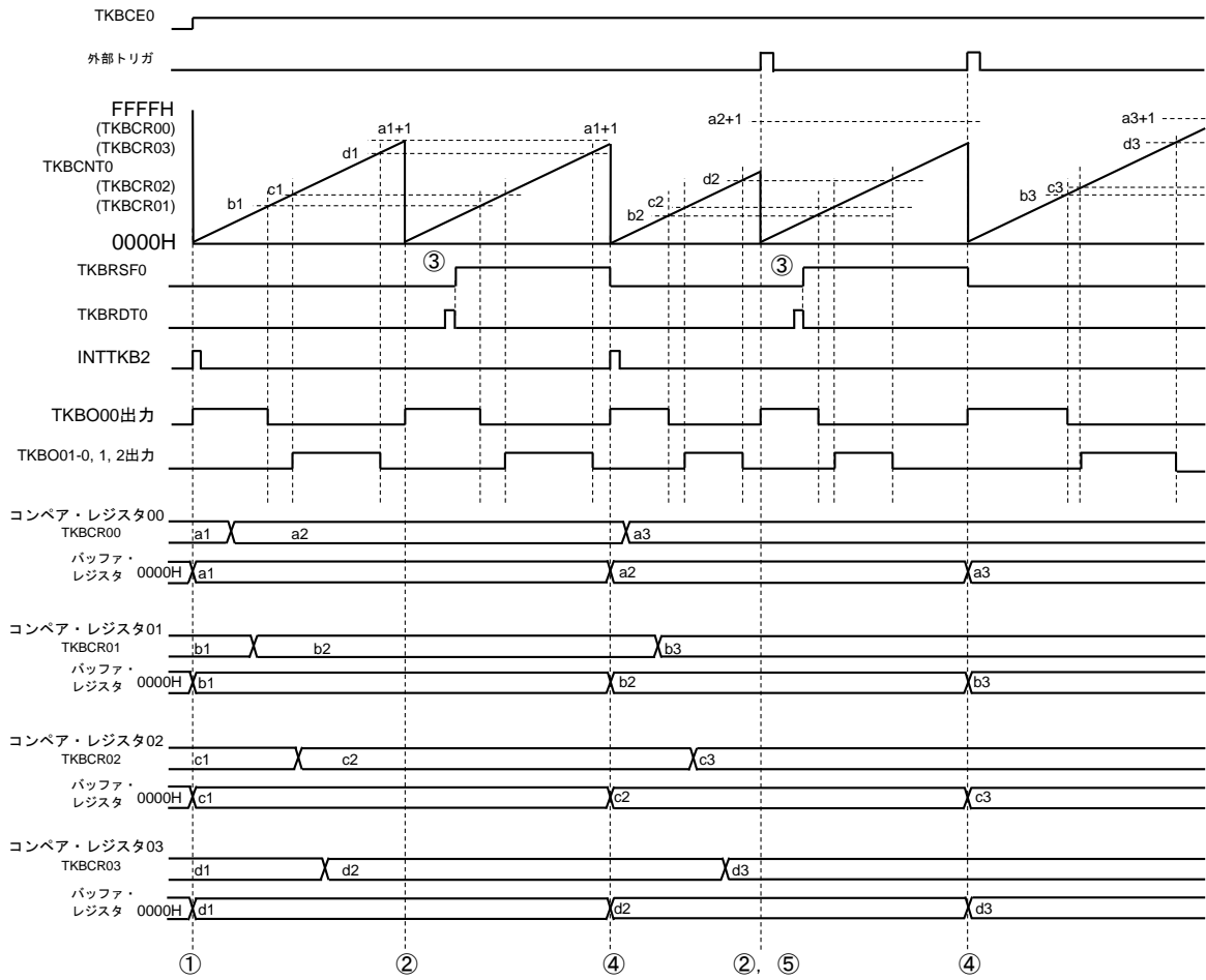
図7-45 一斉書き換え機能：外部トリガ入力による周期制御での単体動作時、カウント動作中のバッファ更新タイミング図（TKBTSE0ビットを1に設定）
