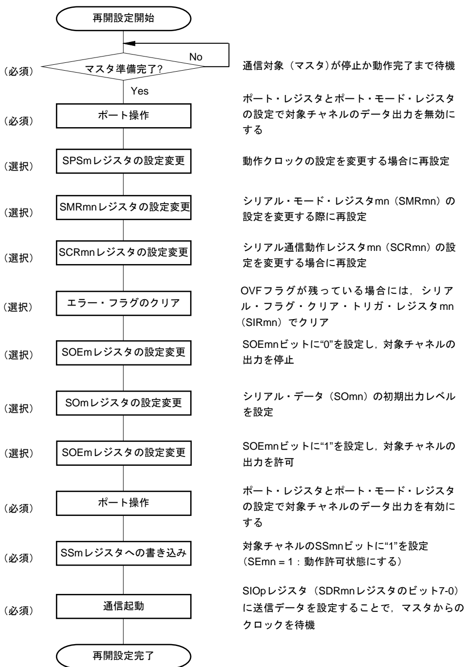
図14-66 スレーブ送受信の再開設定手順
