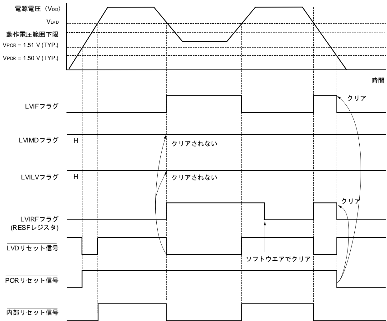
図24-5 内部リセット信号発生タイミング (オプション・バイトのLVIMDS1, LVIMDS0 = 1, 1)
