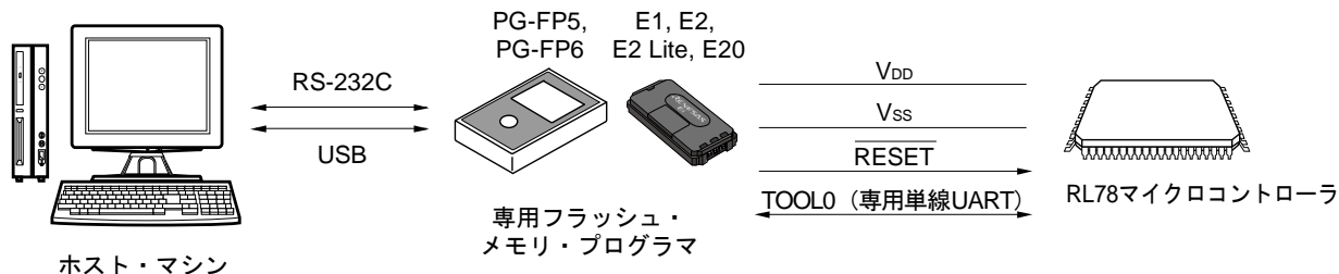
図28-1 フラッシュ・メモリにプログラムを書き込むための環境
