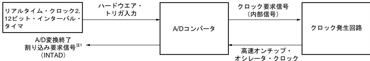
図12-28 SNOOZEモード機能時のブロック図
