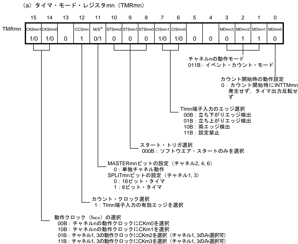
図6-49 外部イベント・カウンタ・モード時のレジスタ設定内容例
