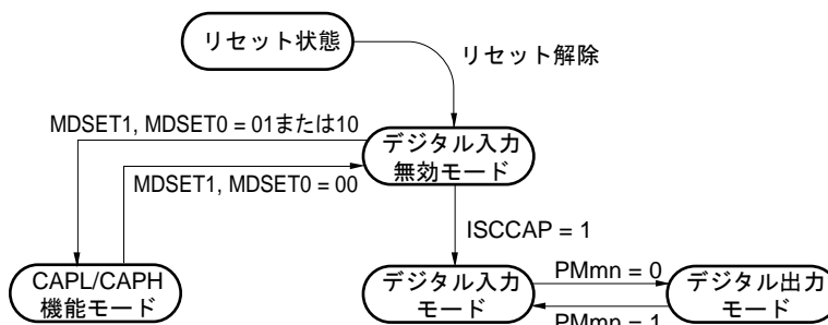
図16-9 CAPL/P126, CAPH/P127端子機能の状態遷移図
