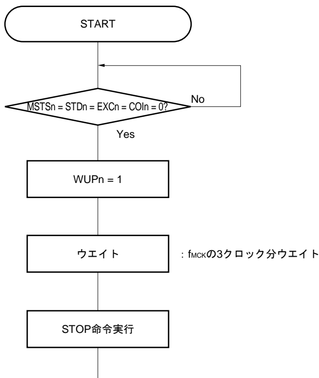
図15-22 WUPn = 1を設定する場合のフロー
