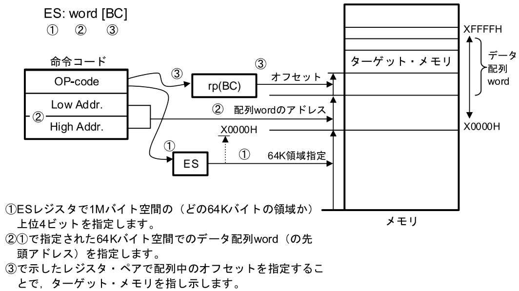
図3-34 ES:word[BC]の例
