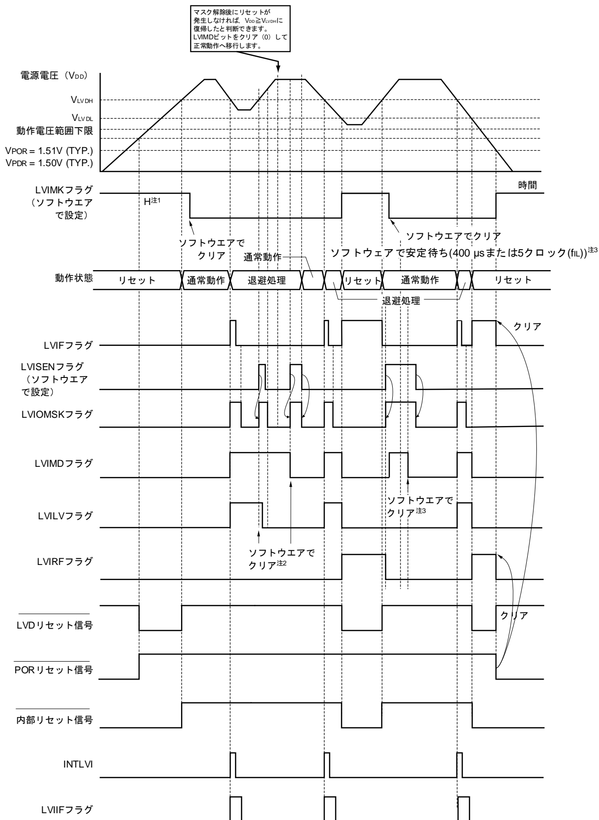
図24-7 割り込み&リセット信号発生タイミング (オプション・バイトのLVIMDS1, LVIMDS0 = 1, 0) (1/2)
