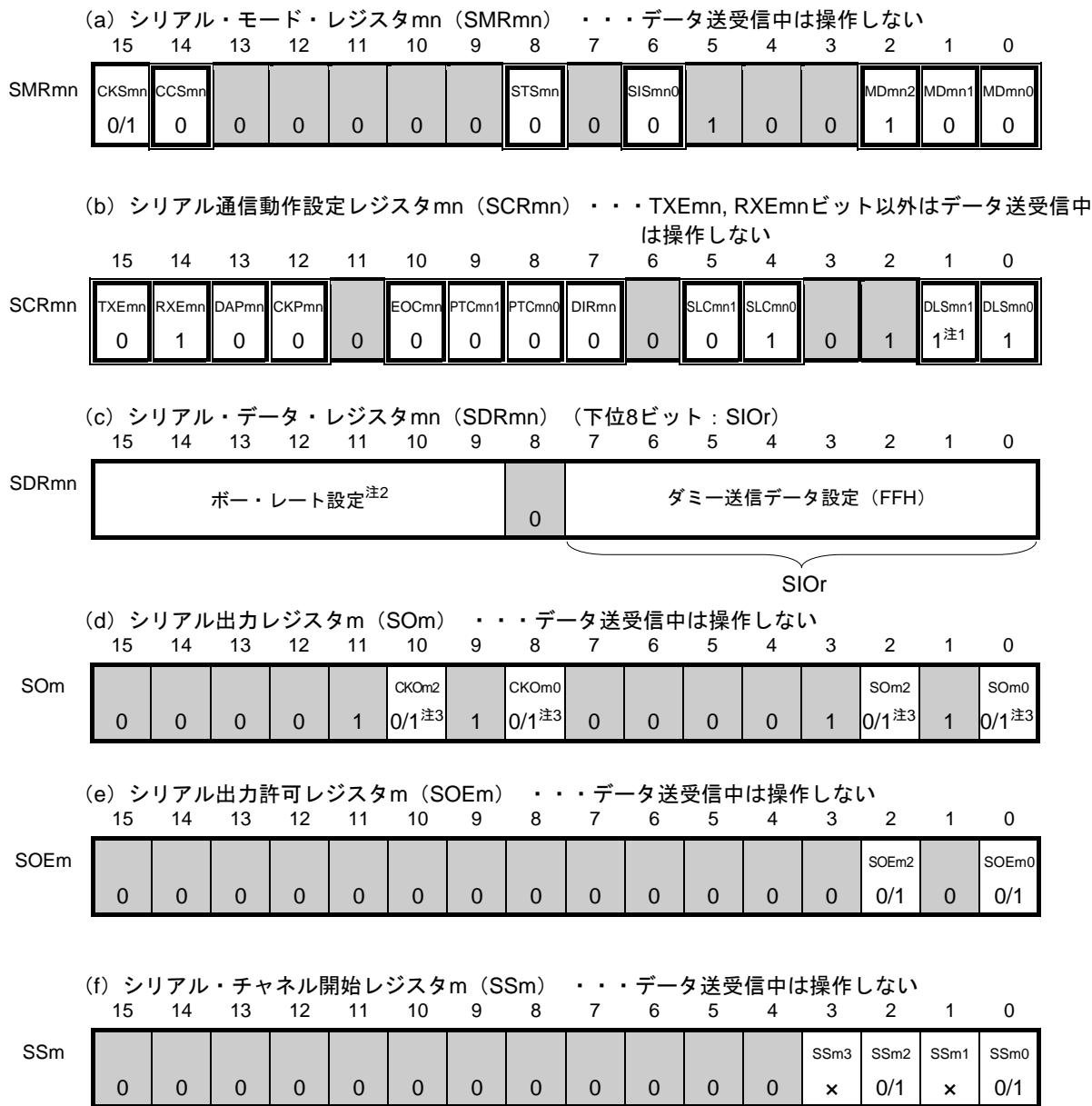
図14-110 簡易I 2 C (IIC00, IIC10) のデータ受信時のレジスタ設定内容例
