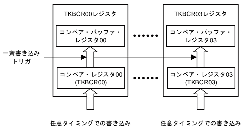
図7-39 コンペア・レジスタ一斉書き換え機能
