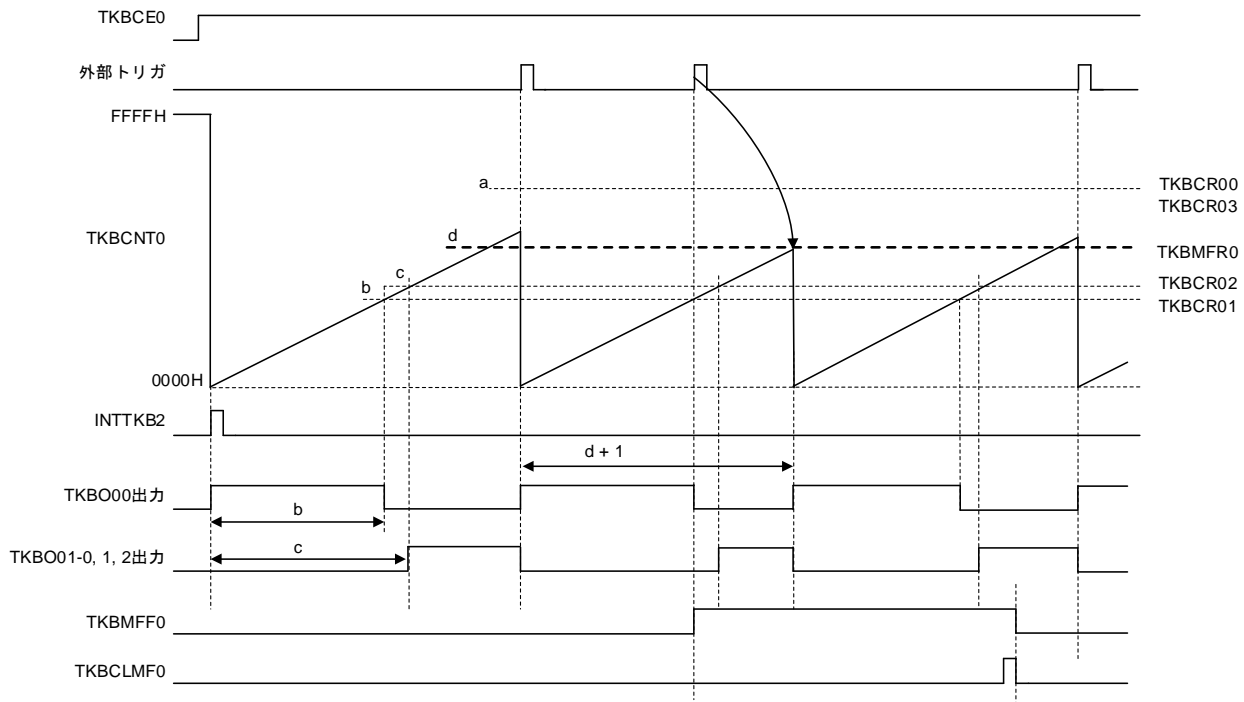
図7-64 最大周波数リミット機能
