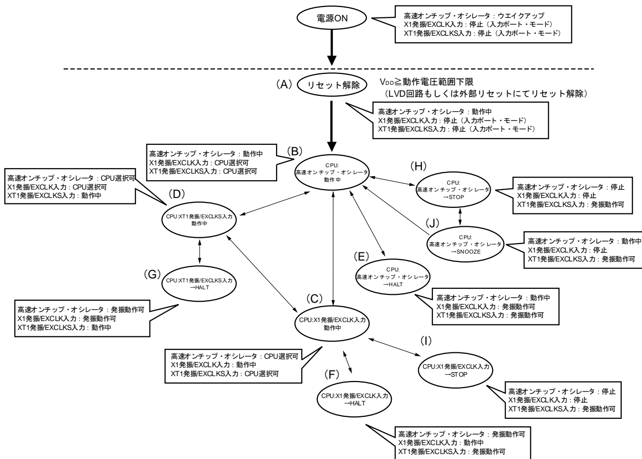
図5-16 CPUクロック状態移行図
