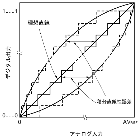
図12-36 積分直線性誤差
