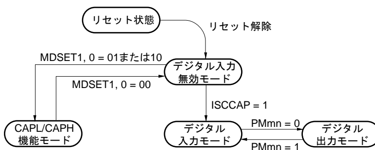
図4-15 CAPL/P126, CAPH/P127端子機能の状態遷移図
