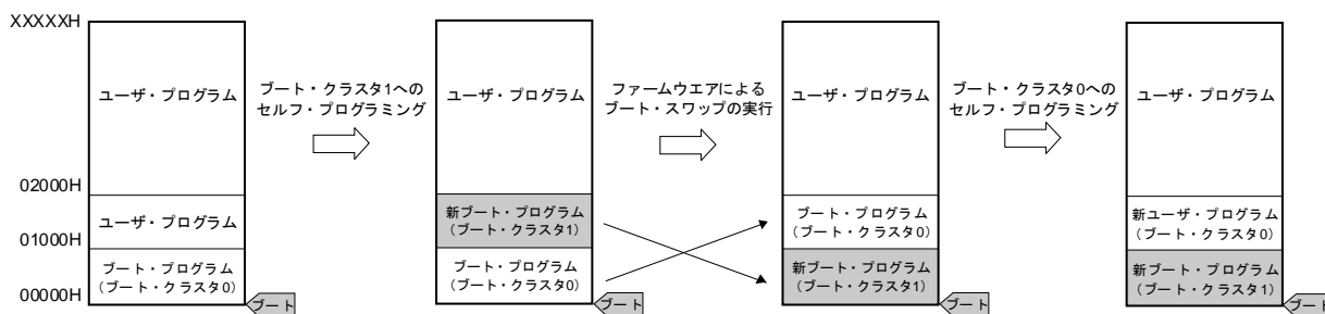
図28-9 ブート・スワップ機能
