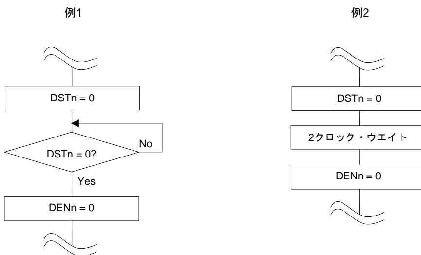
図18-11 DMA転送の強制終了 (1/2)
