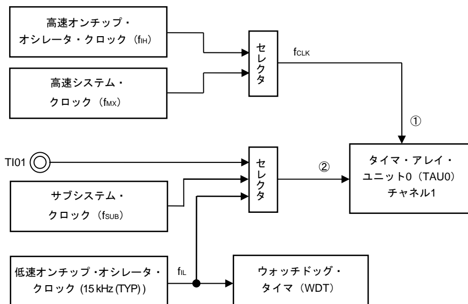
図25-13 周波数検出機能の構成
