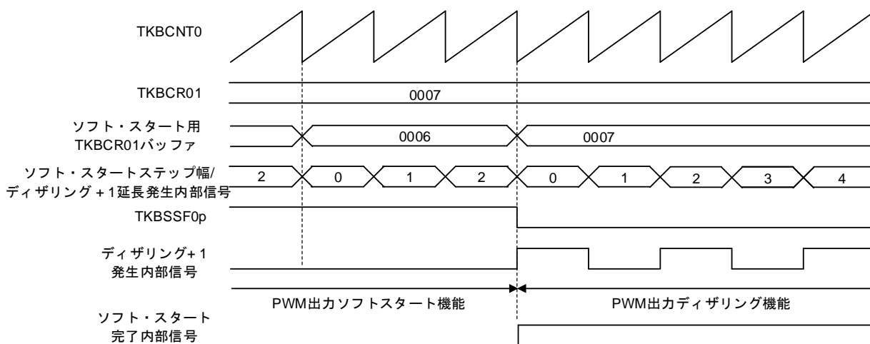
図7-63 PWM出力ソフト・スタート機能の完了とTKBSSF0pの動作
