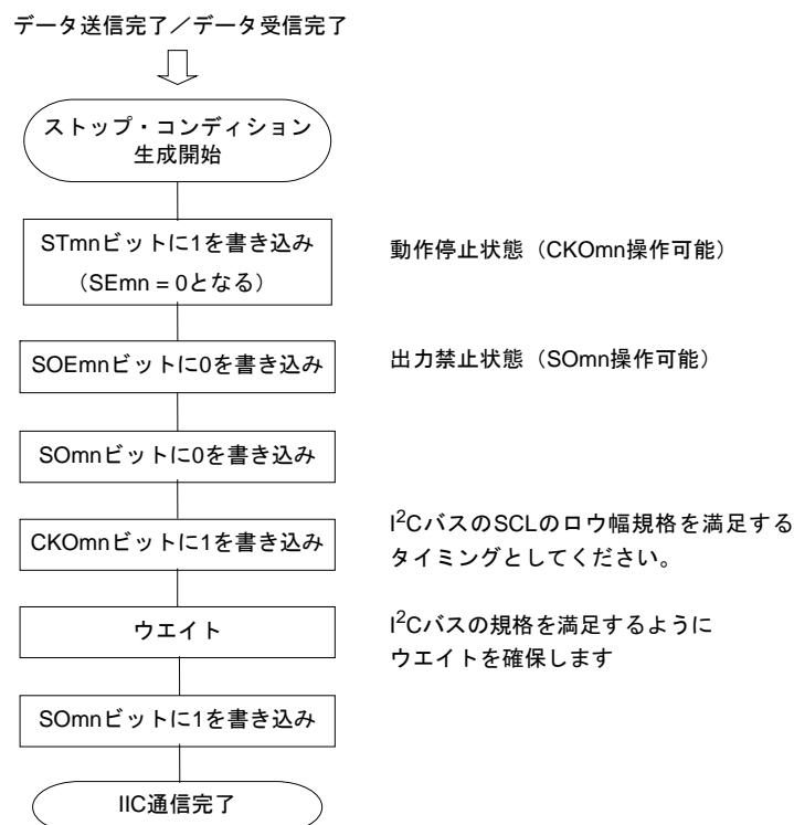
図14-114 ストップ・コンディション発生のフロー・チャート
