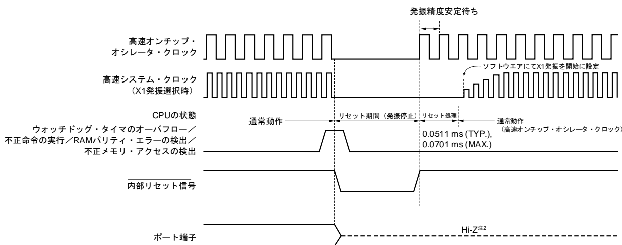
図22-3 ウォッチドッグ・タイマのオーバーフロー／不正命令の実行／RAMパリティ・エラーの検出／不正メモリ・アクセスの検出によるリセット・タイミング
