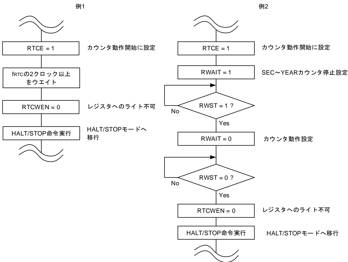
図8-19 RTCE = 1に設定後のHALT/STOPモードへの移行手順
