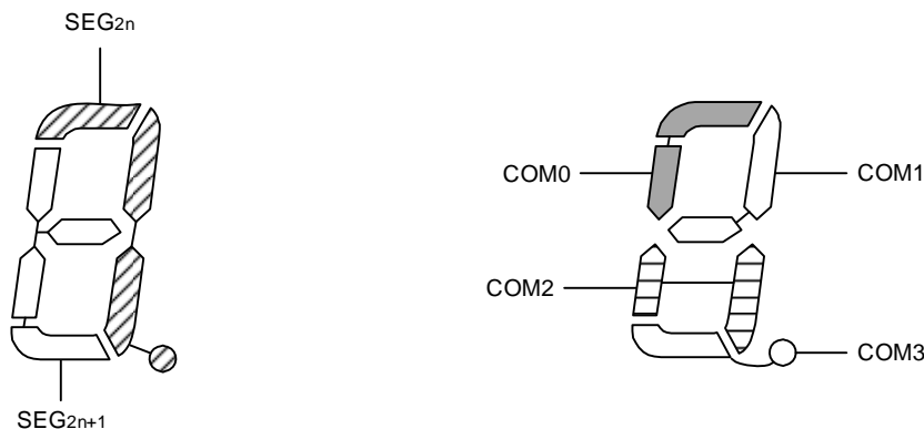
図16-36 4時分割LCD表示パターンと電極結線
