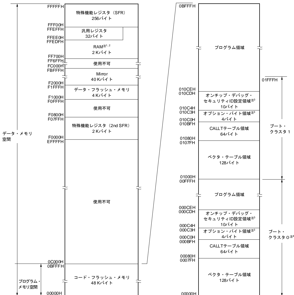
図3-3 メモリ・マップ (R5F10WLD, R5F10WMD)
