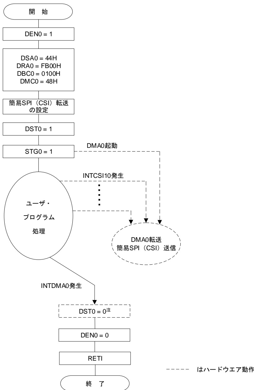
図18-7 簡易SPI (CSI) 連続送信の設定例
