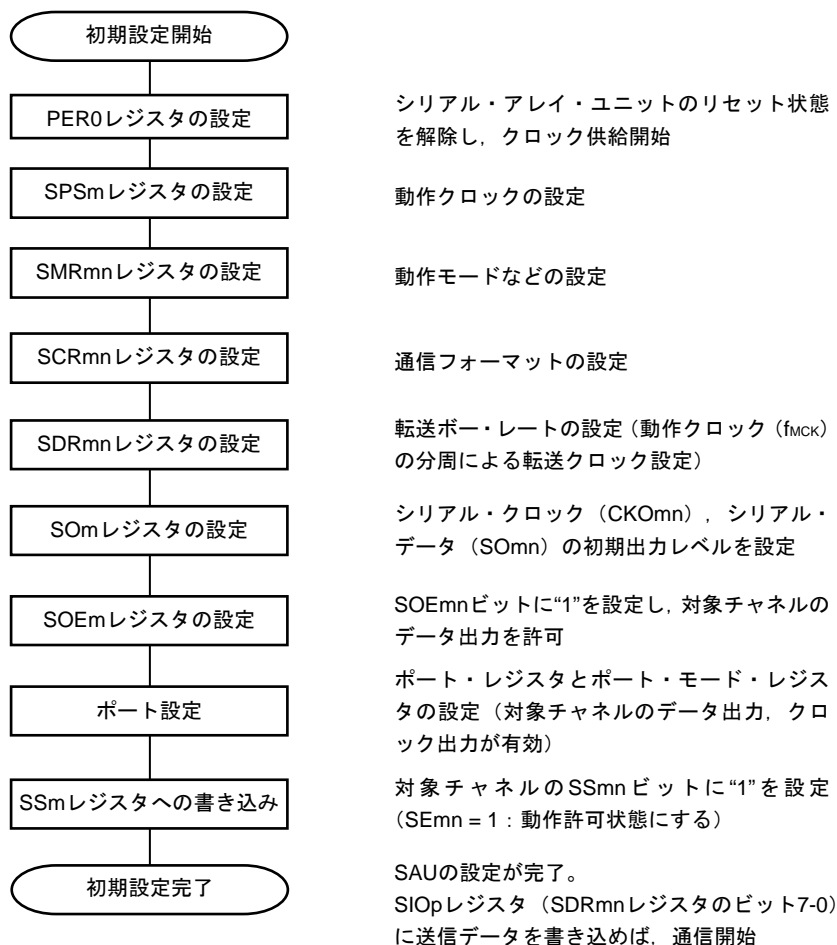
図14-26 マスタ送信の初期設定手順
