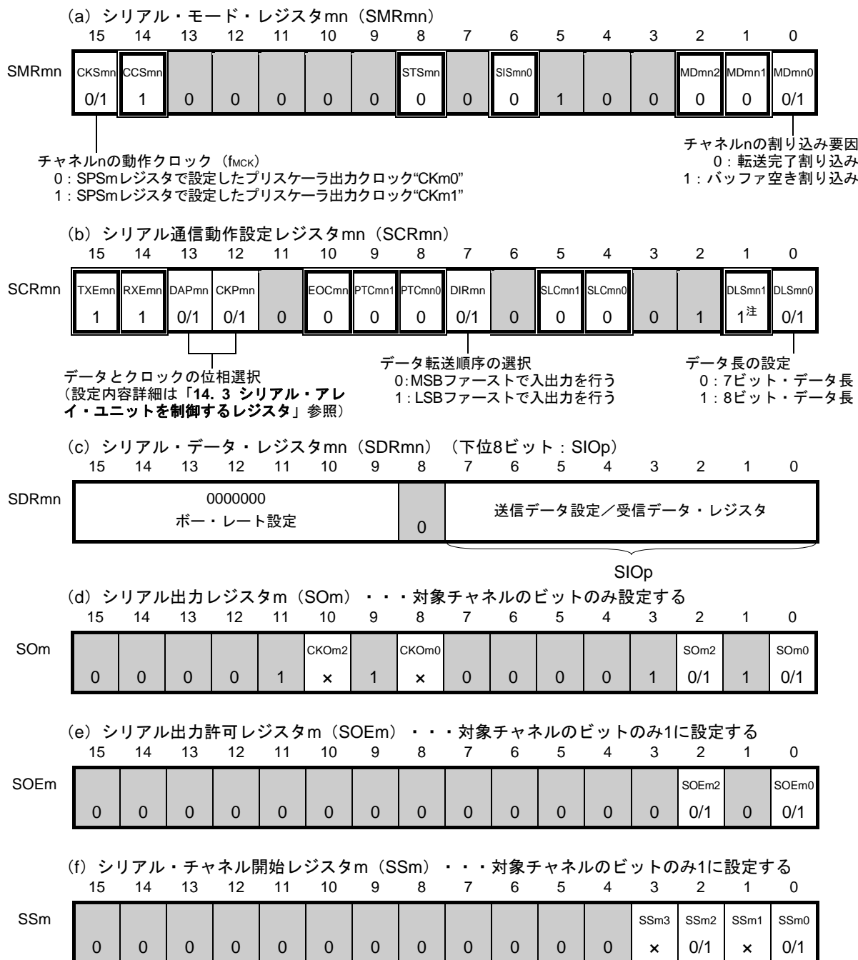
図14-63 簡易SPI (CSI00, CSI10) のスレーブ送受信時のレジスタ設定内容例
