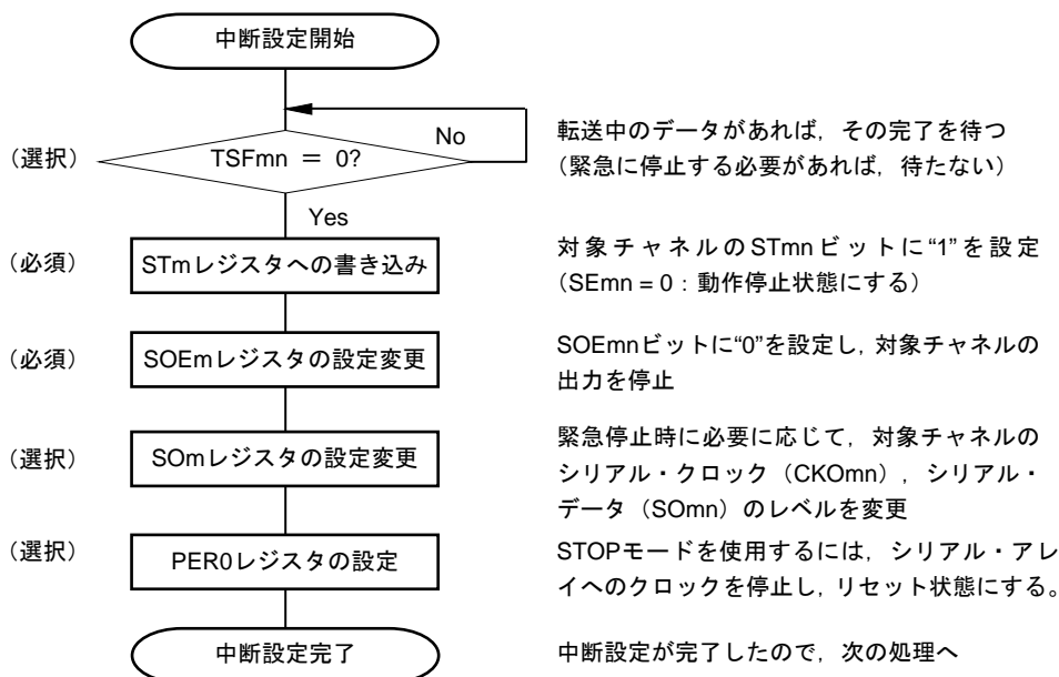
図14-27 マスタ送信の中断手順
