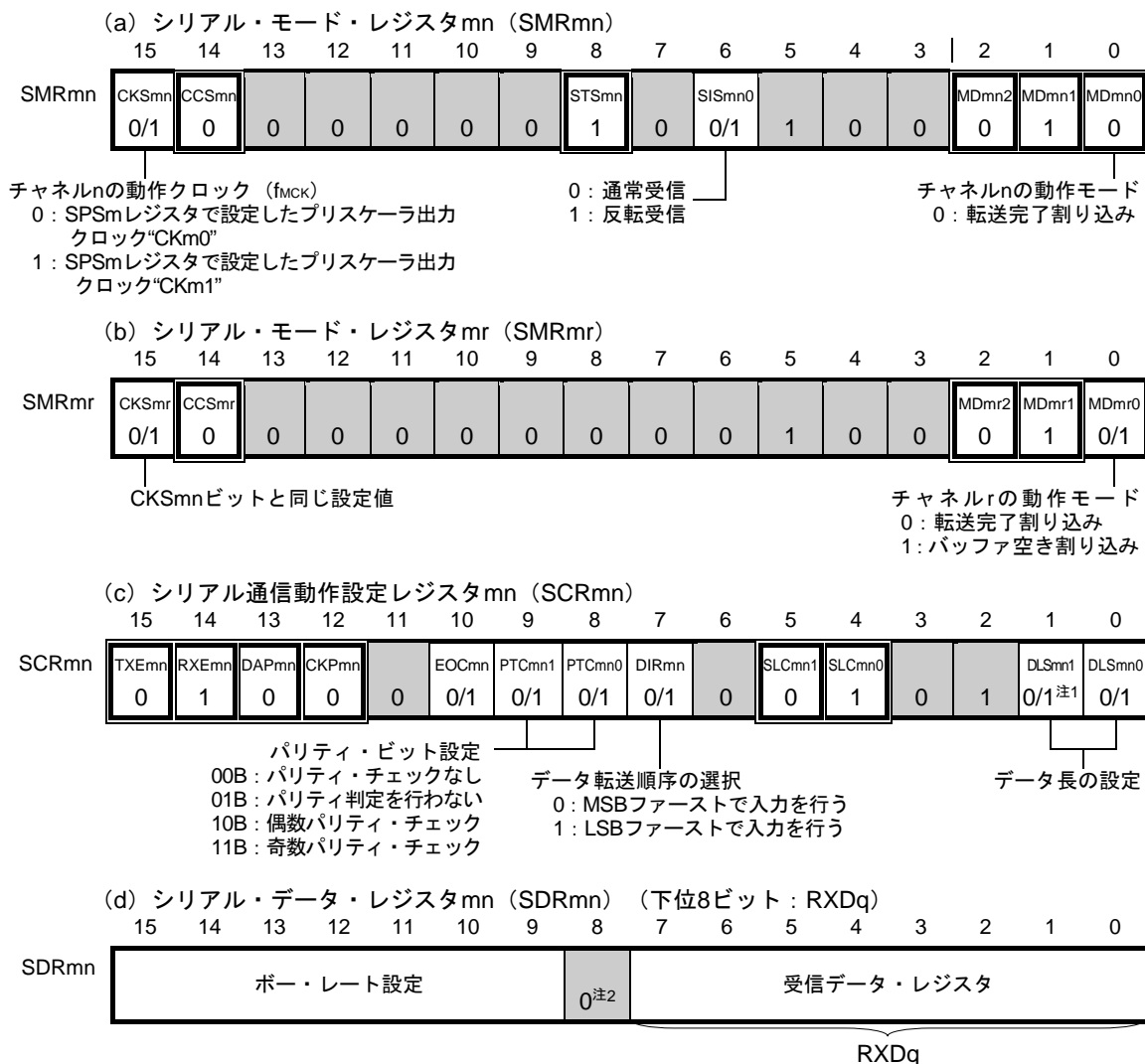
図14-84 UART (UART0-UART3) のUART受信時のレジスタ設定内容例 (80ピン製品) (1/2)
