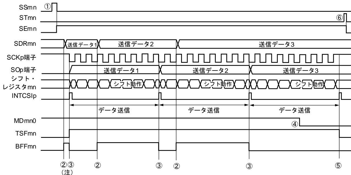
図14-31 マスタ送信（連続送信モード時）のタイミング・チャート（タイプ1：DAPmn = 0, CKPmn = 0）
