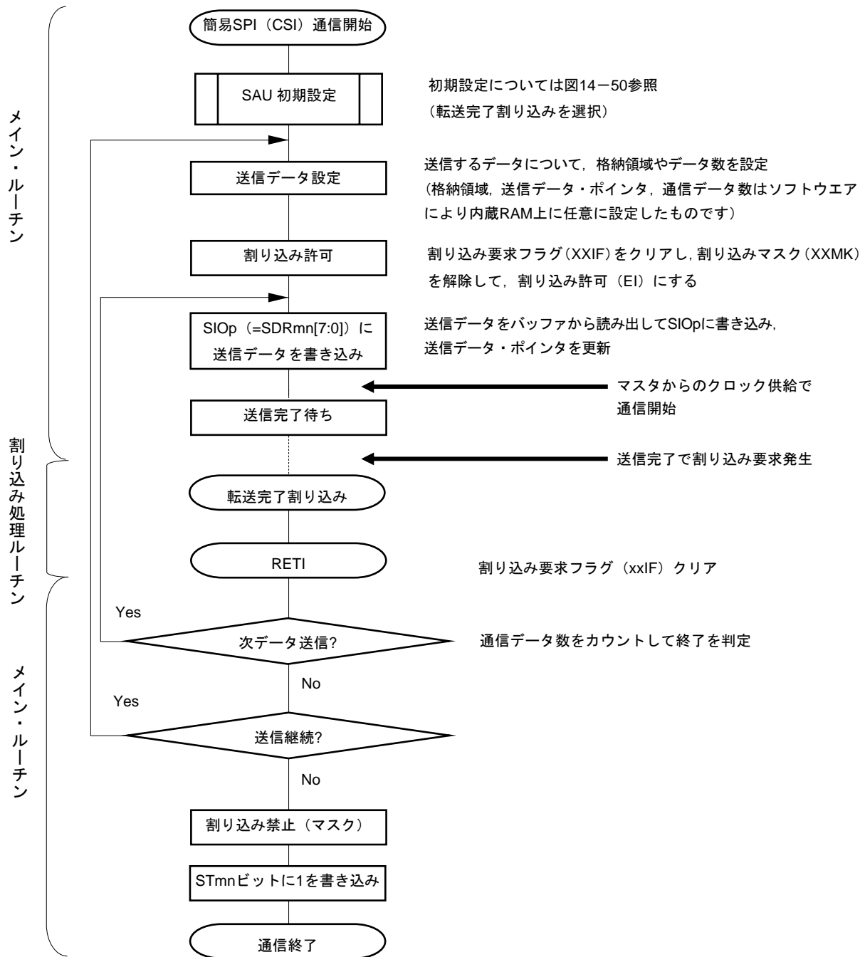
図14-54 スレーブ送信（シングル送信モード時）のフロー・チャート
