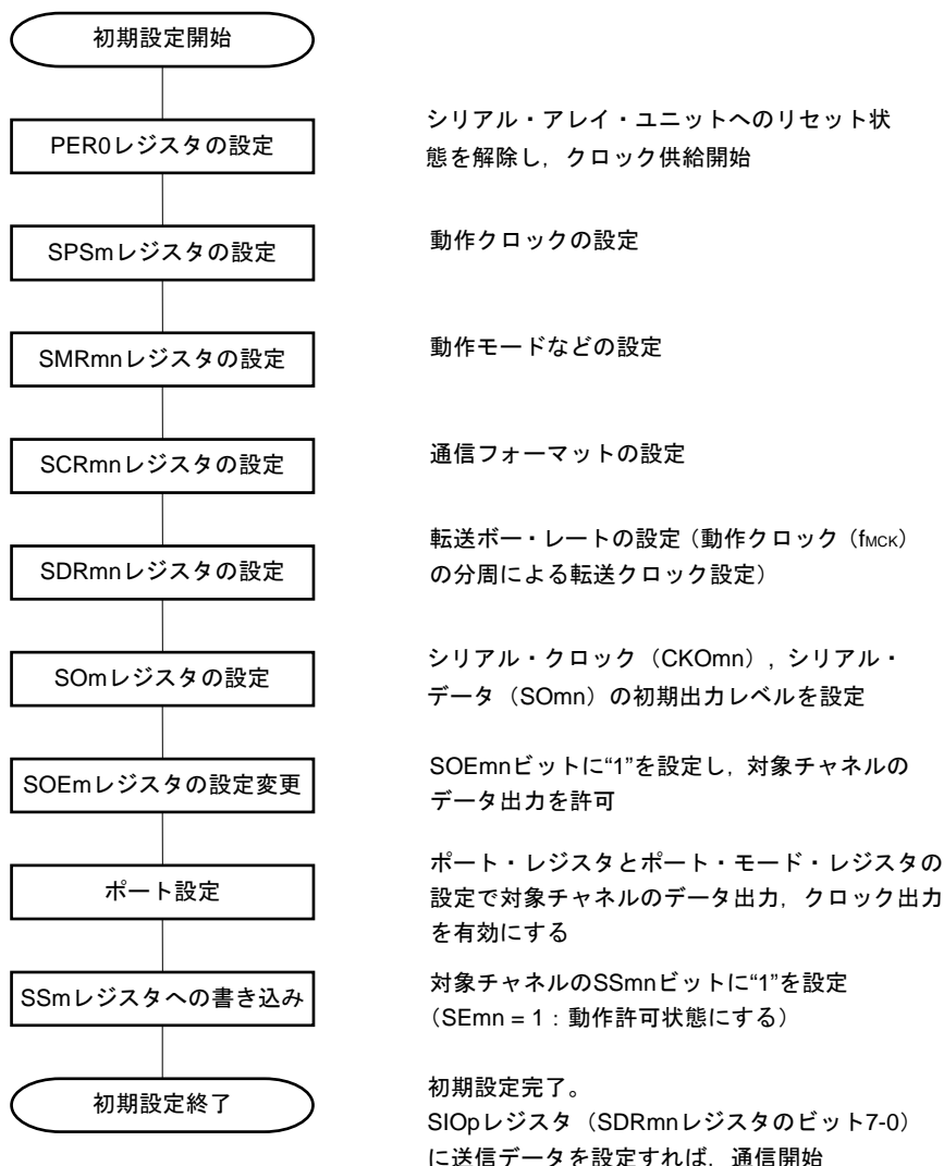
図14-42 マスタ送受信の初期設定手順
