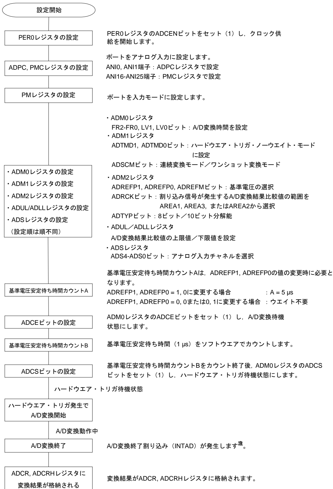
図12-24 ハードウェア・トリガ・ノーウエイト・モード設定
