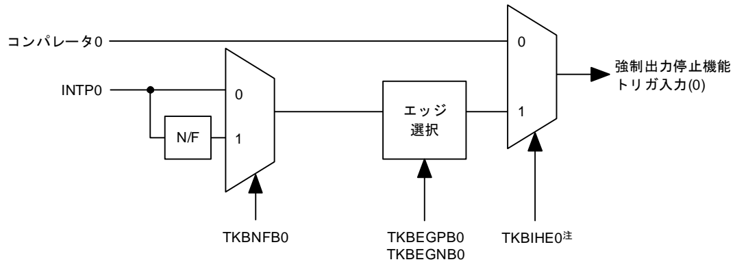
図7-67 IH制御用PWM出力機能使用時の強制出力停止機能トリガ入力選択 (0) の回路構成
