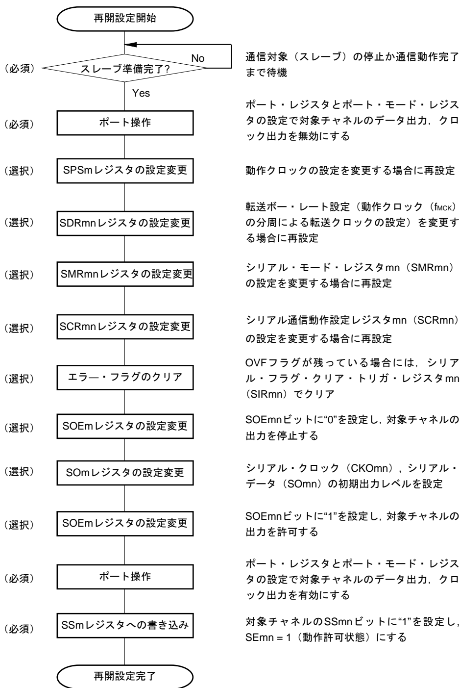
図14-44 マスタ送受信の再開設定手順
