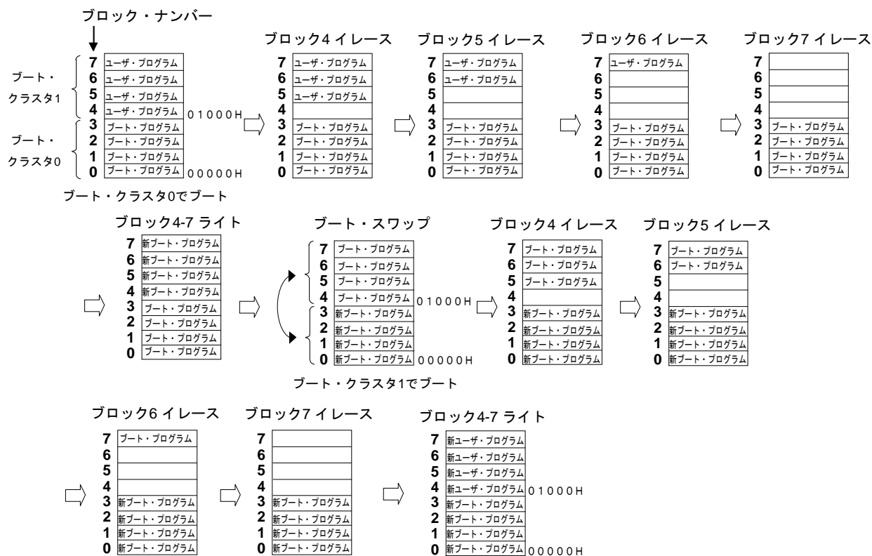
図28-10 ブート・スワップの実行例
