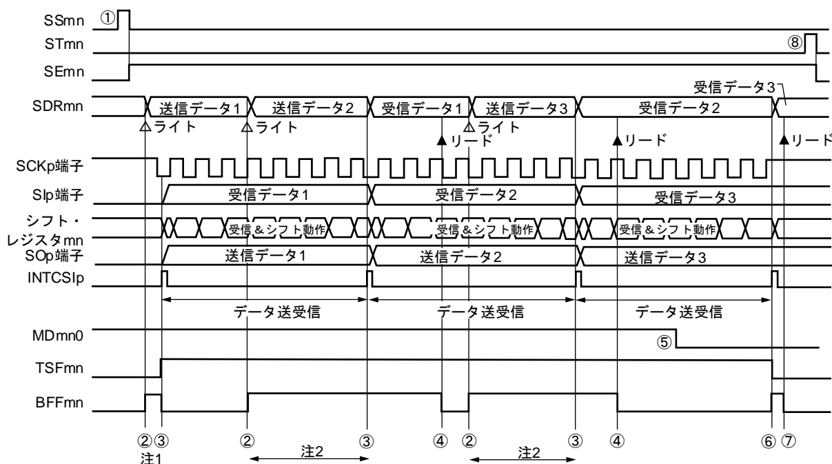
図14-69 スレーブ送受信（連続送受信モード時）のタイミング・チャート（タイプ1：DAPmn = 0, CKPmn = 0）
