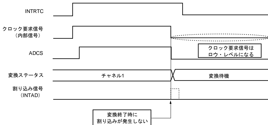
図12-30 A/D変換終了後に割り込みが発生しない場合の動作例
