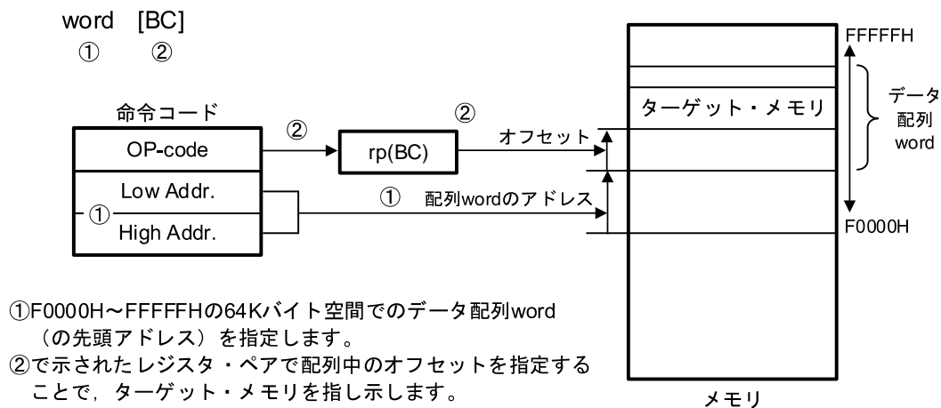
図3-31 word[BC]の例
