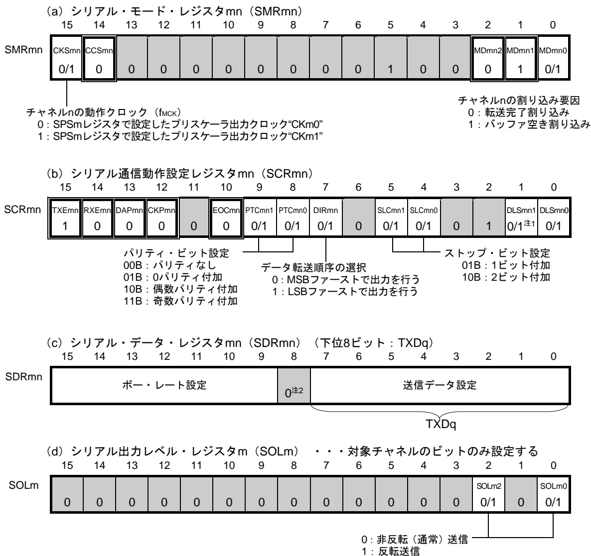
図14-76 UART (UART0-UART3) のUART送信時のレジスタ設定内容例 (80ピン製品) (1/2)
