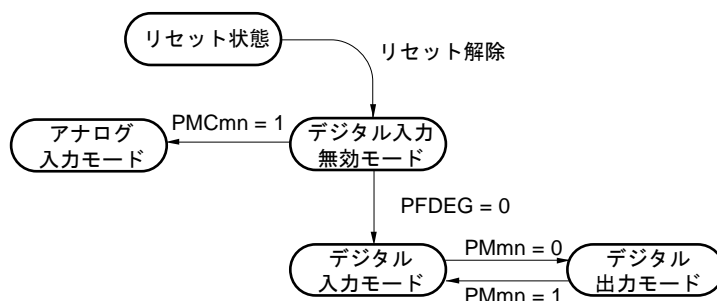
図4-16 IVREF0/ポート端子機能の状態遷移図
