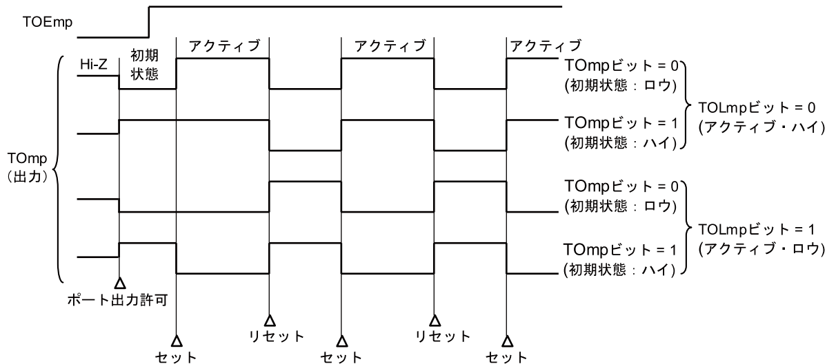
図6-35 PWM出力時 (TOMmp = 1) のTOmp端子出力状態
