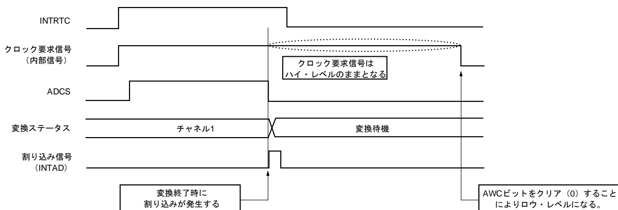
図12-29 A/D変換終了後に割り込みが発生する場合の動作例
