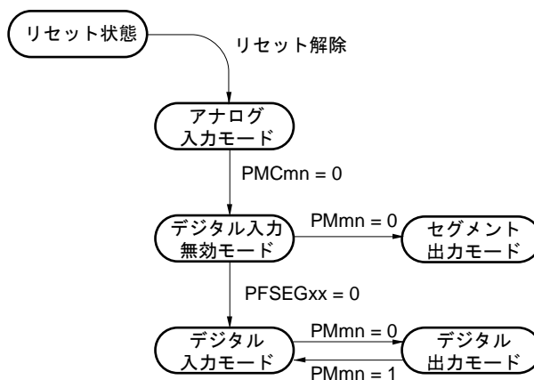
図4-13 ANIxx/SEGxx/ポート端子機能の状態遷移図
