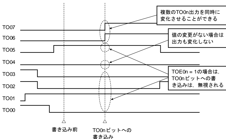
図6-39 TO0nビットの一括操作によるTO0nの端子状態
