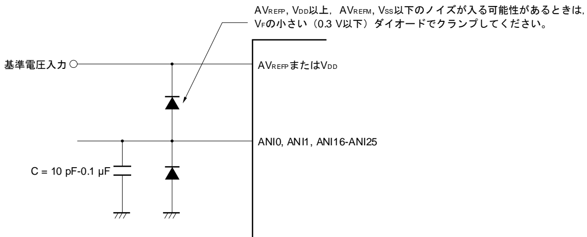
図12-38 アナログ入力端子の処理
