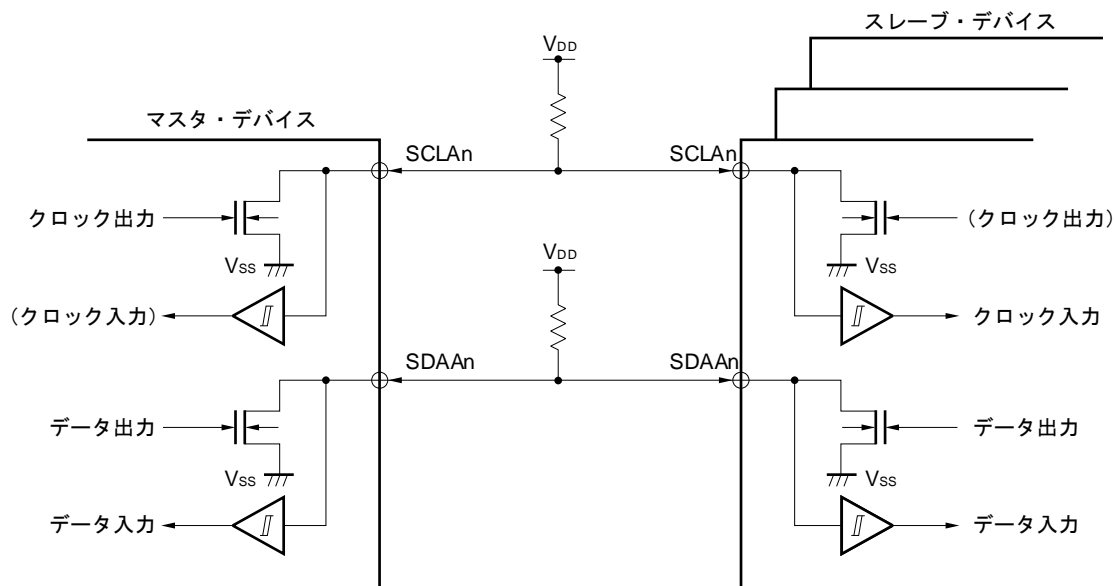
図15-13 端子構成図
