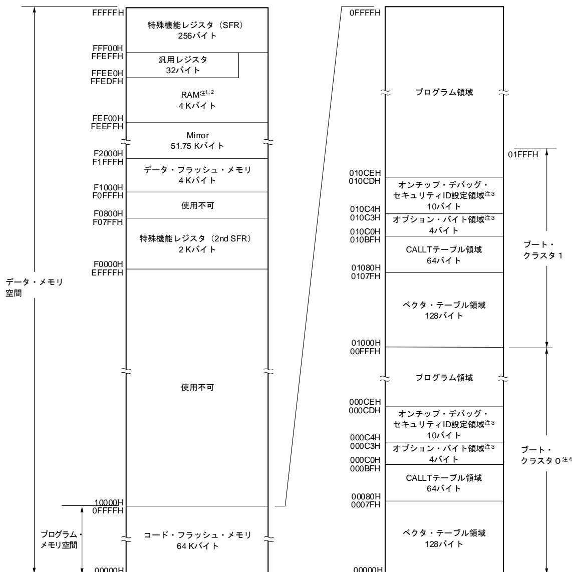
図3-4 メモリ・マップ (R5F10WLE, R5F10WME)
