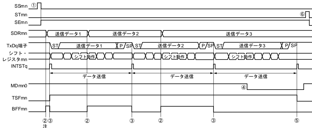
図14-82 UART送信（連続送信モード時）のタイミング・チャート
