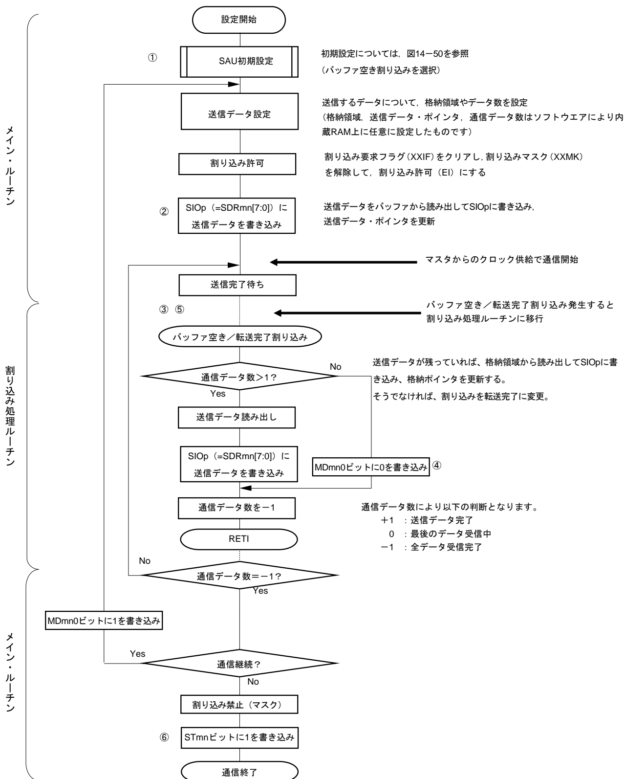
図14-56 スレーブ送信（連続送信モード時）のフロー・チャート
