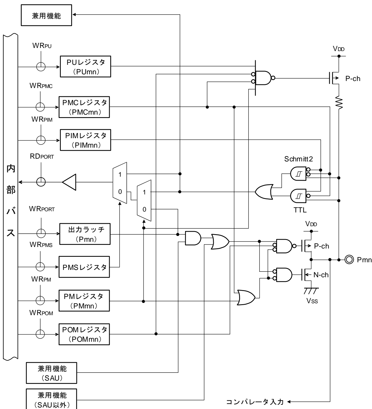
図2-16 端子タイプ 8-6-4 の端子ブロック図
