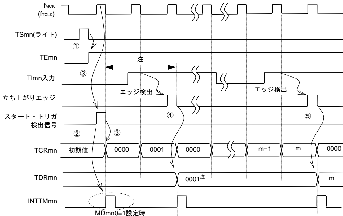
図6-29 動作タイミング（キャプチャ・モード：入力パルス間隔測定）
