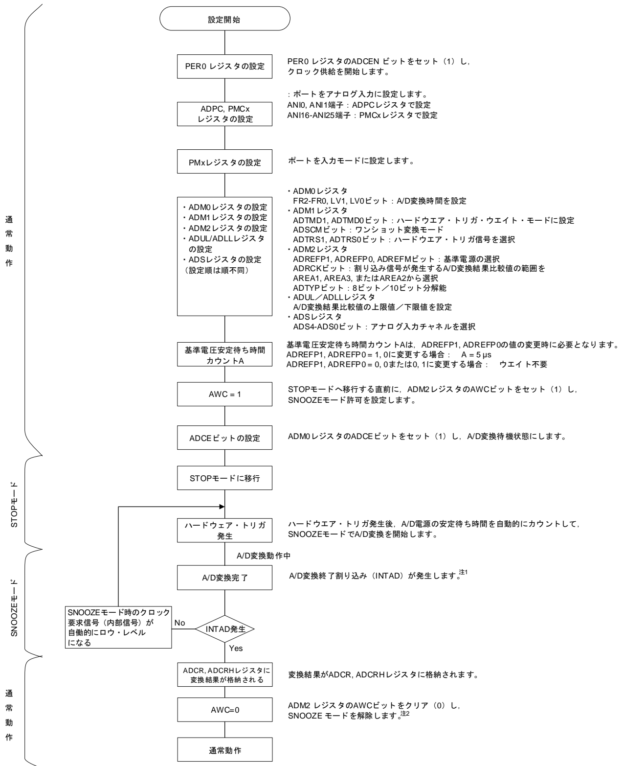
図12-31 SNOOZEモード設定のフローチャート
