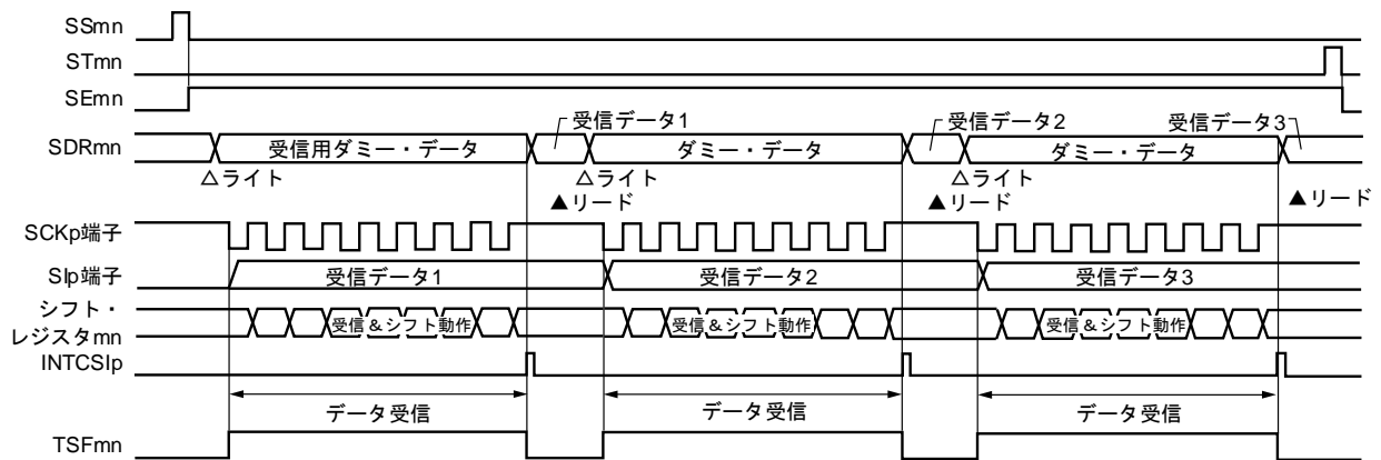
図14-37 マスタ受信（シングル受信モード時）のタイミング・チャート（タイプ1：DAPmn = 0, CKPmn = 0）
