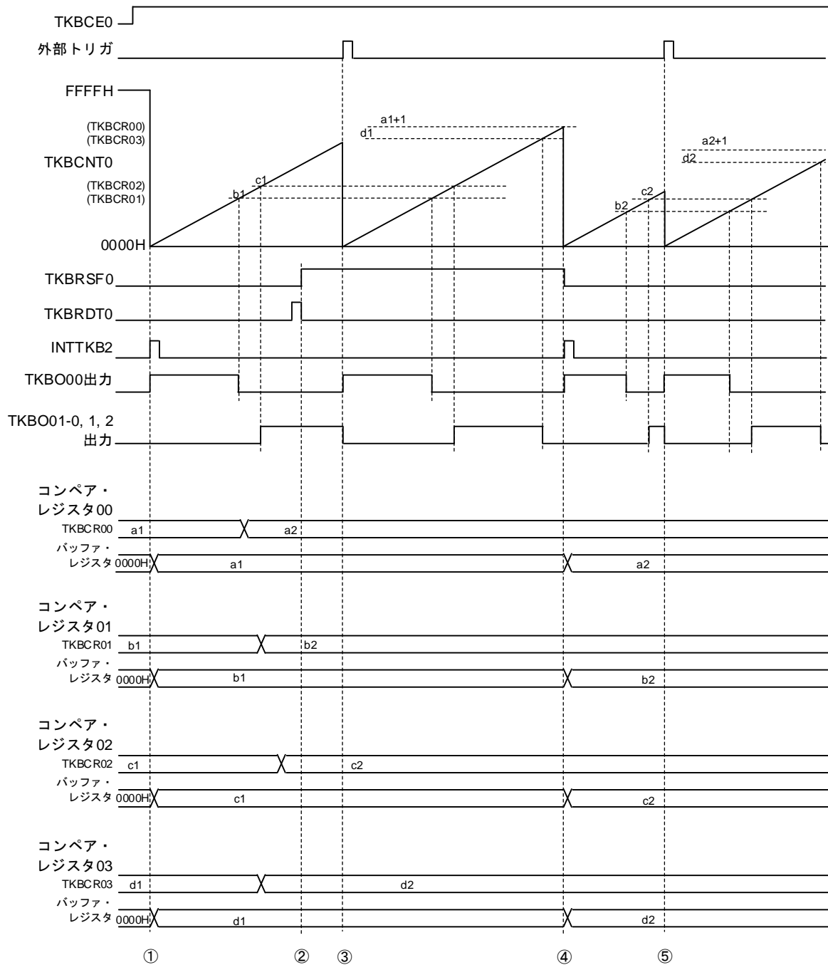
図7-46 一斉書き換え機能：外部トリガ入力による周期制御での単体動作時、カウント動作中のバッファ更新タイミング図（TKBTSE0ビットを0に設定）
