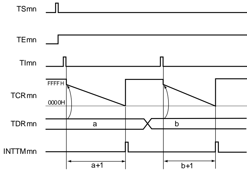
図6-60 デイレイ・カウンタとしての動作の基本タイミング例
