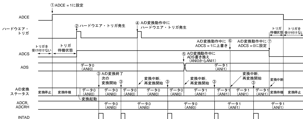
図12-21 ハードウェア・トリガ・ウエイト・モード（連続変換モード）動作タイミング例
