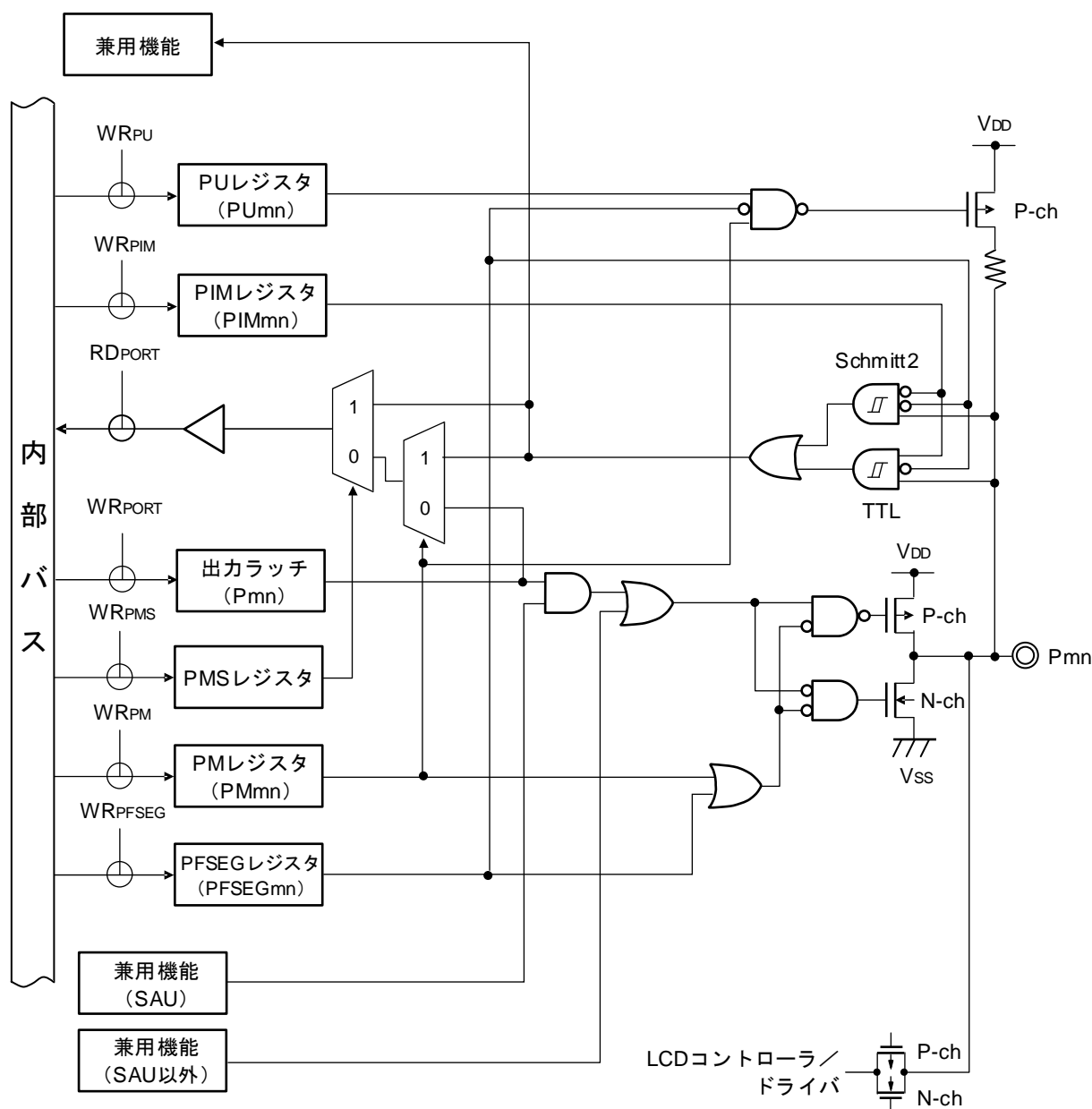
図2-14 端子タイプ 8-5-4 の端子ブロック図
