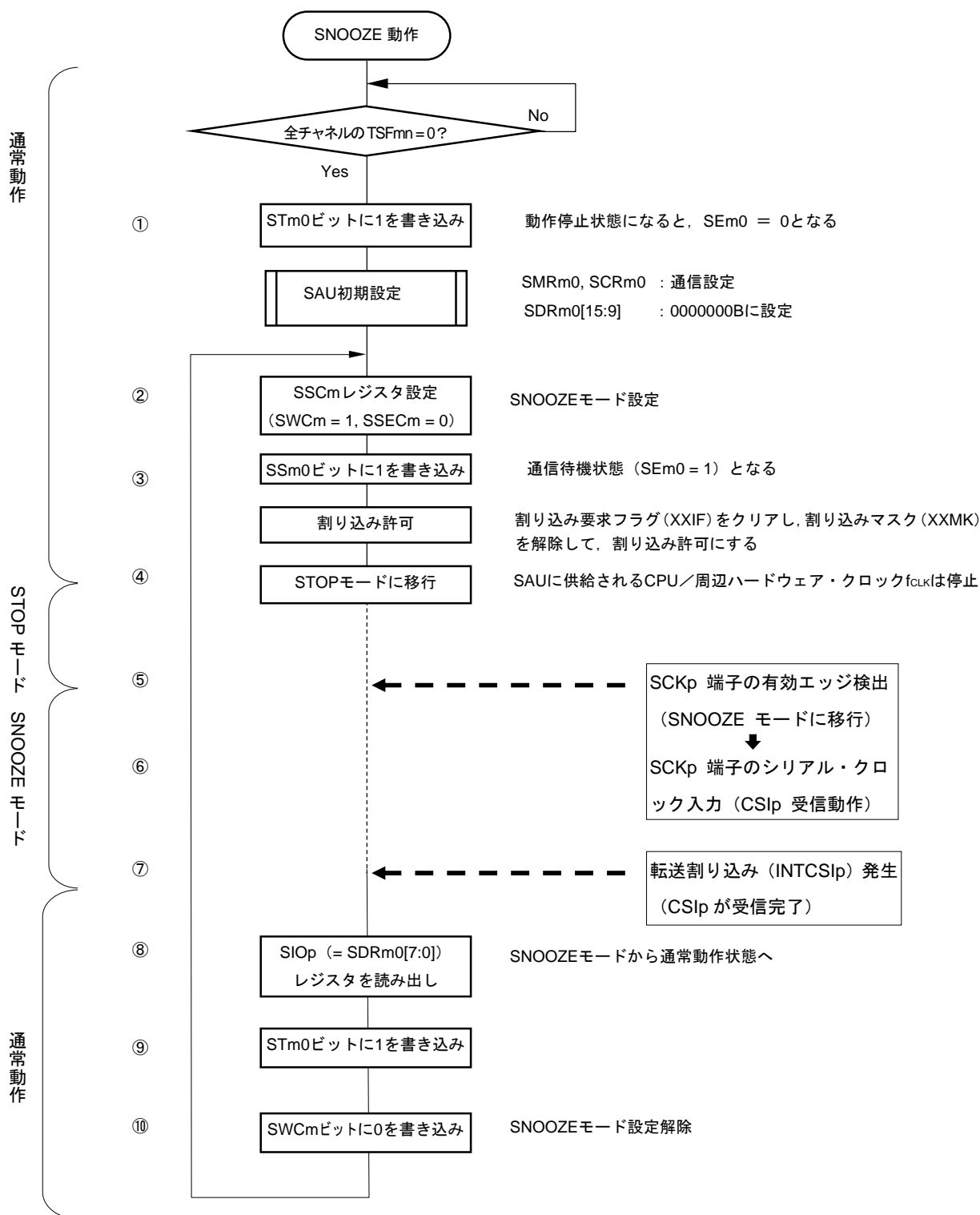
図14-74 SNOOZEモード動作（連続起動）時のフロー・チャート
