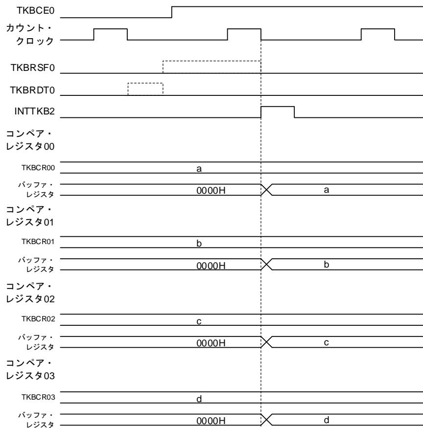
図7-42 一斉書き換え機能：カウント動作開始時のバッファ更新タイミング図
