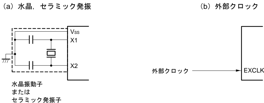
図5-12 X1発振回路の外付け回路例
