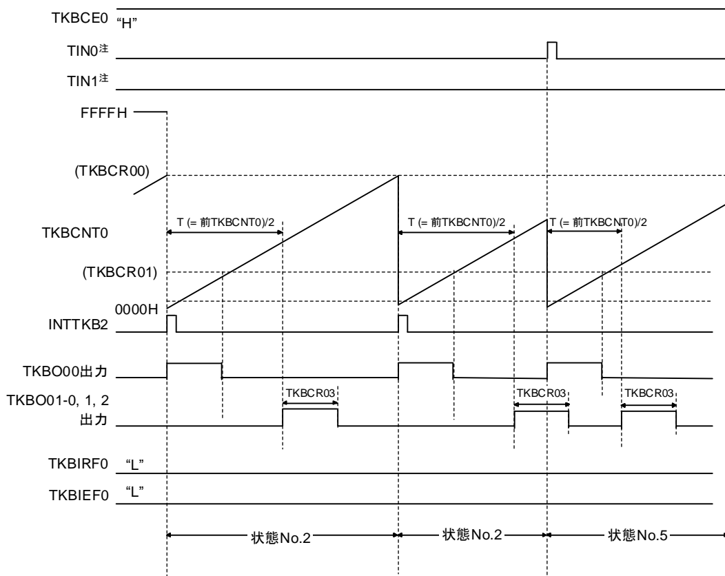
図7-50 インターリーブPFCモードのタイミング図（状態No.5の動作：INT0入力検出（1回目））
