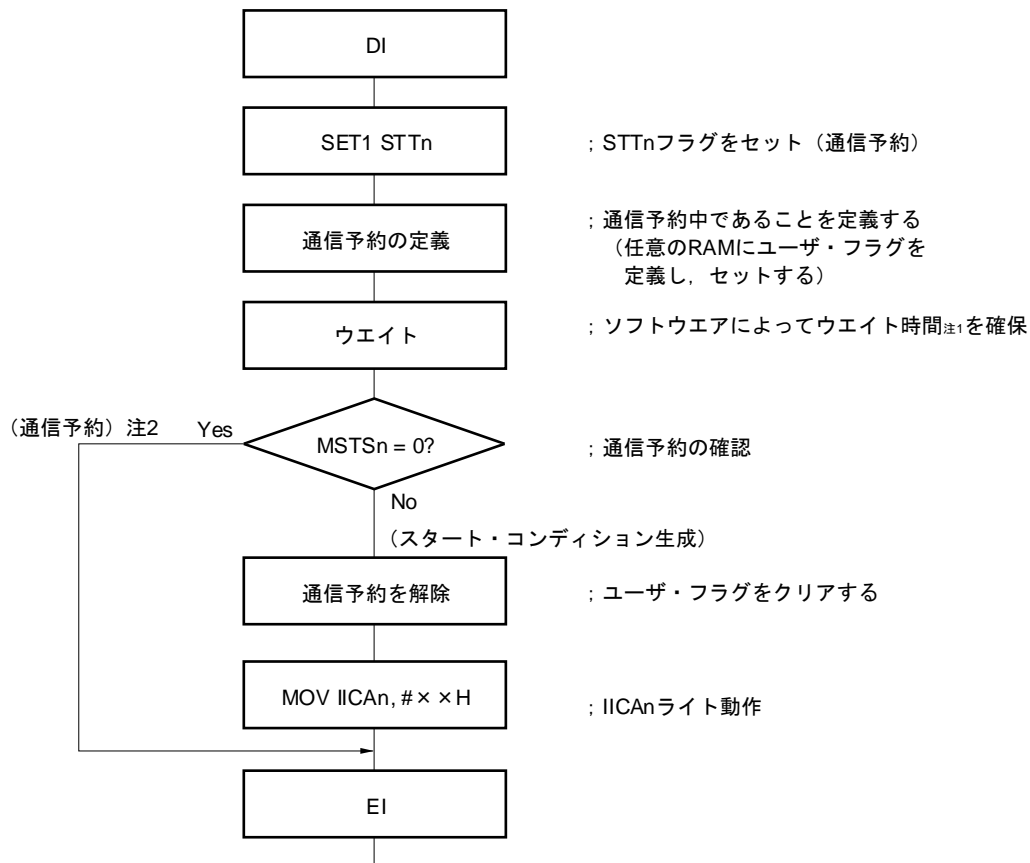
図15-27 通信予約の手順
