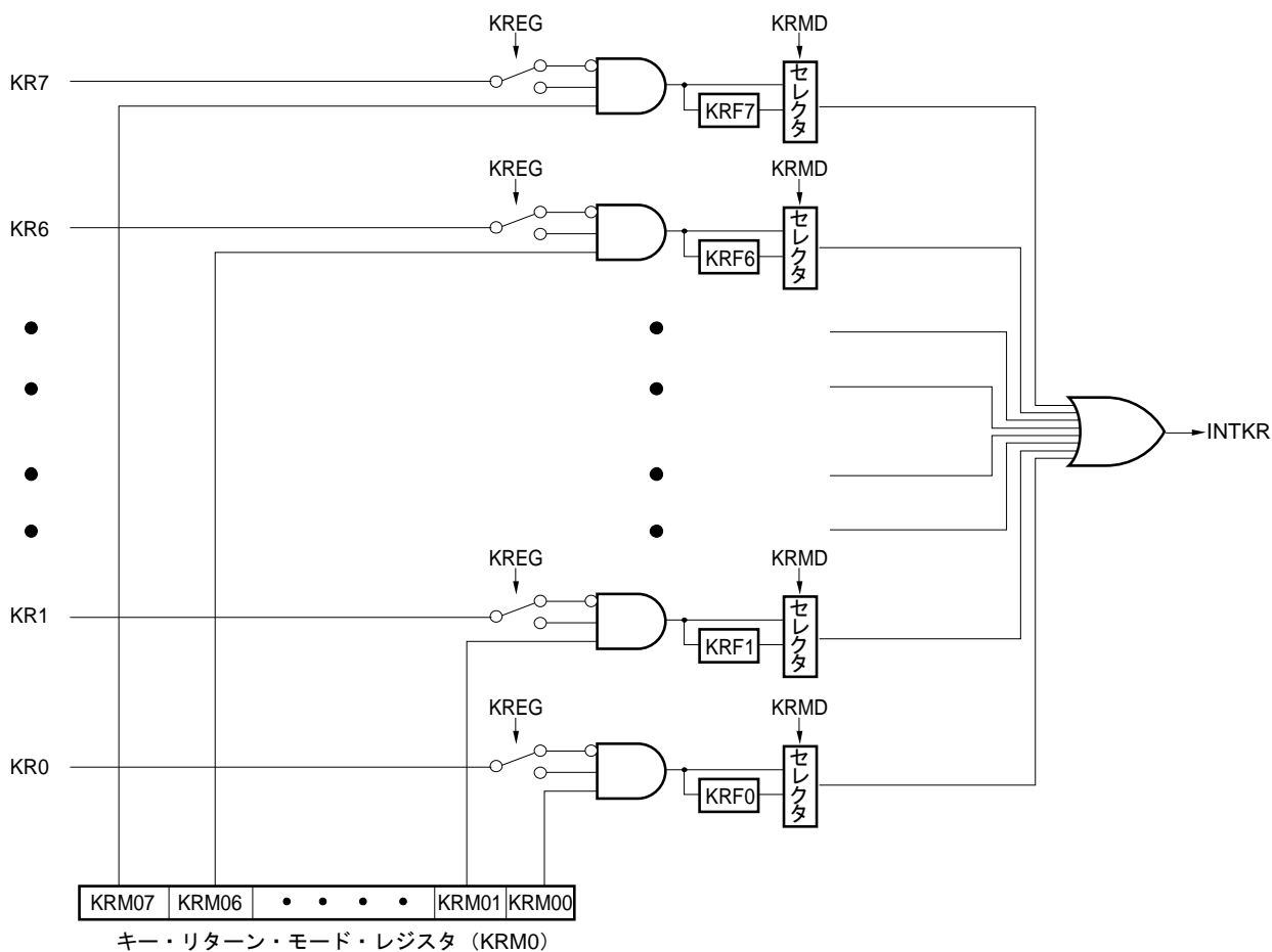
図20-1 キー割り込みのブロック図
