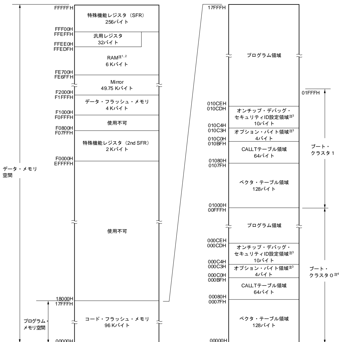
図3-5 メモリ・マップ (R5F10WLF, R5F10WMF)
