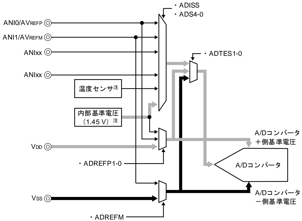
図25-15 A/Dテスト機能の構成
