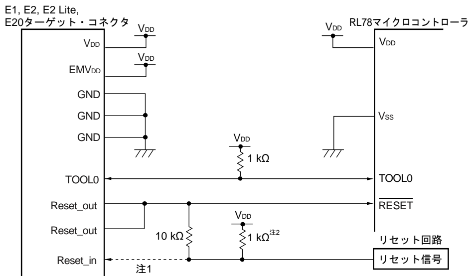
図29-1 E1, E2, E2 Lite, E20オンチップデバッグエミュレータとの接続例
