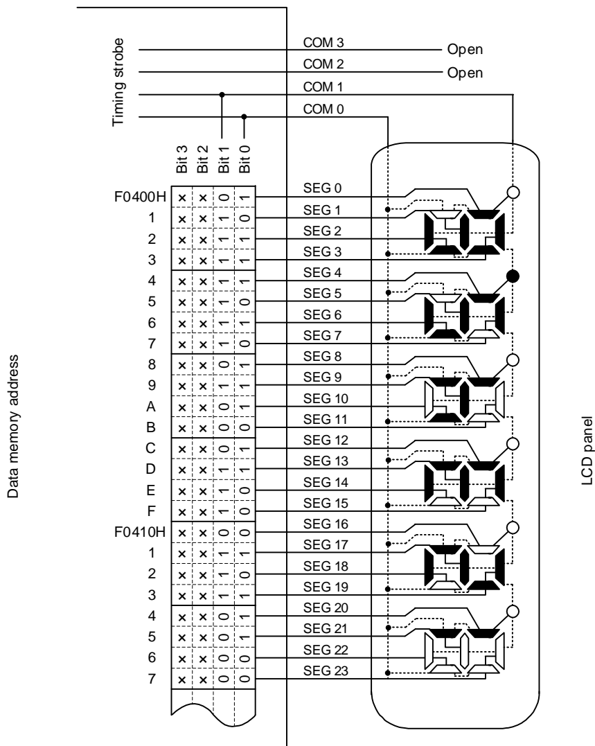
図16-30 2時分割LCDパネルの結線例
