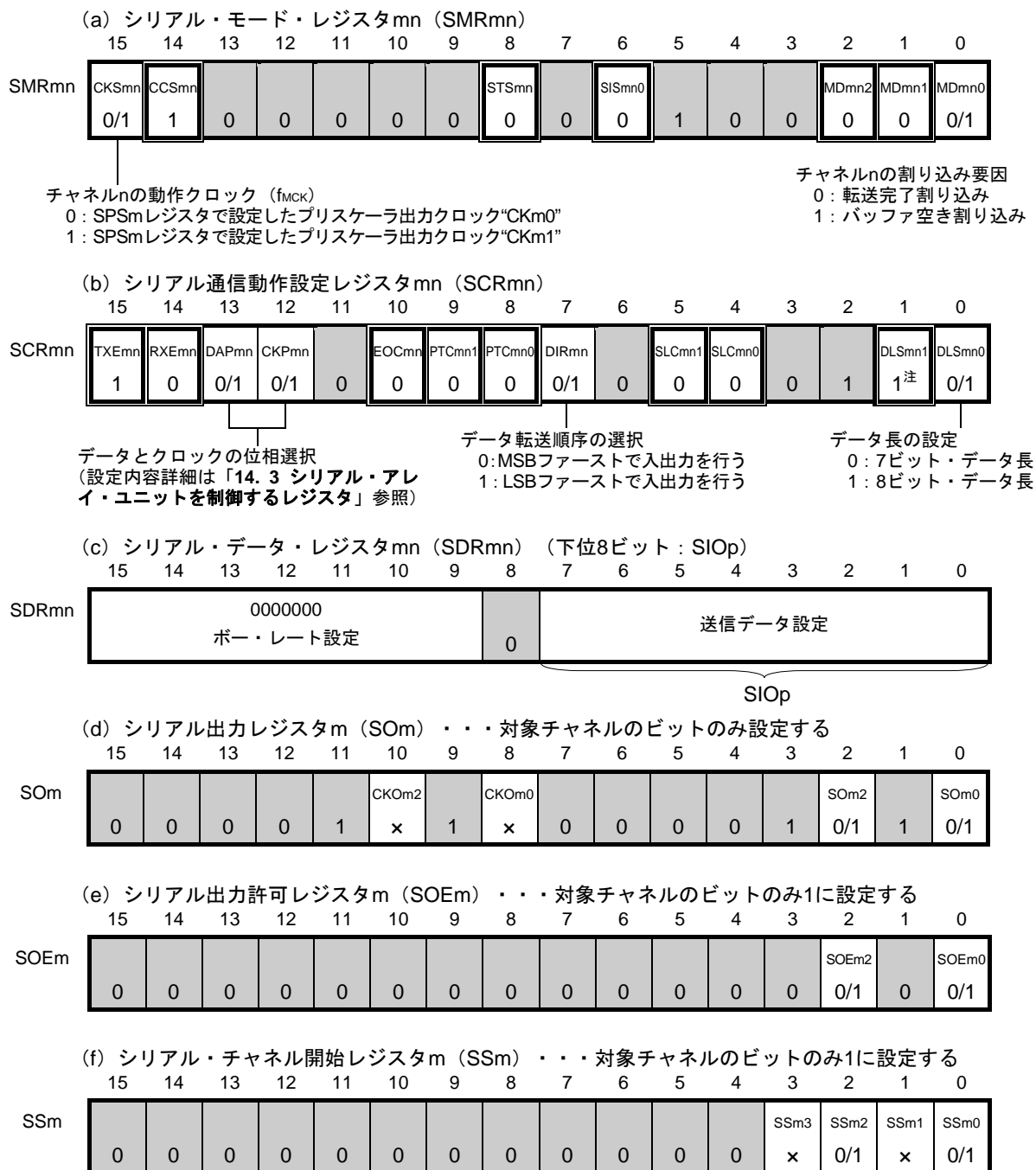
図14-49 簡易SPI (CSI00, CSI10) のスレーブ送信時のレジスタ設定内容例
