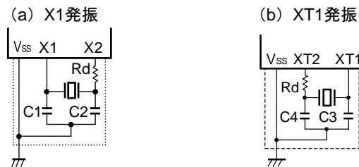
図5-17 外付け発振回路例
