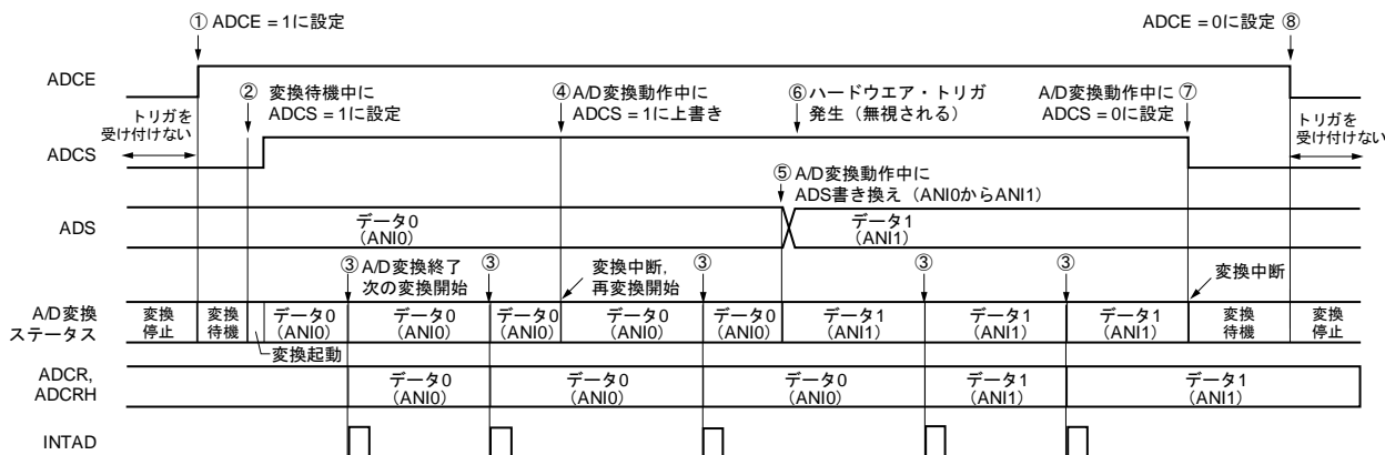
図12-17 ソフトウェア・トリガ・モード（連続変換モード）動作タイミング例
