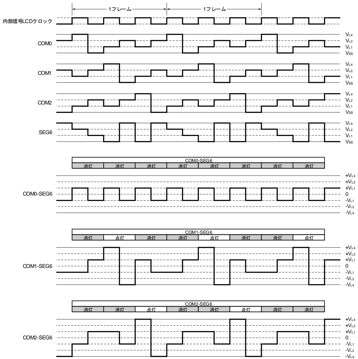
図16-35 SEG6と各コモン信号間の3時分割LCD駆動波形例（1/3バイアス法）
