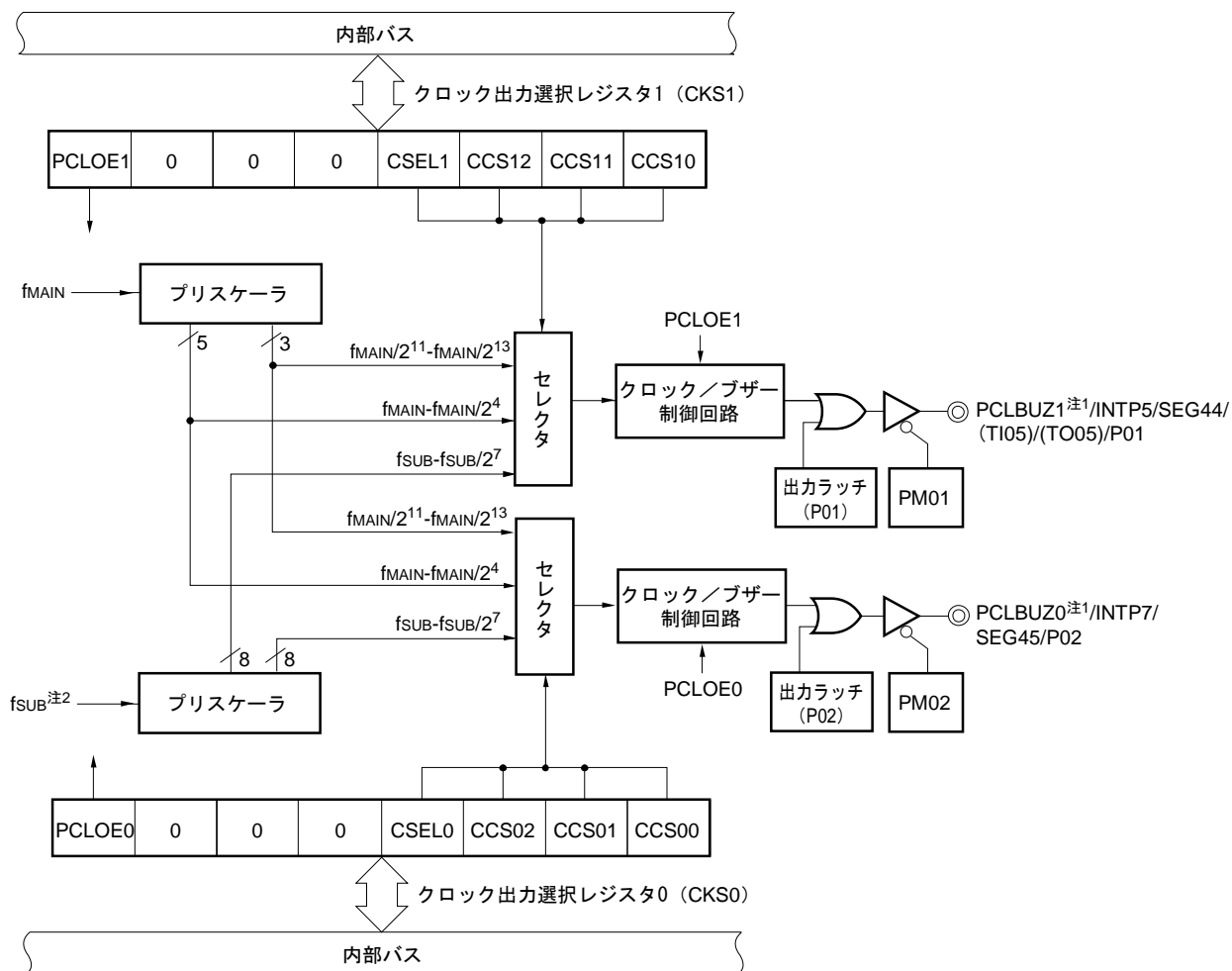
図10-1 クロック出力／ブザー出力制御回路のブロック図
