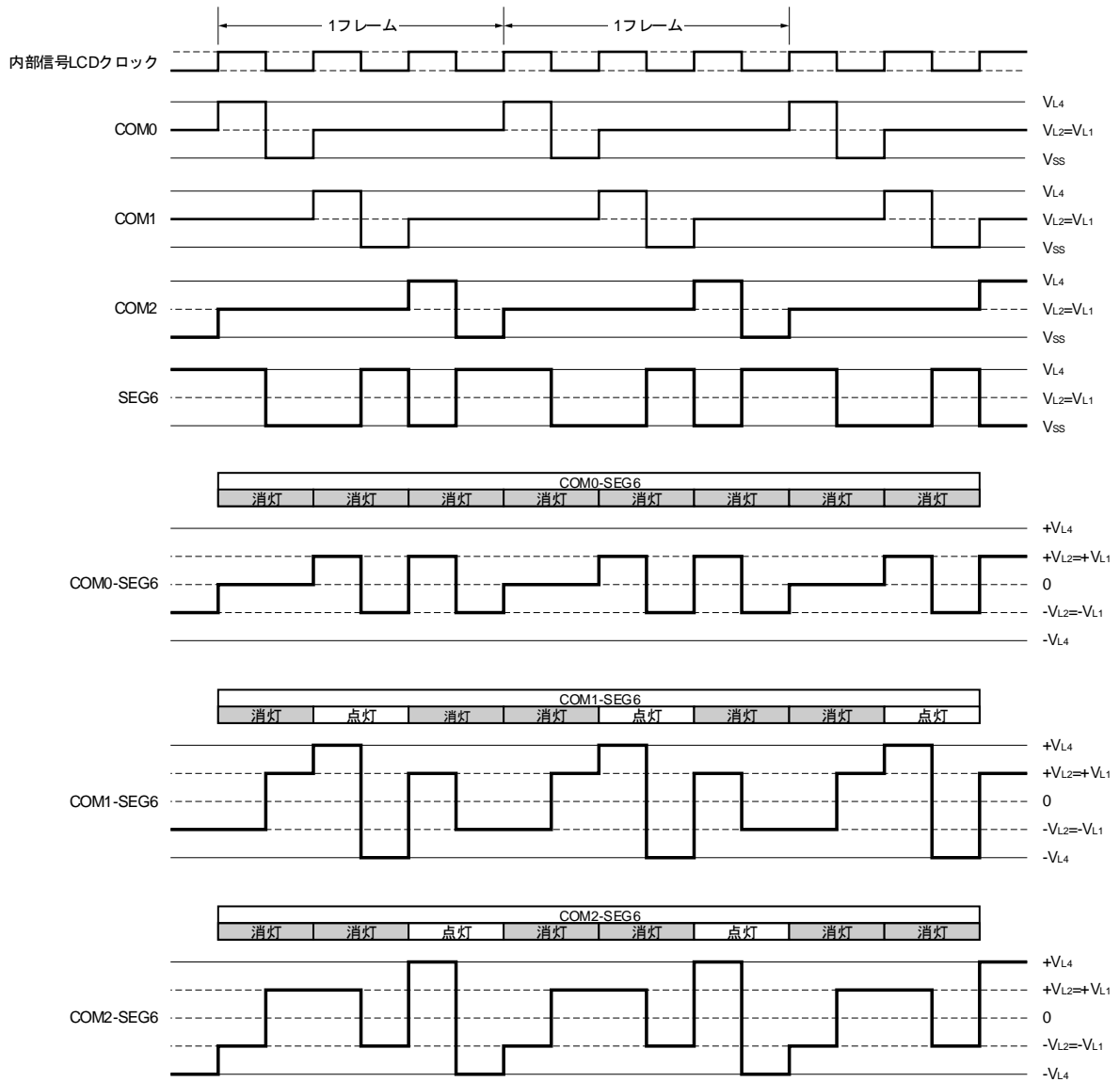
図16-34 SEG6と各コモン信号間の3時分割LCD駆動波形例（1/2バイアス法）
