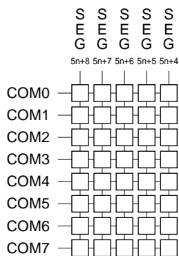
図16-39 8時分割LCD表示パターンと電極結線
