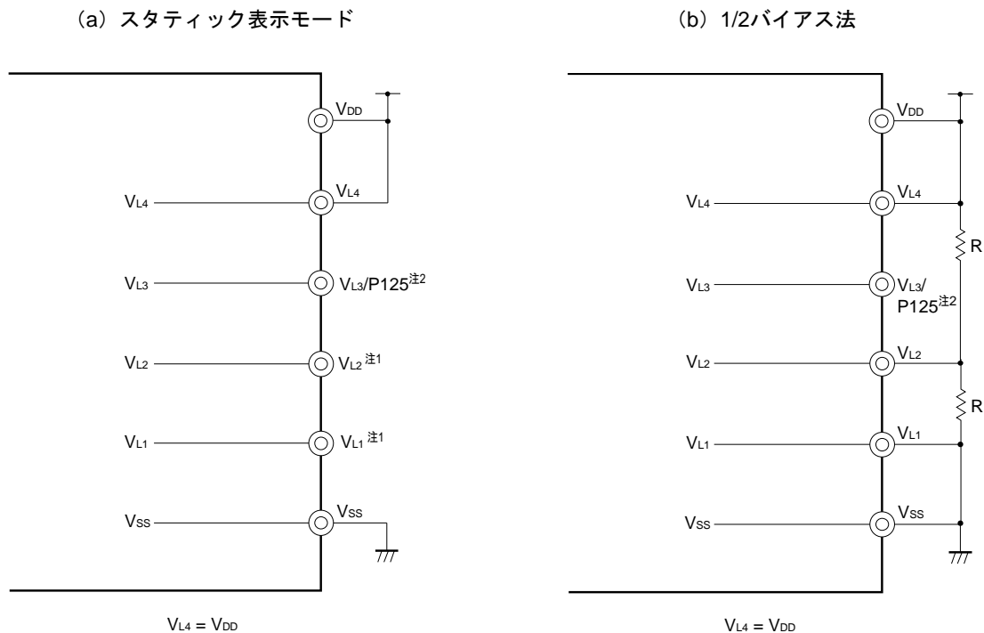
図16-21 LCD駆動用電源の接続例（外部抵抗分割方式）（1/2）
