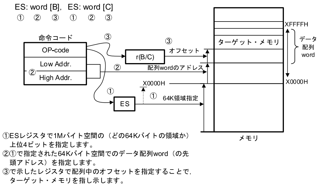
図3-33 ES:word[B], ES:word[C]の例
