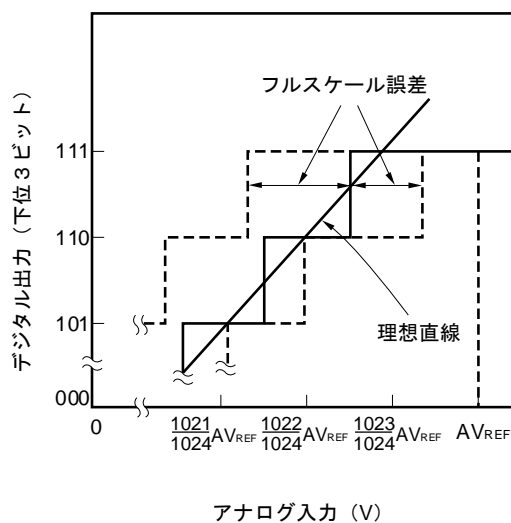
図12-35 フルスケール誤差
