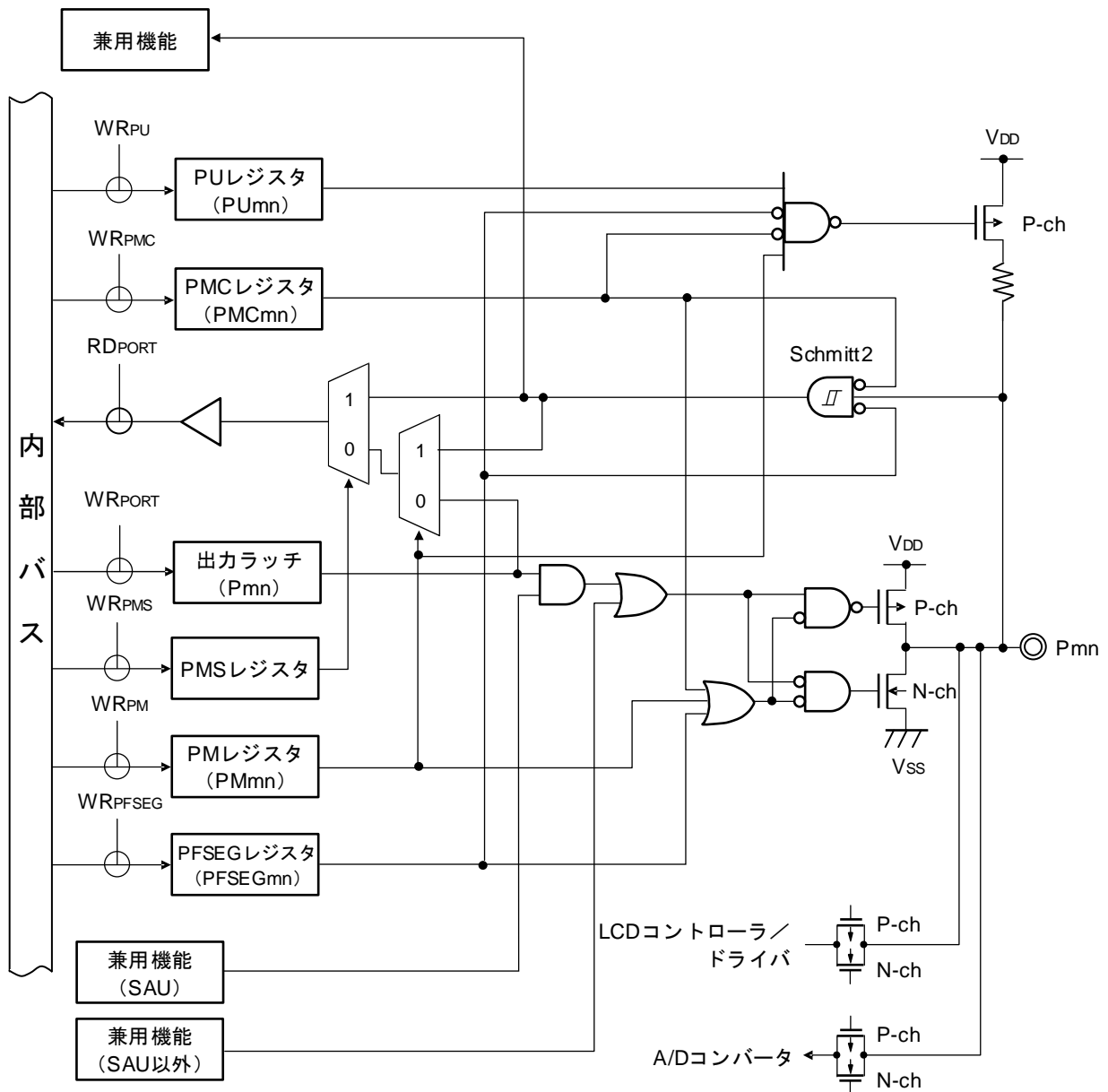
図2-13 端子タイプ 7-10-3 の端子ブロック図
