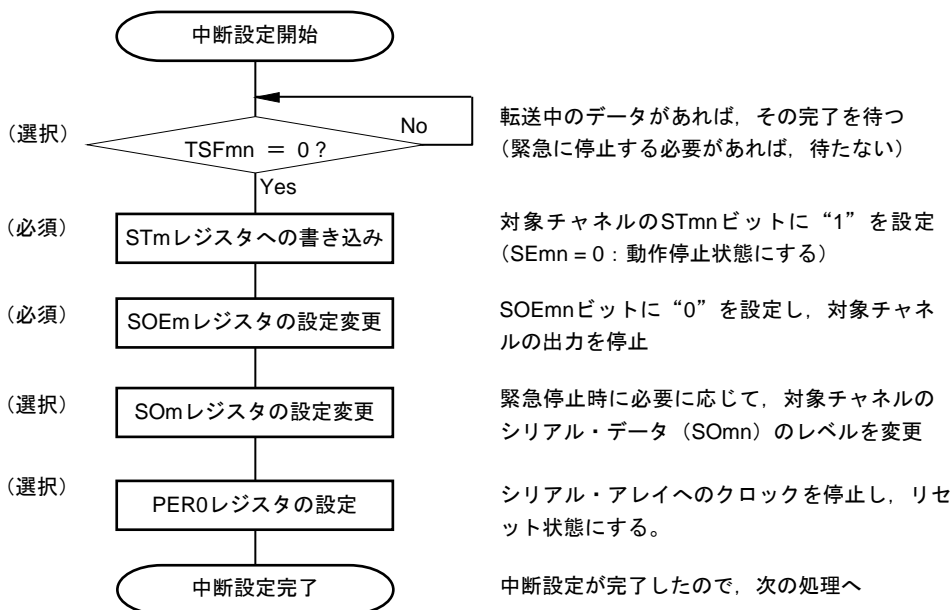
図14-51 スレーブ送信の中断手順
