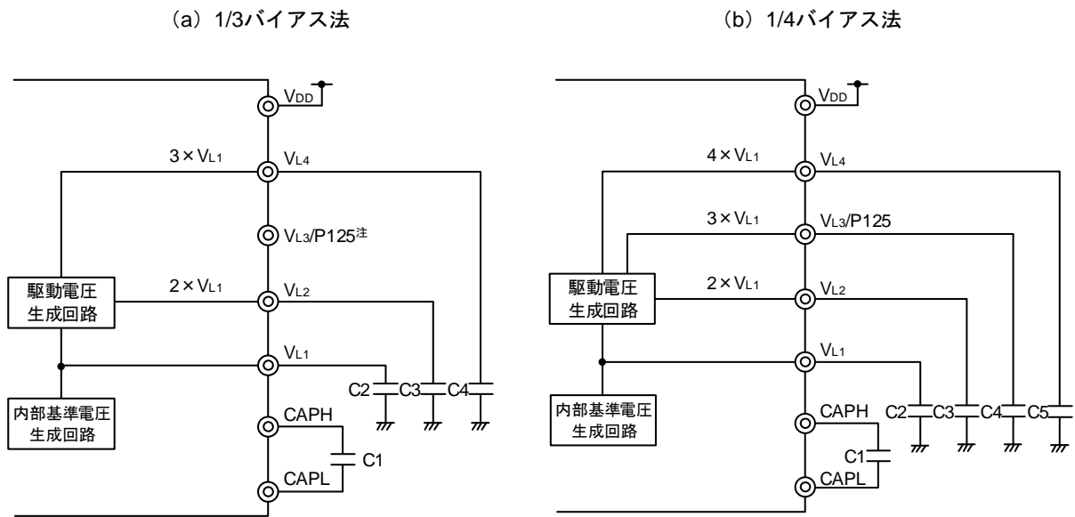
図16-22 LCD駆動用電源の接続例（内部昇圧方式）
