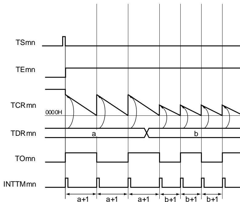
図6-44 インターバル・タイマ／方形波出力としての動作の基本タイミング例 (MDmn0 = 1)
