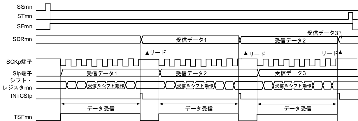
図14-61 スレーブ受信（シングル受信モード時）のタイミング・チャート（タイプ1：DAPmn = 0, CKPmn = 0）
