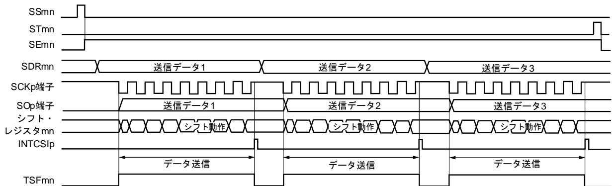
図14-53 スレーブ送信（シングル送信モード時）のタイミング・チャート（タイプ1：DAPmn = 0, CKPmn = 0）
