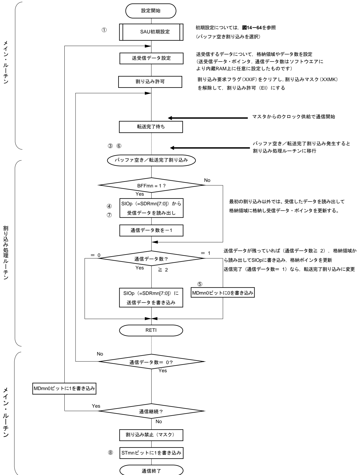
図14-70 スレーブ送受信（連続送受信モード時）のフロー・チャート
