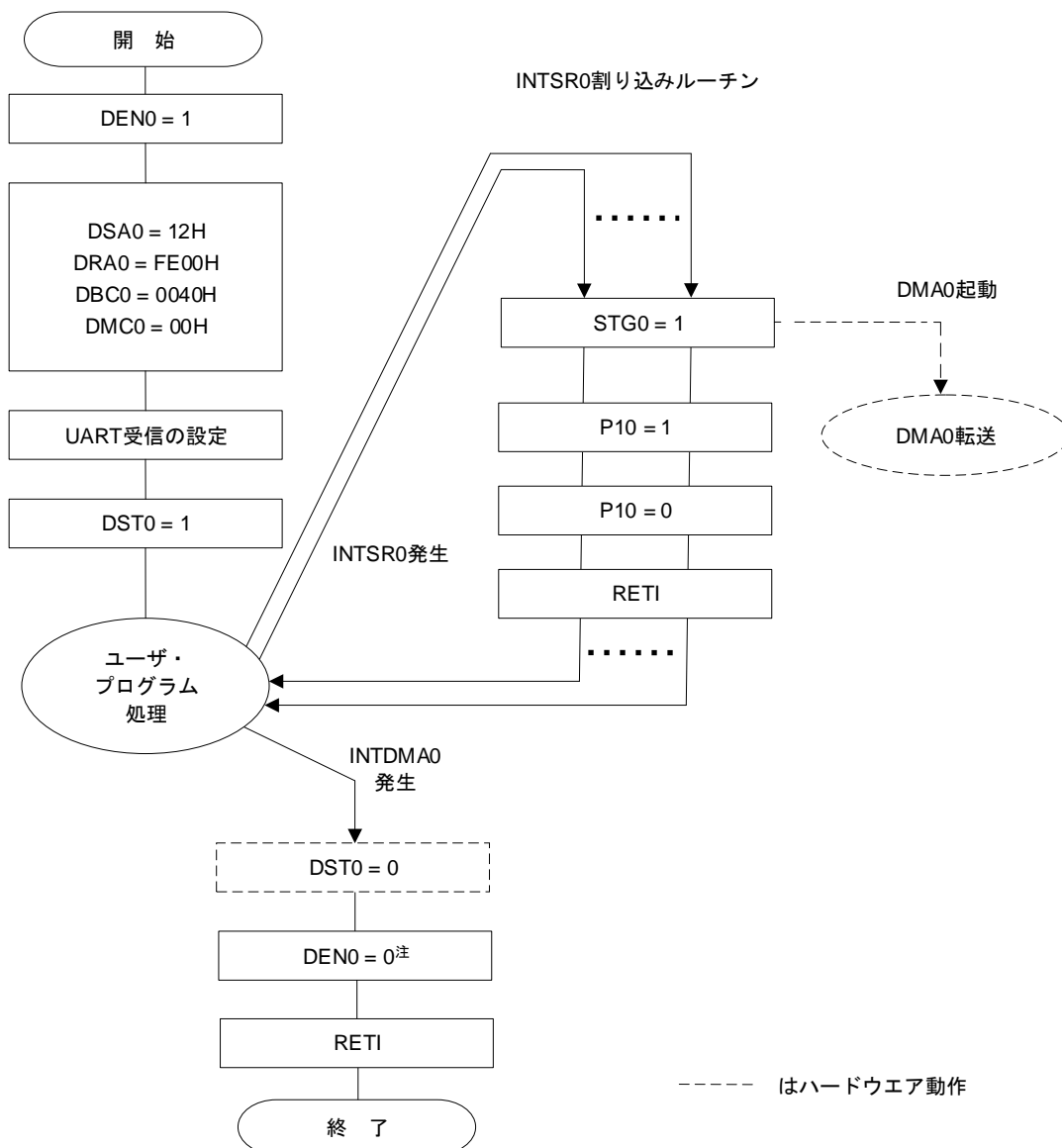
図18-9 UART連続受信+ACK送信の設定例
