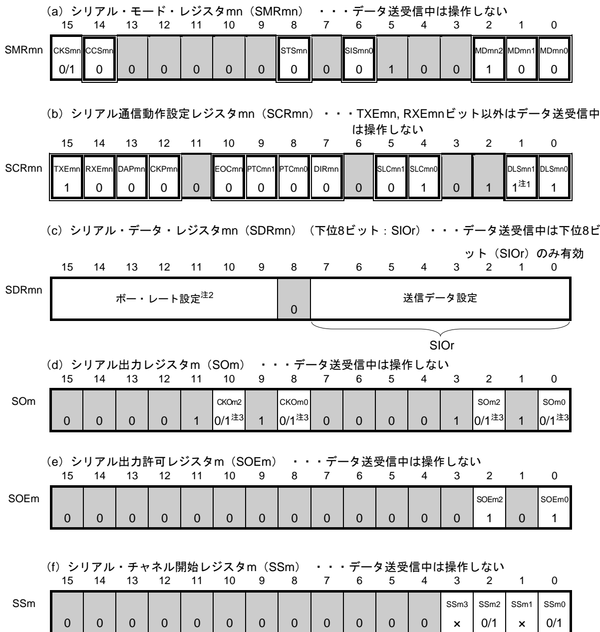
図14-107 簡易I 2 C (IIC00, IIC10) のデータ送信時のレジスタ設定内容例
