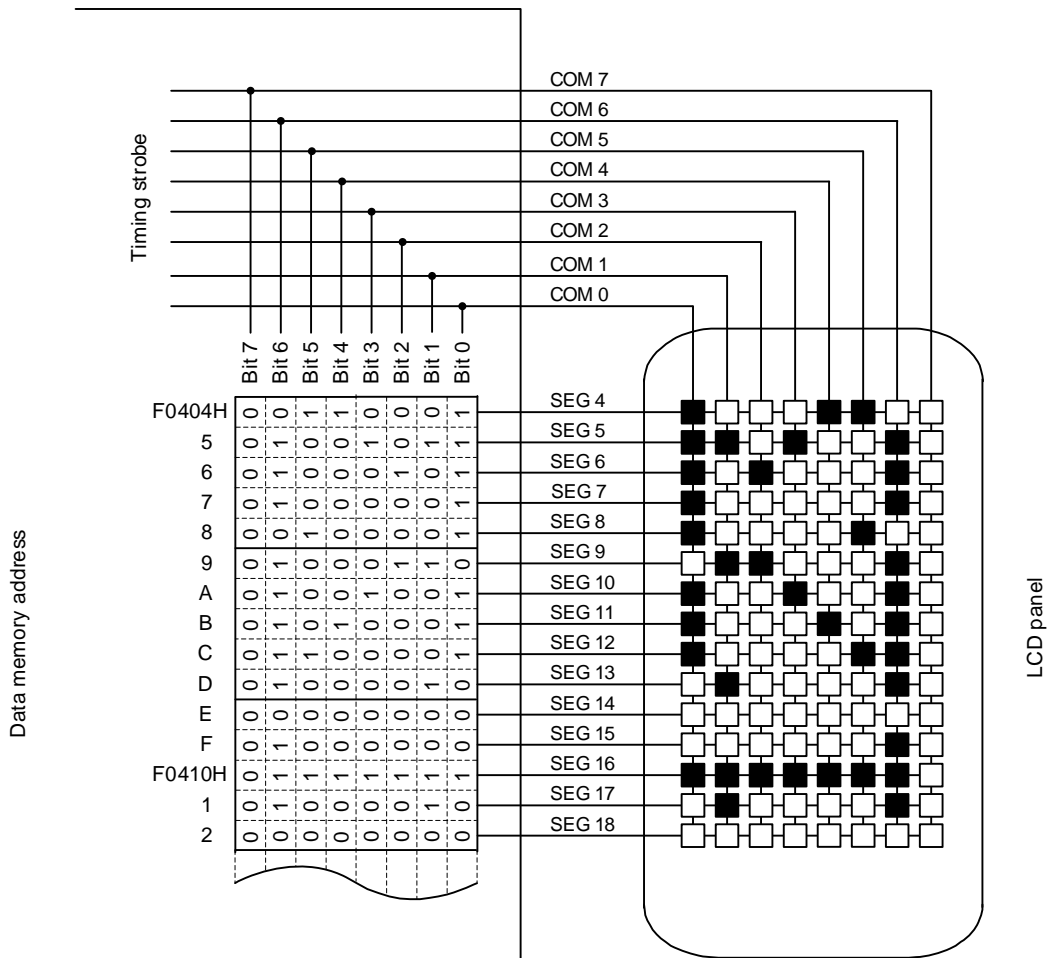
図16-40 8時分割LCDパネルの結線例
