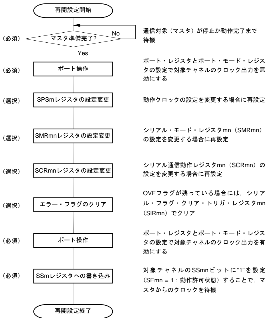
図14-60 スレーブ受信の再開設定手順
