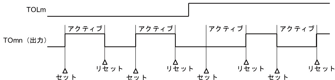
図6-36 タイマ動作中にTOLmレジスタの内容を変更した場合の動作
