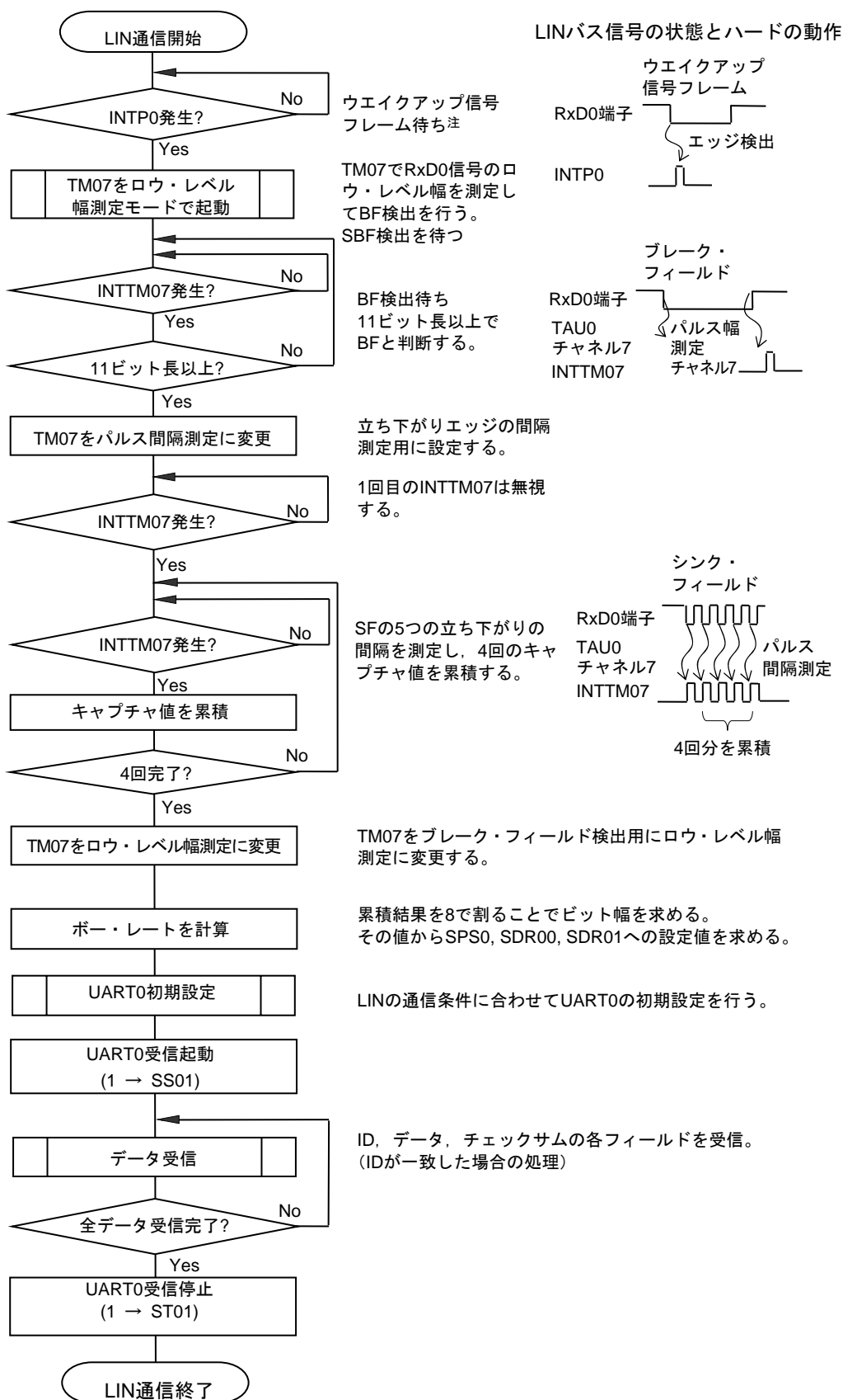
図14-101 LIN受信のフロー・チャート
