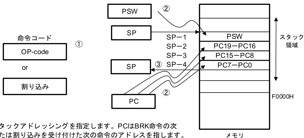
図3-41 割り込み, BRKの例
