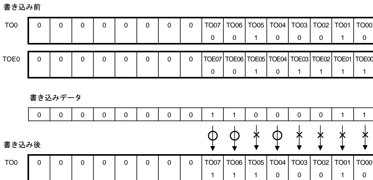
図6-38 TO0nビットの一括操作例
