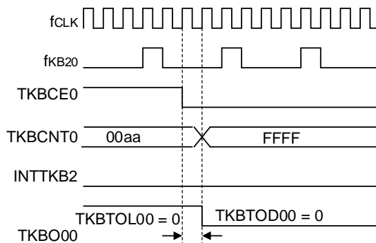
図7-36 動作停止のタイミング図 (TKBCE0を“1”から“0”に変更した場合)
