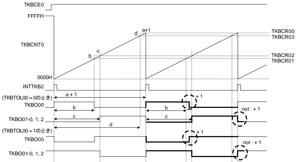
図7-60 ディザリング動作の波形図 (TKBCR03 = TKBCR00+1の場合)
