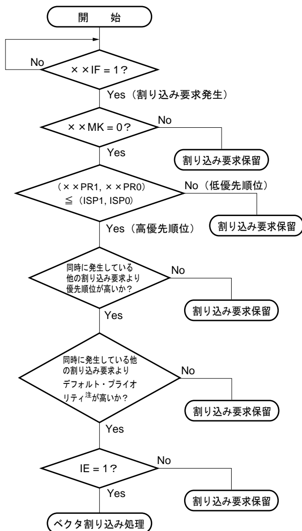
図19-7 割り込み要求受け付け処理アルゴリズム
