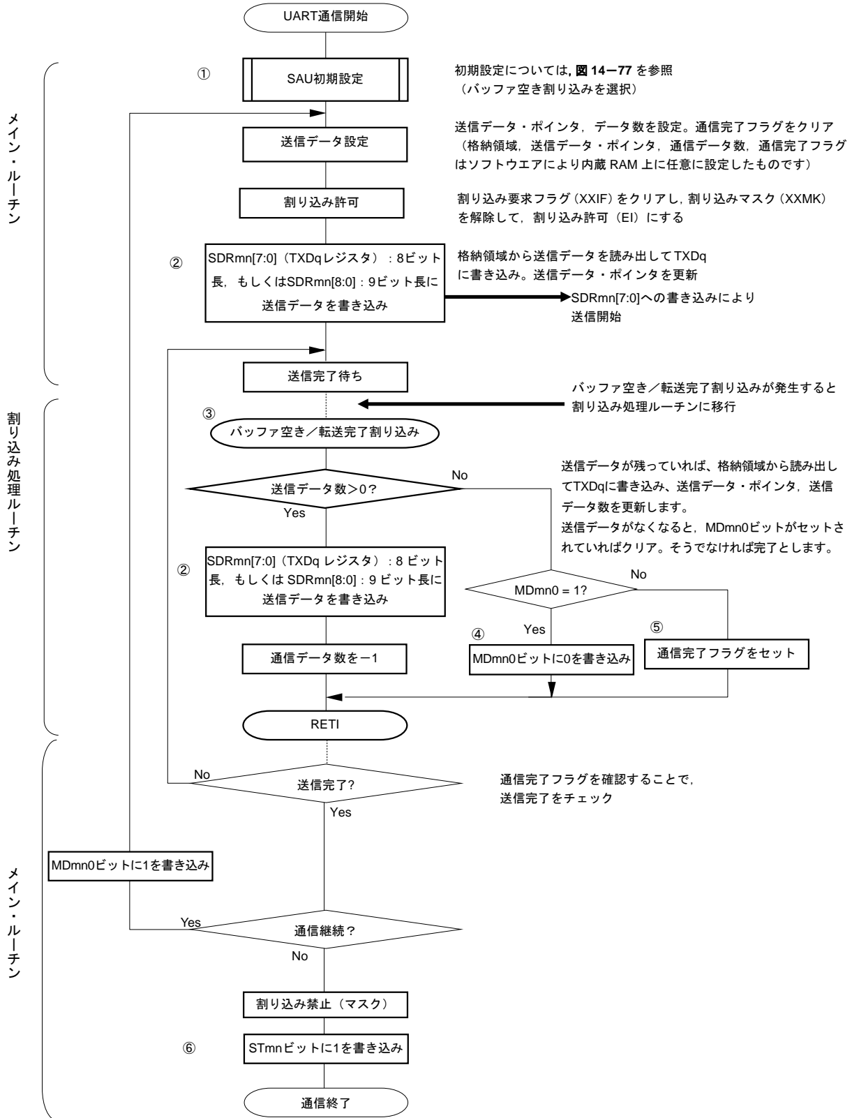
図14-83 UART送信（連続送信モード時）のフロー・チャート
