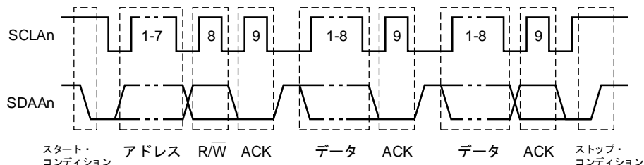
図15-14 I 2 Cバスのシリアル・データ転送タイミング
