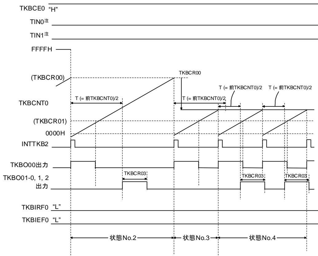
図7-49 インターリーブPFCモードのタイミング図（状態No.3～No.4の動作） （出力のデフォルト値がロウ・レベル（TKBTOD0p = 0）でアクティブ・レベルがハイ・レベル（TKBTOL0p = 0）の場合）
