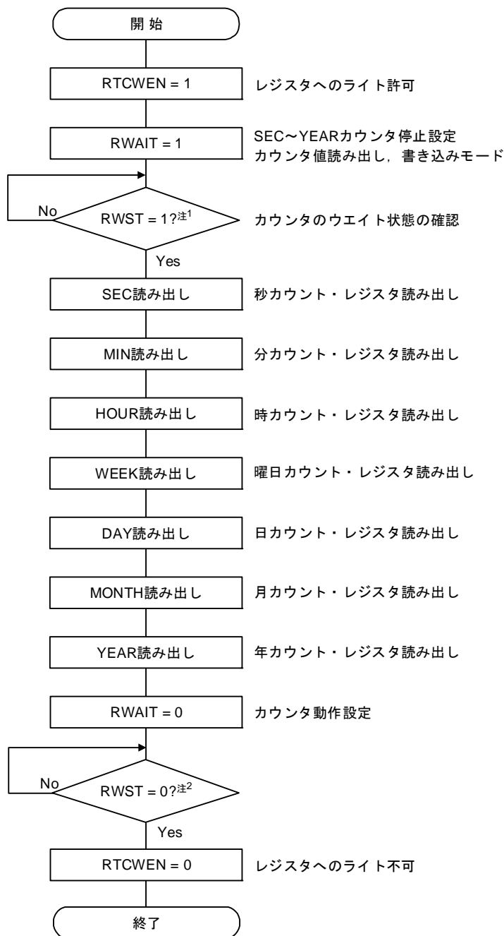
図8-20 リアルタイム・クロック2の読み出し手順
