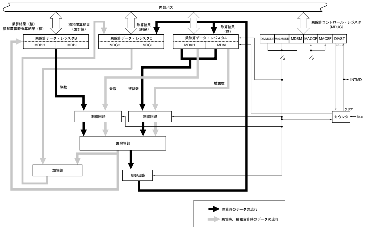
図17-1 乗除積和算器のブロック図
