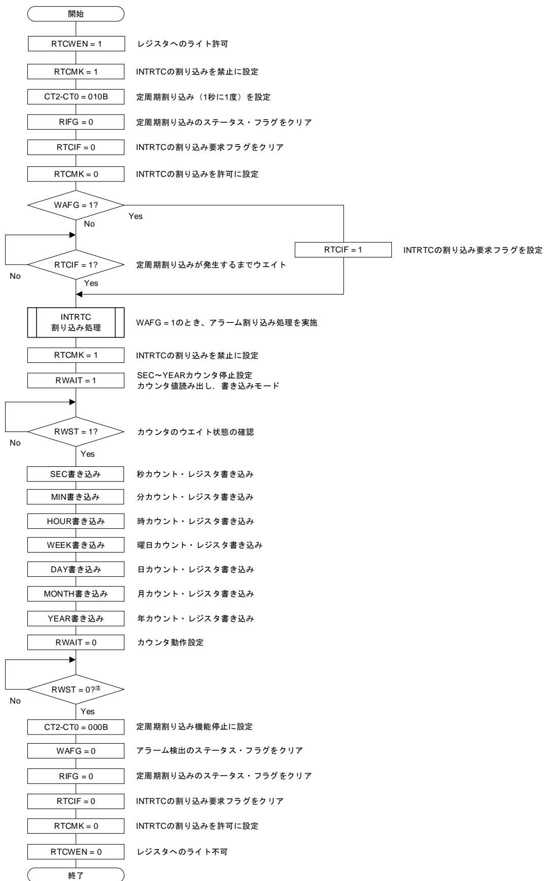
図8-23 リアルタイム・クロック2の書き込み手順（アラーム割り込み機能使用時）
