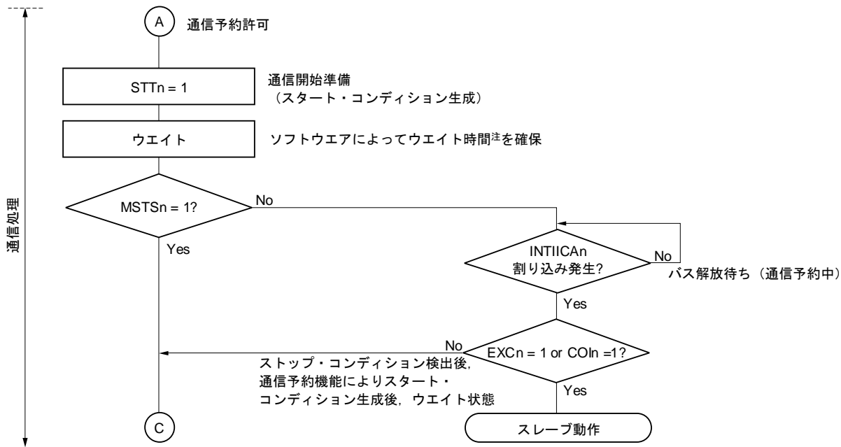
図15-29 マルチマスタ・システムでのマスタ動作 (2/3)
