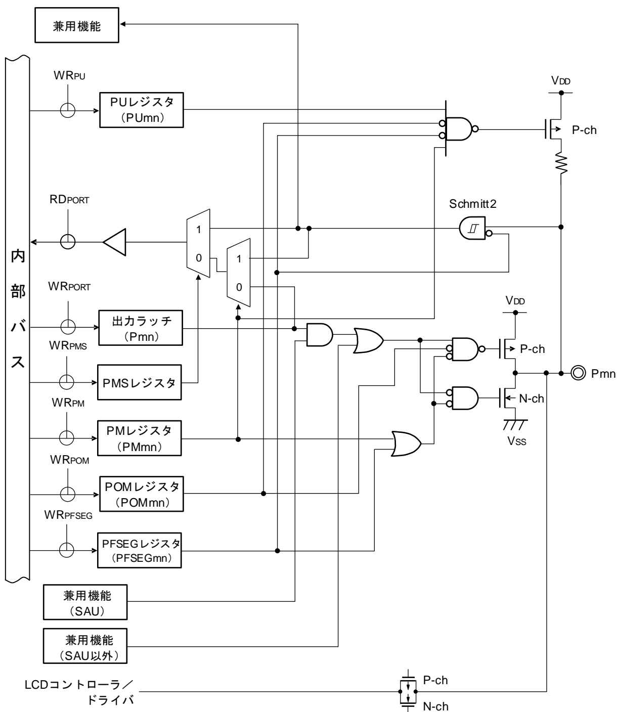
図2-9 端子タイプ 7-5-10 の端子ブロック図
