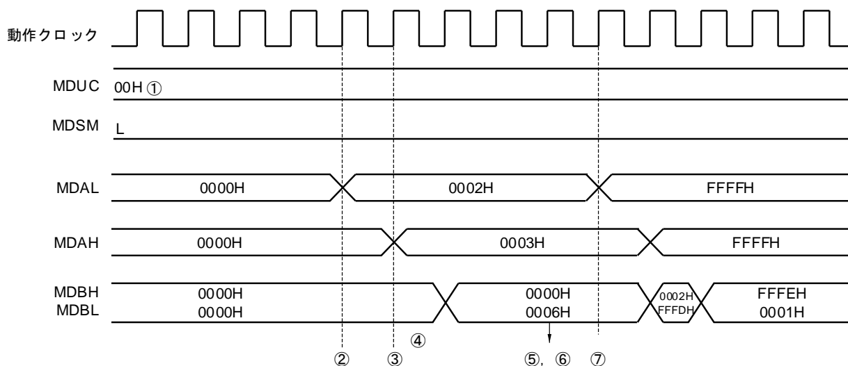
図17-6 乗算（符号なし）動作のタイミング図（2×3=6）
