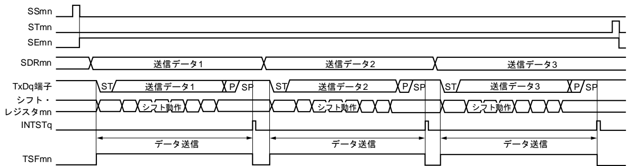
図14-80 UART送信（シングル送信モード時）のタイミング・チャート
