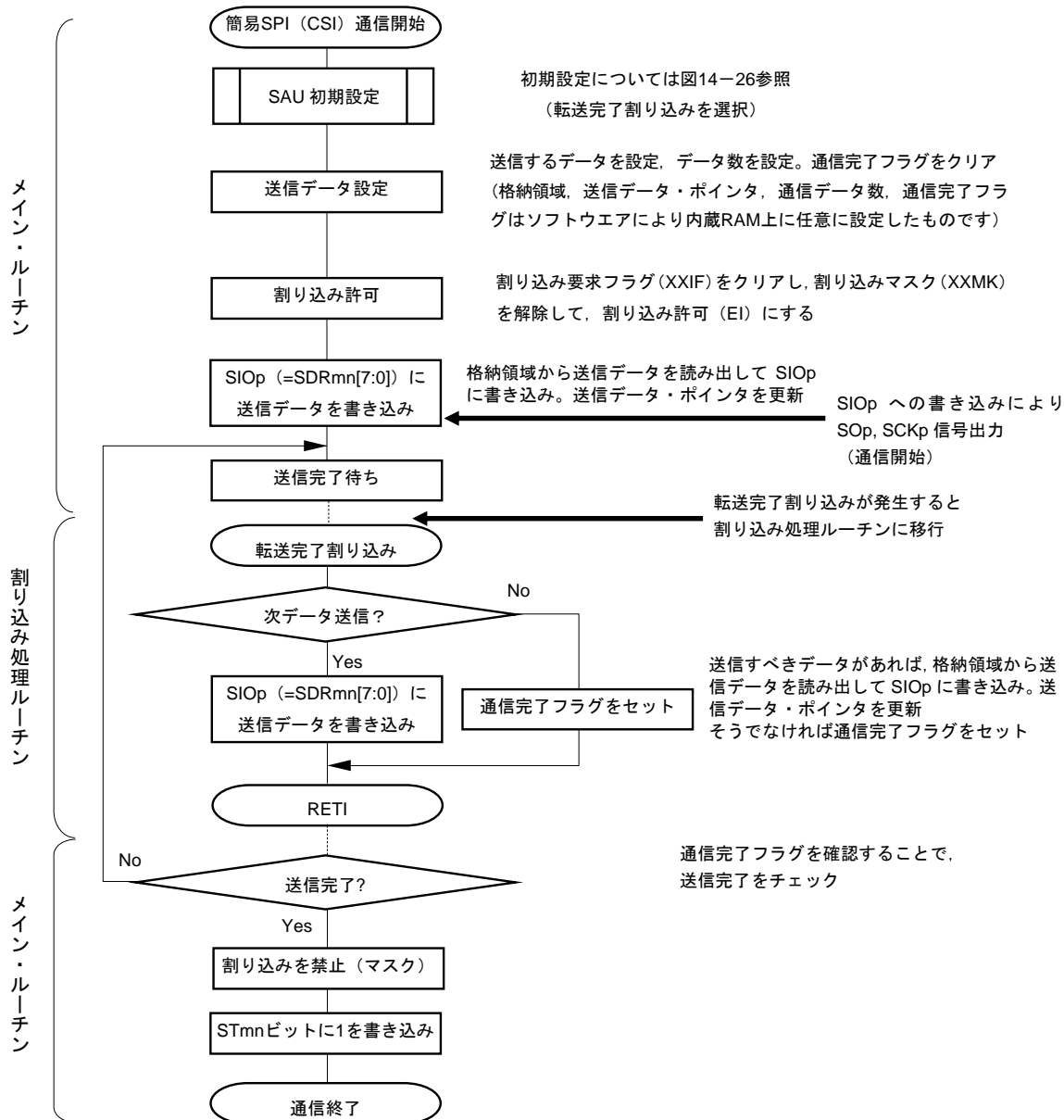
図14-30 マスタ送信（シングル送信モード時）のフロー・チャート
