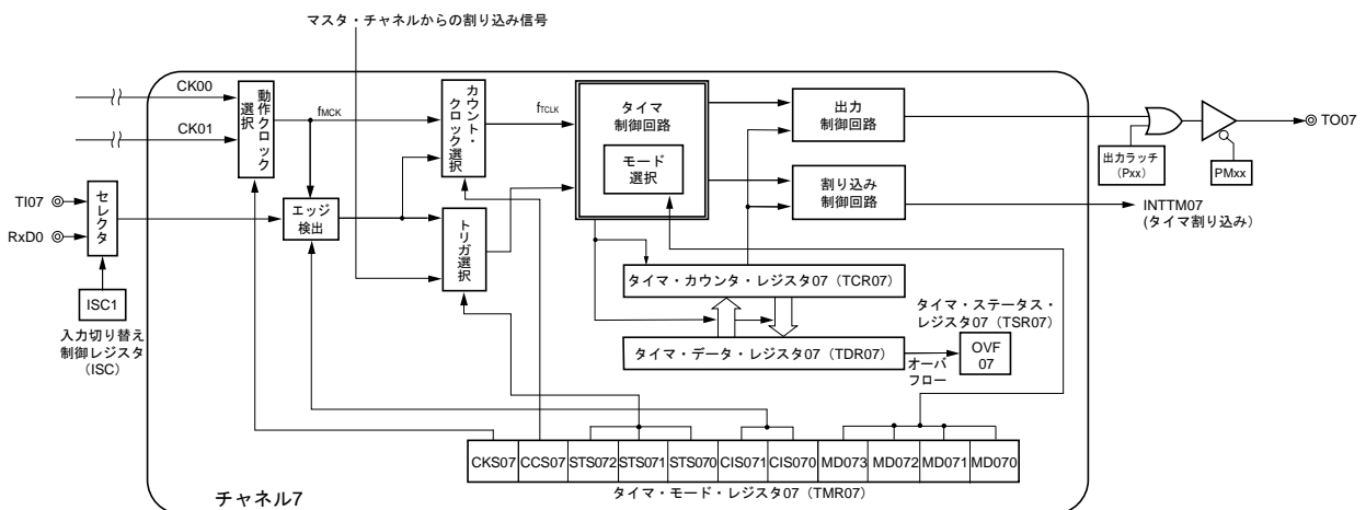
図6-6 タイマ・アレイ・ユニットのチャンネル7内部ブロック図
