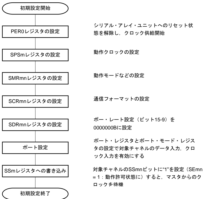
図14-58 スレーブ受信の初期設定手順
