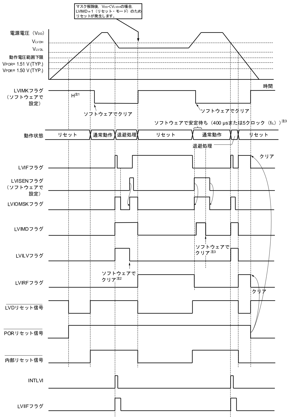
図24-7 割り込み&リセット信号発生タイミング (オプション・バイトのLVIMDS1, LVIMDS0 = 1, 0) (2/2)
