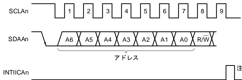
図15-16 アドレス
