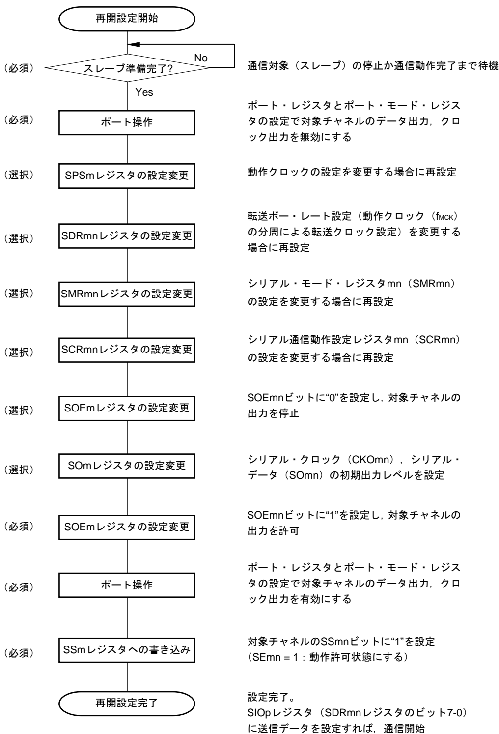
図14-28 マスタ送信の再開設定手順
