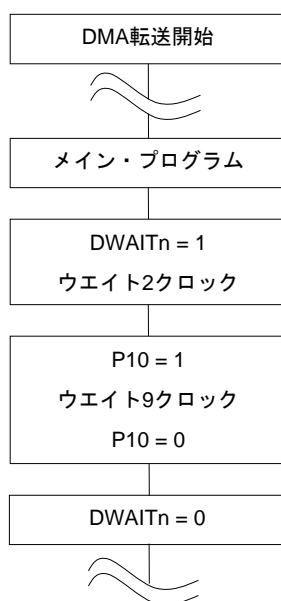
図18-10 DWAITnビットによるDMA転送保留の設定例
