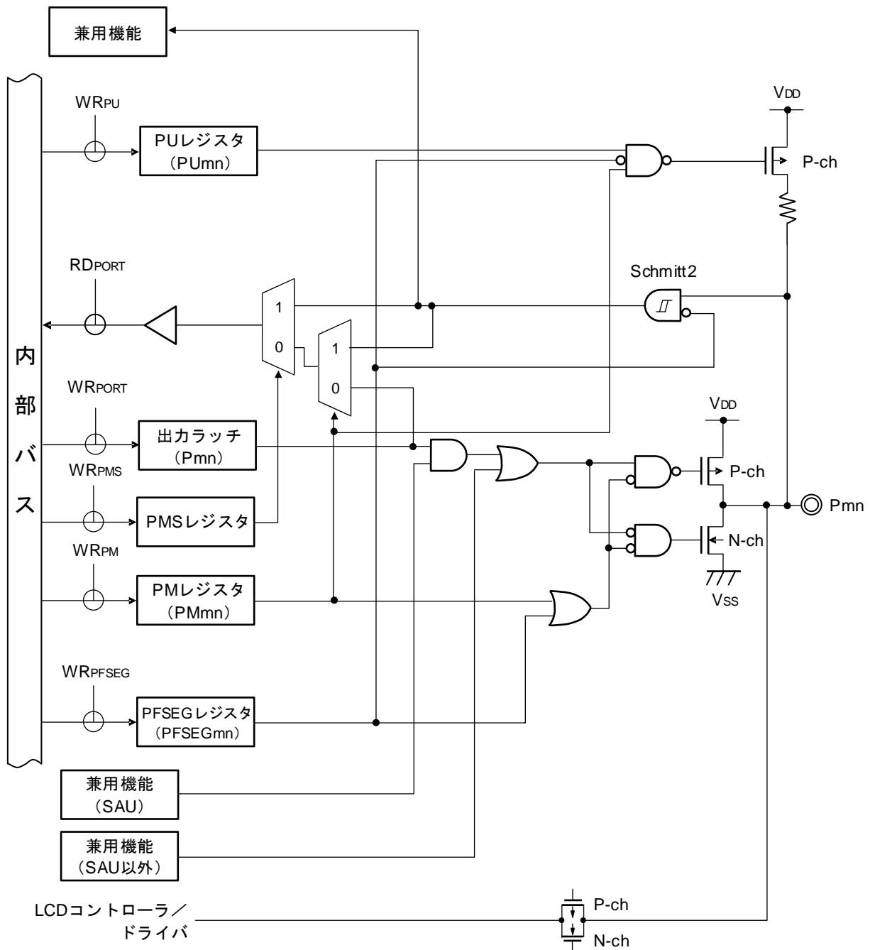
図2-6 端子タイプ 7-5-4 の端子ブロック図
