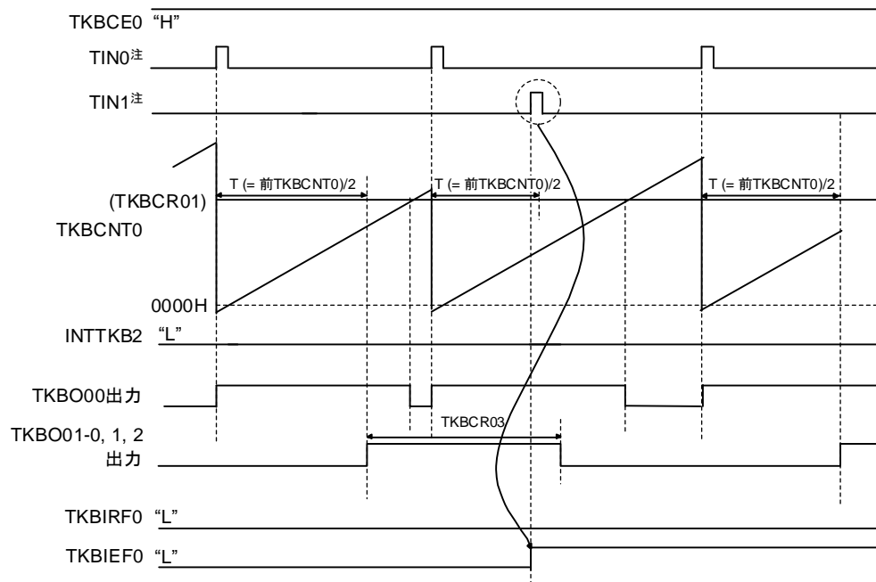
図7-55 インターリーブPFCモードのタイミング図 (TKBO01-0, TKBO01-1, TKBO01-2中に再度トリガが発生した場合)
