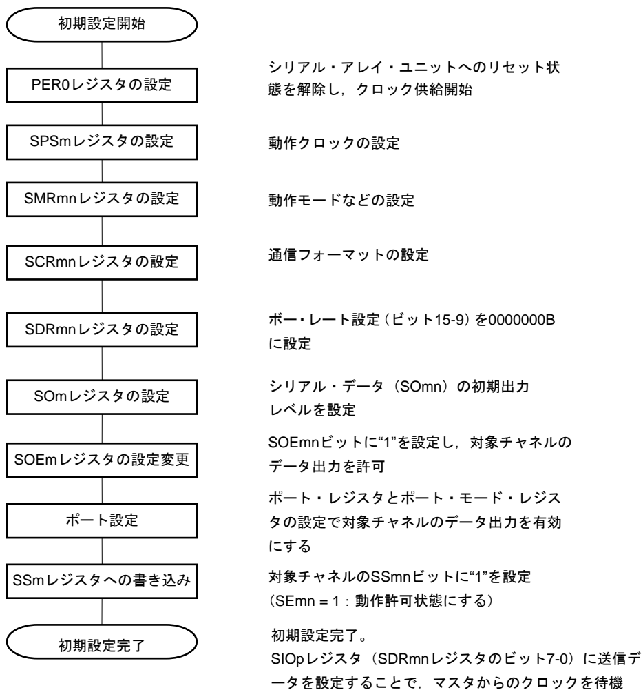
図14-64 スレーブ送受信の初期設定手順
