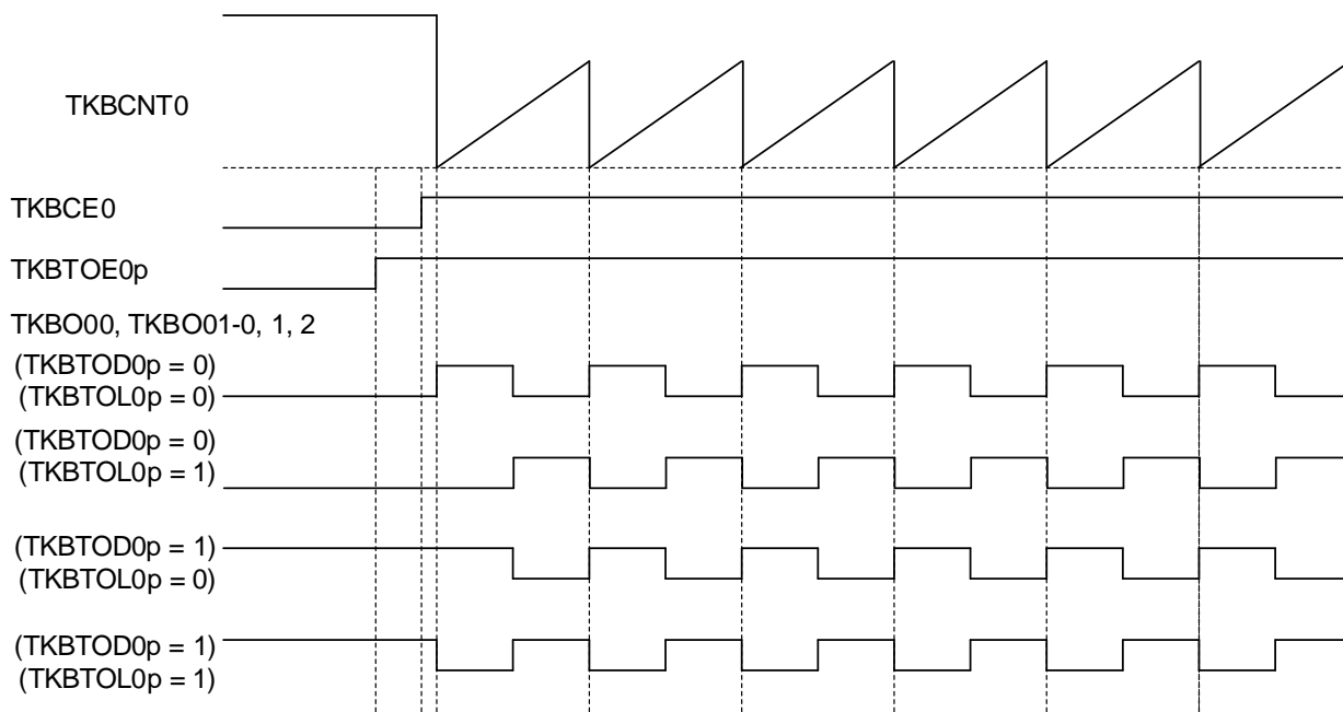
図7-27 デフォルトレベルとアクティブ・レベルのタイミング図 (基本動作)
