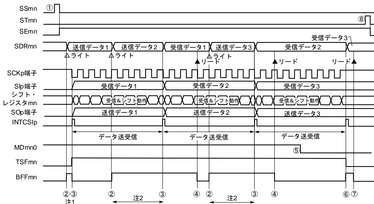
図14-47 マスタ送受信（連続送受信モード時）のタイミング・チャート（タイプ1：DAPmn = 0, CKPmn = 0）
