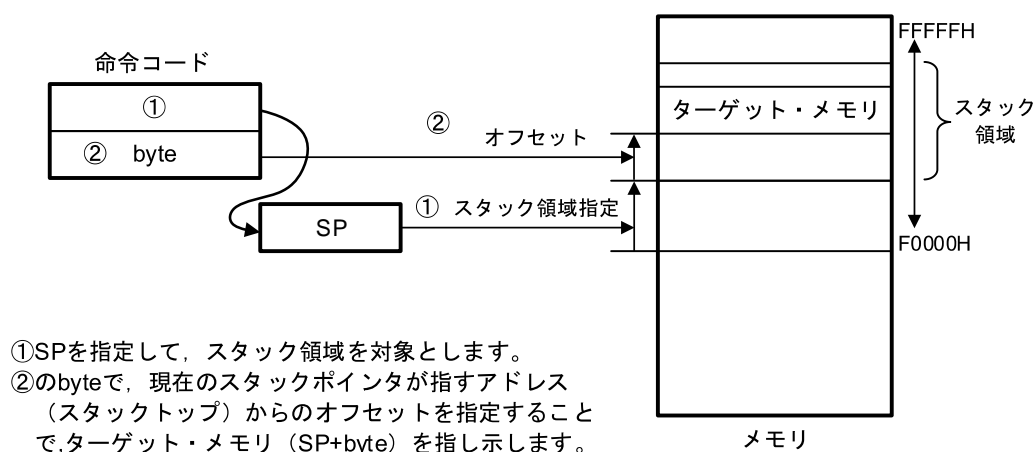
図3-28 [SP+byte]の例
