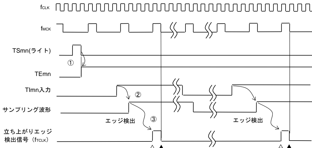
図6-26 カウント・クロック ( f_{CLK} ) のタイミング (CCSmn = 1, ノイズ・フィルタ未使用時)
