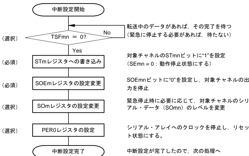
図14-78 UART送信の中断手順
