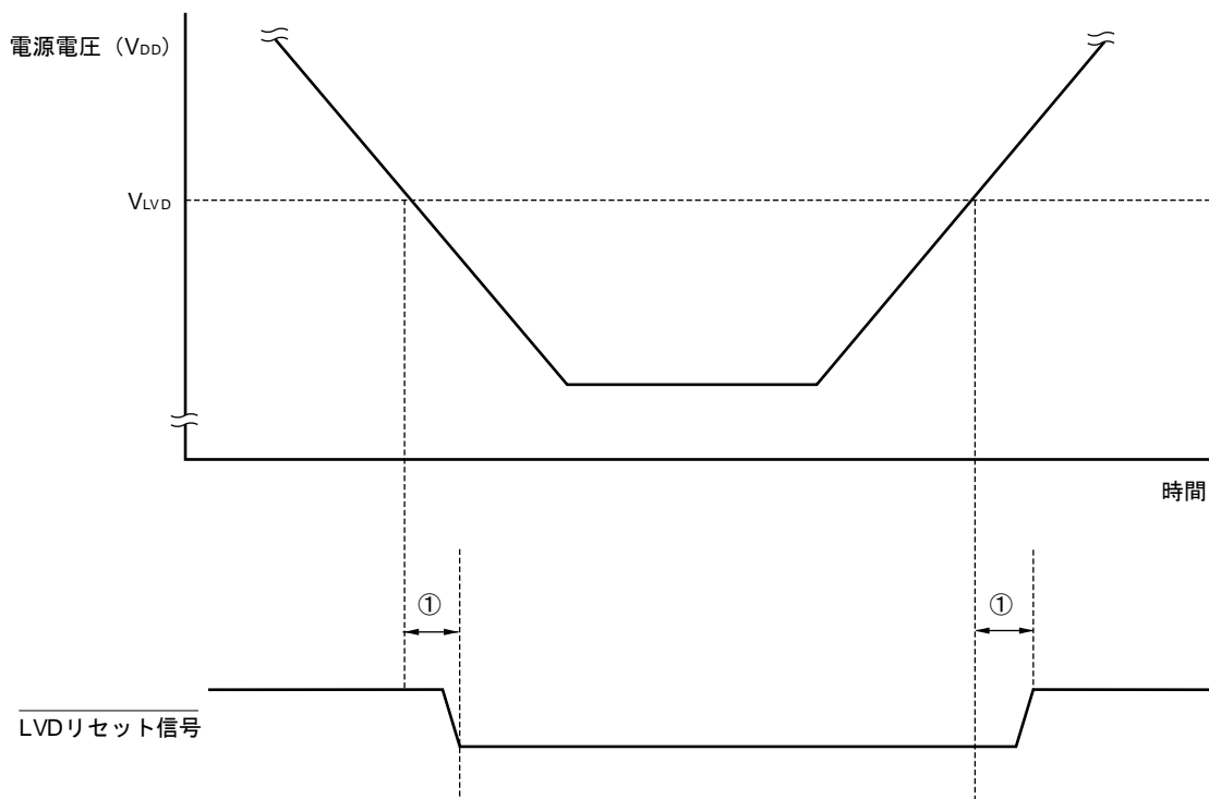
図24-11 LVDリセット要因発生からLVDリセット発生または解除までの遅延
