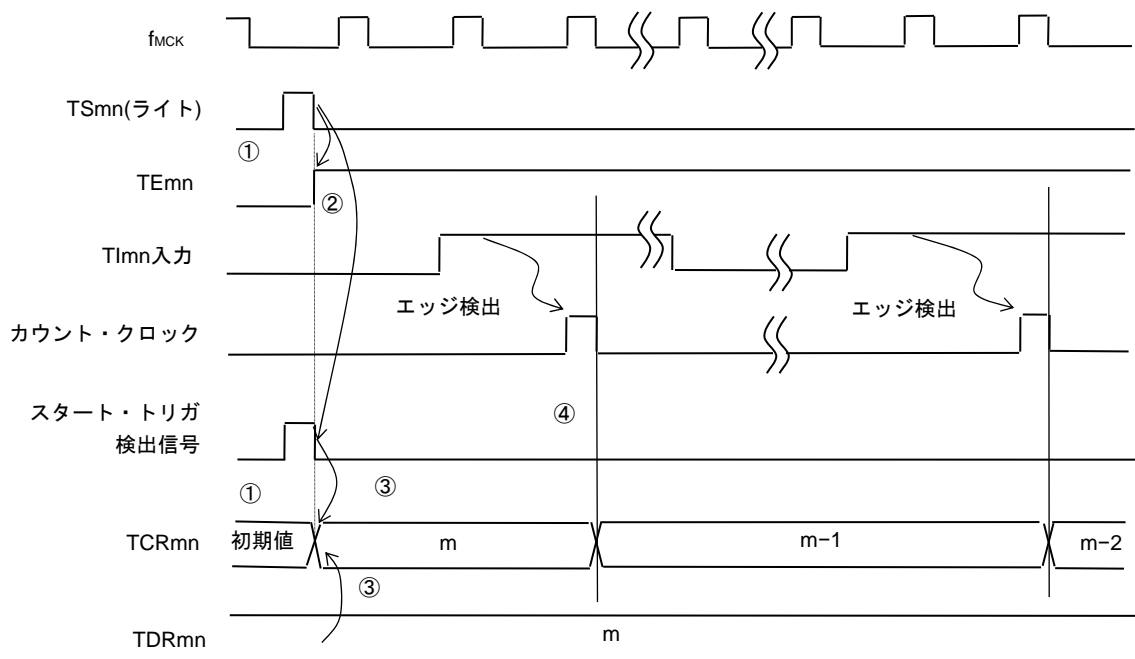
図6-28 動作タイミング (イベント・カウンタ・モード)
