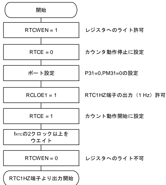
図8-25 1 Hz出力の設定手順
