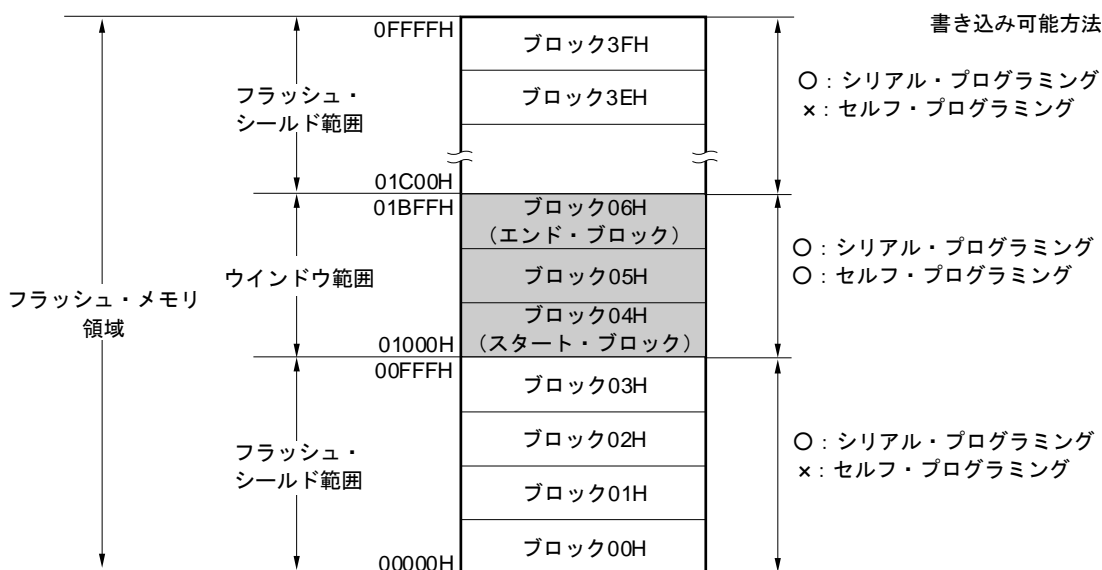
図28-11 フラッシュ・シールド・ウインドウの設定例 (対象デバイス：R5F10WLE, スタート・ブロック：04H, エンド・ブロック：06Hの場合)
