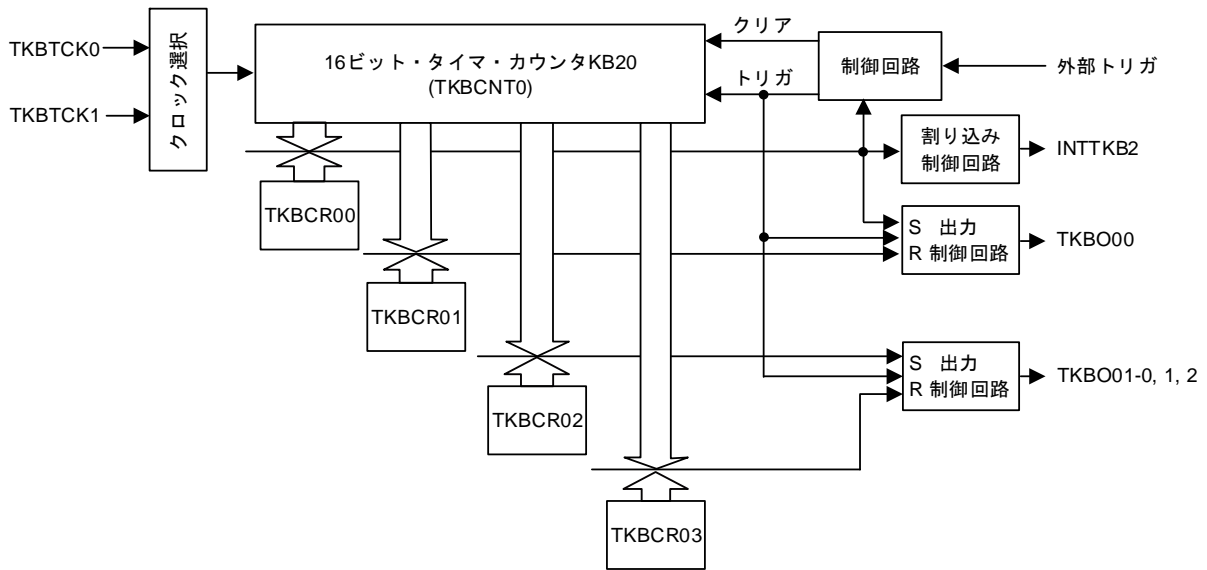
図7-44 単体動作時の構成図（外部トリガ入力による周期制御）
