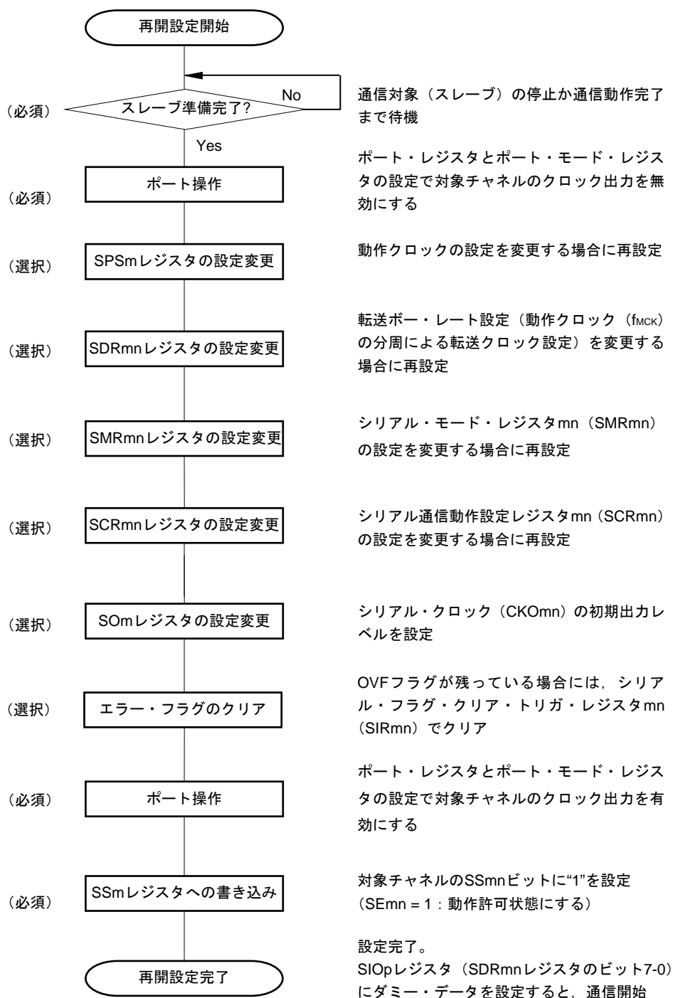
図14-36 マスタ受信の再開設定手順
