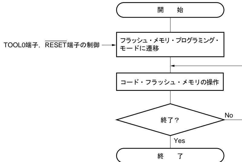
図28-6 コード・フラッシュ・メモリの操作手順
