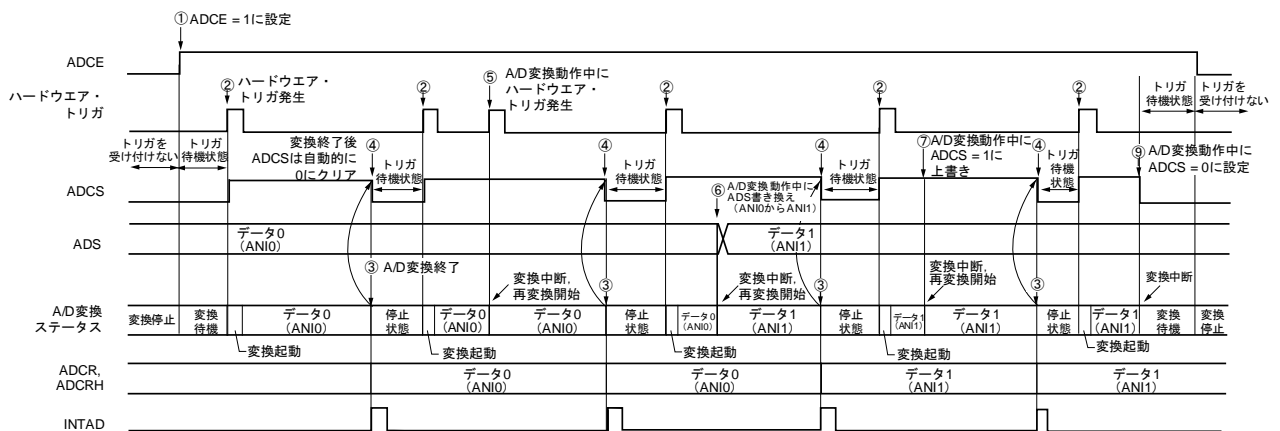
図12-22 ハードウェア・トリガ・ウエイト・モード（ワンショット変換モード）動作タイミング例
