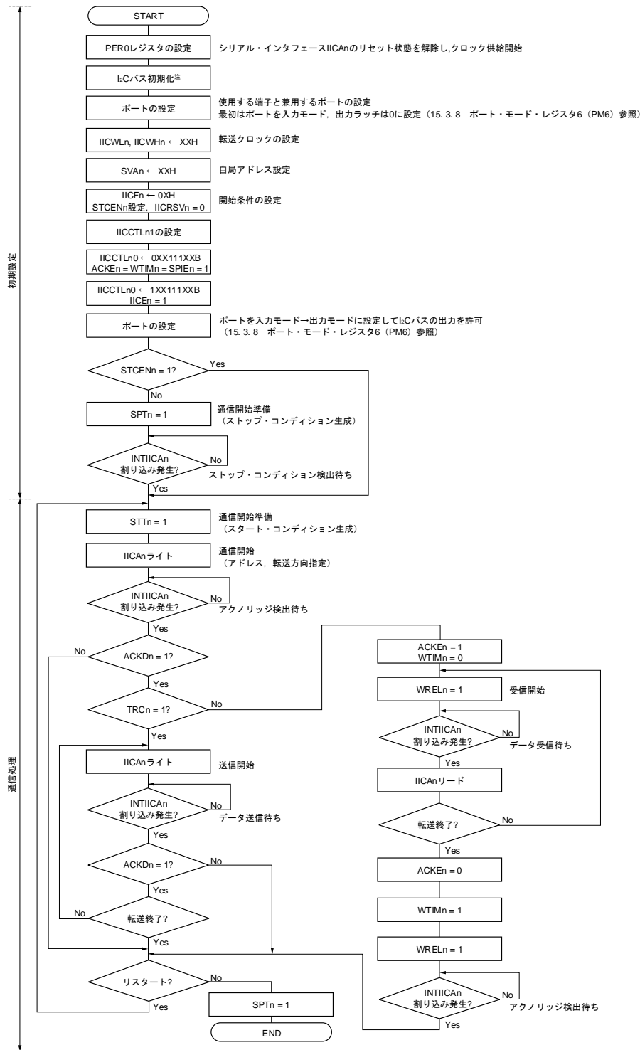
図15-28 シングルマスタ・システムでのマスタ動作
