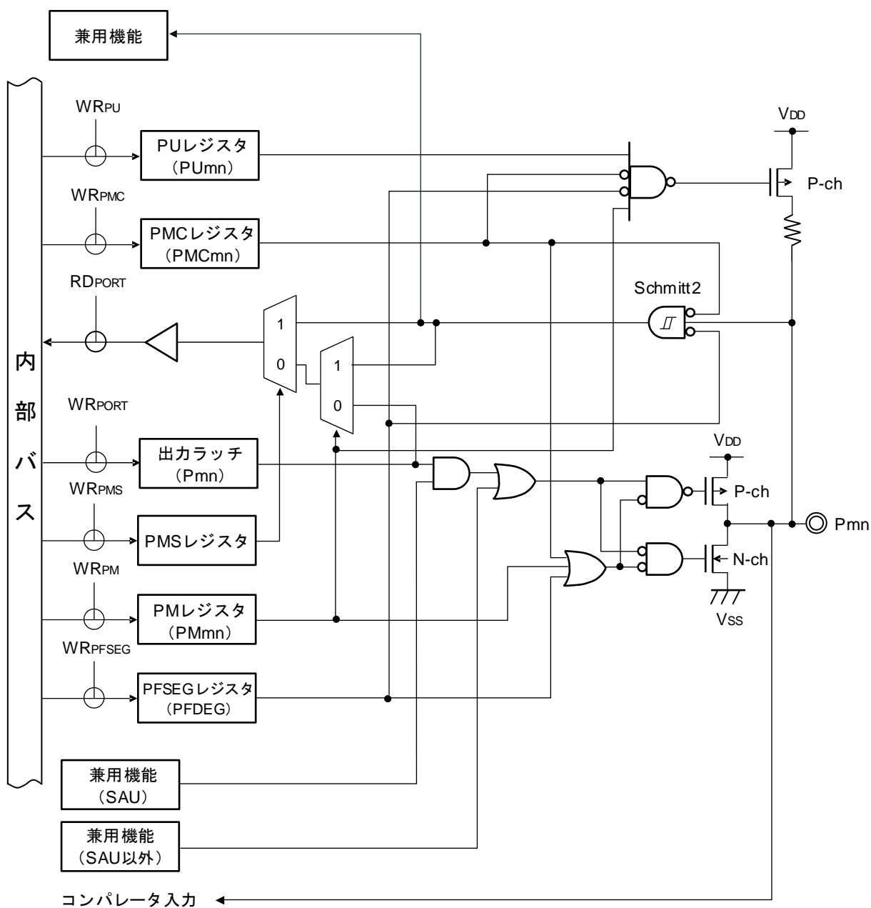
図2-12 端子タイプ 7-6-9 の端子ブロック図
