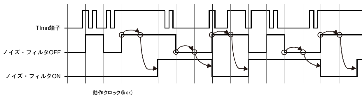
図6-42 TImn入力端子に対するノイズ・フィルタON/OFFによるサンプリング波形
