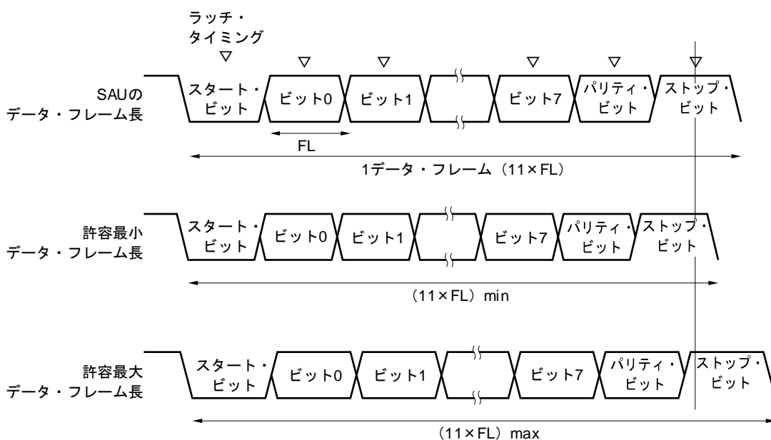
図14-95 受信時の許容ボー・レート範囲 (1データ・フレーム長 = 11ビットの場合)
