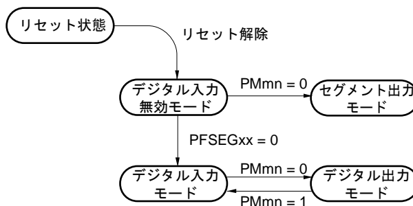
図16-11 SEGxx/ポート端子機能の状態遷移図
