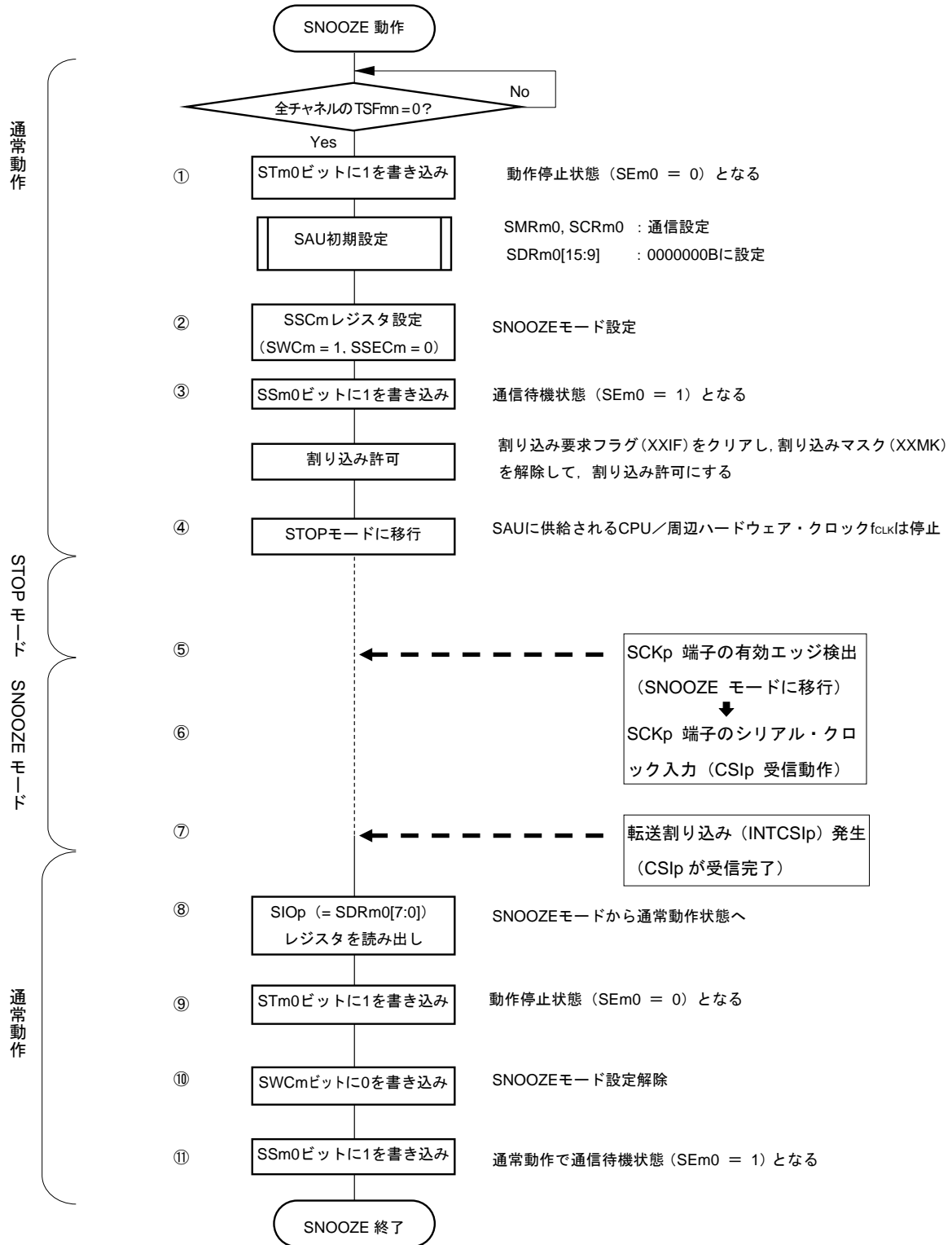
図14-72 SNOOZEモード動作（1回起動）時のフロー・チャート
