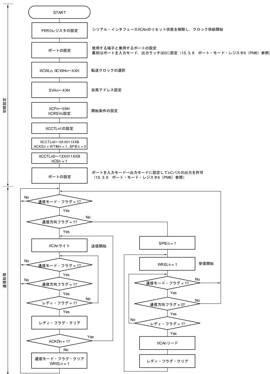
図15-30 スレーブ動作手順 (1)
