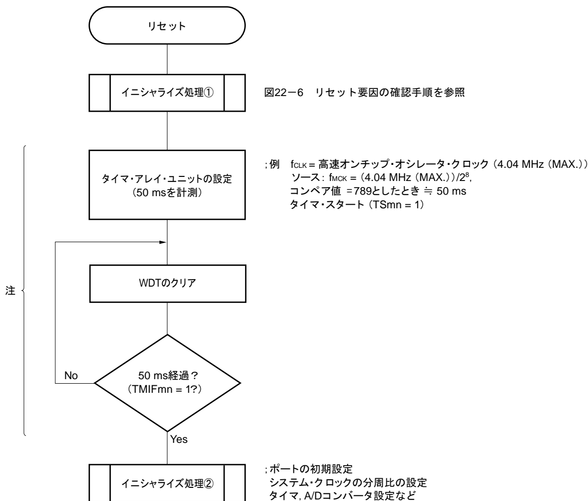
図24-10 LVD検出電圧付近での電源電圧変動が50 ms以下の場合のソフト処理例
