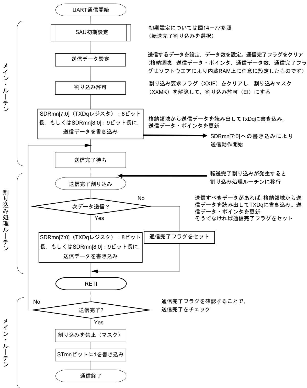
図14-81 UART送信（シングル送信モード時）のフロー・チャート
