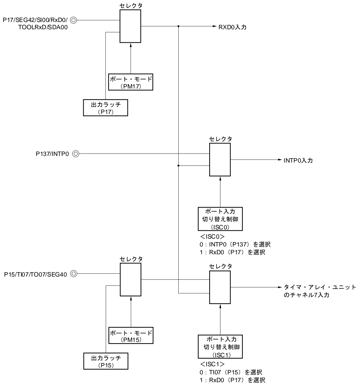
図14-102 LINの受信操作のポート構成図
