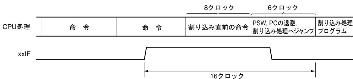
図19-9 割り込み要求の受け付けタイミング（最大時間）
