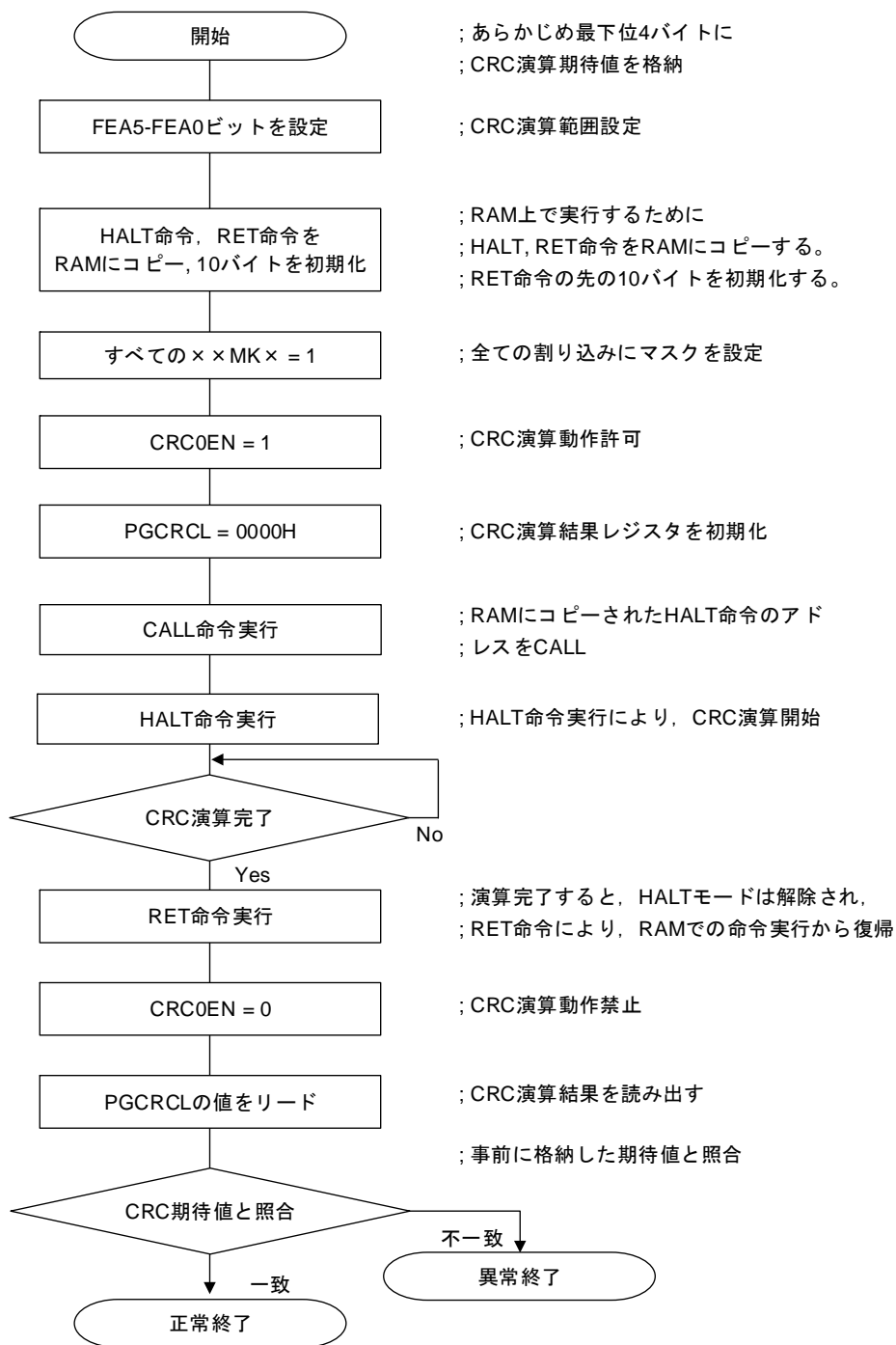
図25-3 フラッシュ・メモリCRC演算機能（高速CRC）のフロー・チャート
