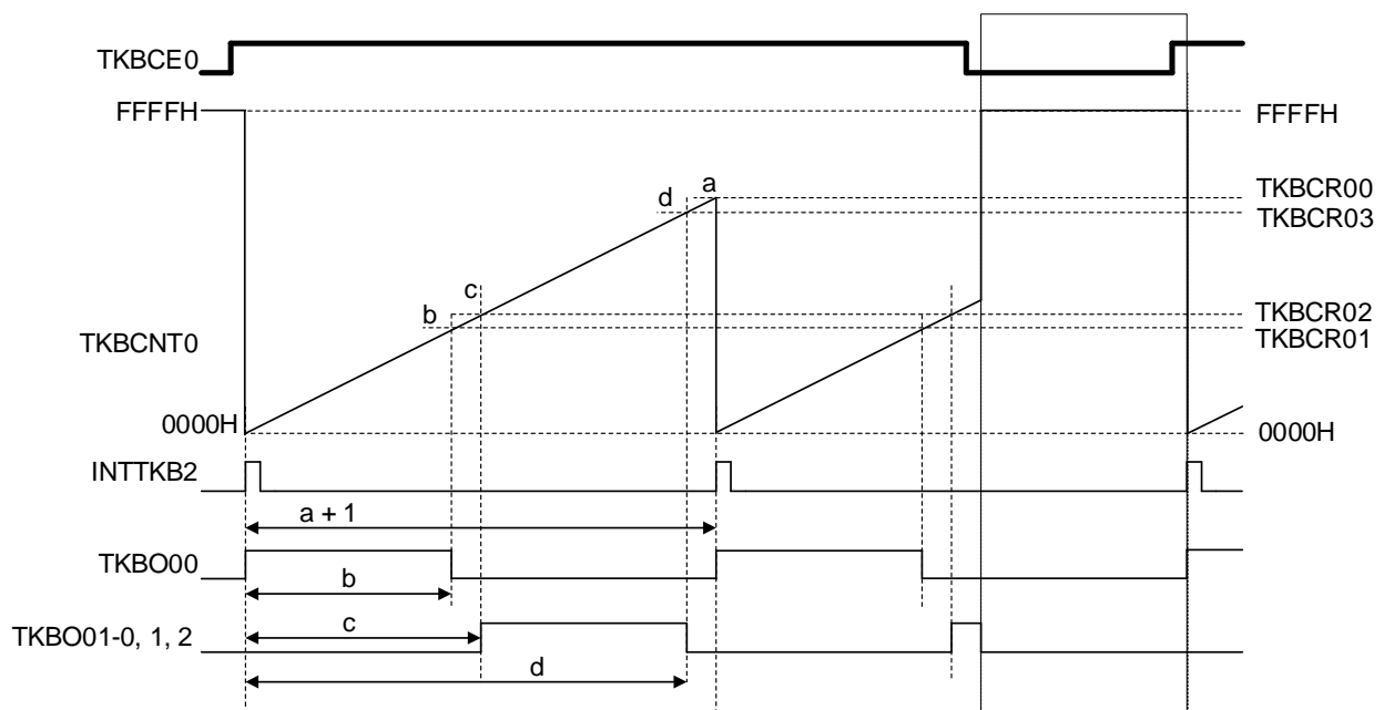
図7-34 動作停止のタイミング図 (TKBTOL0p = 0, TKBTOD0p = 0時)
