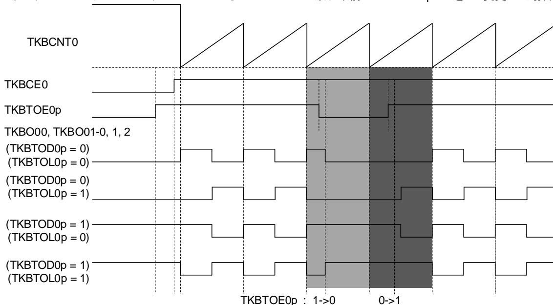
図7-29 デフォルトレベルとアクティブ・レベルのタイミング図
