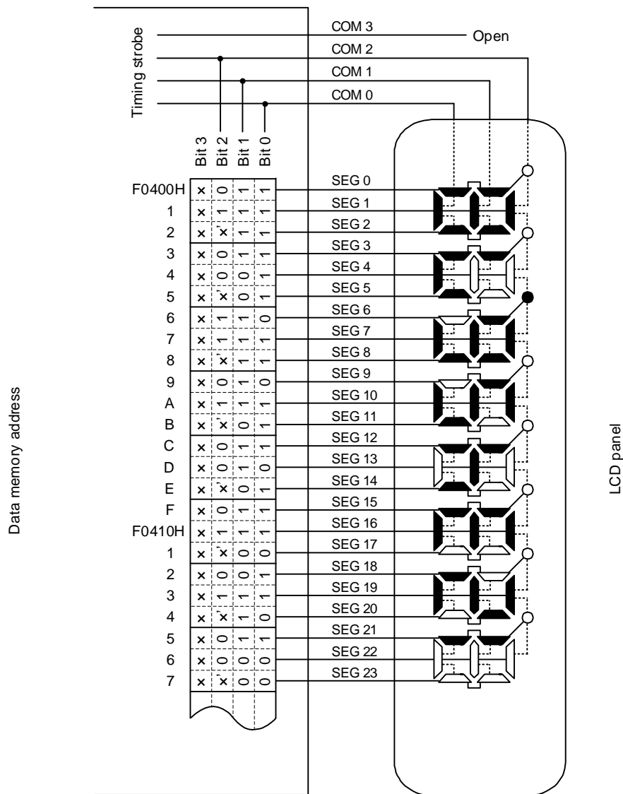
図16-33 3時分割LCDパネルの結線例
