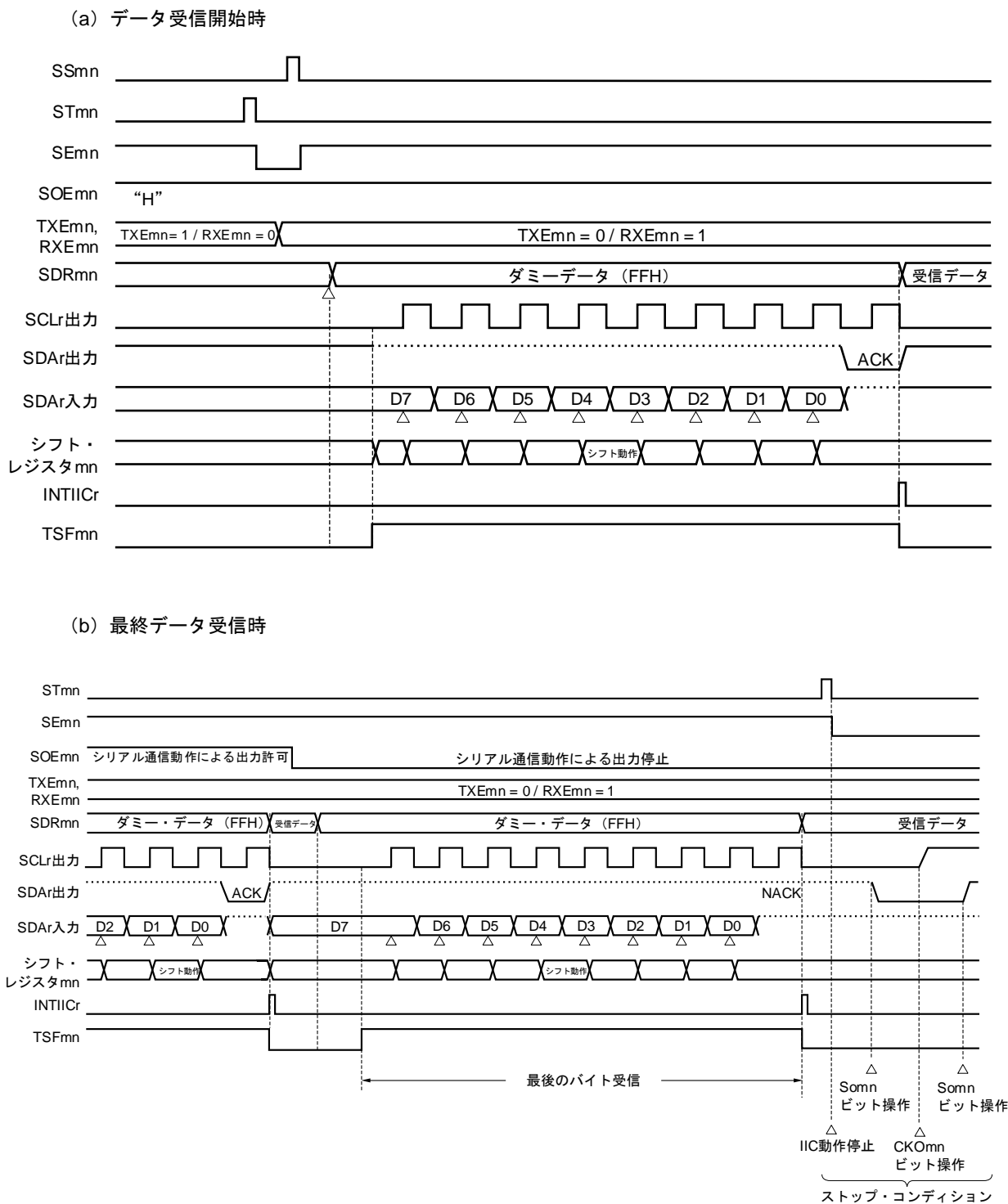
図14-111 データ受信のタイミング・チャート
