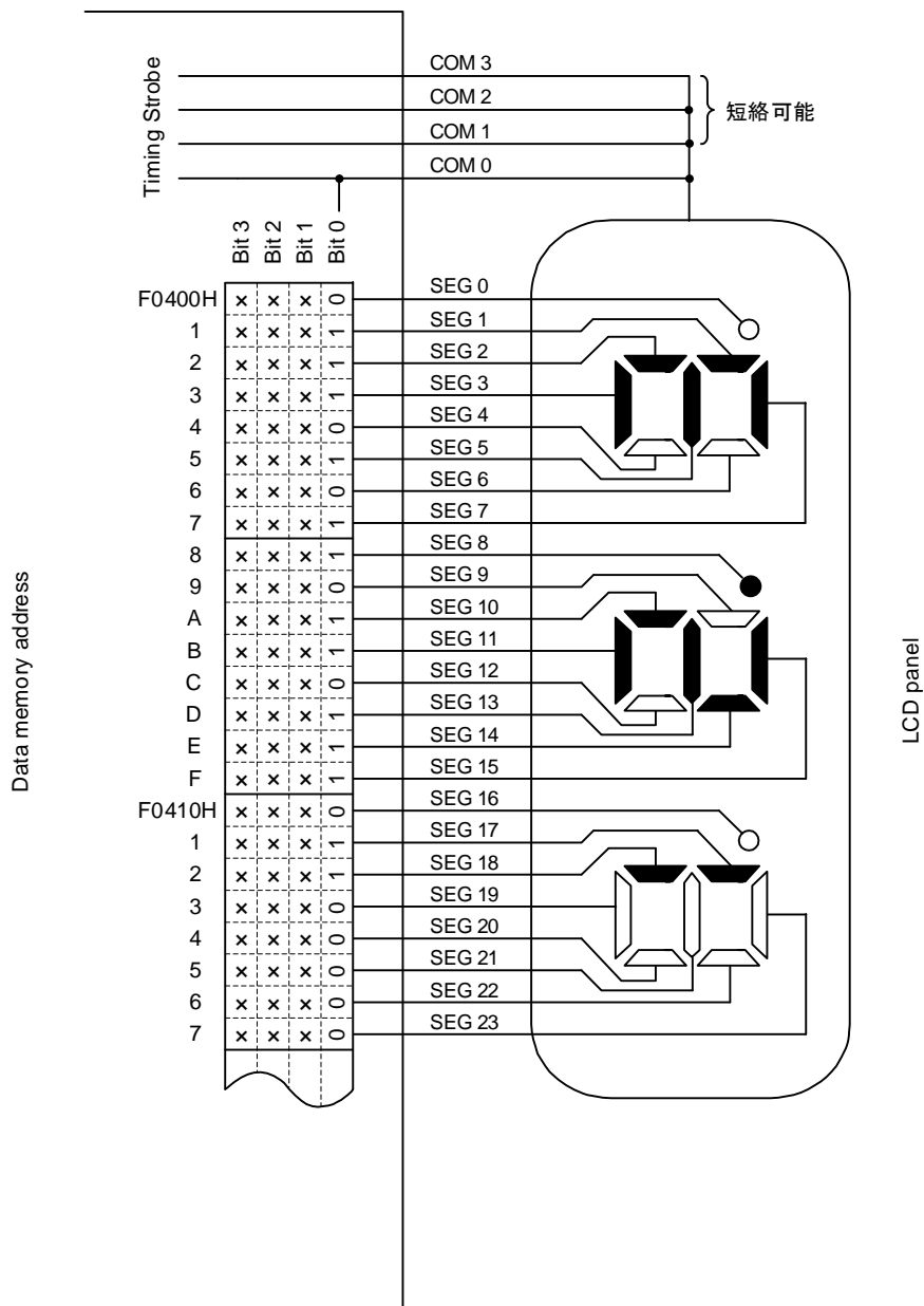
図16-27 スタティックLCDパネルの結線例
