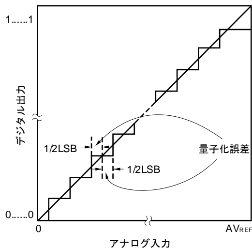
図12-33 量子化誤差
