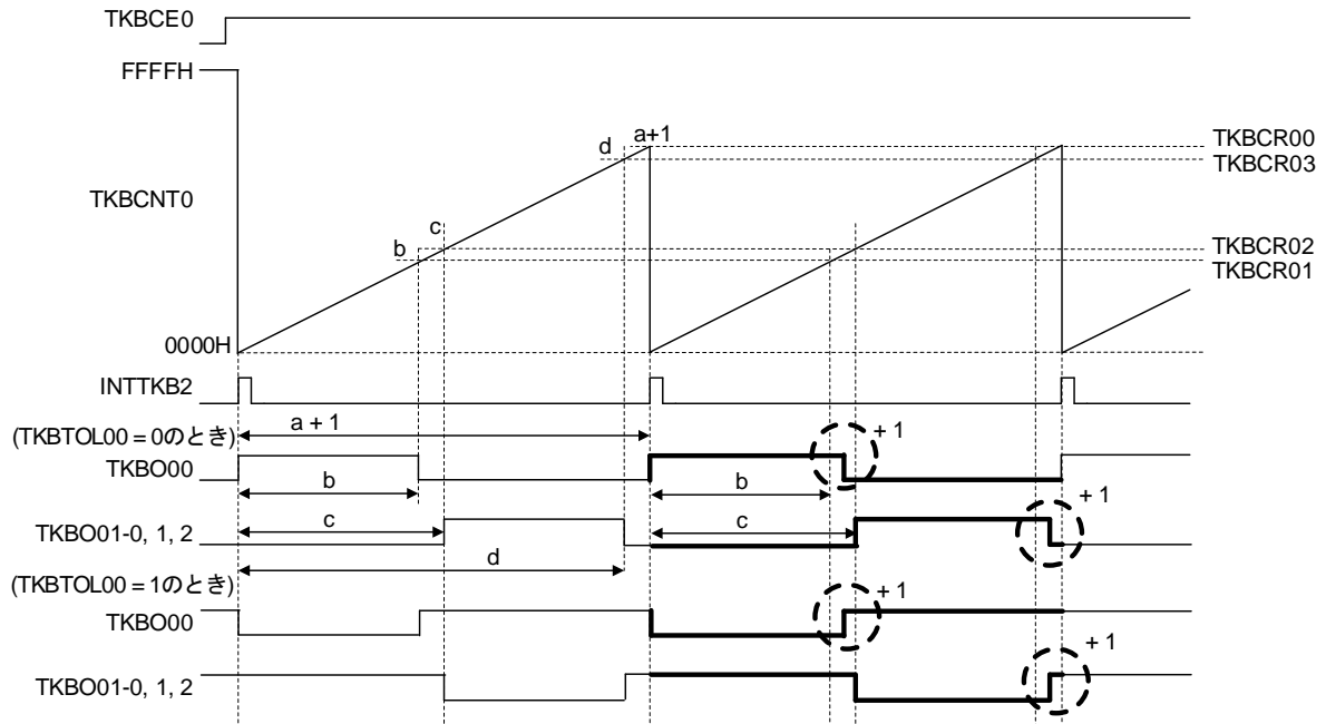
図7-59 ディザリング動作の波形図
