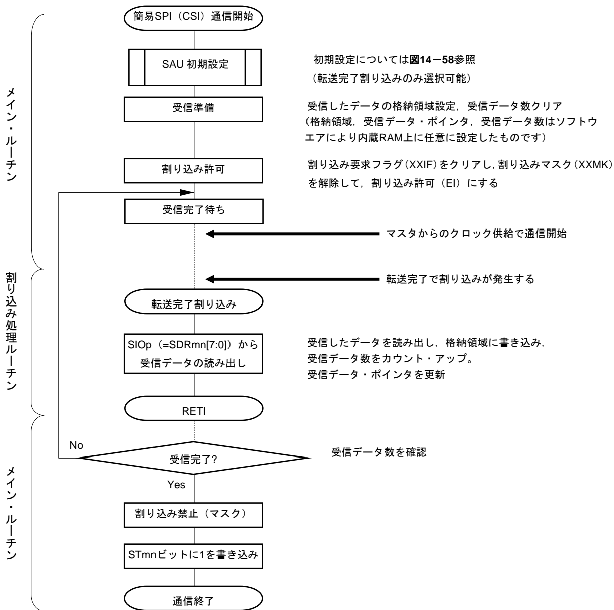
図14-62 スレーブ受信（シングル受信モード時）のフロー・チャート
