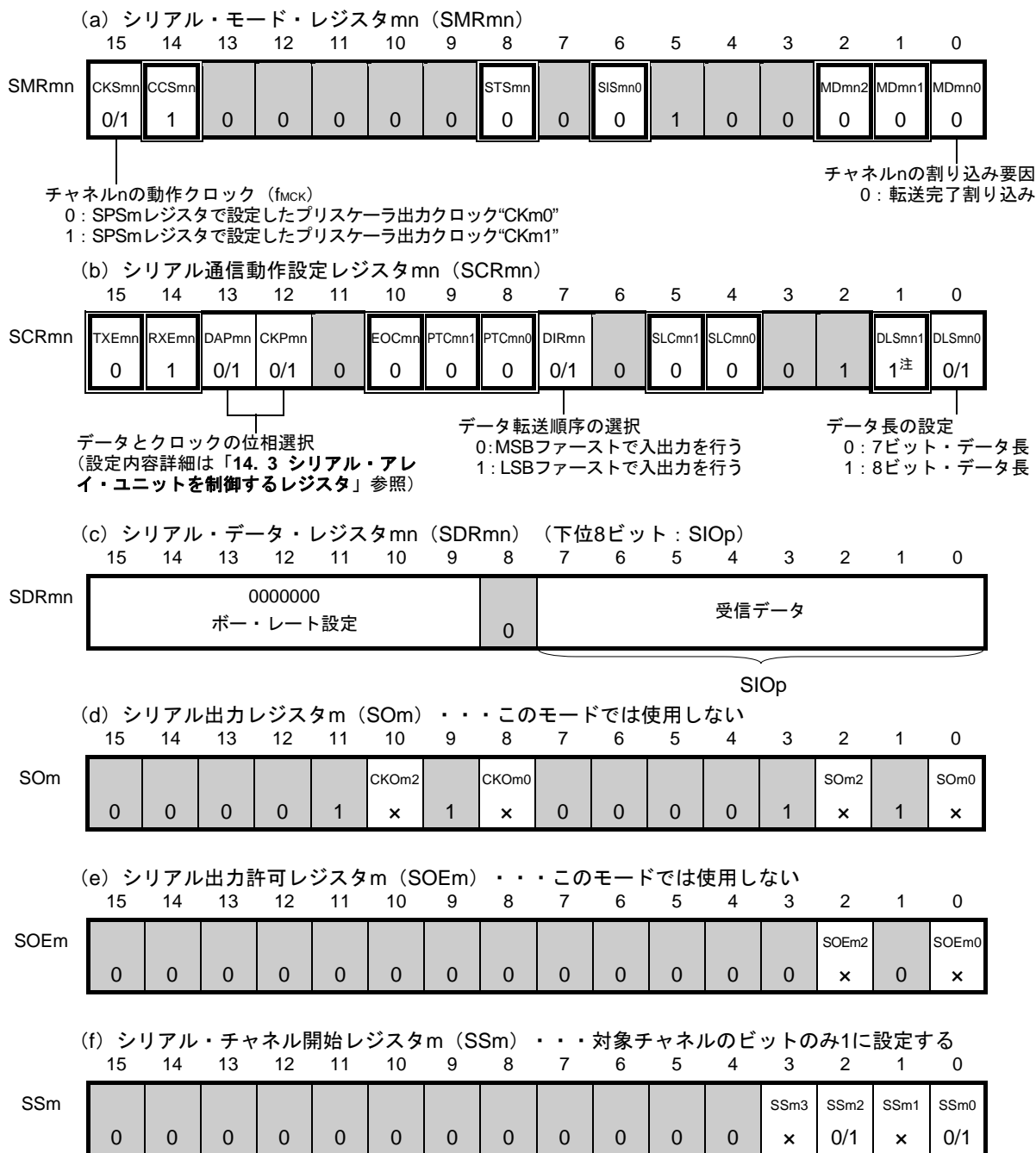
図14-57 簡易SPI (CSI00, CSI10) のスレーブ受信時のレジスタ設定内容例
