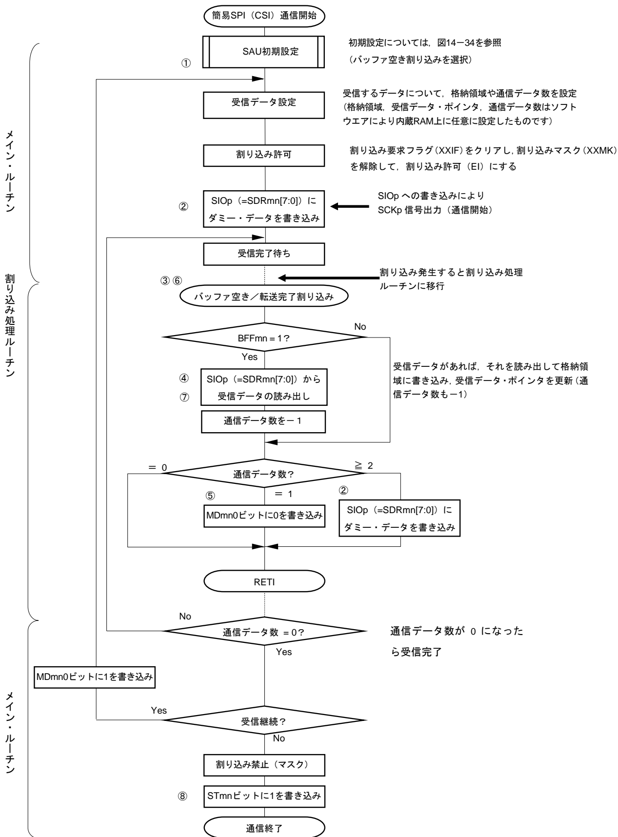
図14-40 マスタ受信（連続受信モード時）のフロー・チャート
