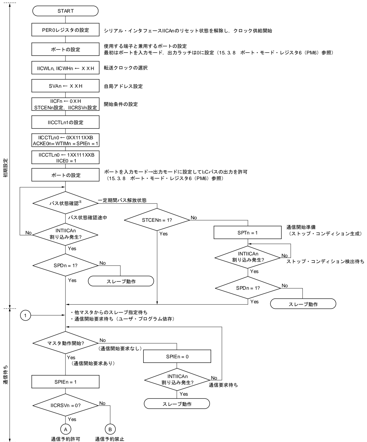
図15-29 マルチマスタ・システムでのマスタ動作 (1/3)
