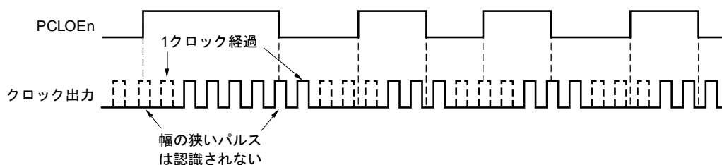
図10-4 PCLBUZn端子からのクロック出力のタイミング
