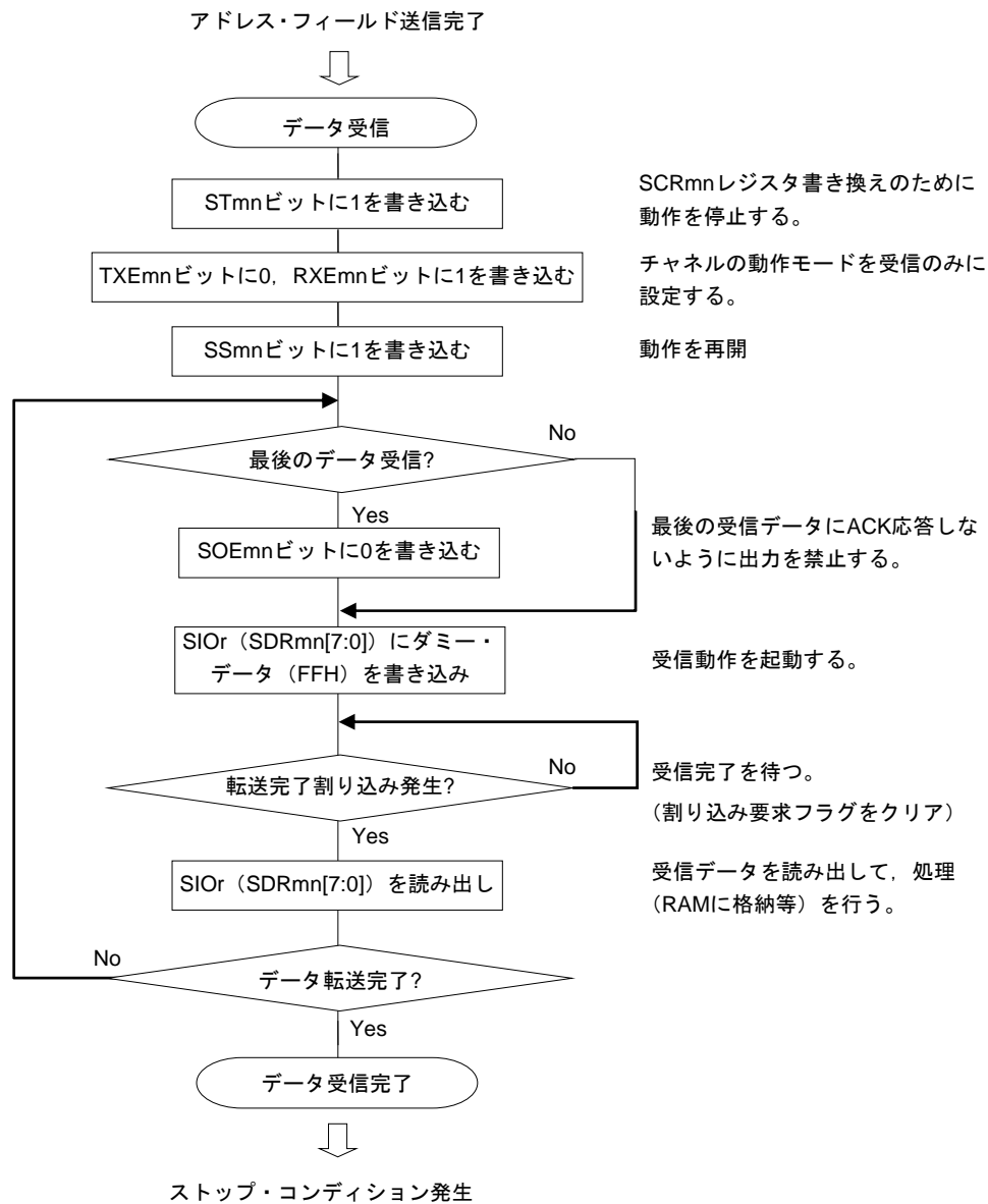
図14-112 データ受信のフロー・チャート
