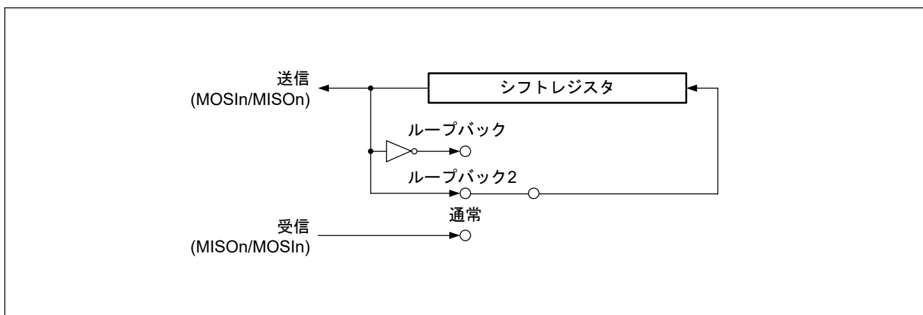
図 27.42 ループバックモード時のシフトレジスタ入出力経路の構成 (マスタモード)
