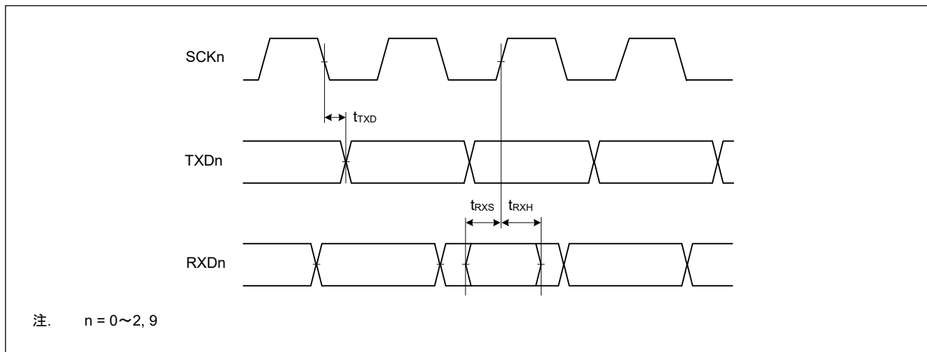
図 39.21 クロック同期式モードにおける SCI 入出力タイミング
