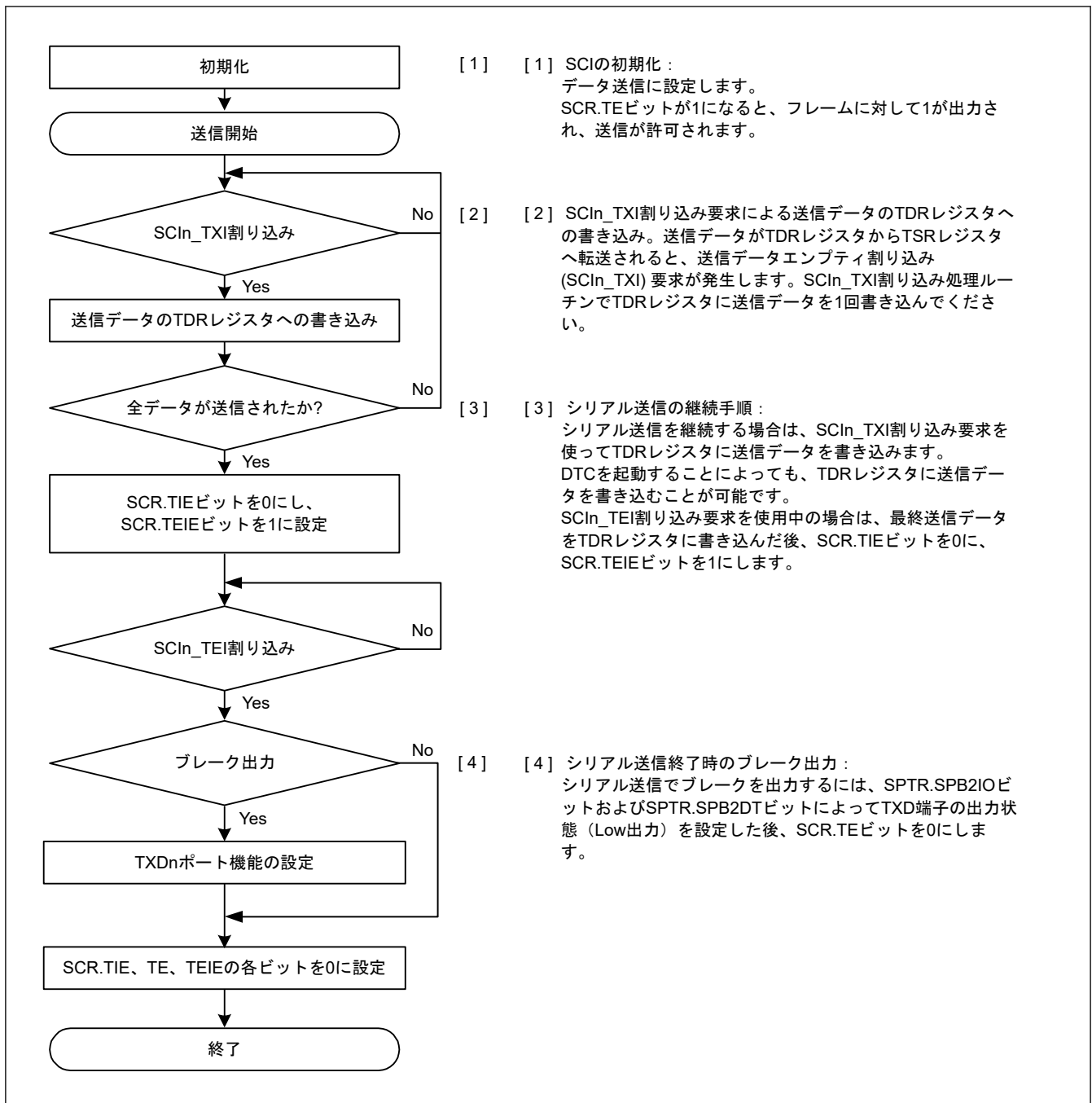
図 25.10 調歩同期式モードにおけるシリアル送金のフローチャート例 (非 FIFO 選択時)
