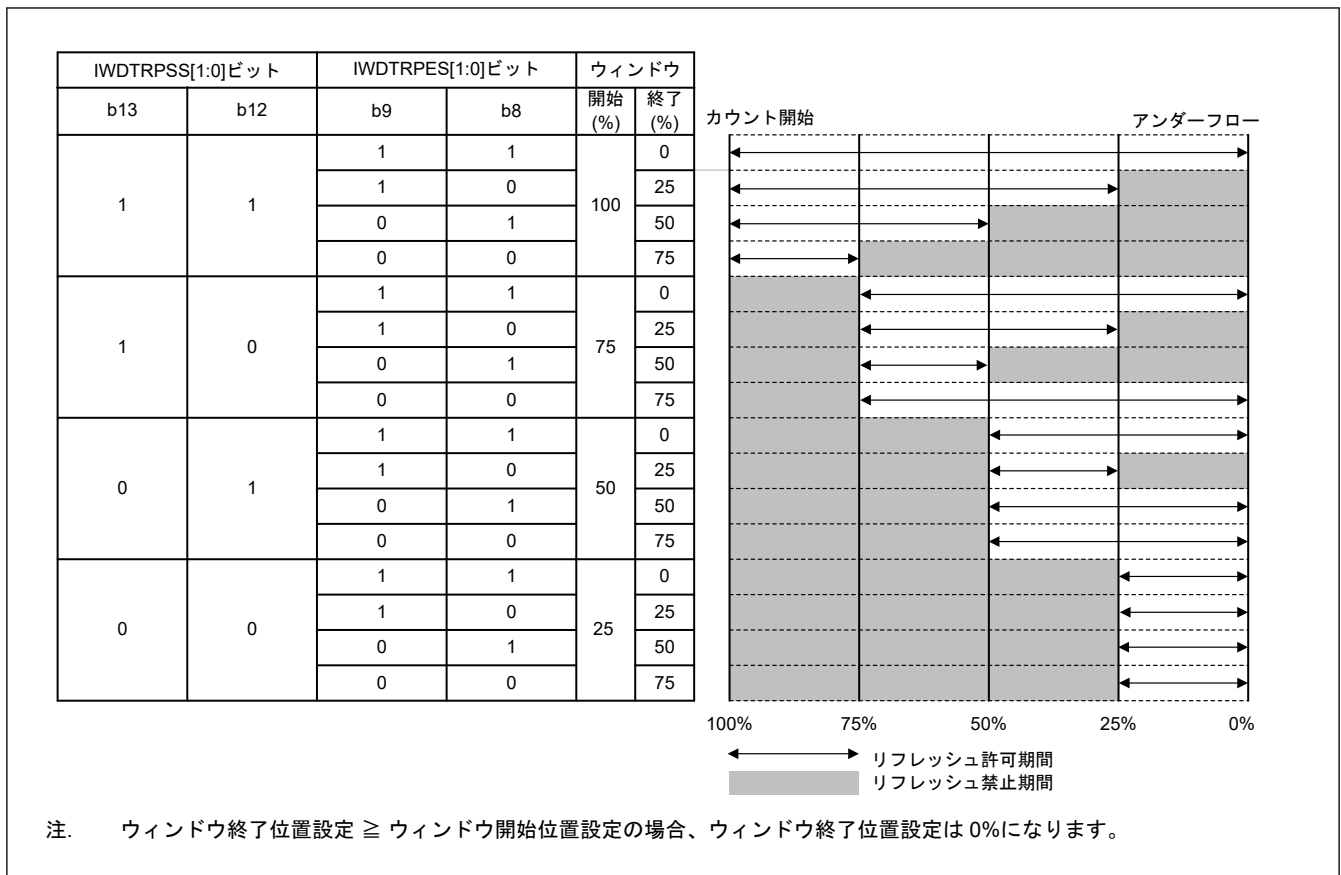
図 24.2 IWDRPSS[1:0]および IWDTPES[1:0]ビットとリフレッシュ許可期間
