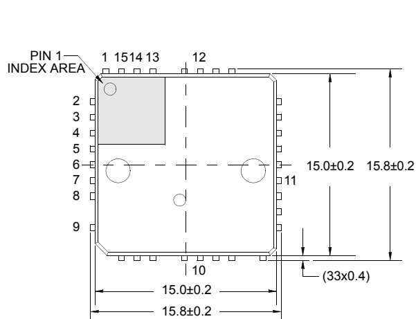
上面図
