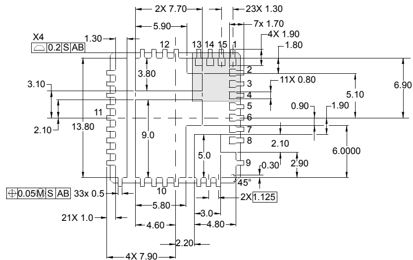
底面図
