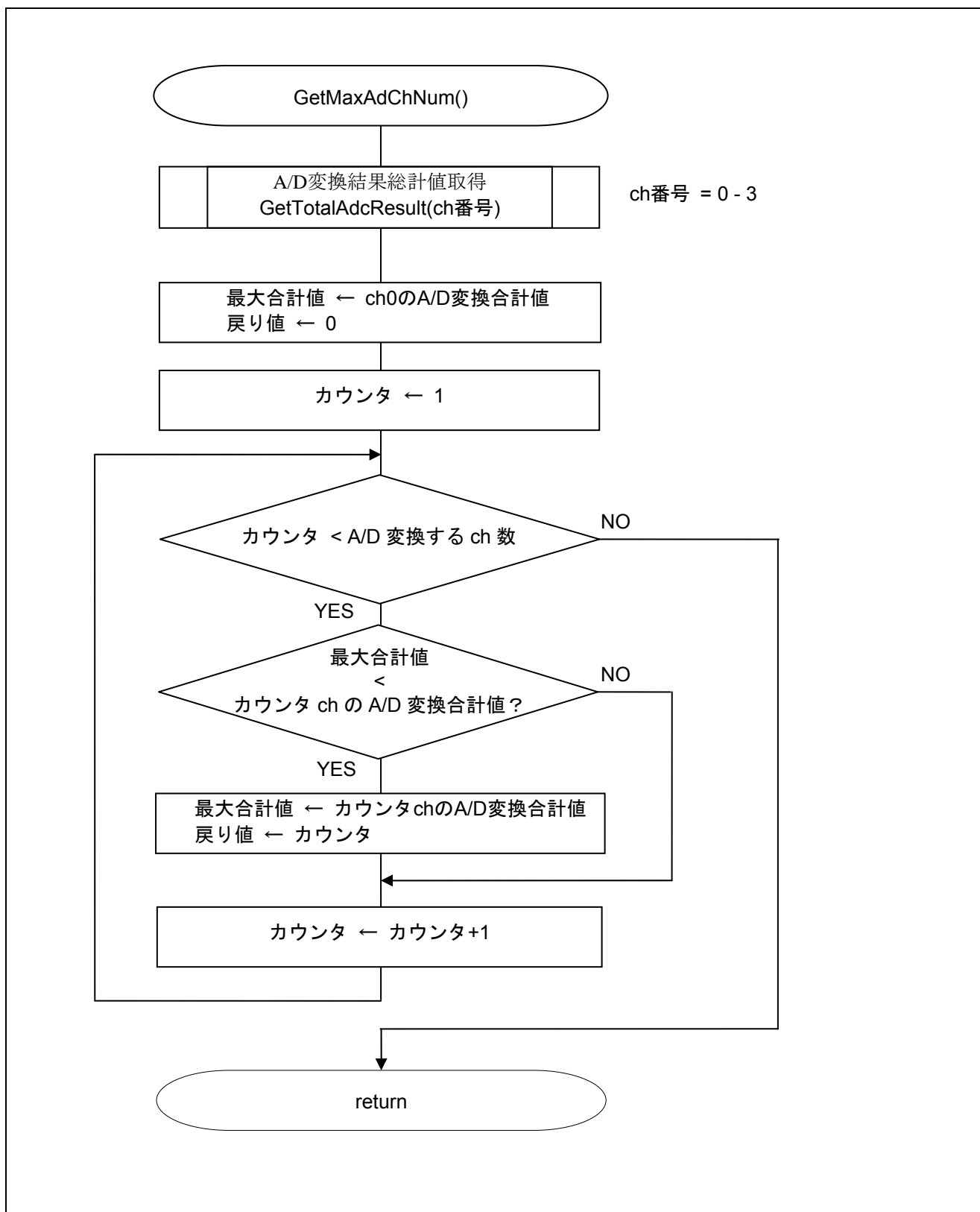
図 5.14 A/D 変換結果の合計値が最大となるチャンネル番号の取得処理
