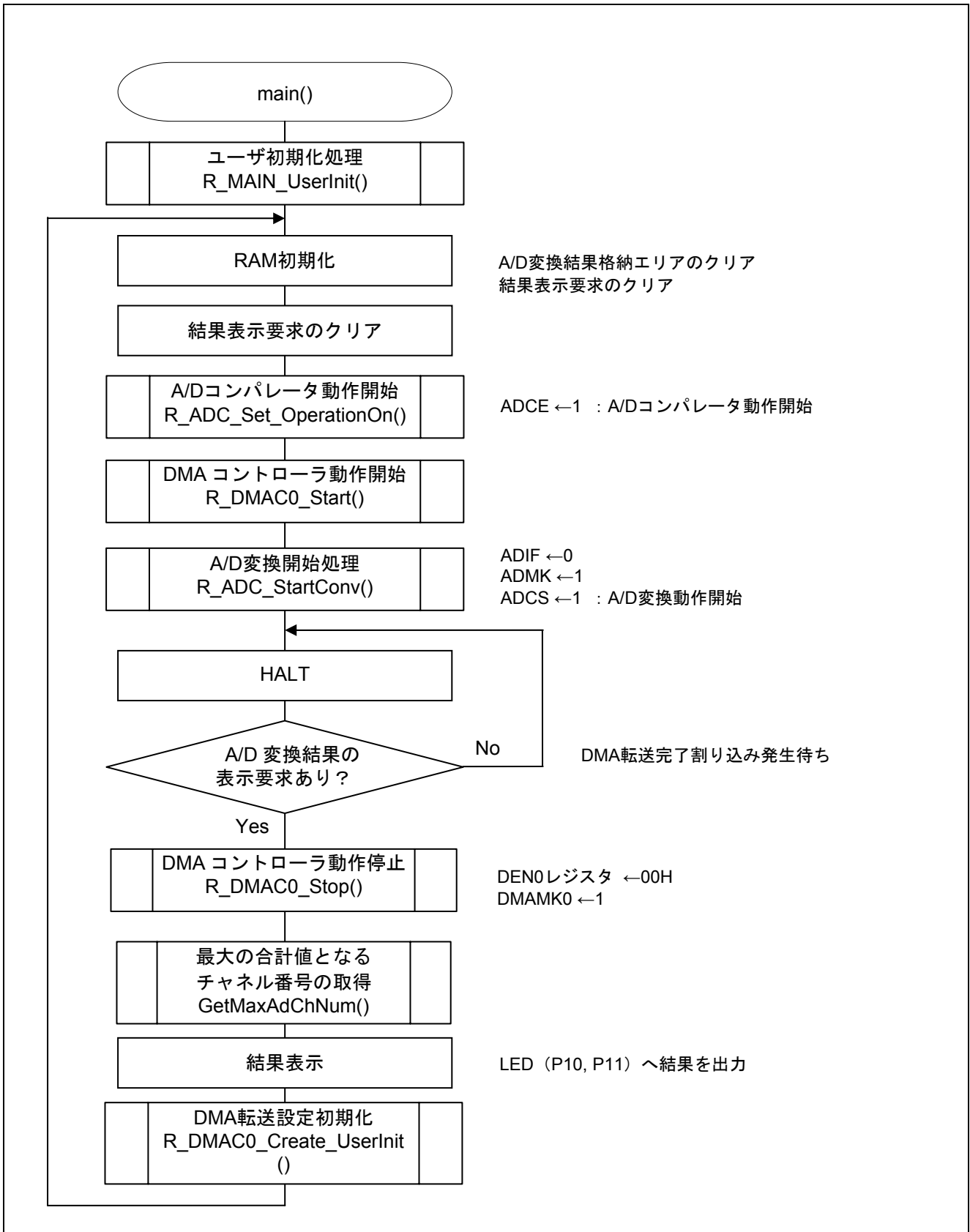
図 5.9 メイン処理
