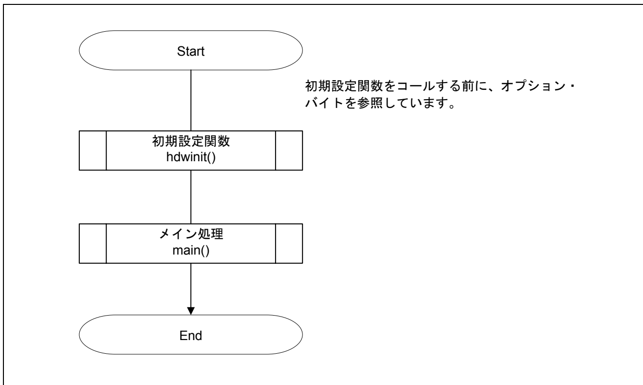
図 5.1 全体フロー
