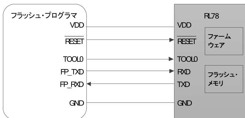
図1 - 3 2線UART通信図
