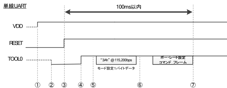
図1-4 フラッシュ・メモリ・プログラミング・モードへの遷移および通信方式の選択
