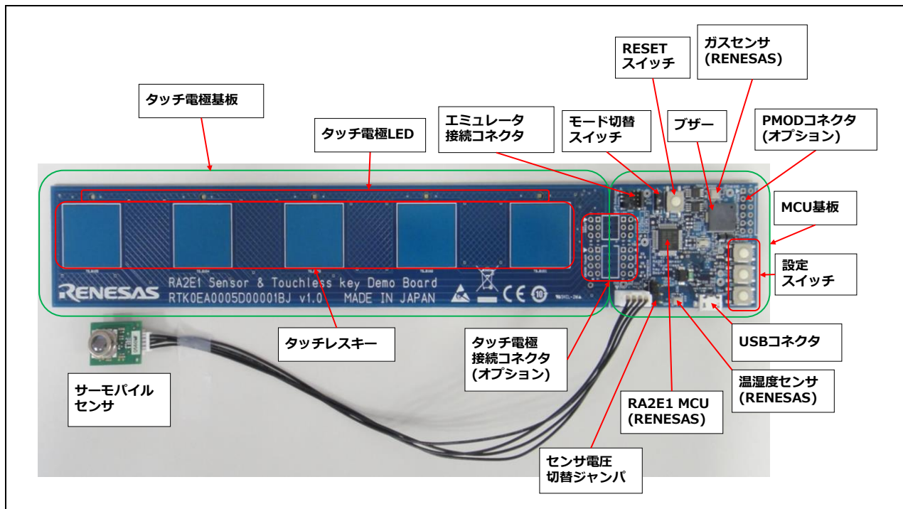
図 2-1 製品の外観
