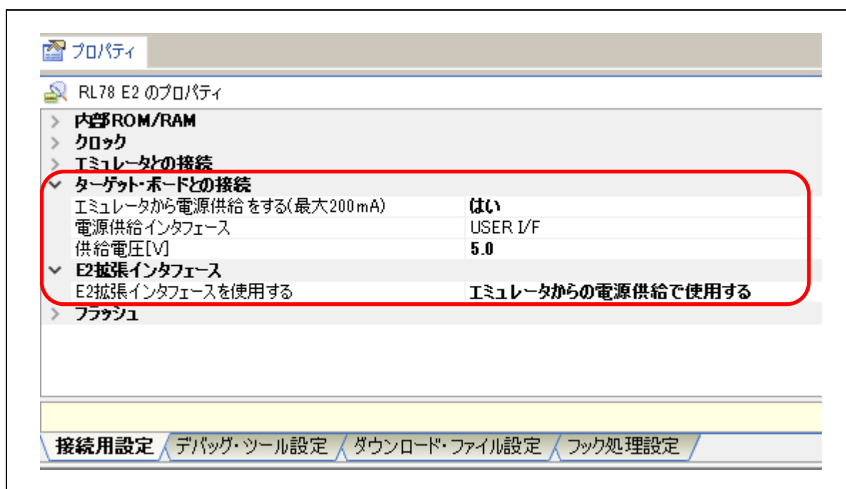
図 4-1 E2 エミュレータデバッガの接続設定
