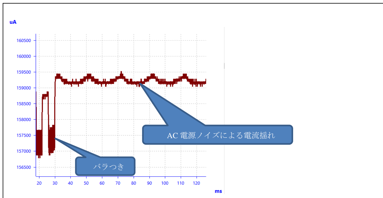
図 5-5 消費電流測定結果の特性
