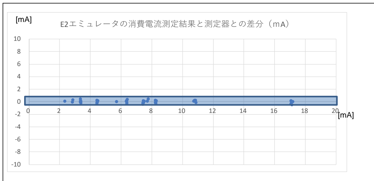
図 5-4 消費電流測定結果と測定器の差分 2
