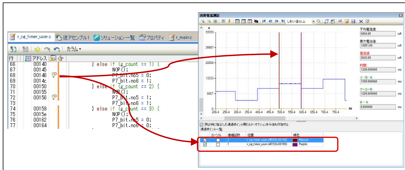
図 4-19 通過ポイントとプログラムの連携
