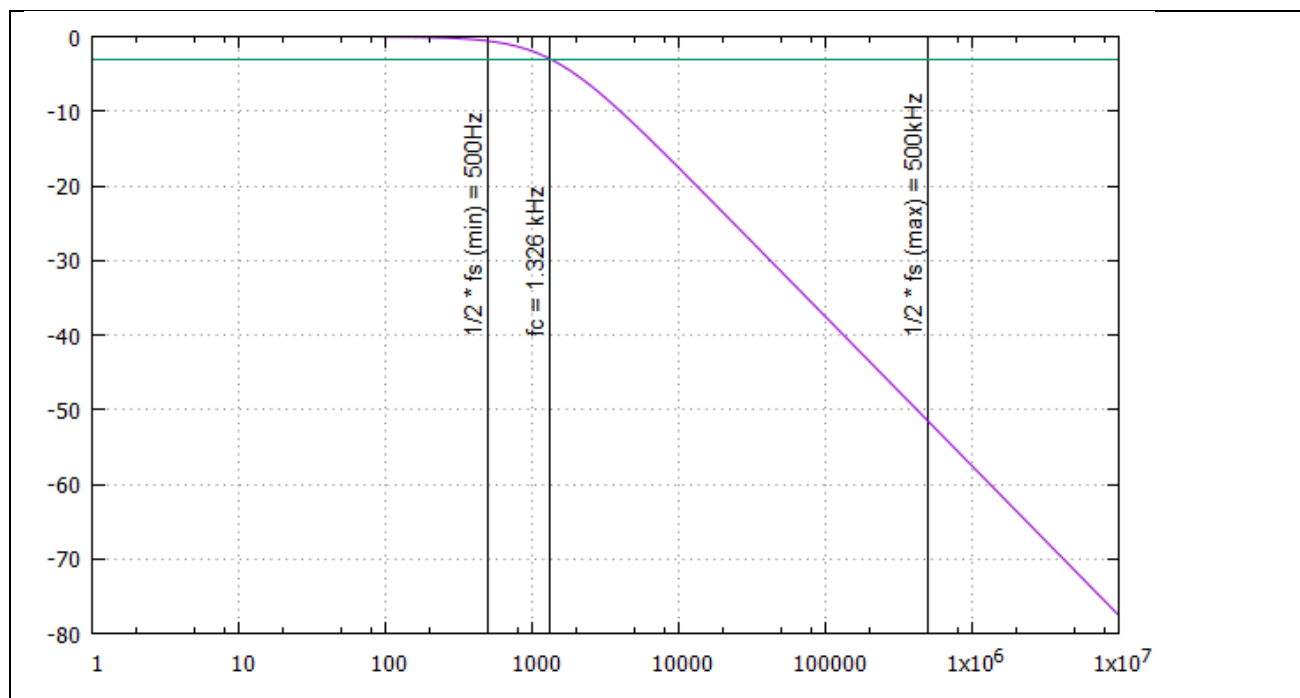
図 5-1 電流変化に対する応答特性
