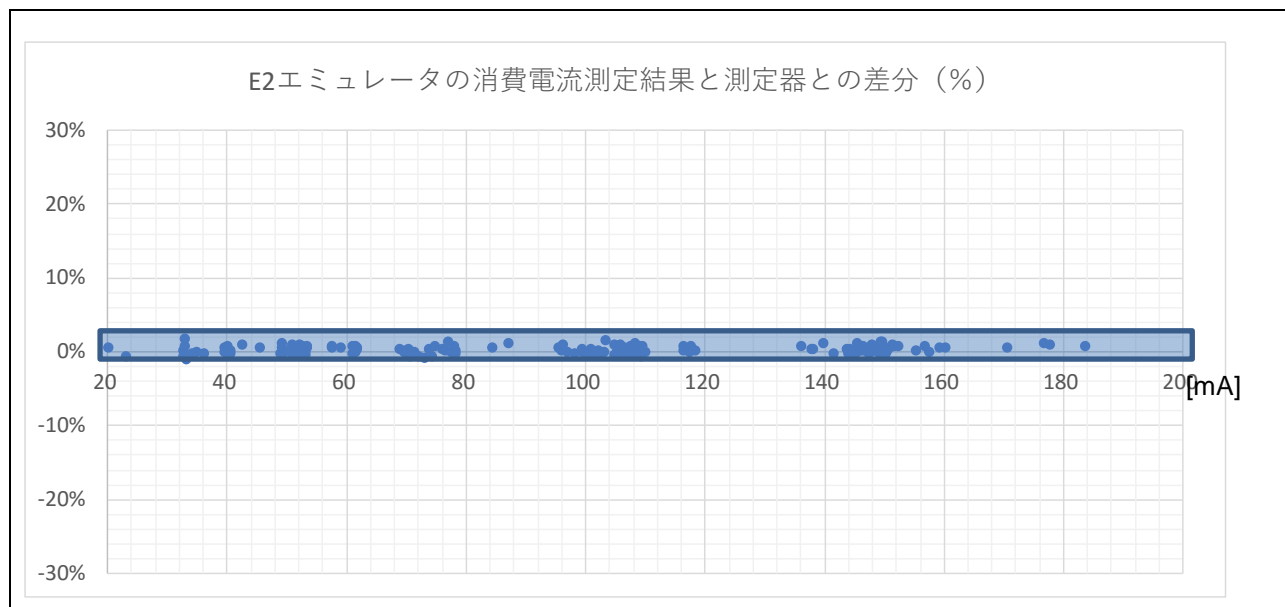
図 5-3 消費電流測定結果と測定器の差分 1
