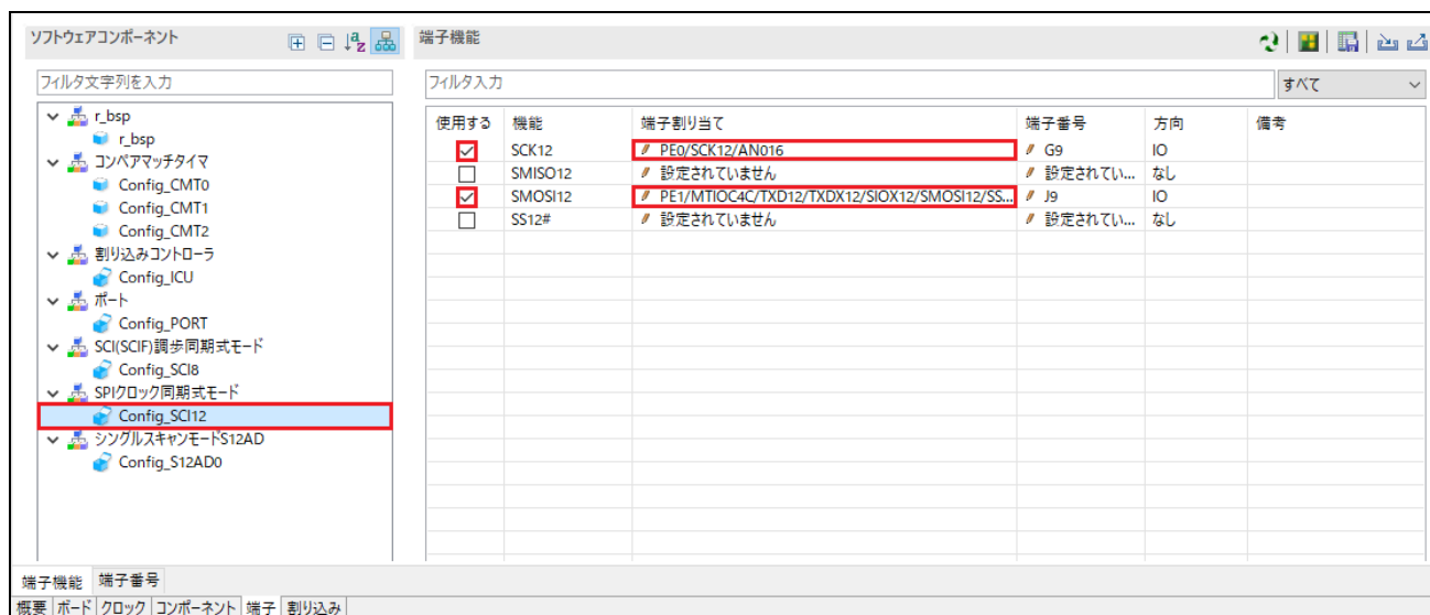
図 4-44 端子設定 - Config_SCI12
