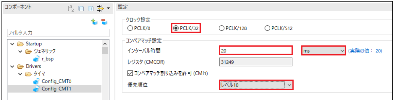
図 4-13 Config_CMT1 設定
