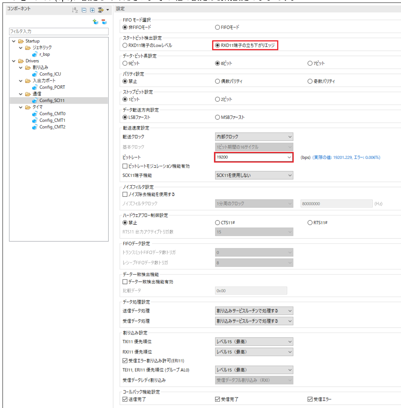
図 4-31 Config_SCI11 設定
