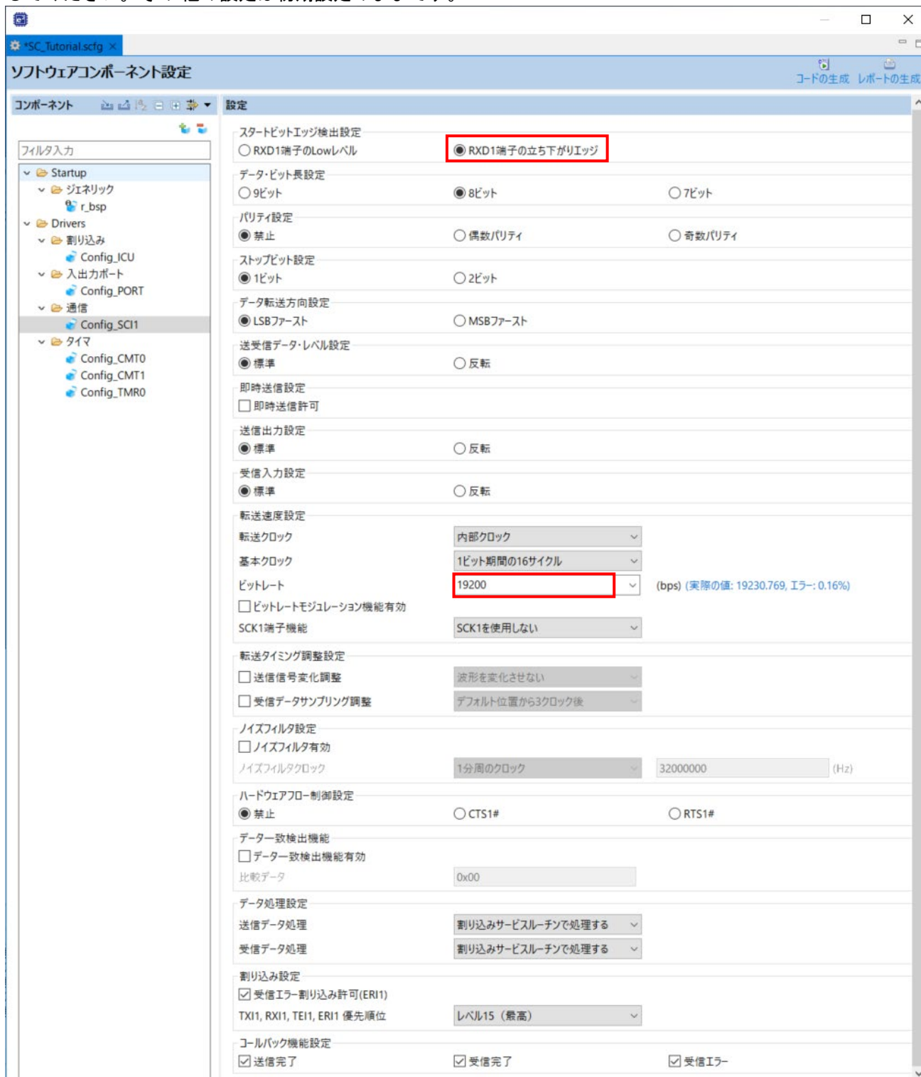
図 4-36 Config_SCI1 設定
