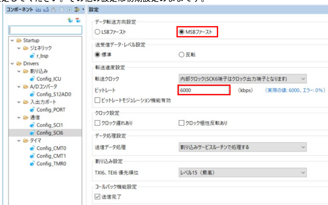
図 4-41 Config_SCI6 設定
