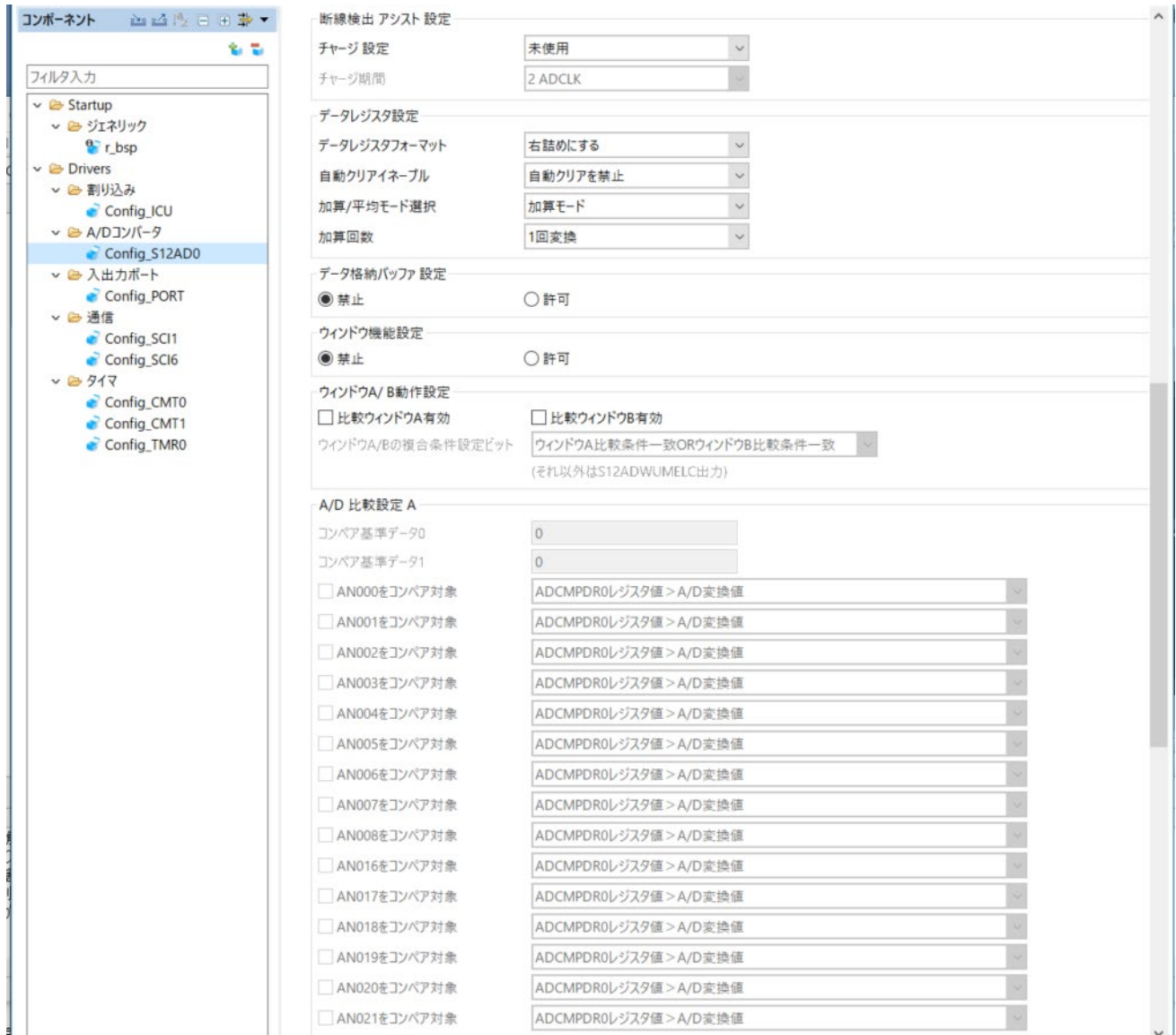
図 4-45 Config_S12AD0 設定(2)
