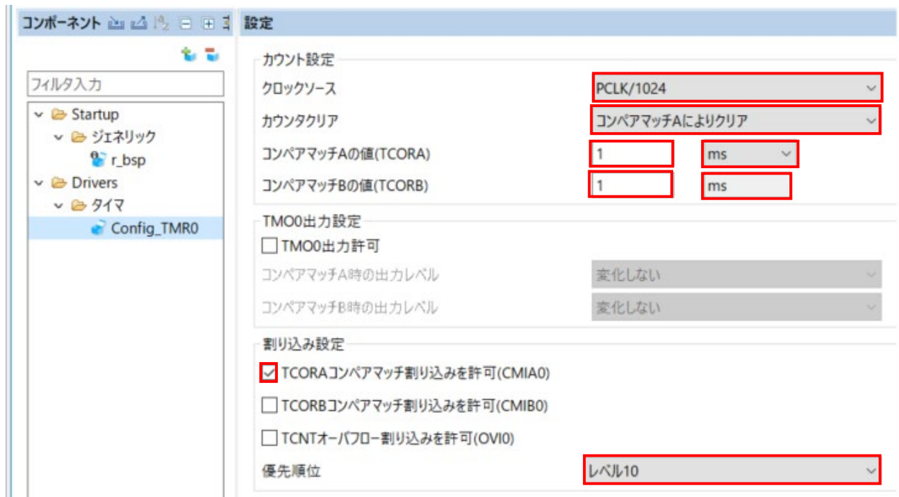
図 4-13 Config_TMR0 設定
