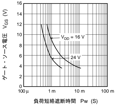
ゲート・ソース電圧対 負荷短絡遮断時間特性
