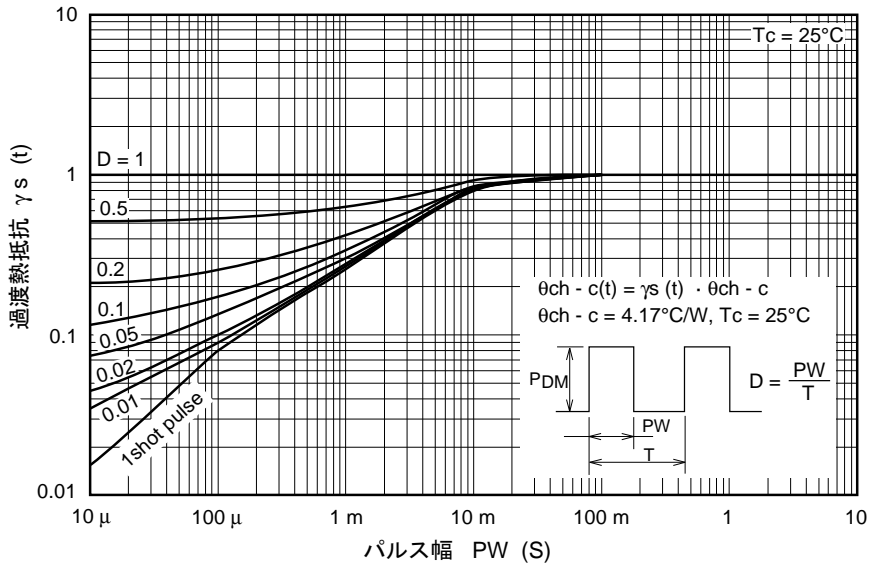
規格化過渡熱抵抗特性
