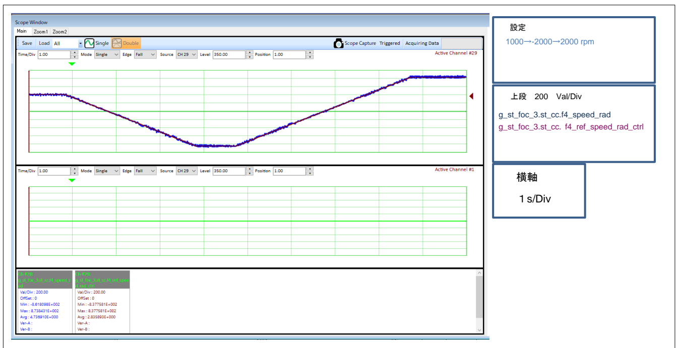
図 5-6 過渡時駆動波形 (2/2) (モータ 3)
