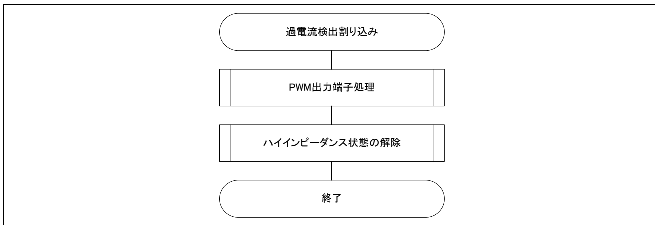
図 3-13 過電流検出割り込み処理フローチャート
