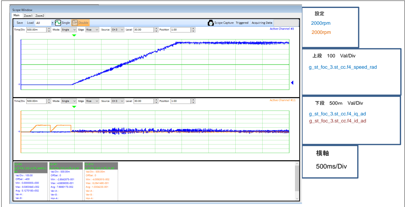
図 5-3 起動時駆動波形 (3/3) (モータ 3)
