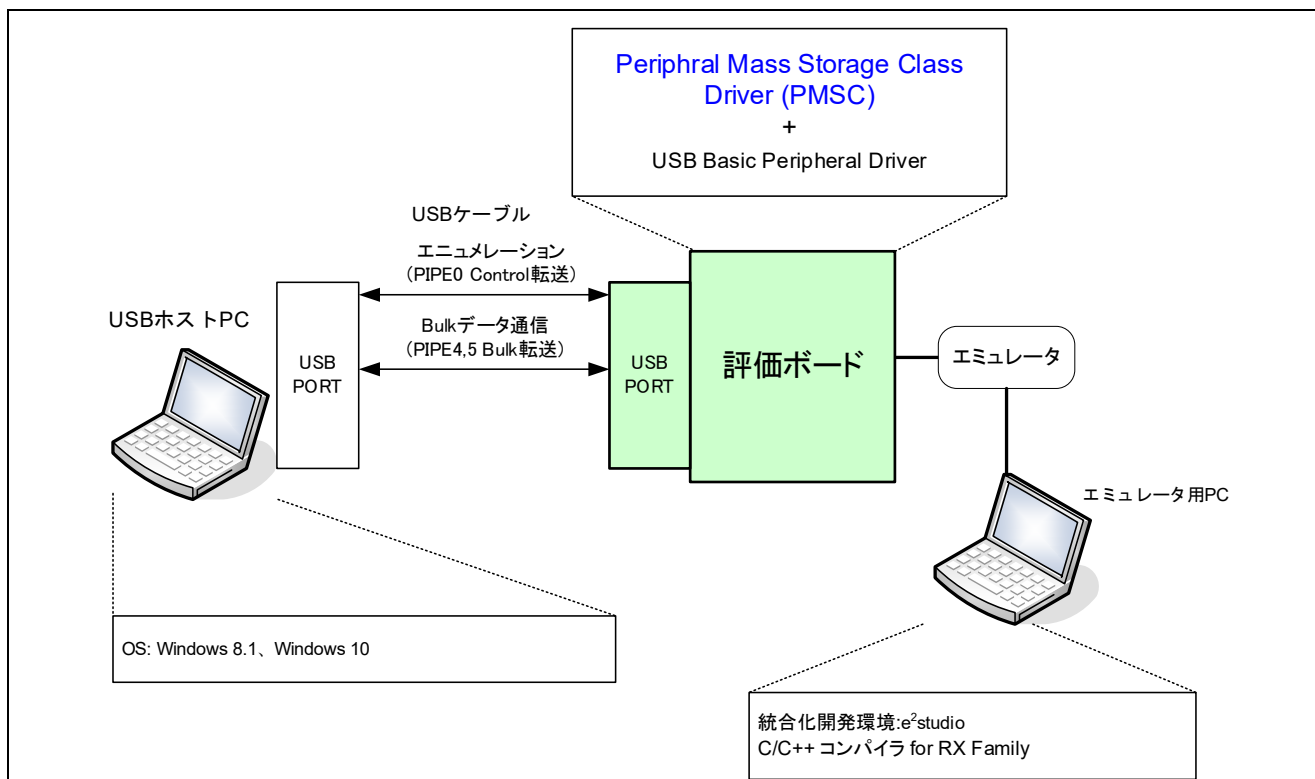
Figure 3-1 動作環境例
