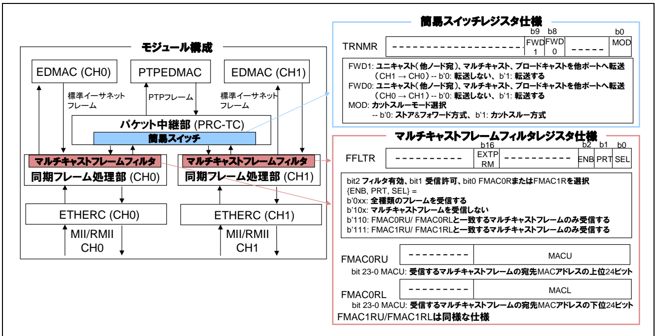
図 4.1 標準イーサネットの拡張機能
