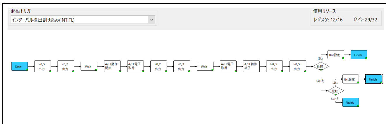
図 6-1 Config_SMS のフロー図
