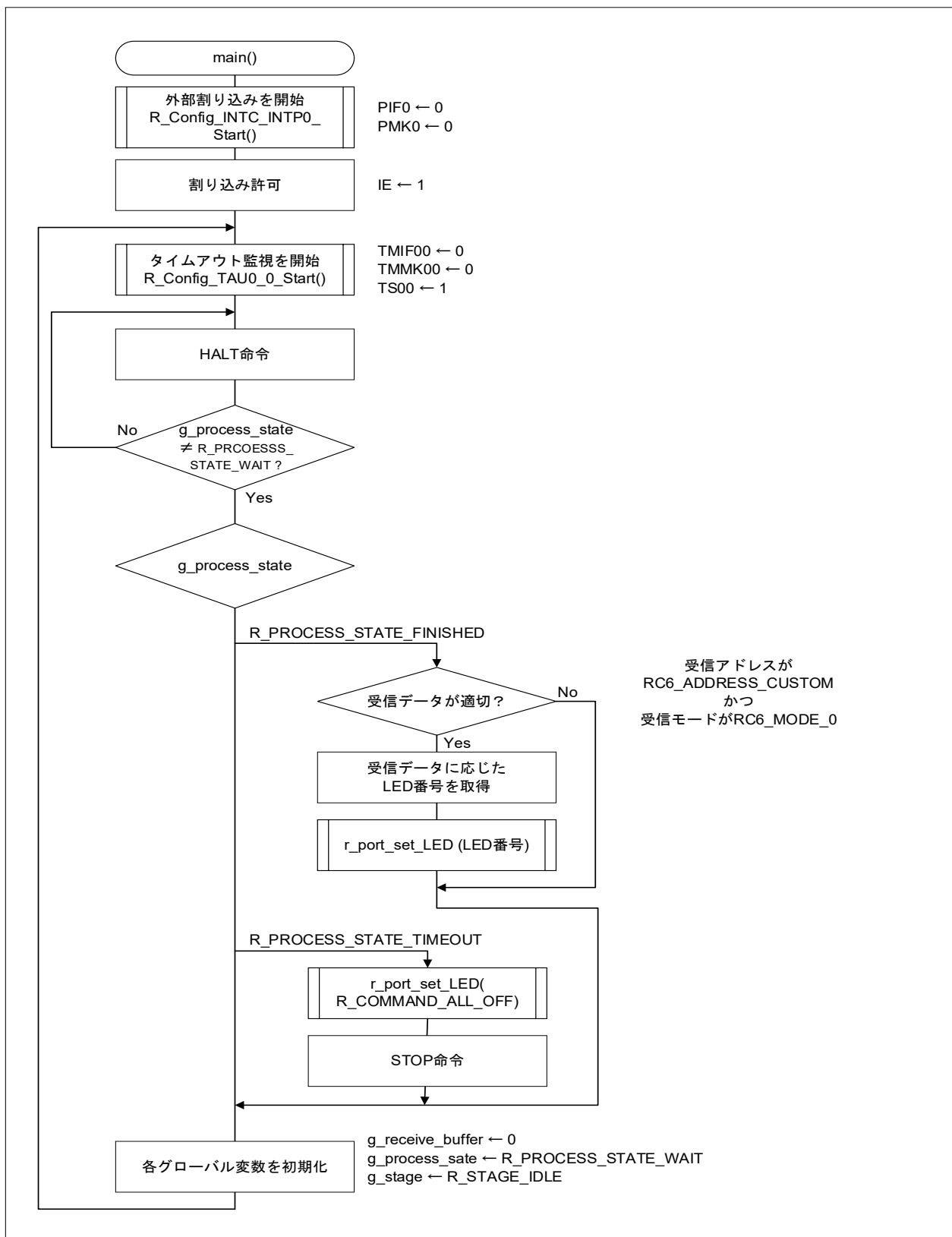
図 4-1 メイン処理
