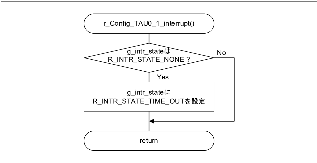
図 4-8 STOP モード移行用タイマ割り込み
