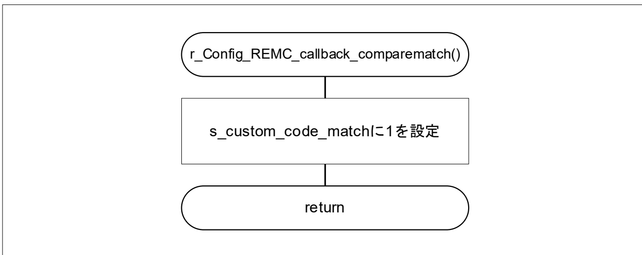
図 4-4 REMC コンペアー一致割り込み
