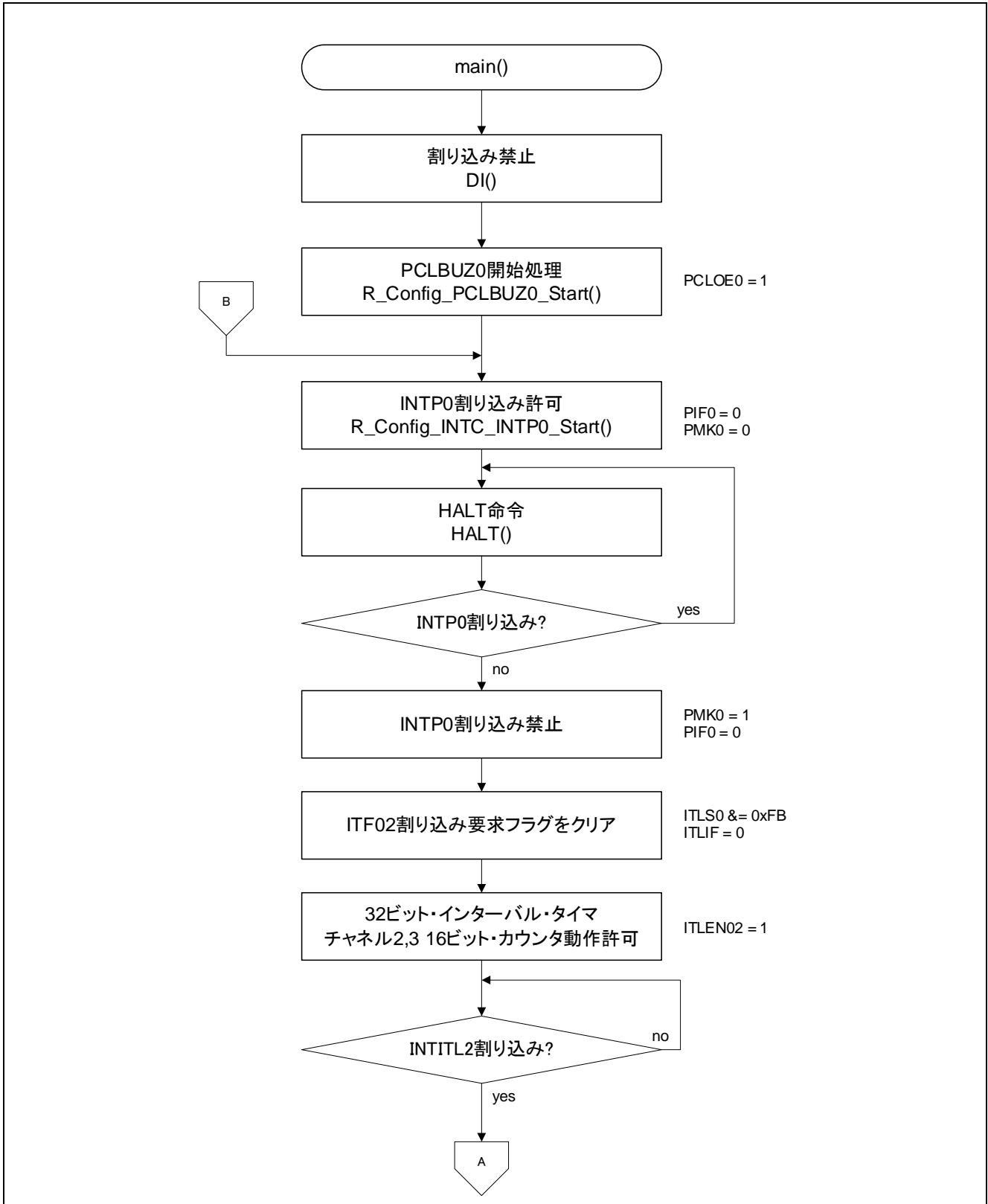
図 4-1 メイン処理 (1/2)
