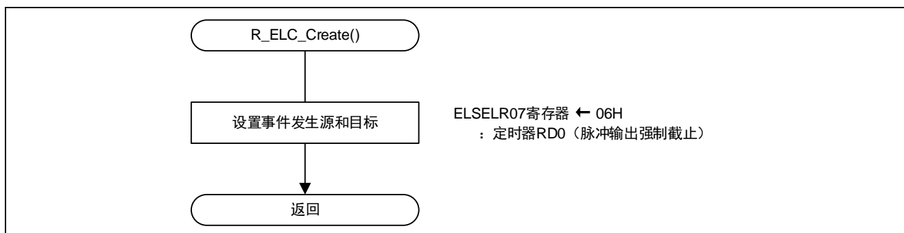
图 4.9 ELC 初始化设置
