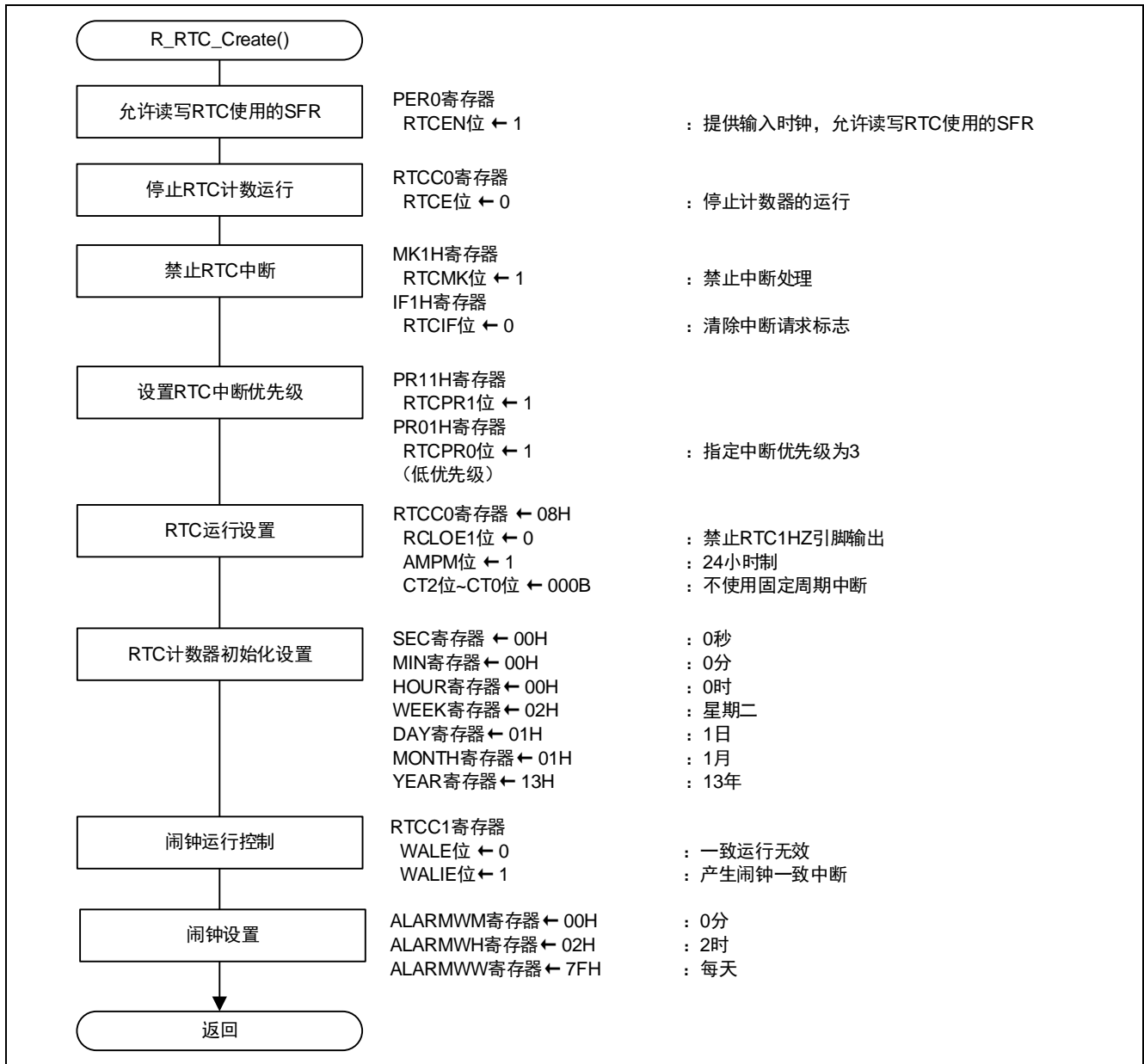
图 4.6 RTC 初始化设置
