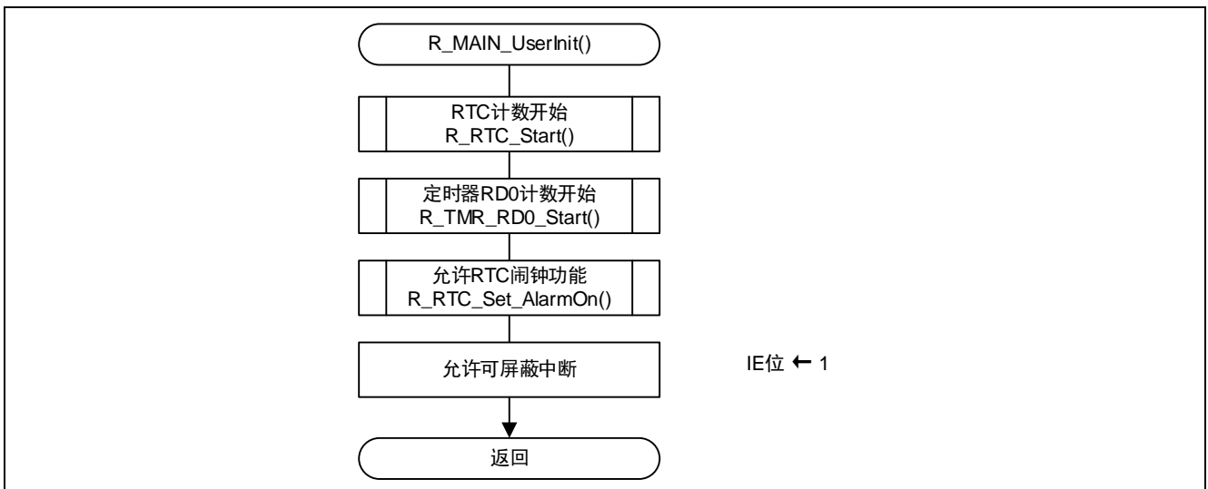
图 5.12 主函数初始化处理
