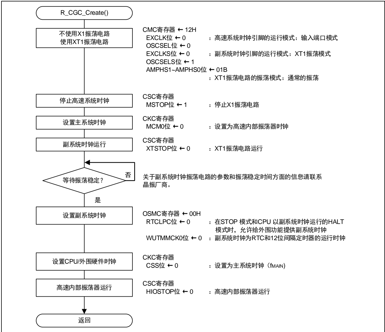
图 4.5 CPU 时钟设置
