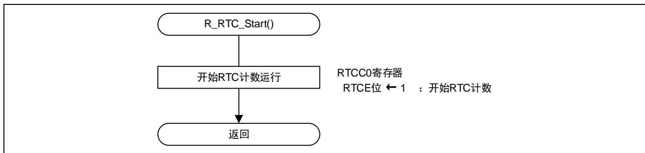
图 4.7 RTC 计时开始
