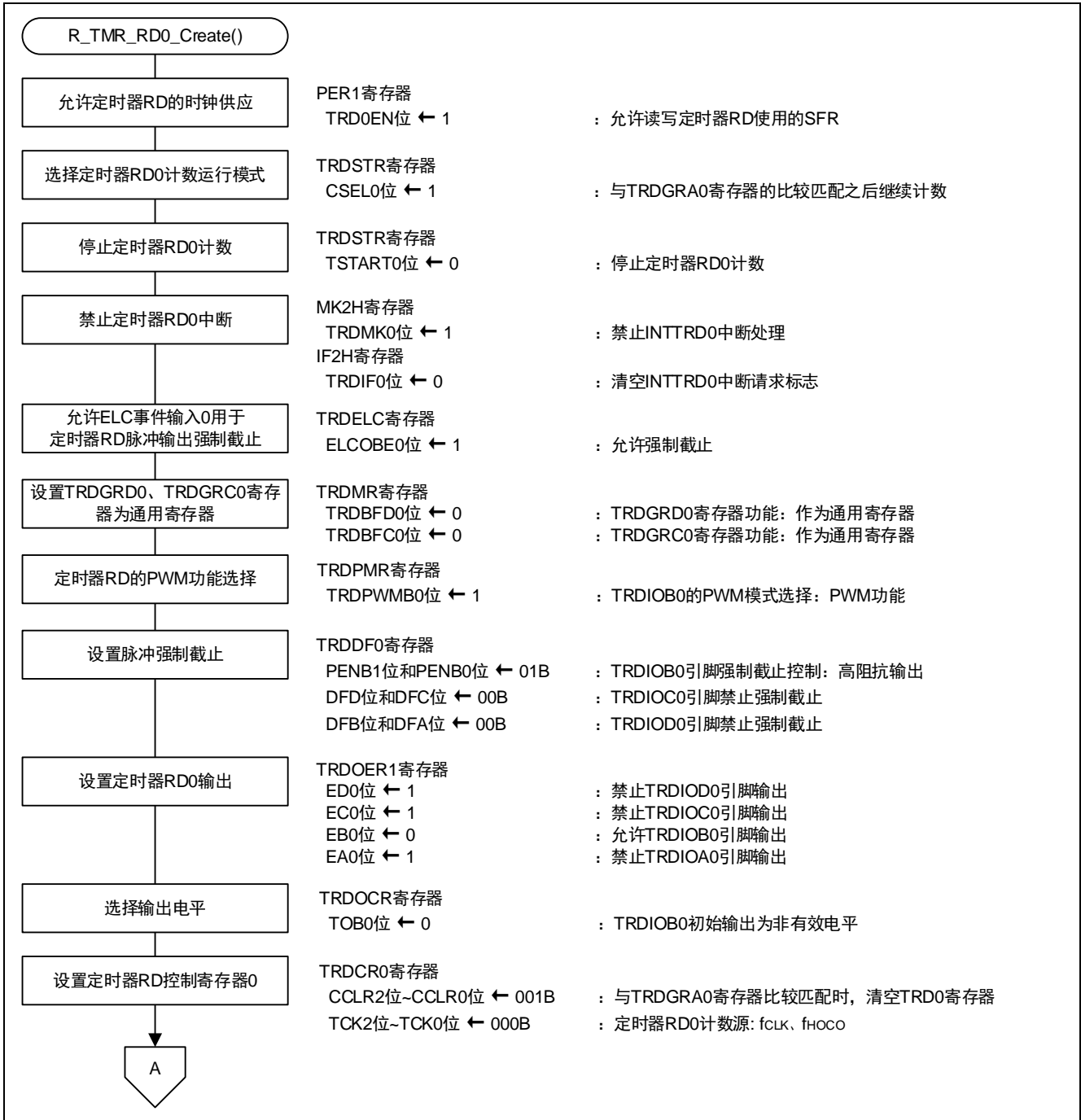
图 4.10 定时器 RD0 初始化设置 (1/2)
