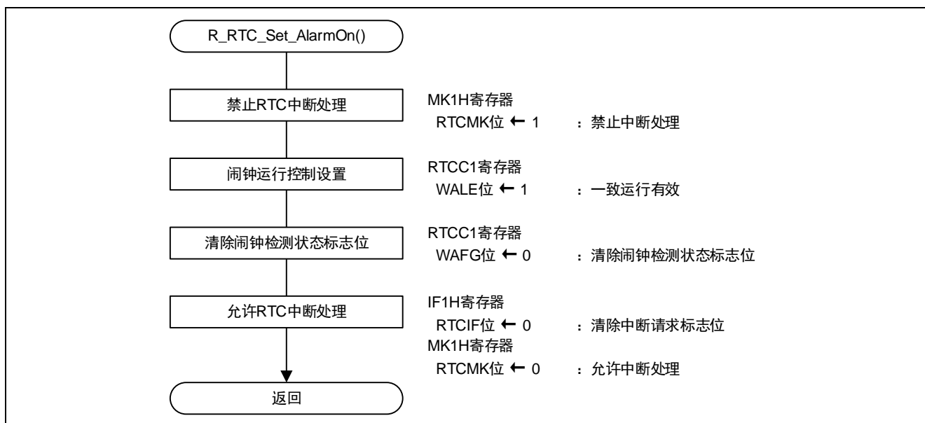
图 4.8 RTC 初始化设置
