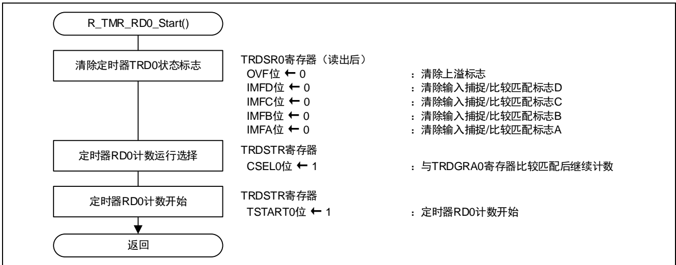
图 4.12 定时器 RD0 计数开始
