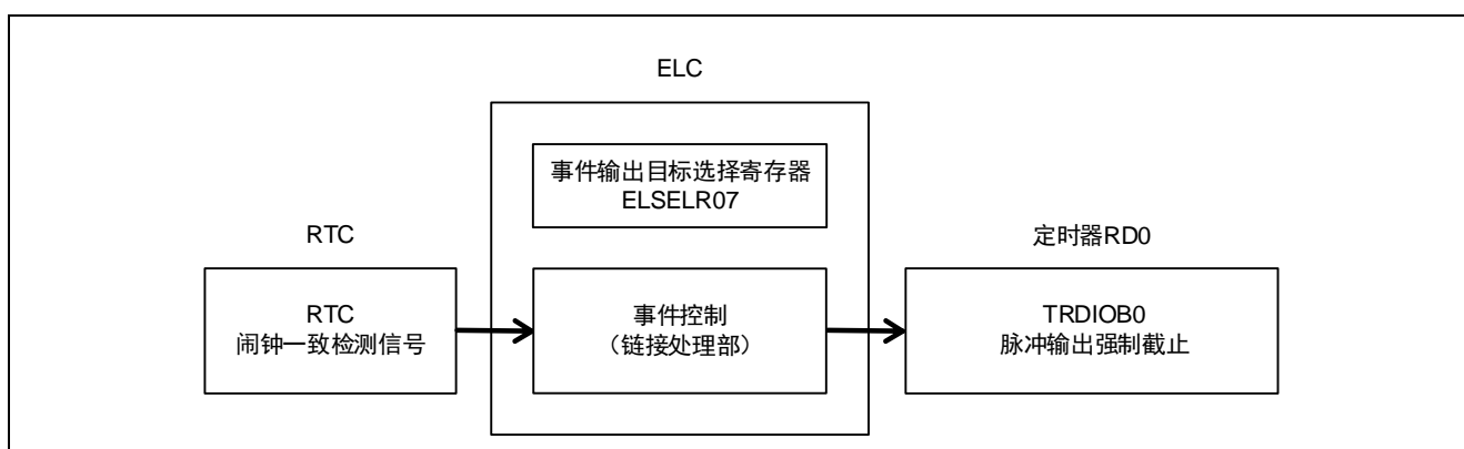
图 1.1 外围功能关系图
