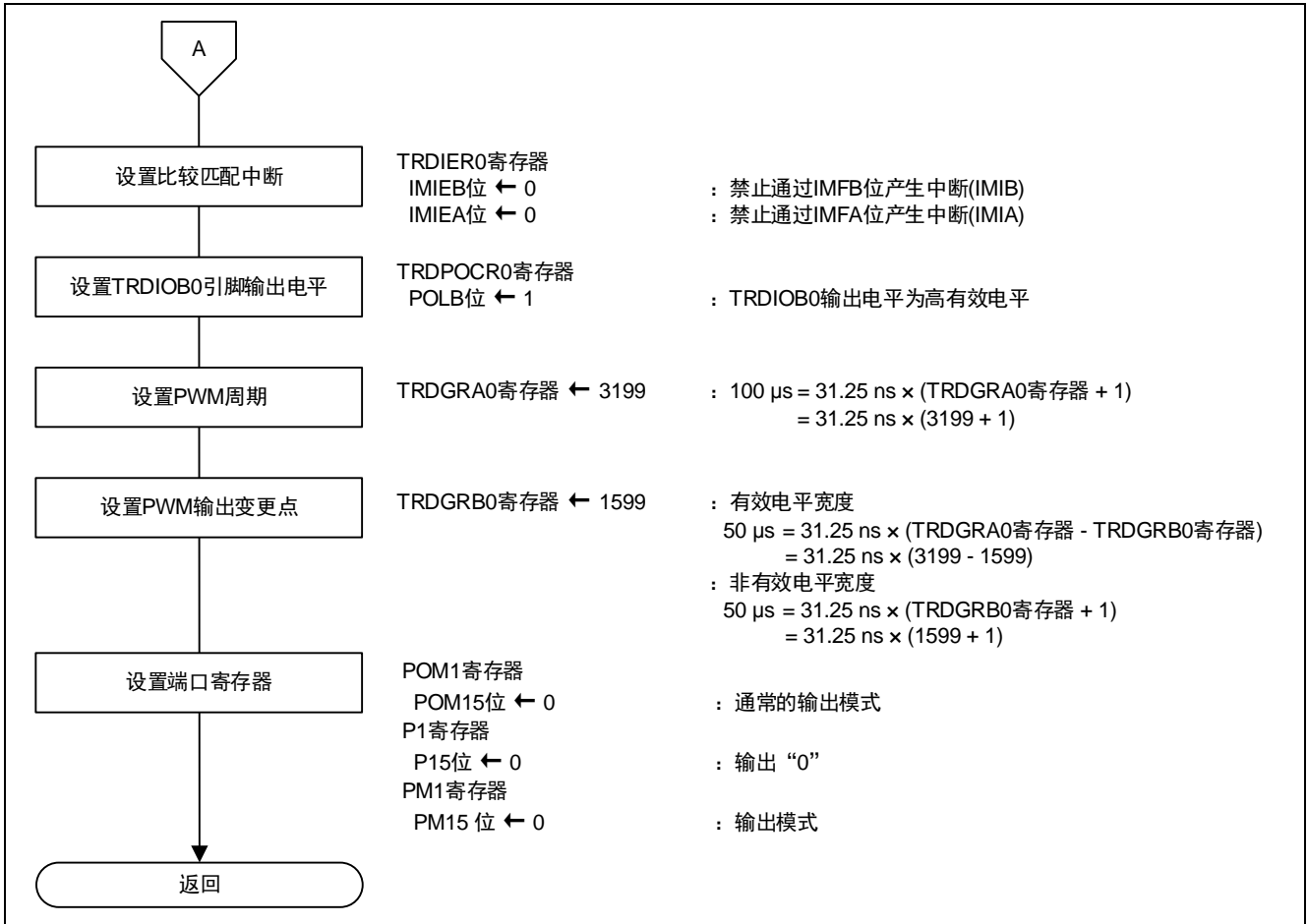
图 4.11 定时器 RD0 初始化设置 (2/2)
