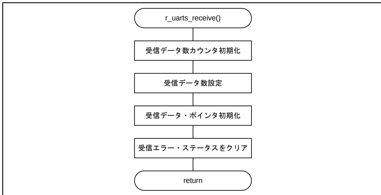
図 5.13 ソフトウェア UART 受信ステータス初期化関数
