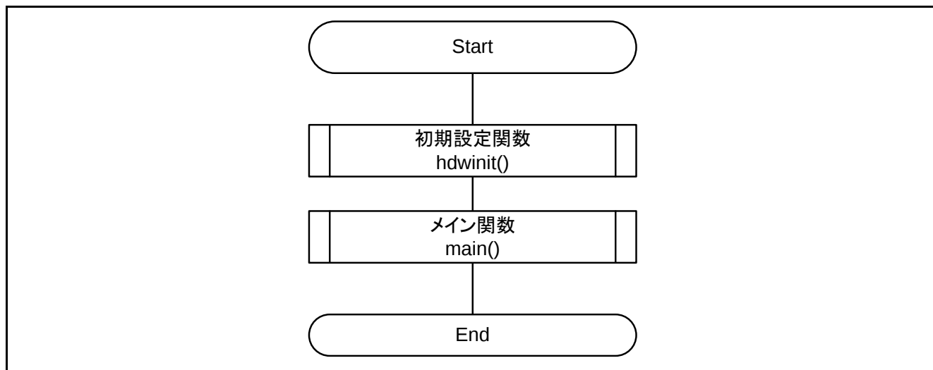
図 5.1 全体フロー
