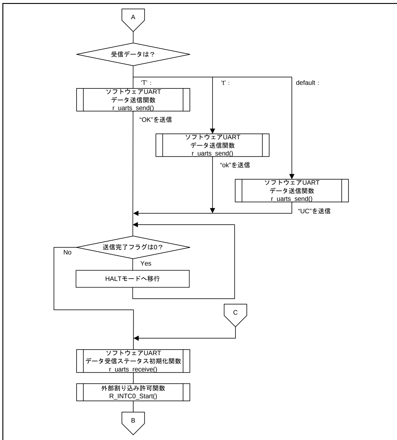
図 5.9 メイン関数 (2/2)
