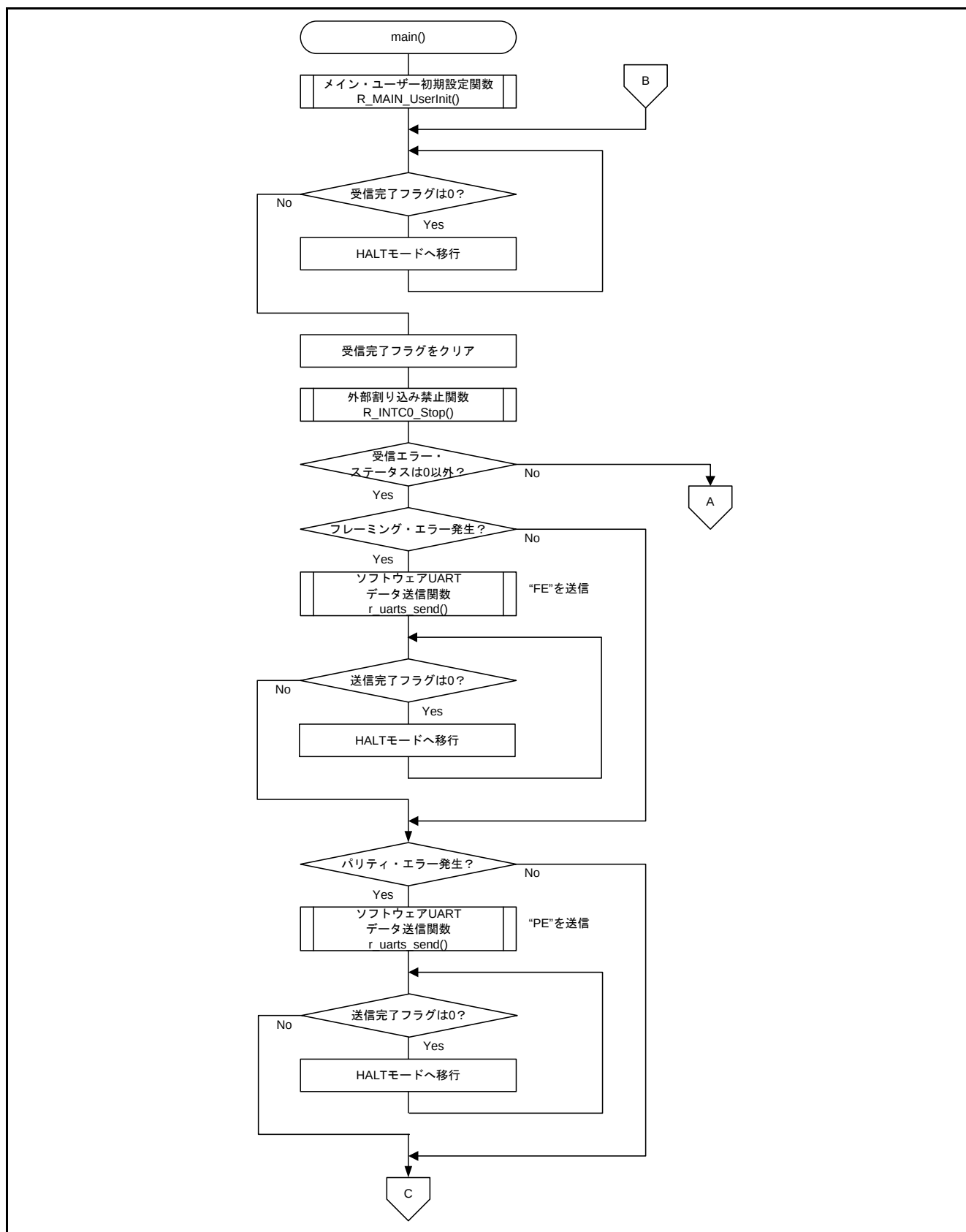
図 5.8 メイン関数 (1/2)
