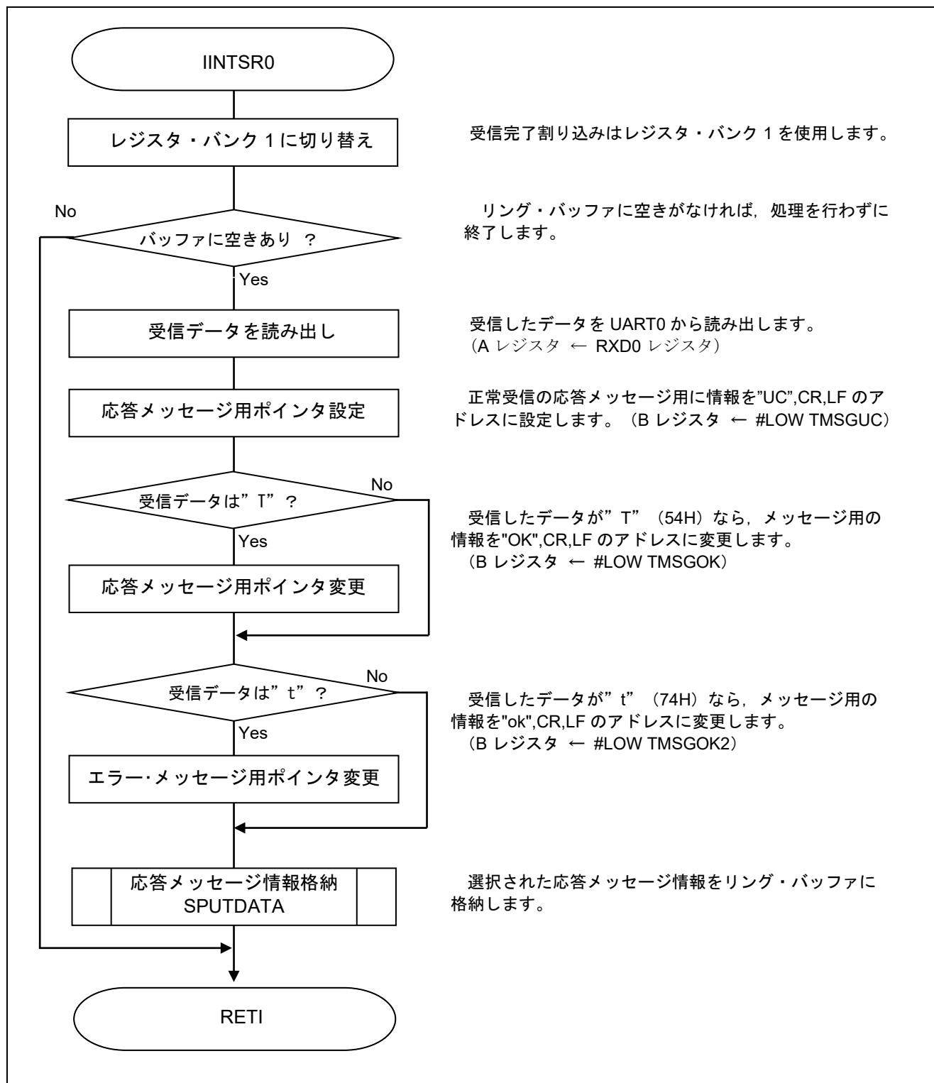
図 5.12 UART0 受信完了割り込み処理
