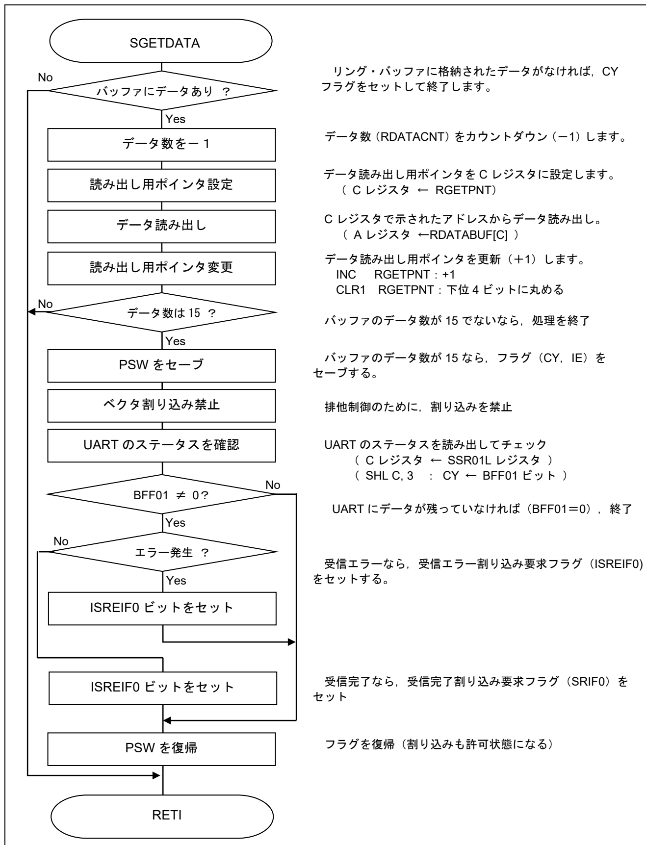
図 5.11 リング・バッファ読み出し処理
