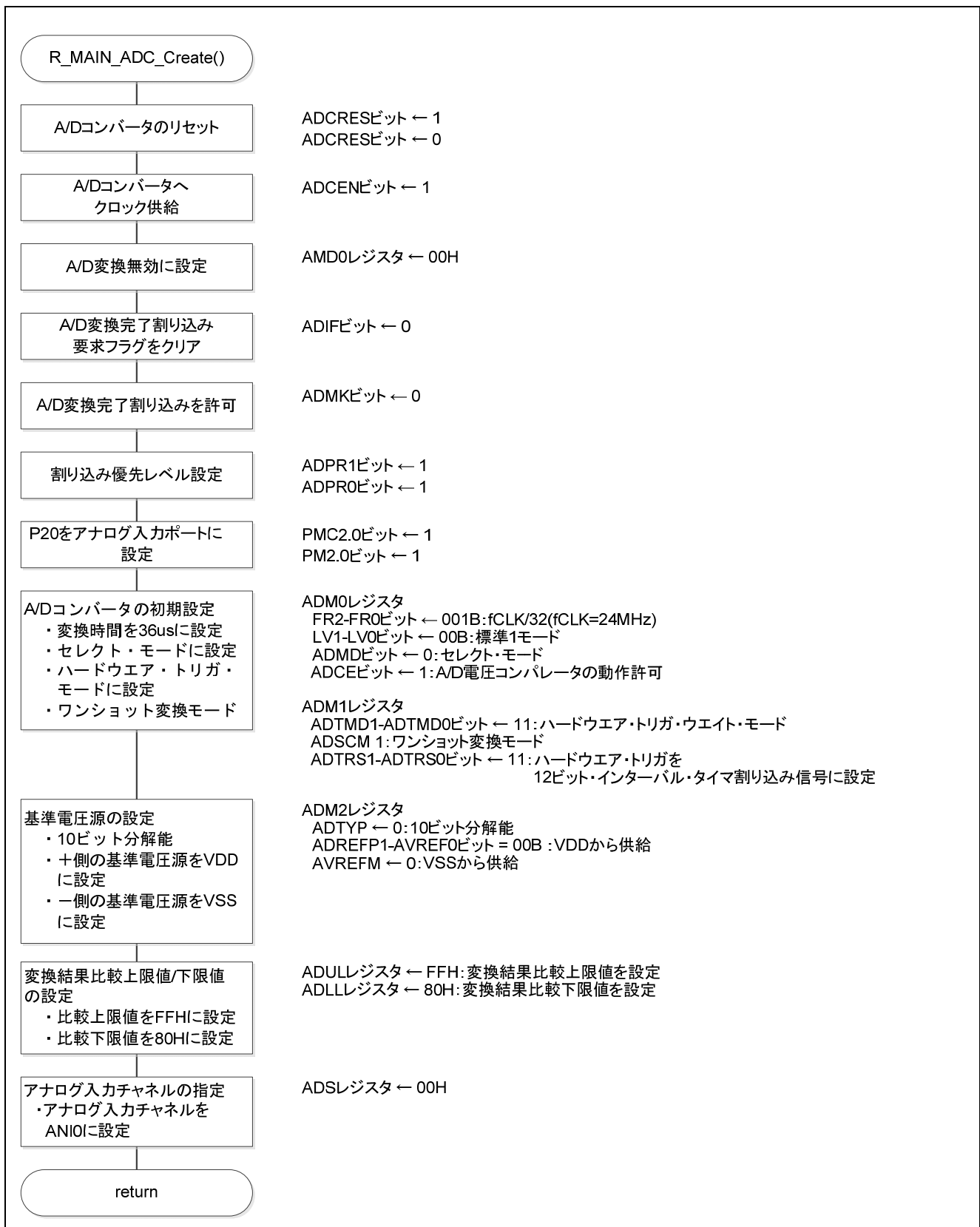
図 5.29 A/D コンバータ初期設定
