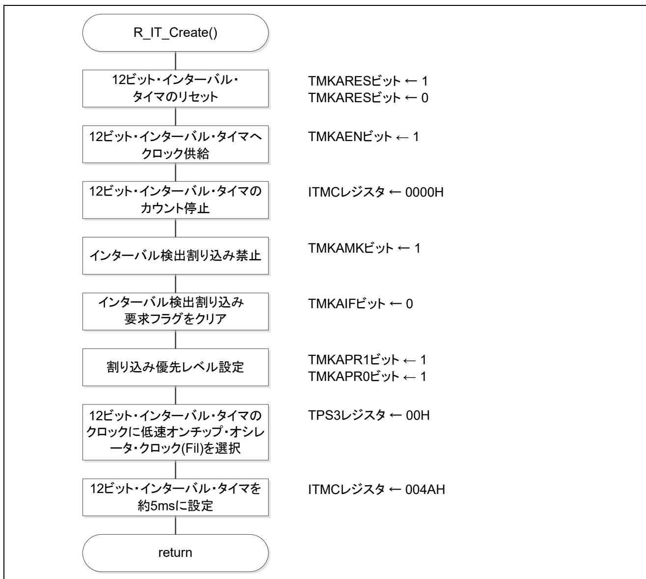
図 5.7 12 ビット・インターバル・タイマの設定
