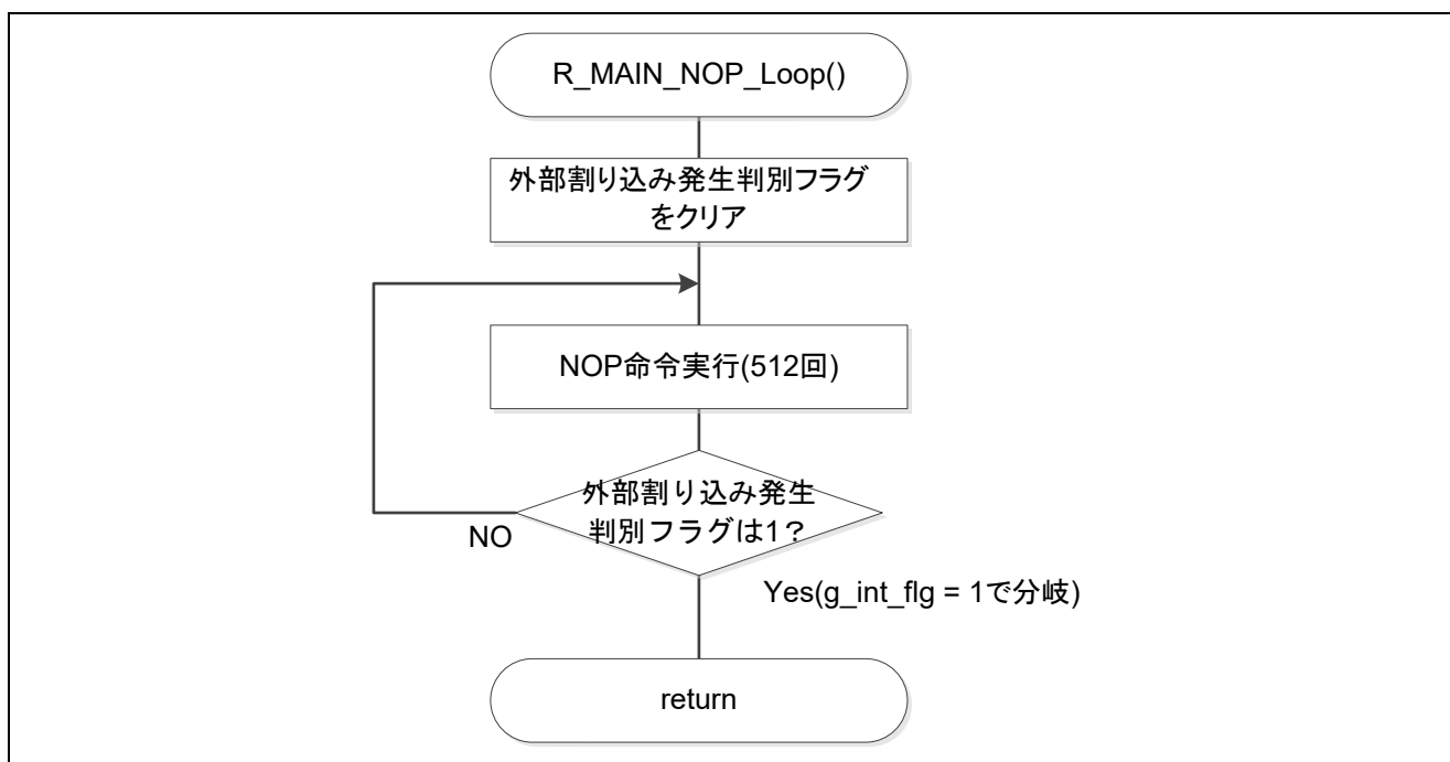
図 5.13 CPU 動作(NOP 命令実行)
