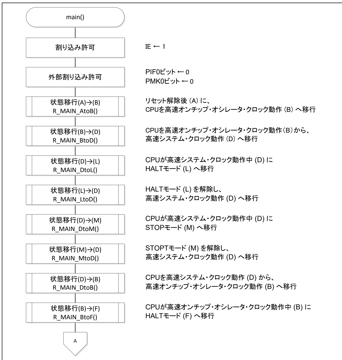
図 5.8 メイン処理(1/4)
