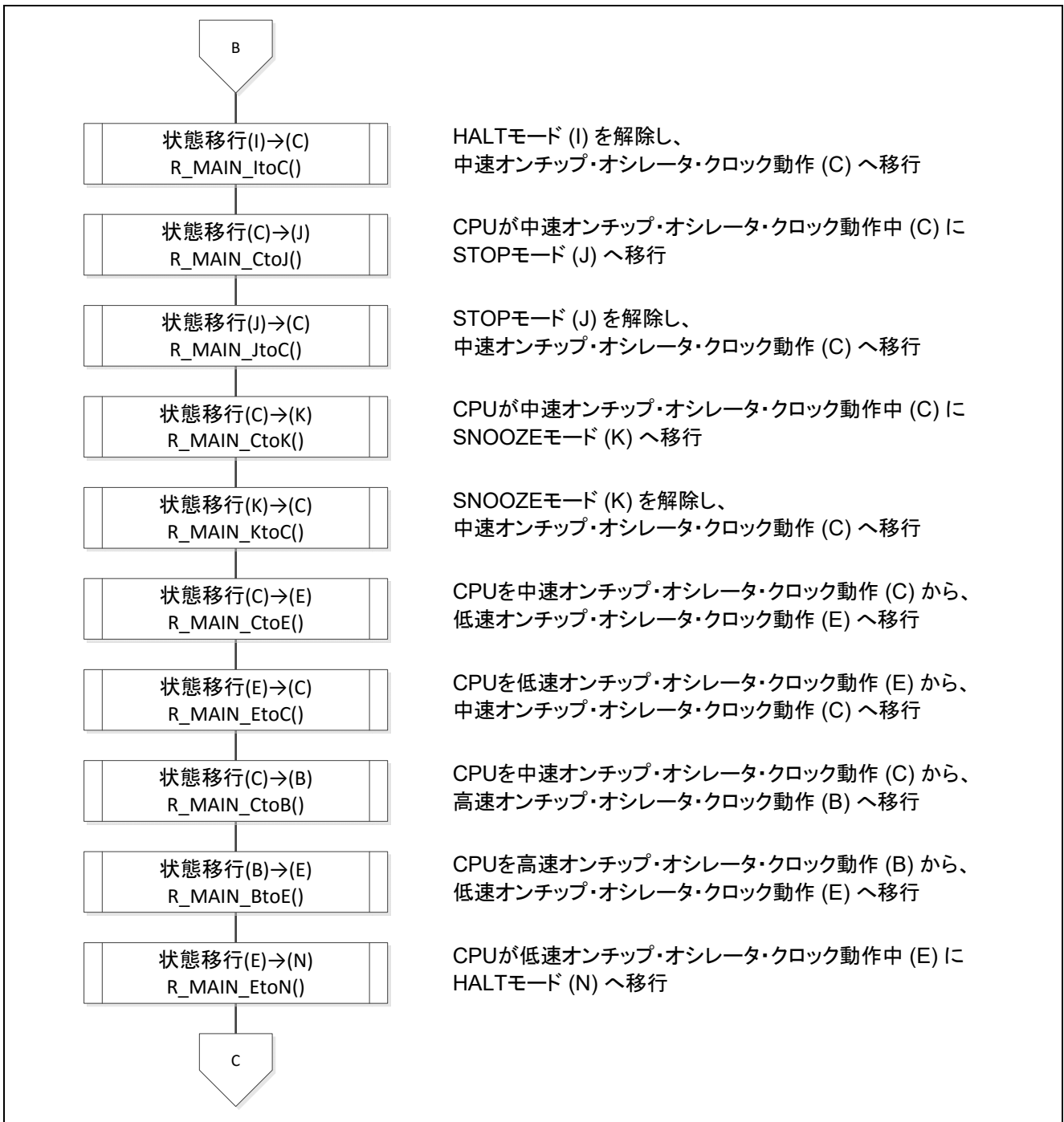
図 5.10 メイン処理(3/4)
