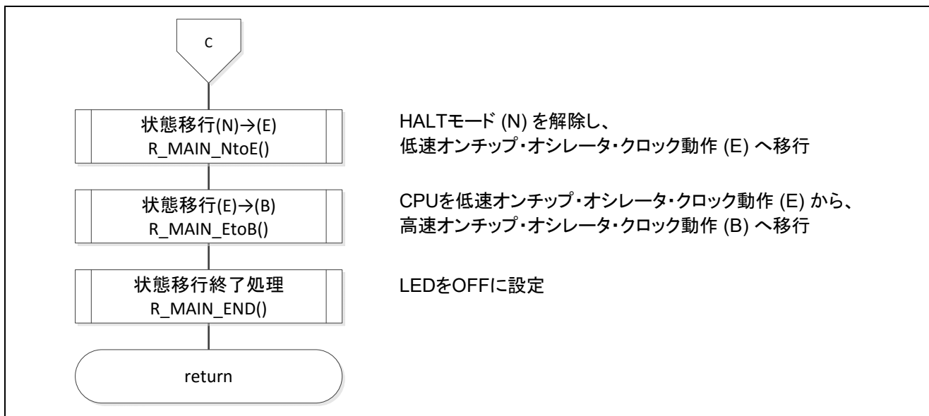
図 5.11 メイン処理(4/4)
