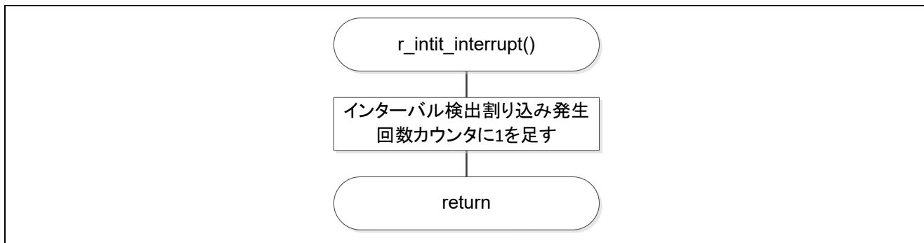
図 5.61 12 ビット・インターバル・タイマ割り込み処理
