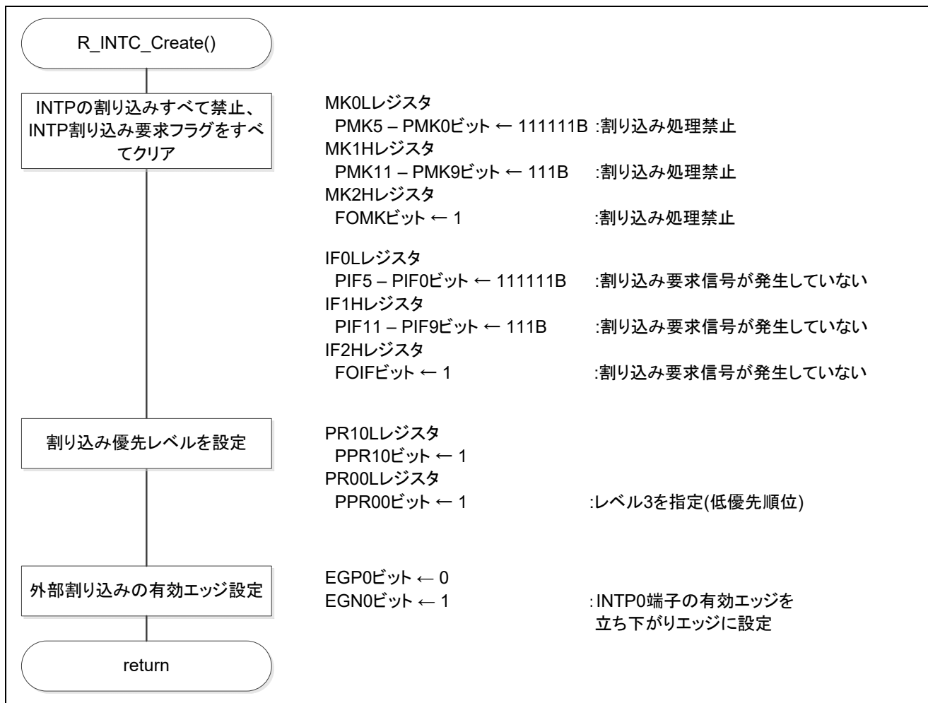
図 5.6 外部割り込みの設定
