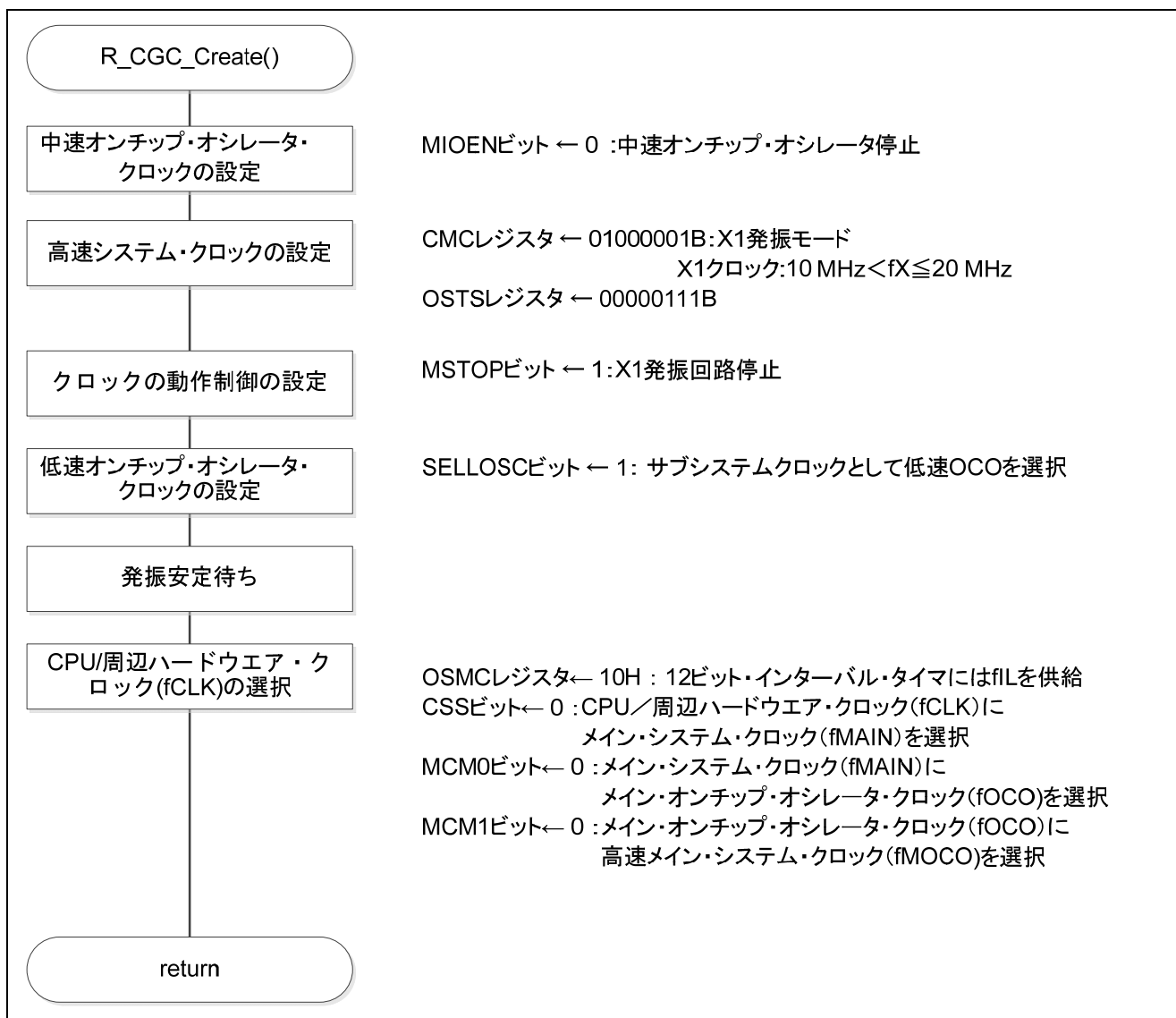
図 5.5 クロック発生回路の設定
