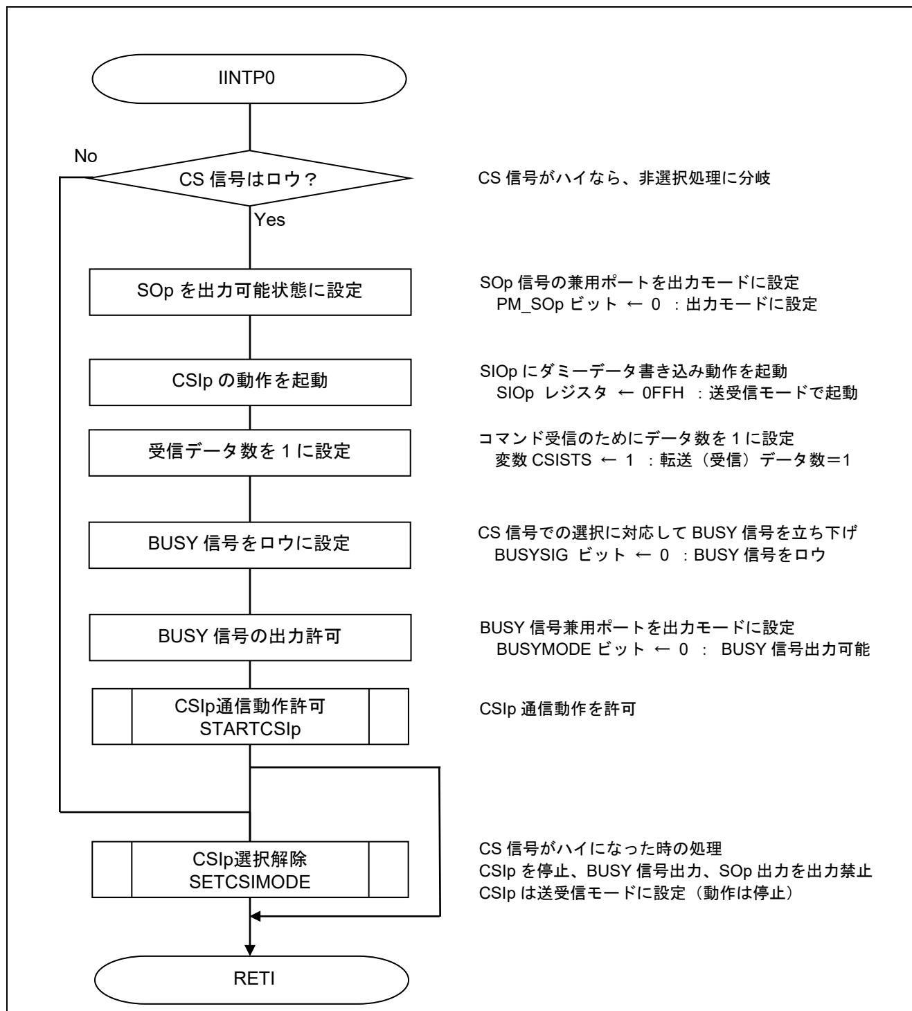
図 5.15 INTP0 割り込み処理関数
