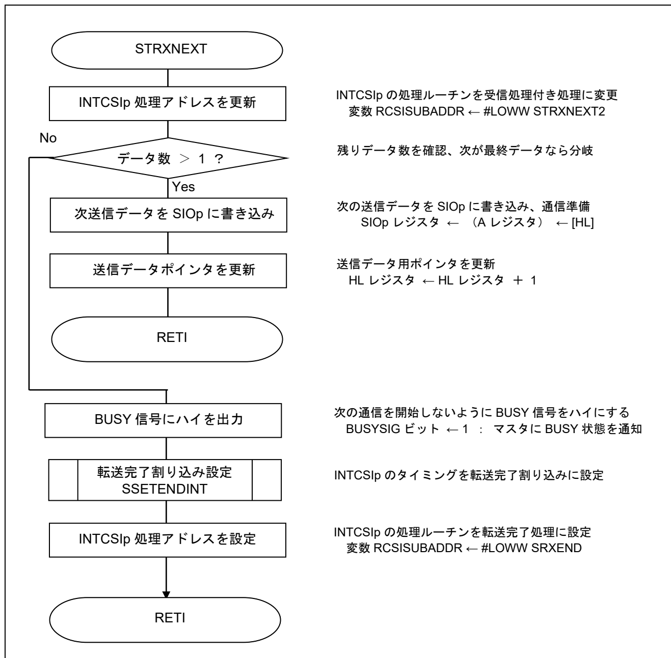
図 5.23 連続送受信時通信開始割り込み処理
