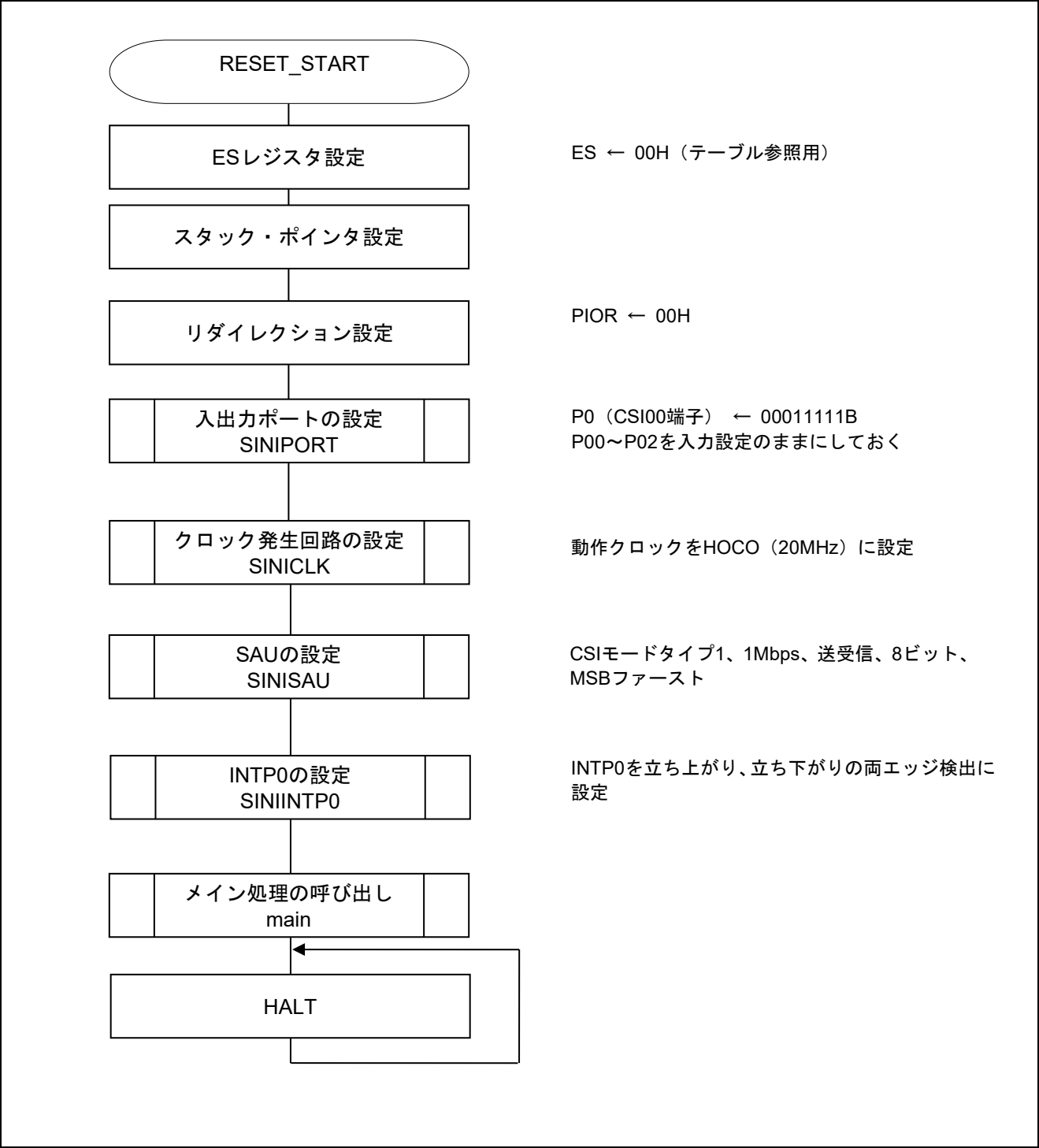
図 5.2 CPU 初期化関数
