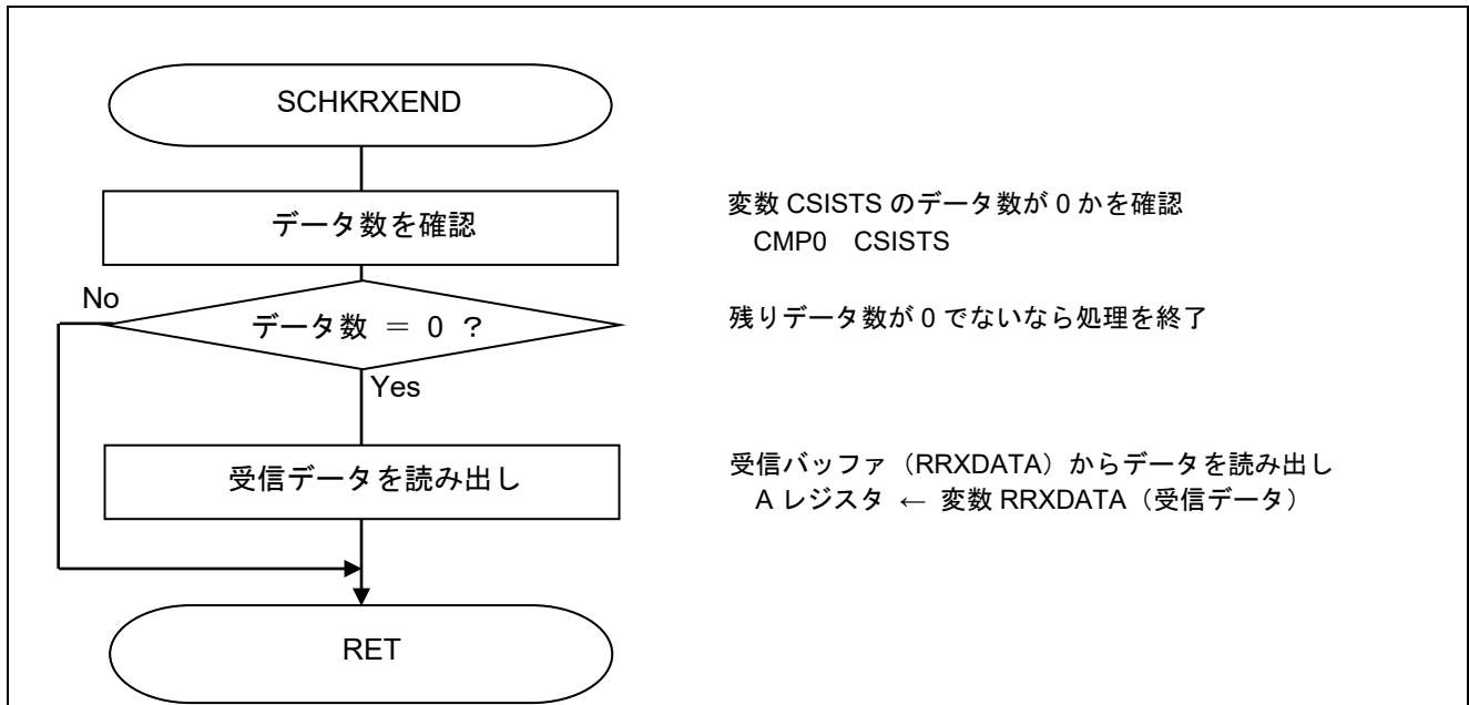
図 5.25 1 キャラクタの転送状態チェック関数
