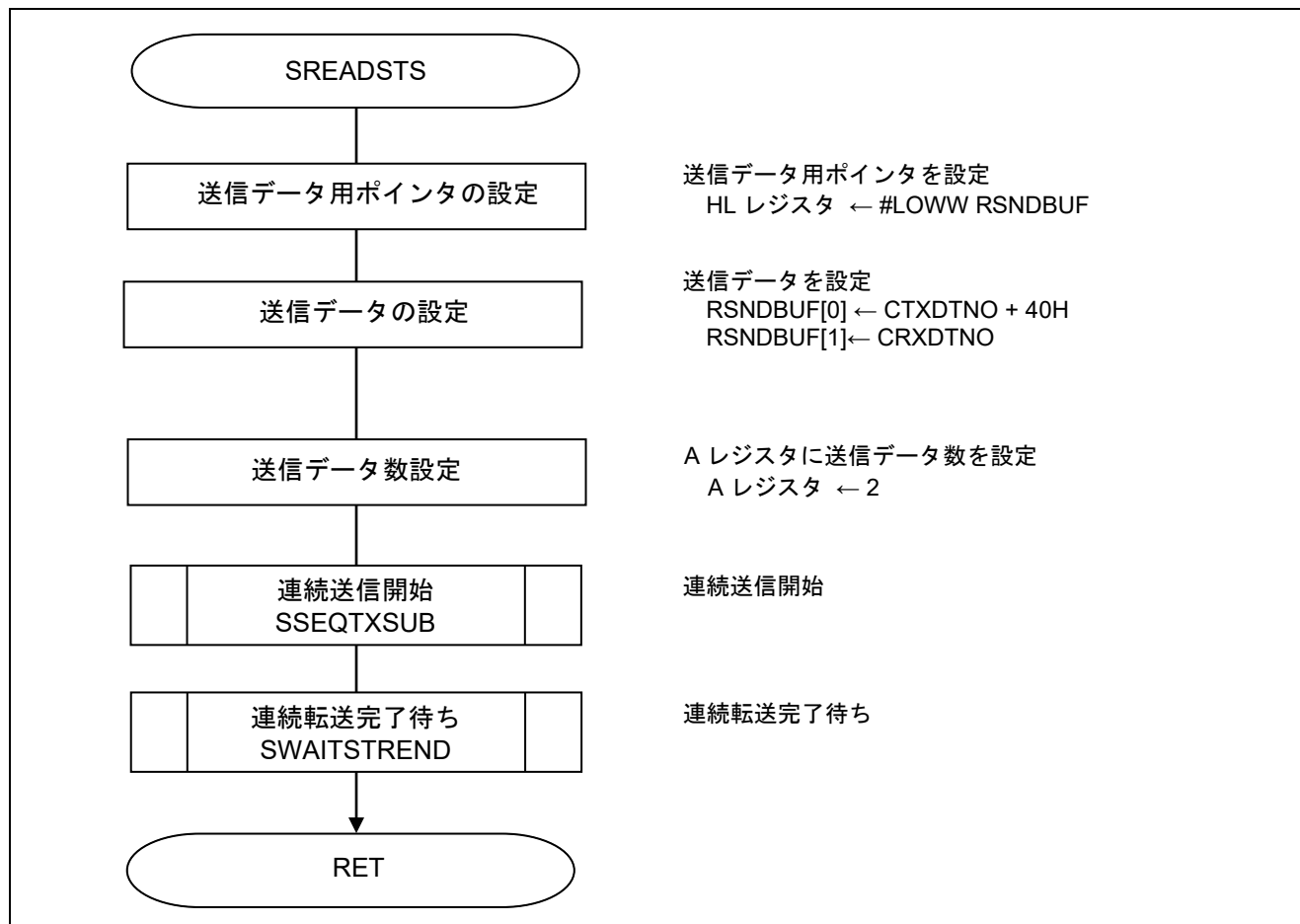
図 5.10 ステータス確認コマンド処理関数
