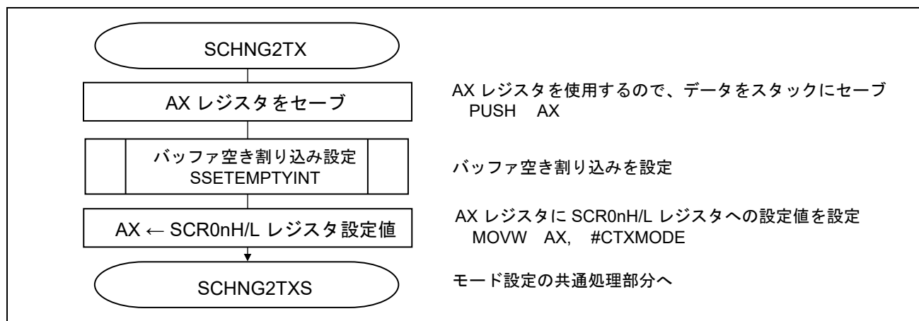
図 5.36 送信モード設定処理
