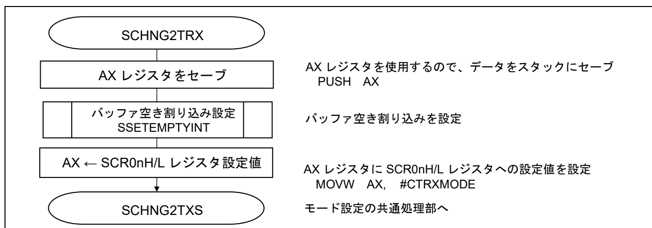
図 5.38 送受信モード設定処理
