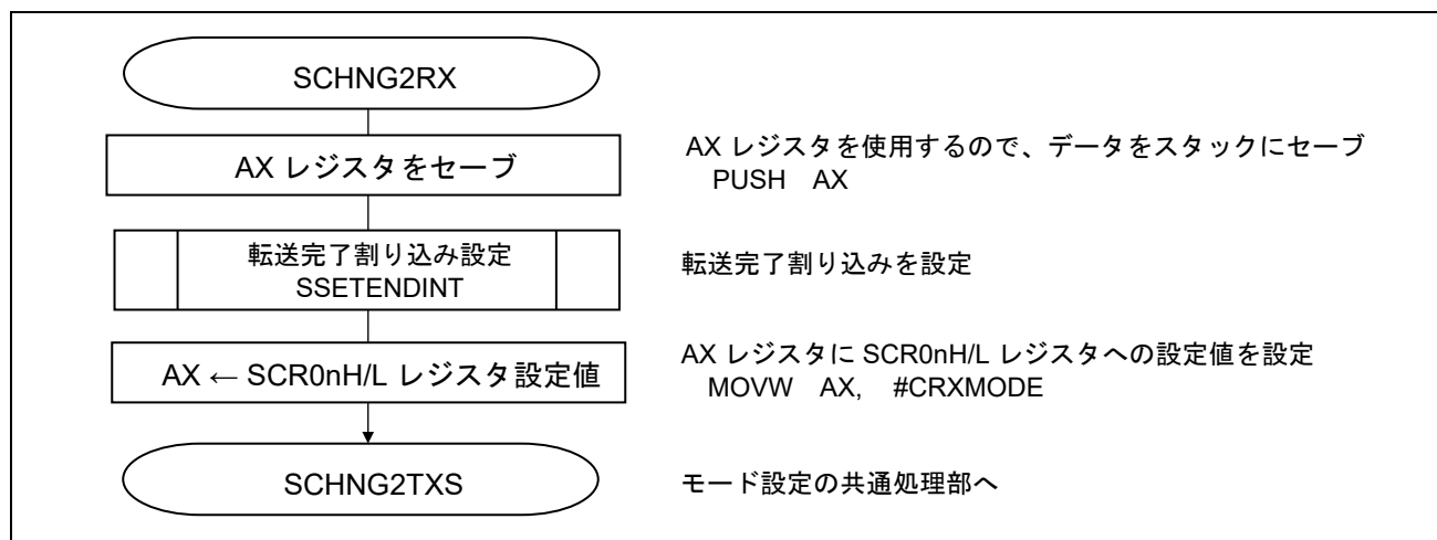
図 5.37 送信モード設定処理
