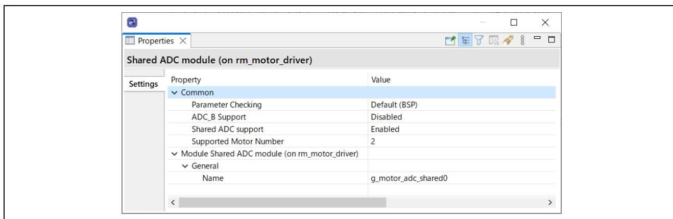
図 2-11 ADC シェアードモジュールの FSP コンフィグレーション
