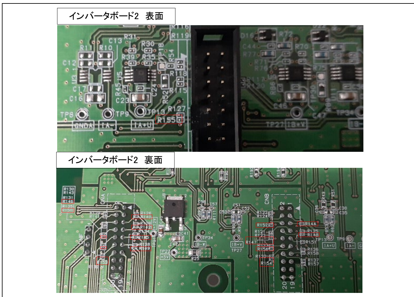
図 2-5 インバータボード2 抵抗実装
