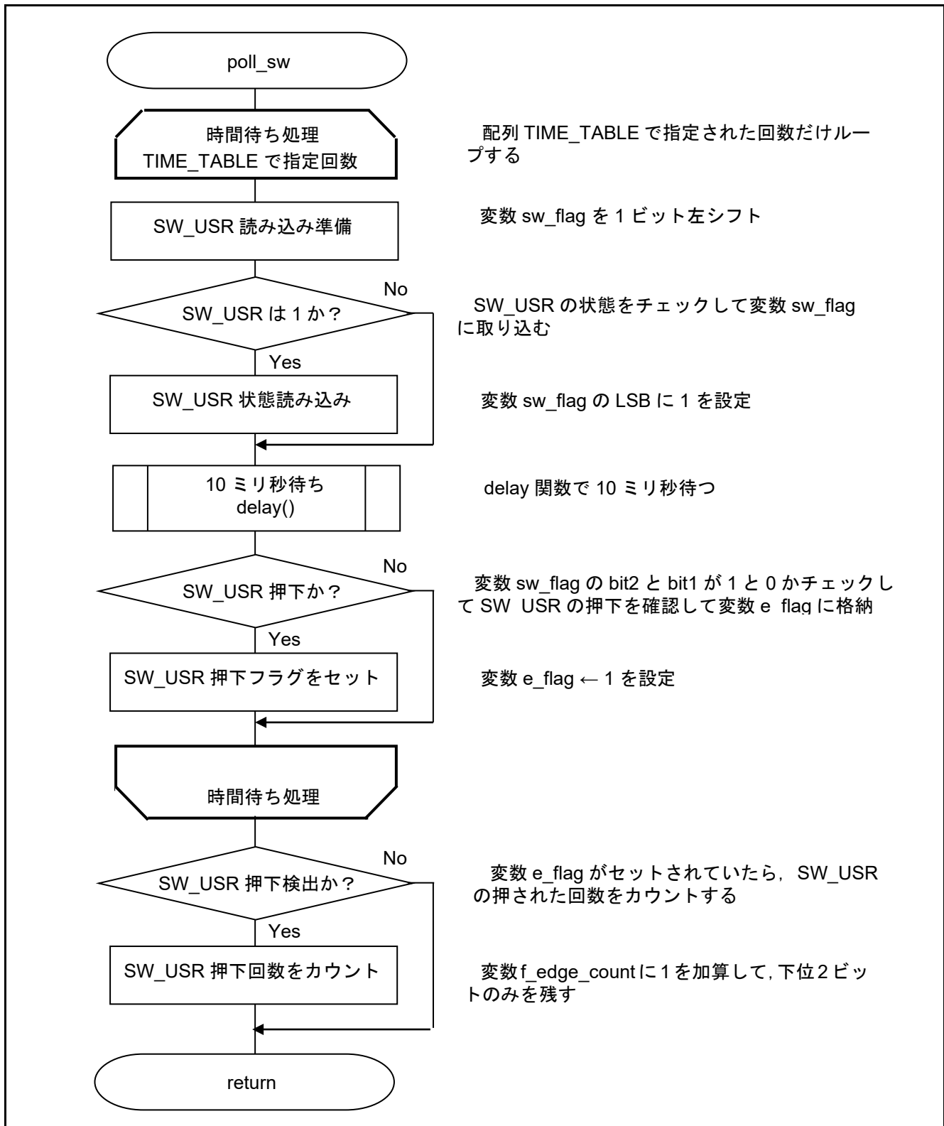
図 5.3 SW_USR チェック及び時間待ち関数
