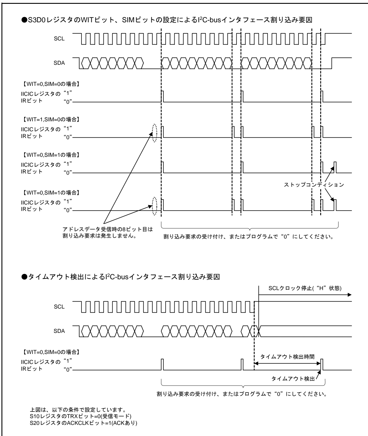
図 6.1 I 2 C-busインタフェース割り込み要求発生タイミング
