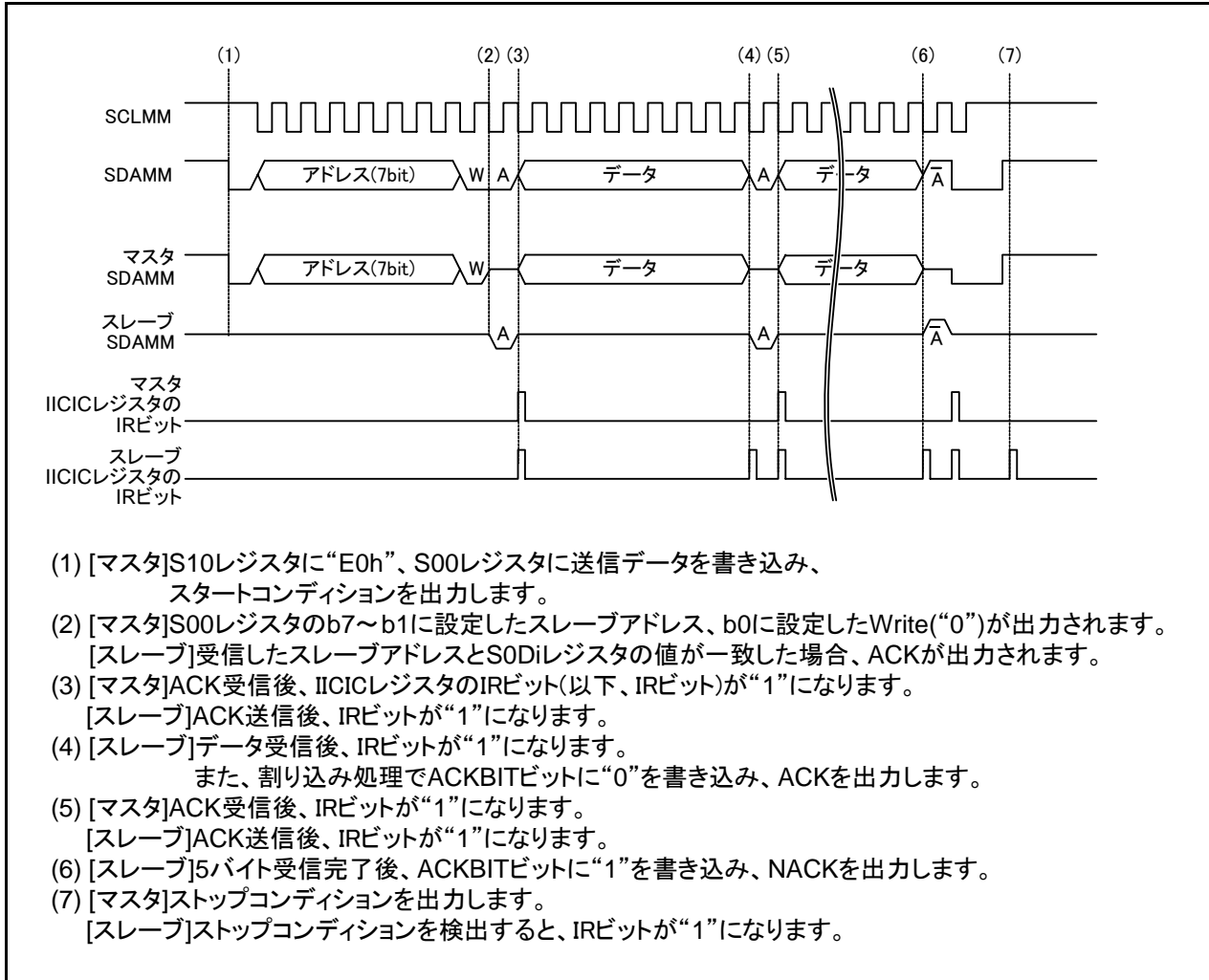
図 8.4 マスタ送信—スレーブ受信の動作例
