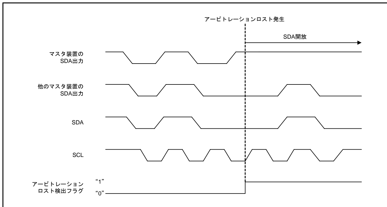
図 5.1 アービトレーションロスト検出フラグの動作タイミング
