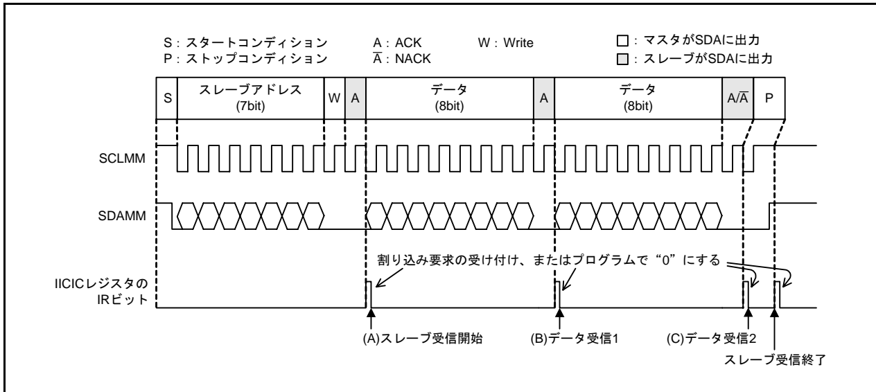
図 4.3 スレーブ受信の動作例
