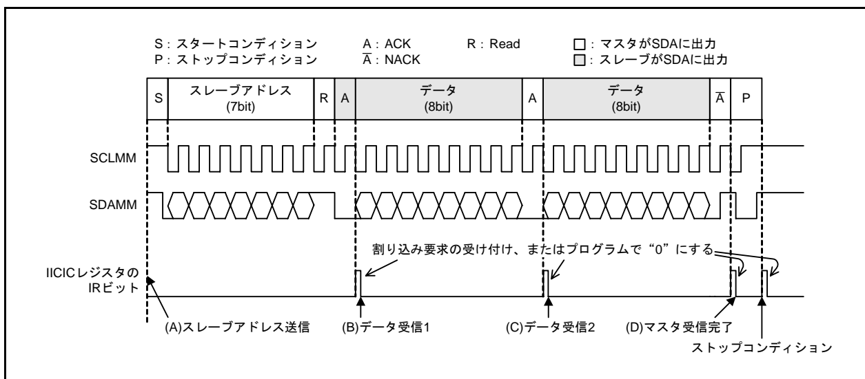
図 4.2 マスタ受信の動作例
