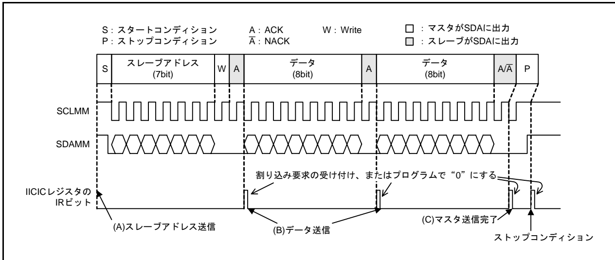
図 4.1 マスタ送信の動作例
