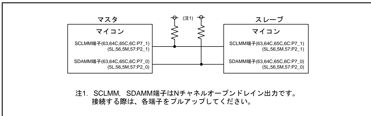
図 8.1 接続例
