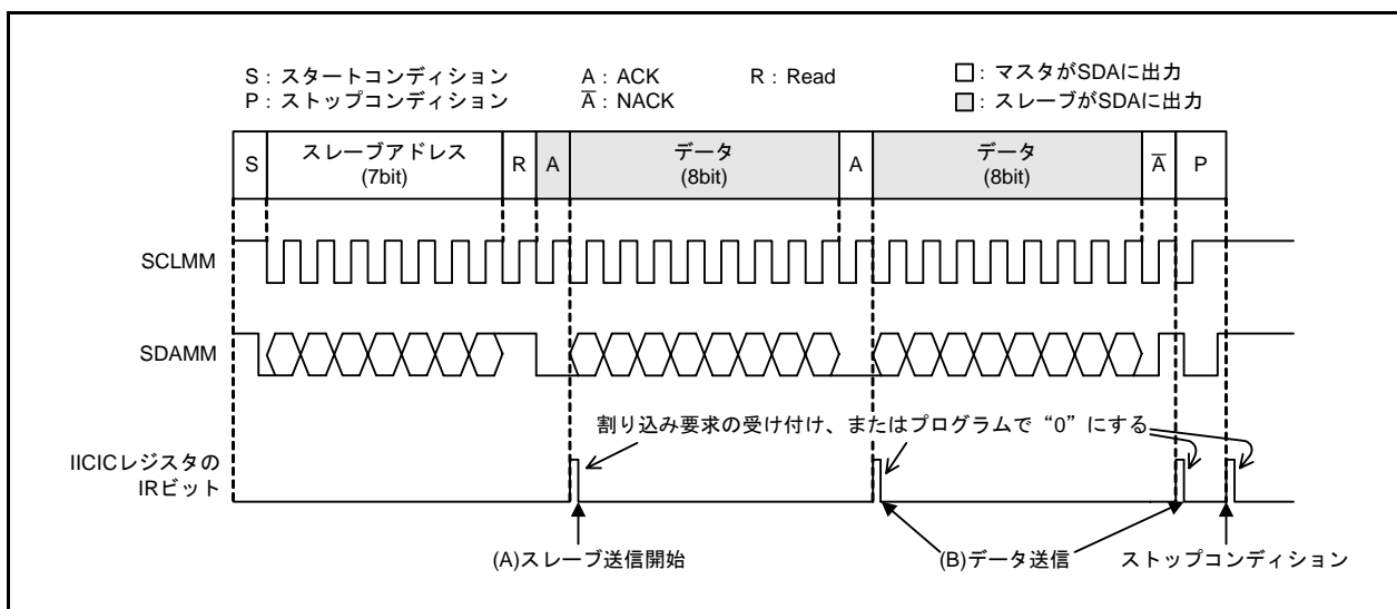
図 4.4 スレーブ送信の動作例
