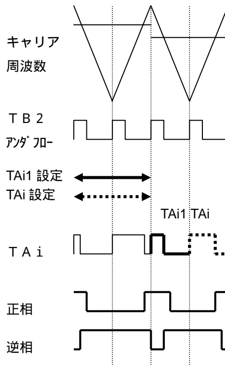
図4.5 三相モード1のTAi、TAi1レジスタの設定と出力の関係
