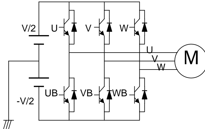
図3.3 パワートランジスタ回路
