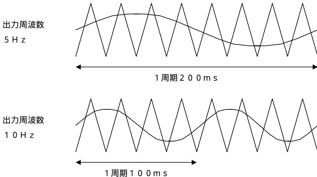
図 5.10 出力周波数の可変
