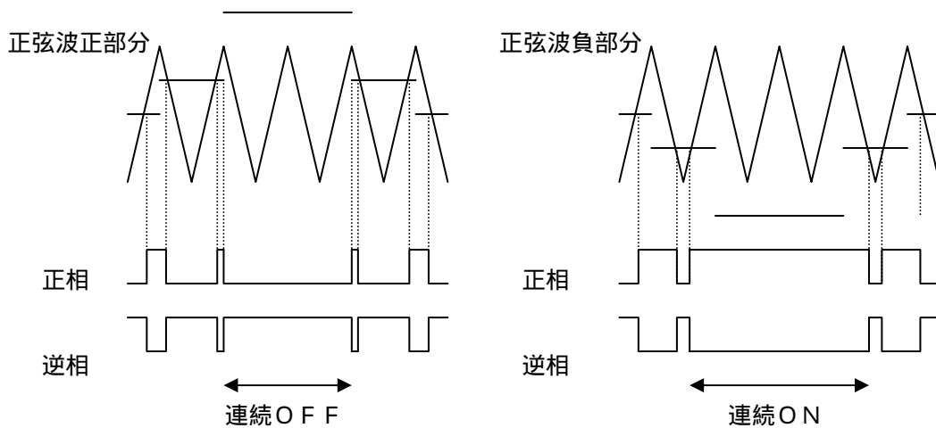
図4.11 二相変調出力のイメージ波形（制御内容は5章）
