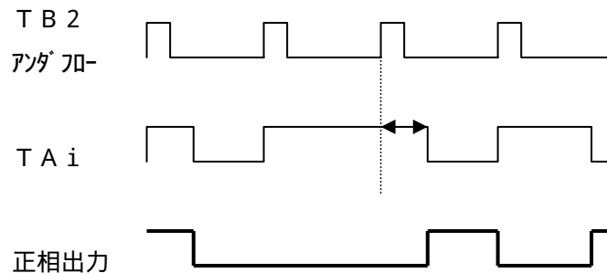
図 4 . 8 T A i > T B 2 設定時の出力波形
