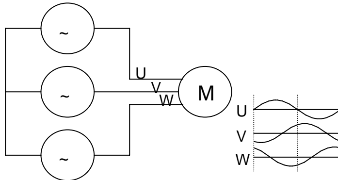
図3.1 三相モータの駆動
