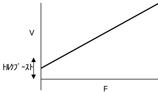
図5.3 V/F制御
