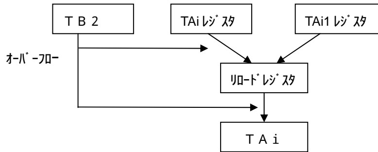
図4.5 三相モード1のTAi、TAi1レジスタの設定と出力の関係
