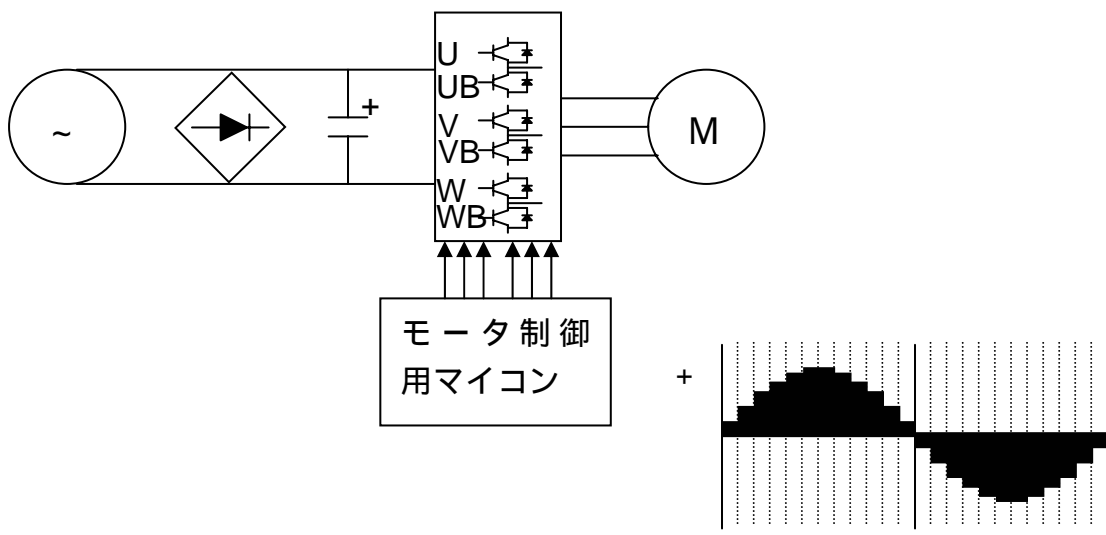
図3.2 マイコンを使用したインバータ制御例
