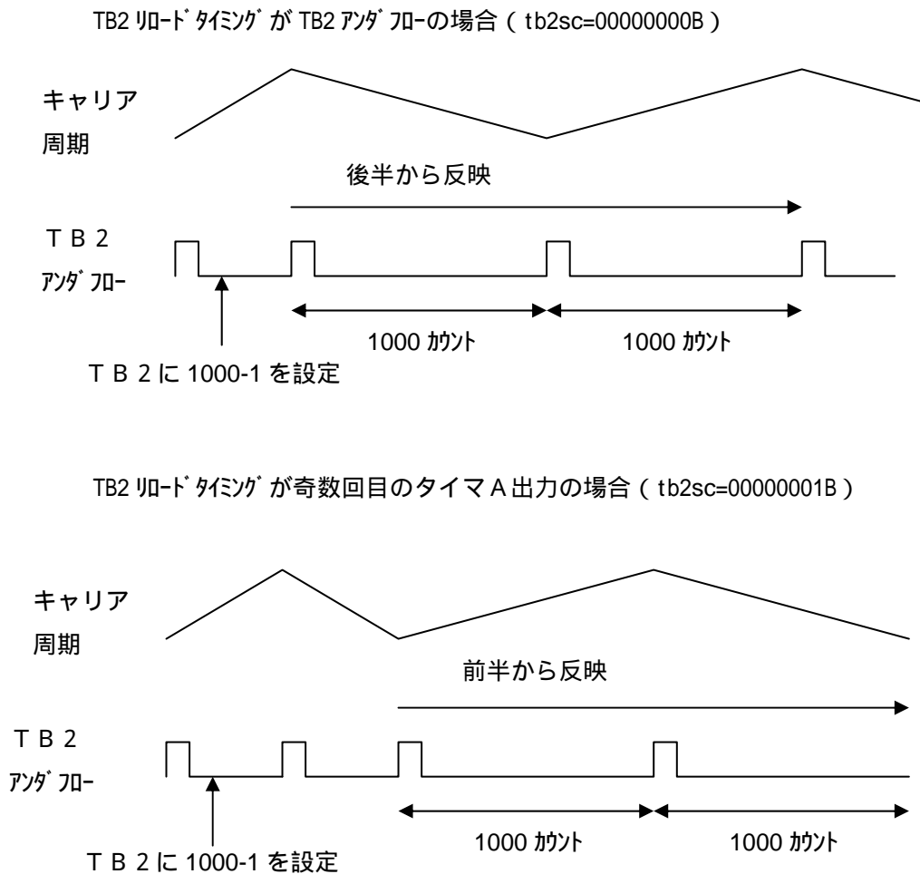
図 4 . 1 0 キャリア周期の設定と反映
