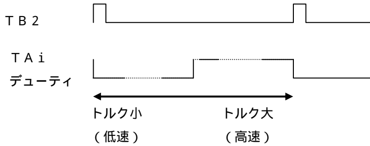
図6.3 トルク指令値とTAiの関係
