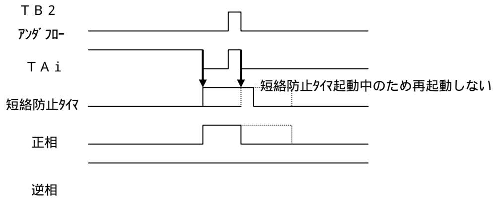
PWMデューティの変化と短絡防止時間
