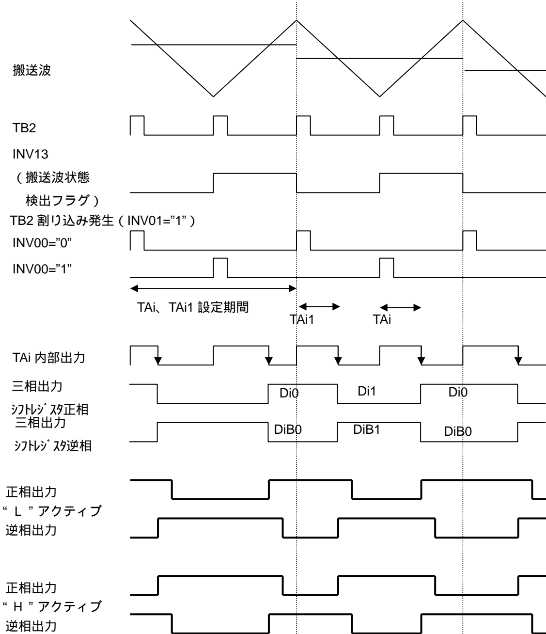
図 4 . 6 三相モード 1 と他設定の関係 ( invc0=*0**11**B; invc1=01****1*B; idb0=00010101B; idb1=00101010B )
