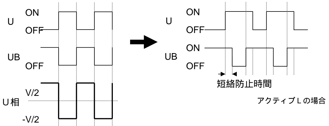
図3.4 マイコンの出力波形と生成される波形
