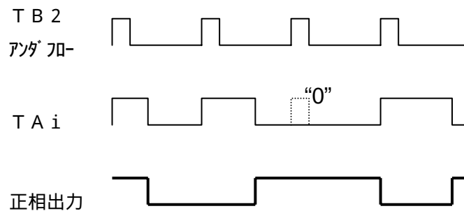
図 4 . 7 T A i = 0 設定時の正相波形
