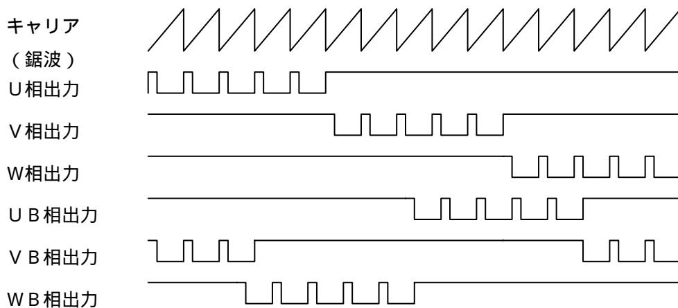
図4.12 120°通電出力のイメージ波形（制御内容は6章）
