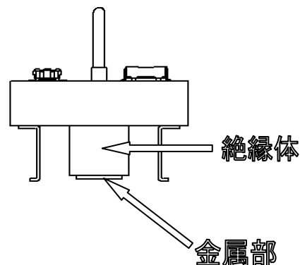
図2-4 TC突起図
