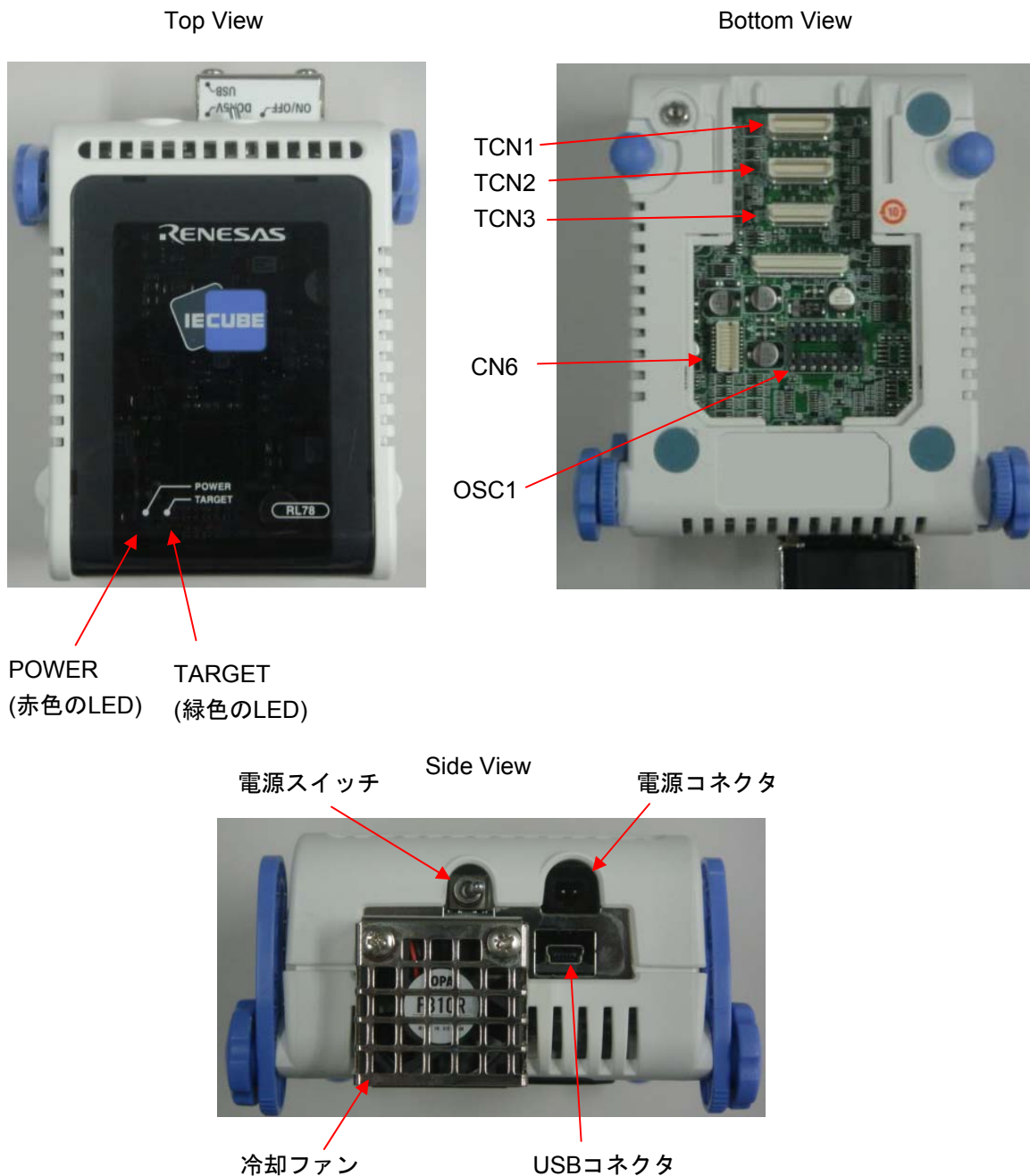
図1-1 QB-RL78L12の各部の名称
