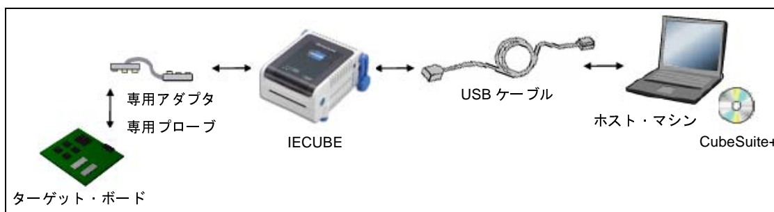
図 2—1 ホスト・マシンとデバッグ・ツールとの接続例【IECUBE】
