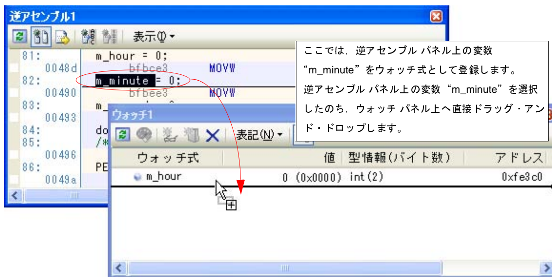
図 2—114 他のパネルからウォッチ式登録する場合の例
