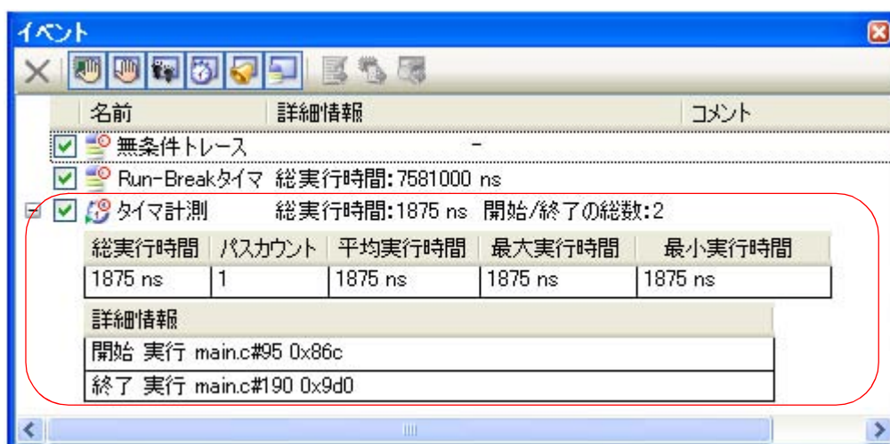
図 2—133 タイマ計測イベント（タイマ開始イベント／タイマ終了イベント）の測定結果例
