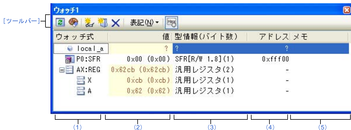
図 A—27 ウォッチパネル
