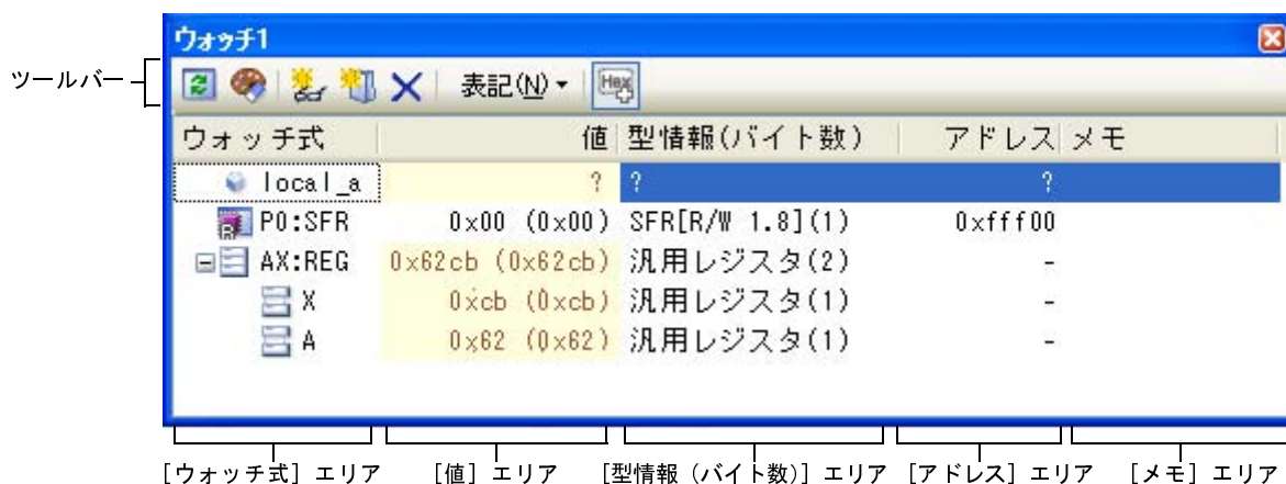
図 2—113 ウォッチ式の内容の表示 (ウォッチパネル)
