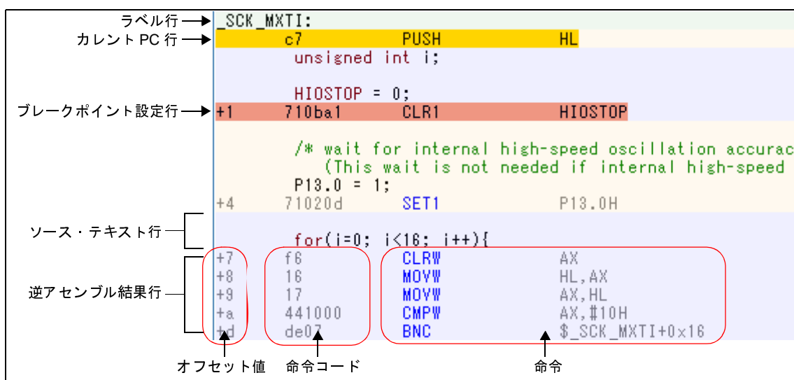
図 A—23 逆アセンブル・エリアの表示内容（混合表示モードの場合）
