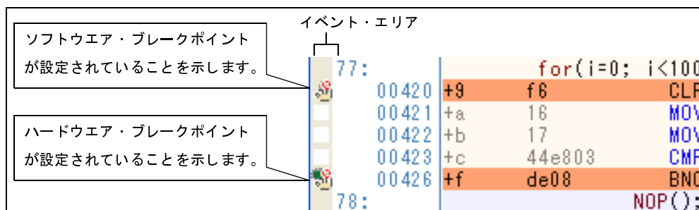
図 2—96 ブレークポイントの設定例（逆アセンブルパネルの場合）
