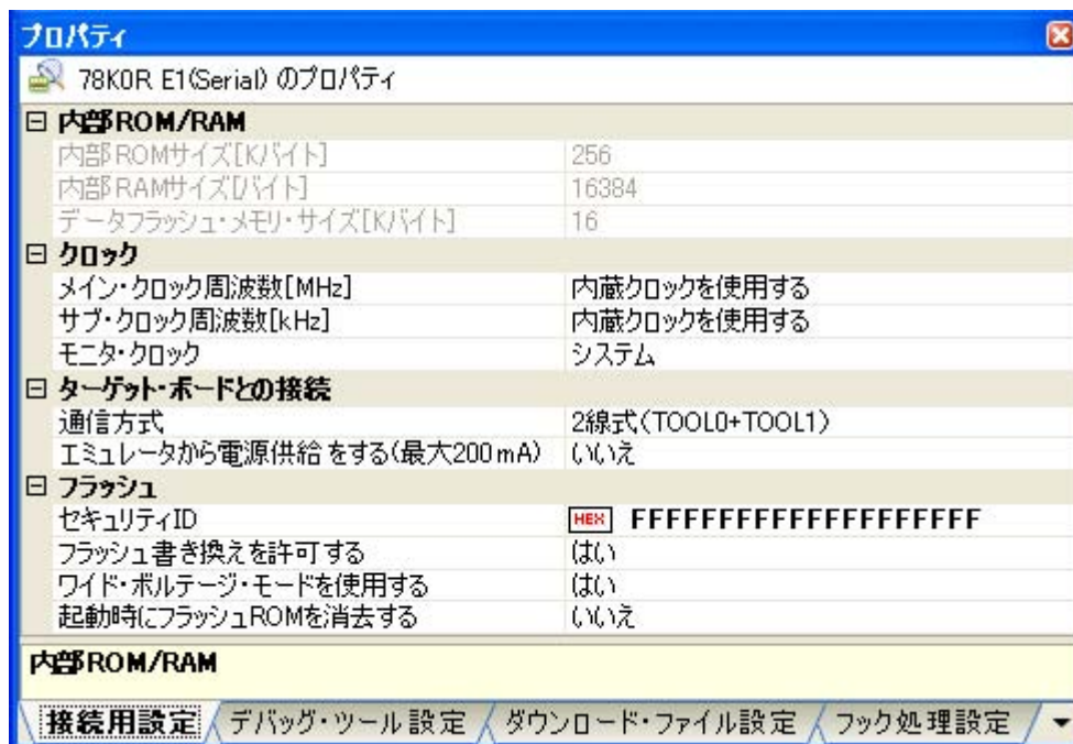
図 2—34 動作環境設定【E1】（プロパティ パネル）
