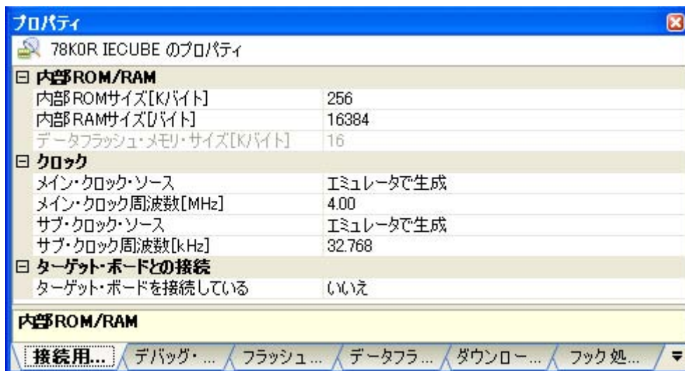
図 2—8 動作環境設定【IECUBE】（プロパティパネル）
