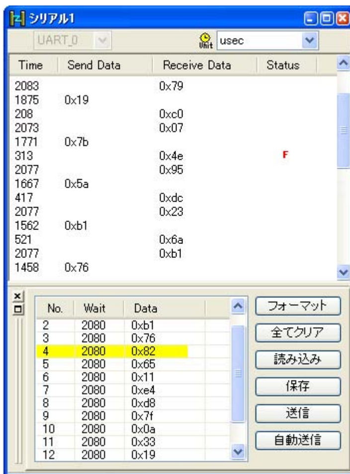
図 2—150 シリアル通信を行う（シリアル ウィンドウ）
