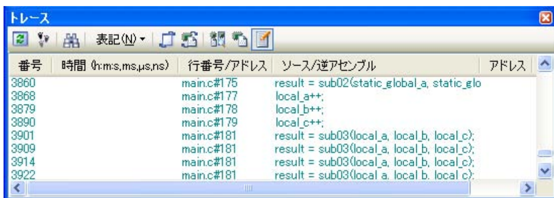
図 2—124 ソース表示モードの例（トレース パネル）
