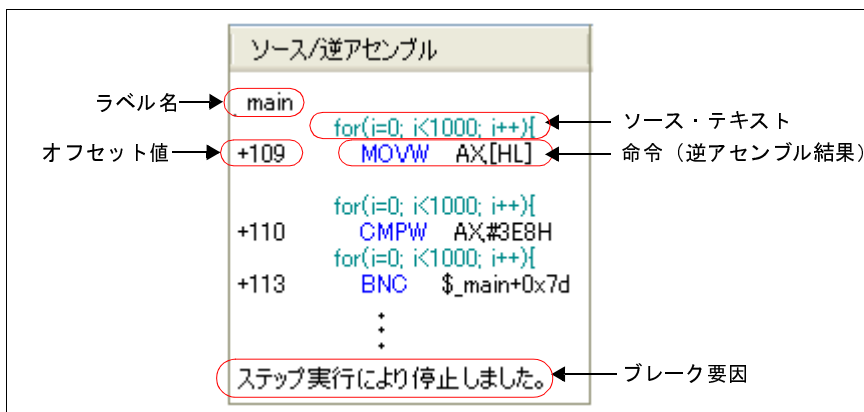
図 A—30 [ソース/逆アセンブル] エリアの表示内容（デフォルト）
