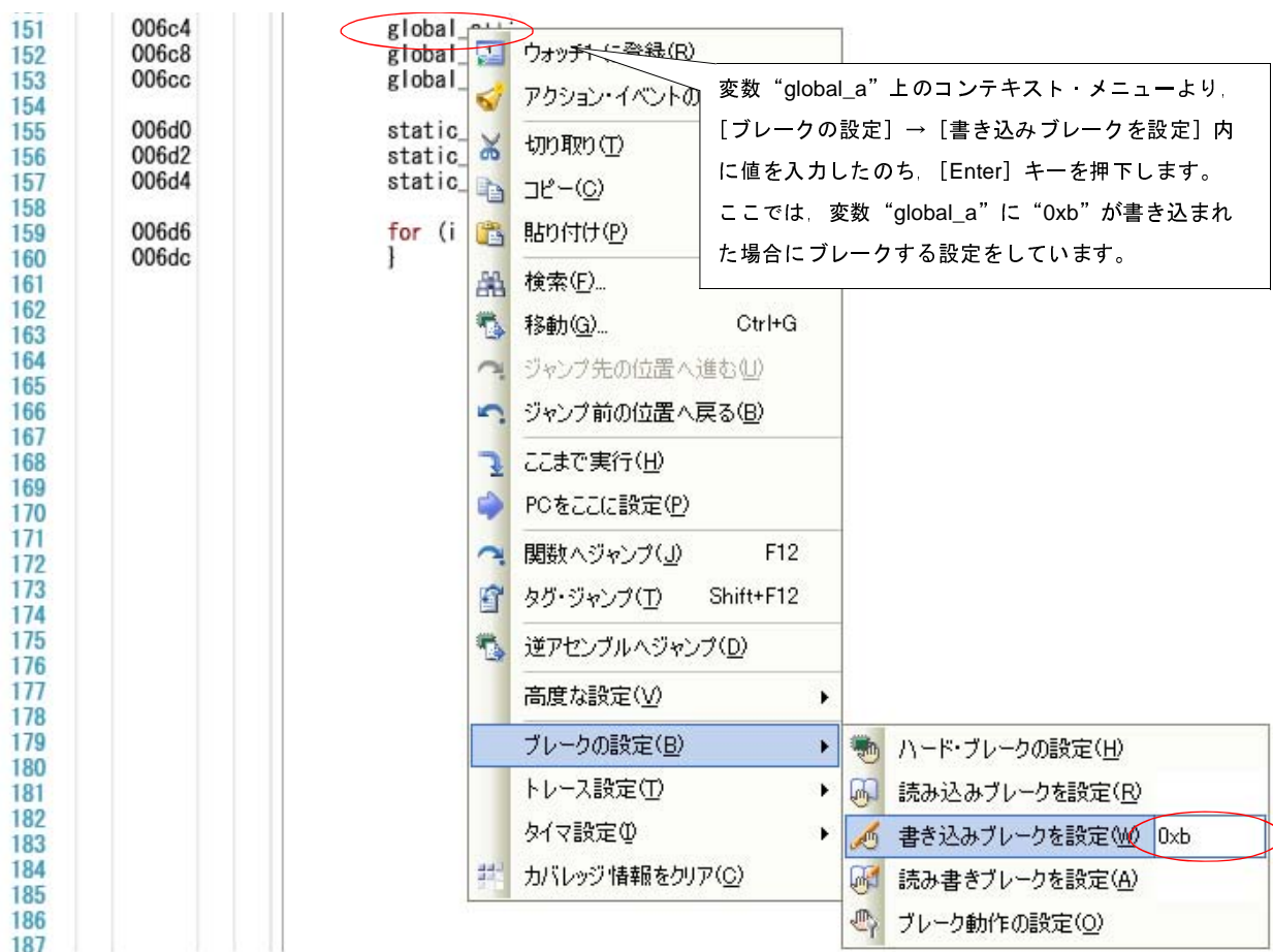
図 2—97 ソース・テキスト上の変数に対するブレーク・イベントの設定例
