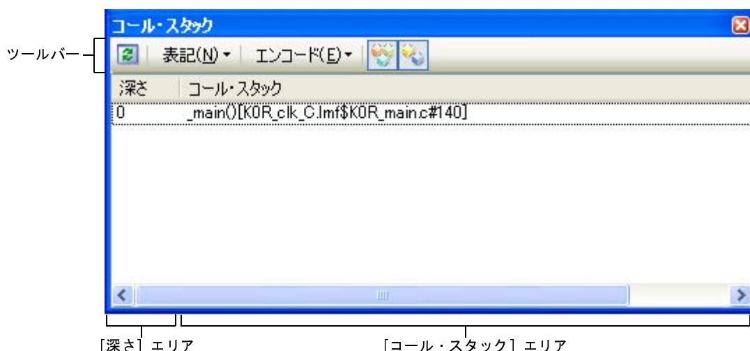
図 2—117 コール・スタック情報の表示 (コール・スタック パネル)
