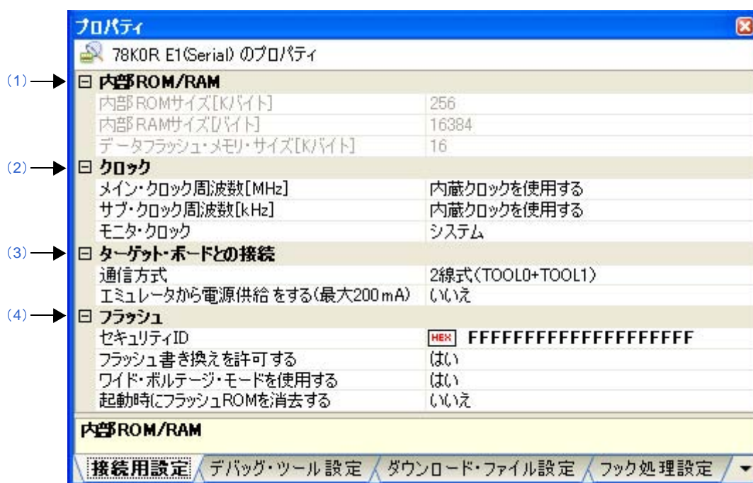
図 A—7 プロパティ パネル : [接続用設定] タブ【E1】
