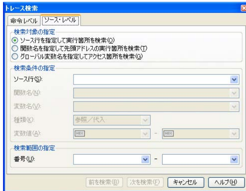
図 2—127 ソース・レベルでのトレース・データの検索
