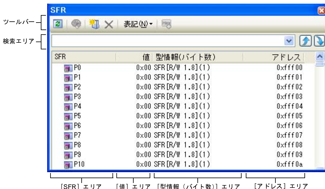
図 2—109 SFR の内容の表示 (SFR パネル)
