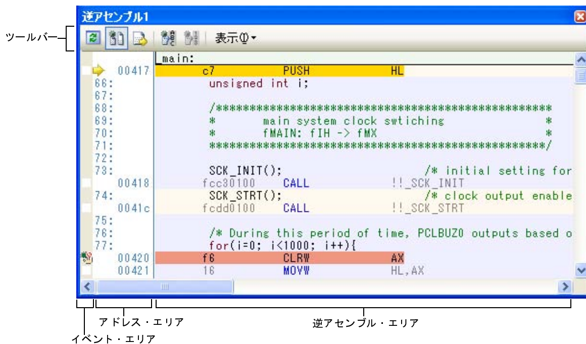
図 2—86 逆アセンブル結果の表示（逆アセンブルパネル）
