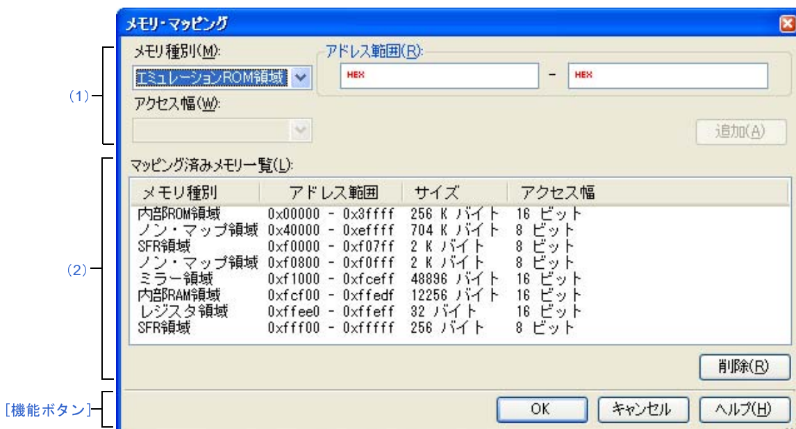
図 A—34 メモリ・マッピング ダイアログ 【(シミュレータ)】
