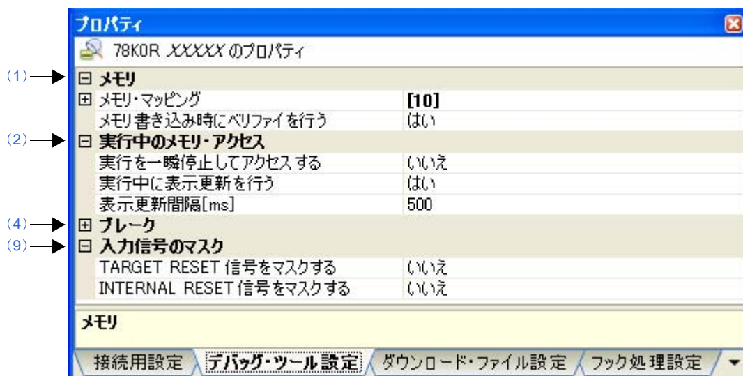
図 A—10 プロパティパネル：[デバッグ・ツール設定] タブ【MINICUBE2】[E1] [E20] [EZ Emulator]
