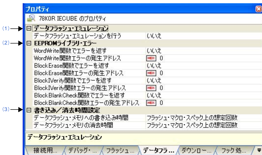
図 A—13 プロパティ パネル：[データフラッシュ・エミュレーション設定] タブ
