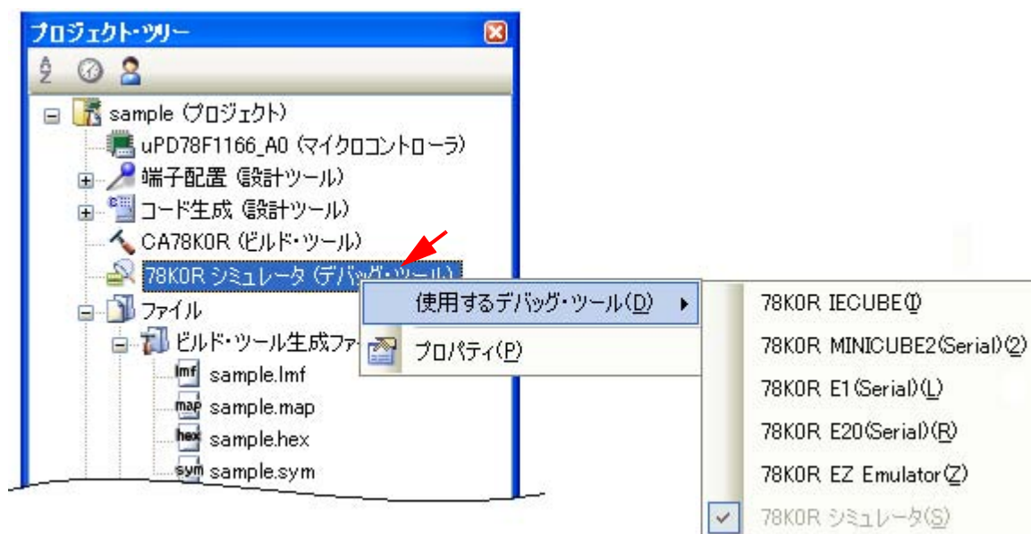
図 2-7 使用するデバッグ・ツールの選択/切り替え
