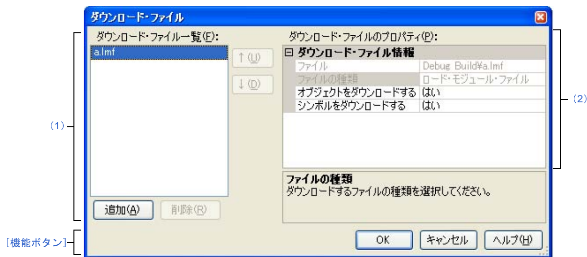
図 A—35 ダウンロード・ファイル ダイアログ
