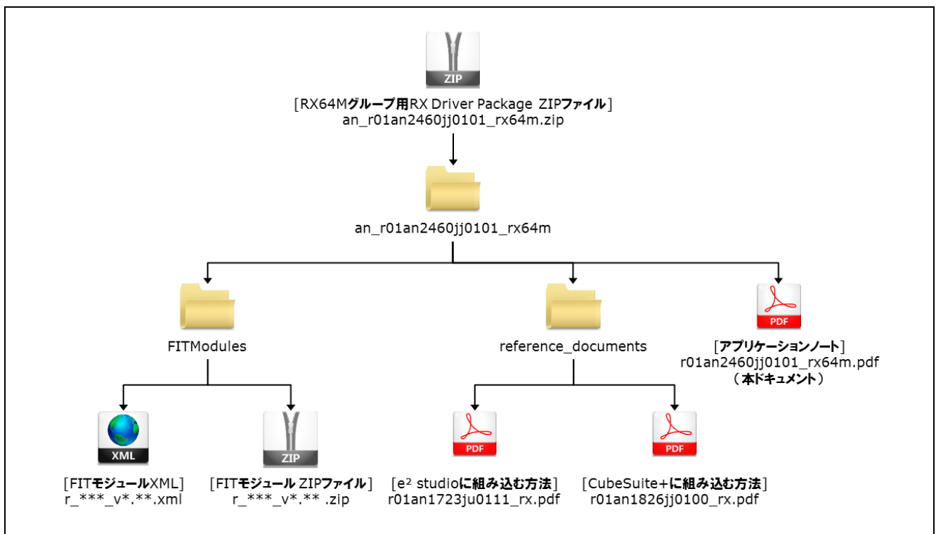
図3.1.1 RX64M グループ用 RX Driver Package フォルダ構成
