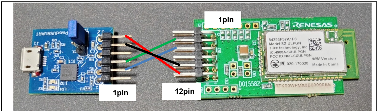
図 4.5 DIGILENT Pmod USBUART と SX-ULPGN の接続
