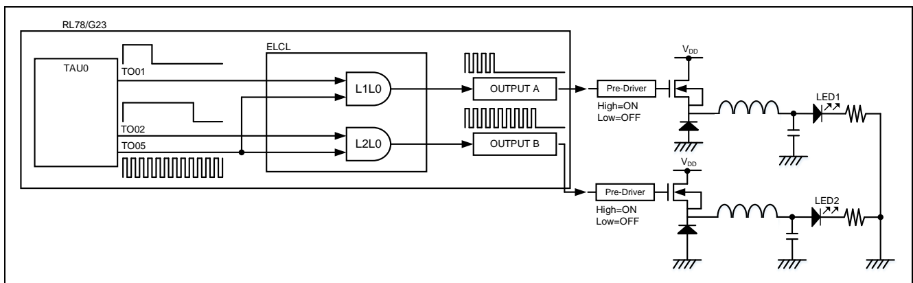
図 1-1 システム構成
