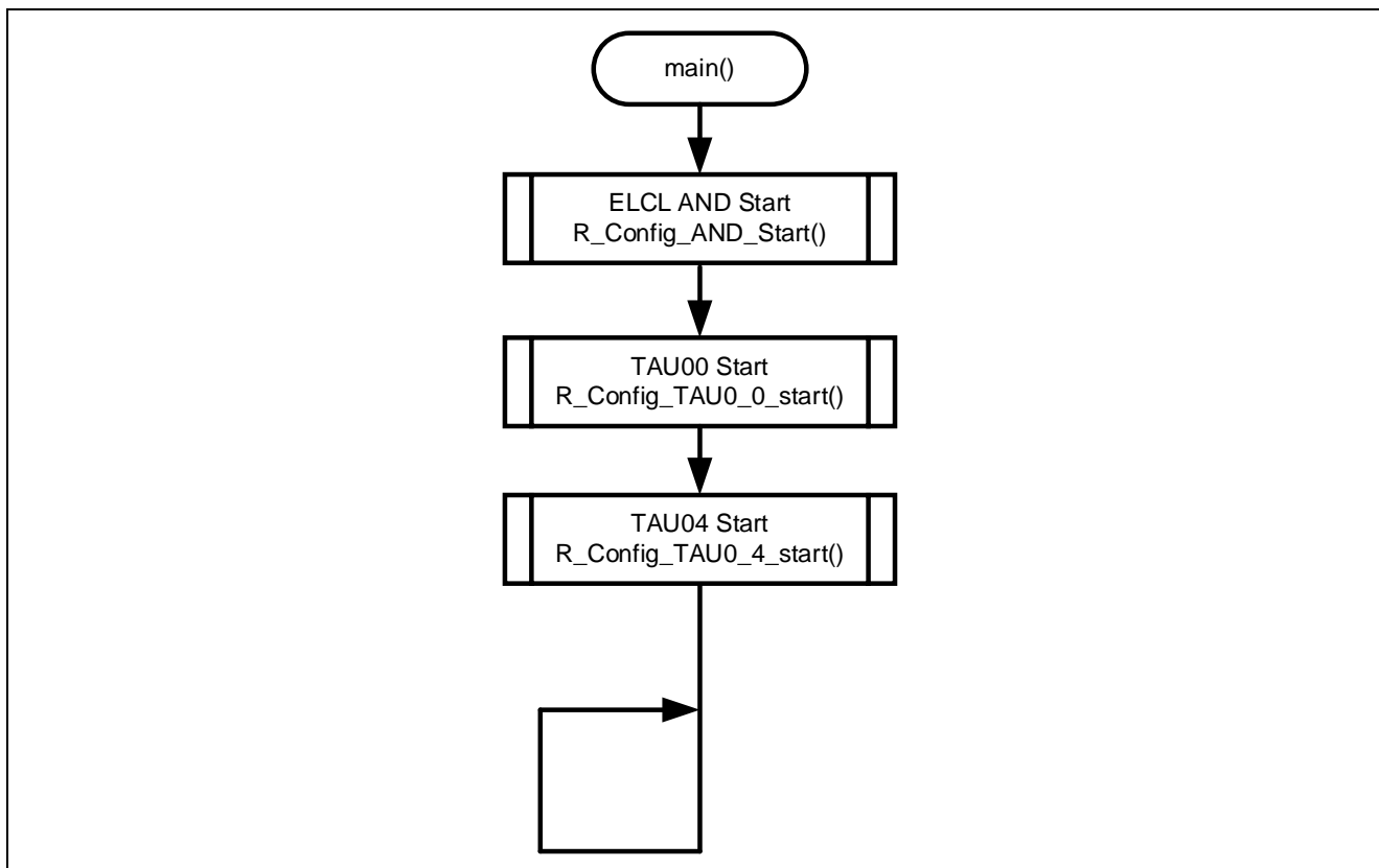
図 4-2 メイン処理
